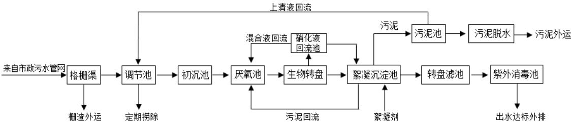
图8 污水处理厂污水处理工艺流程图
