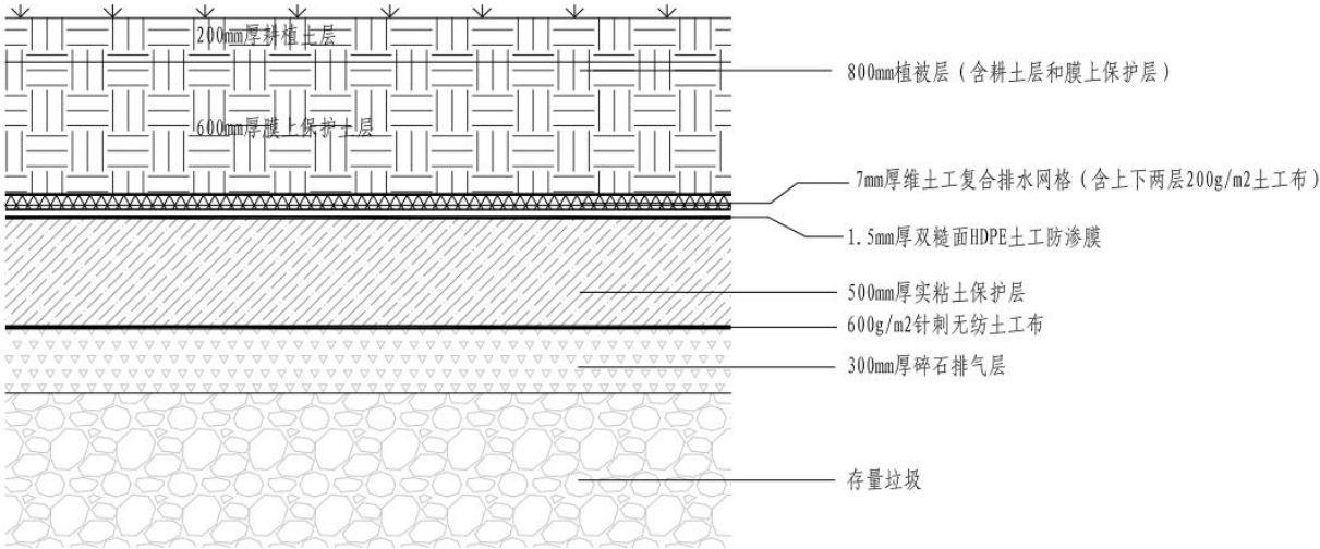
图 1-2 封场覆盖系统结构示意图
