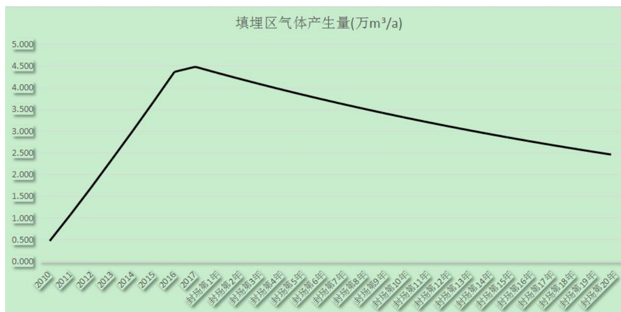
图 5-3 填埋气体产生量与填埋时间关系图
