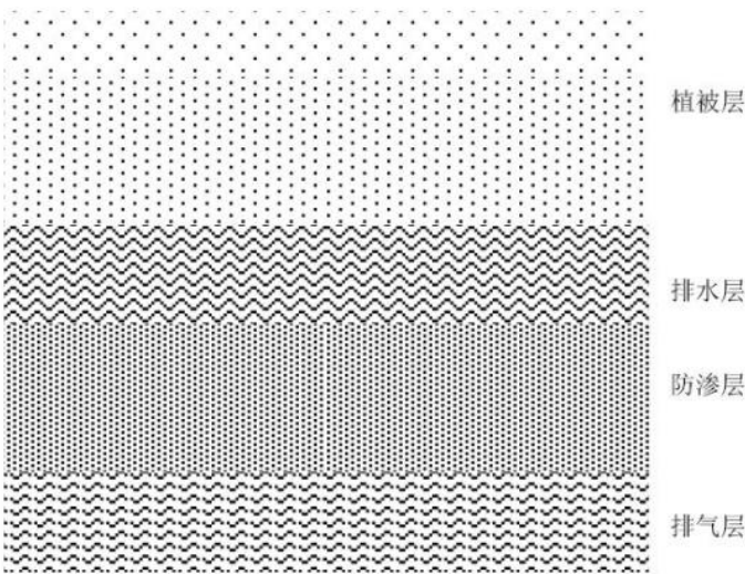
图 1-1 堆体表面覆盖构造图
