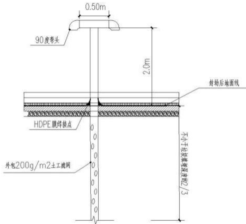
图 1-2 填埋气井样图
