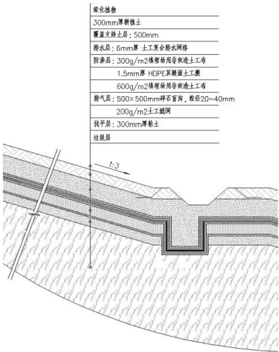
图 1-1 就地封场系统结构图
