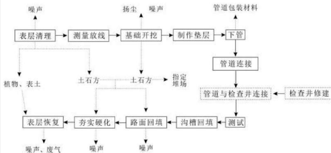
图 5 工程配套管网工艺流程
