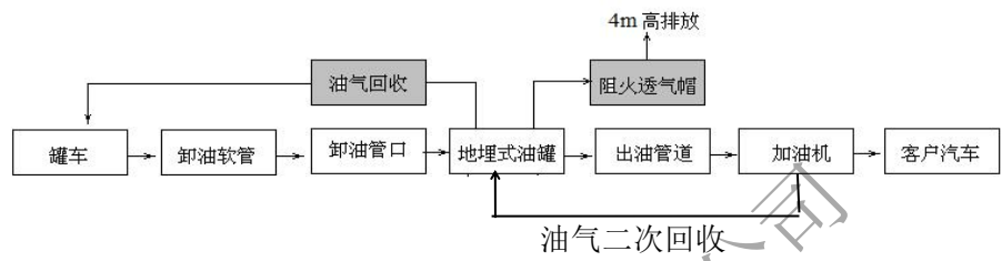
图 6 工艺流程图
