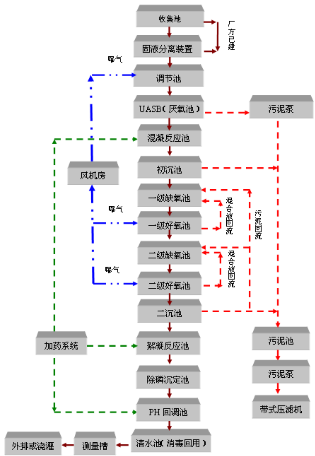
图1 本项目污水处理工艺流程图
