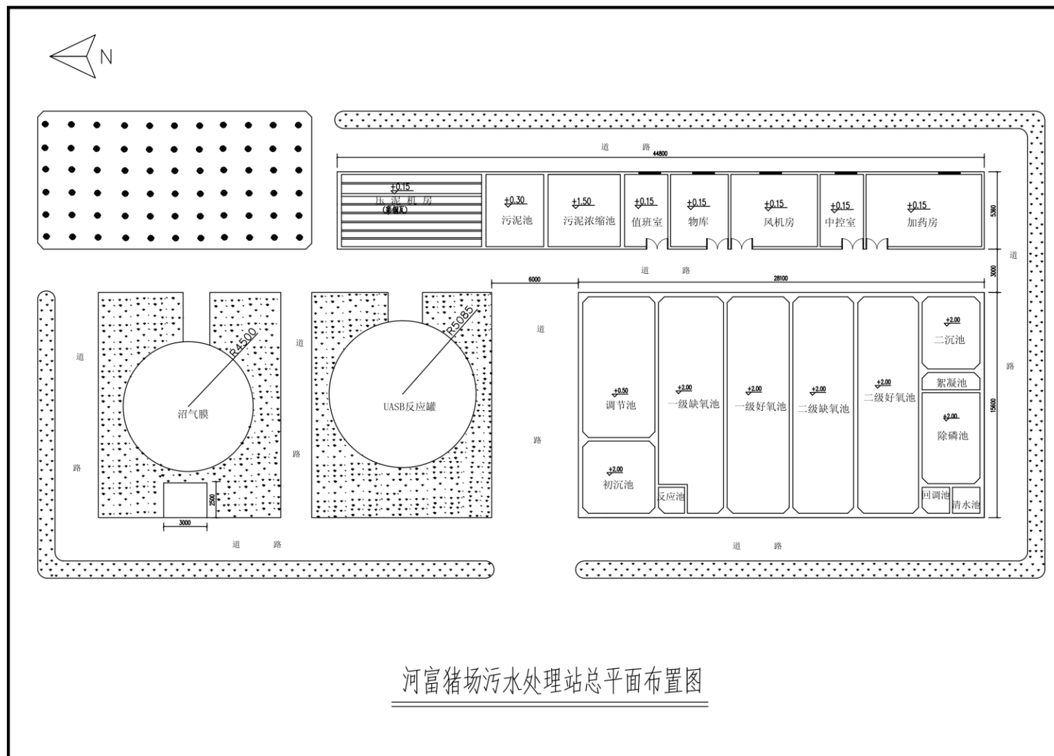
附图四 项目污水处理站总平面布置图
