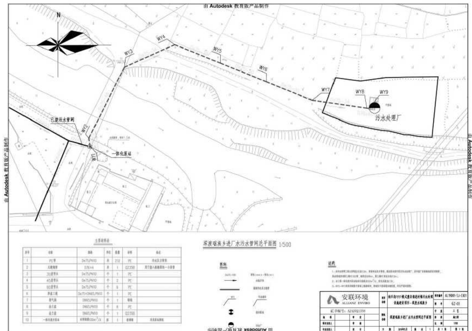
图 4 项目管网平面布置图
