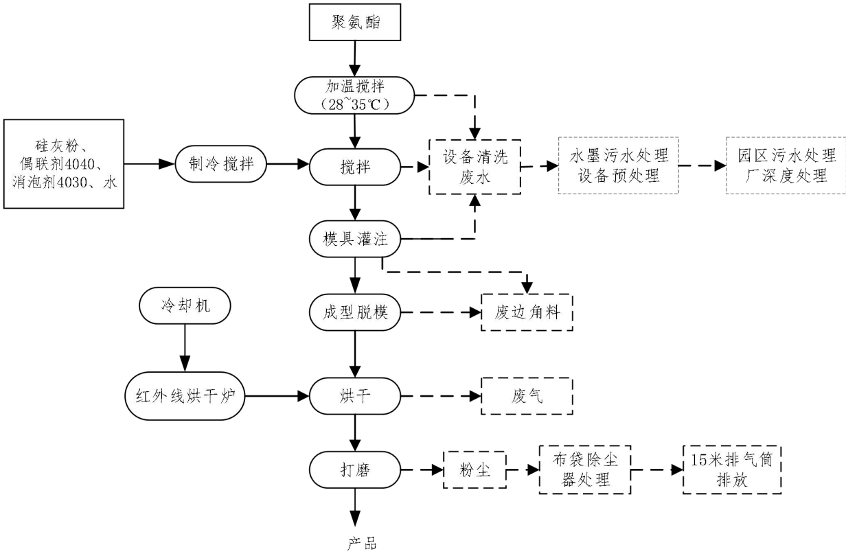
图 5-1 项目粉扑产品生产工艺流程图
