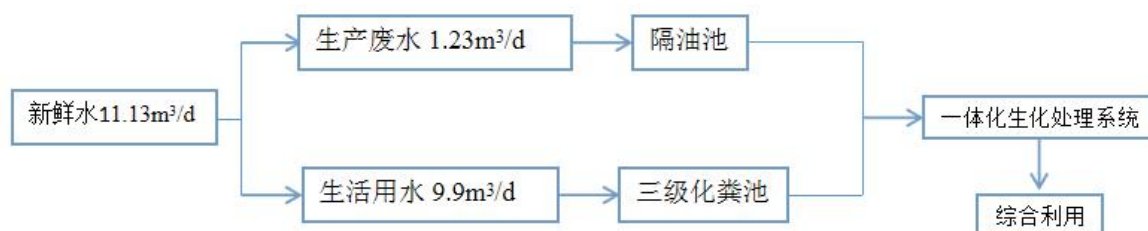
图 2-6 水平衡图
