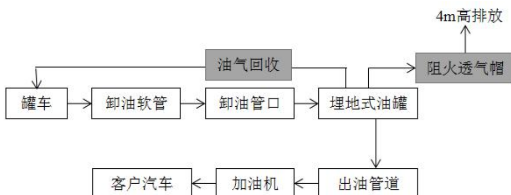
图 2-7 工艺流程图
