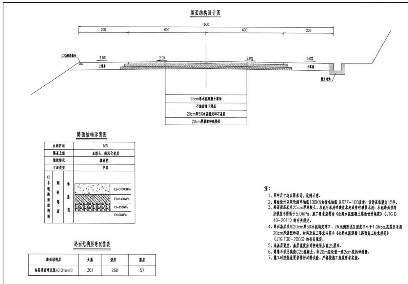
图 3 南韶高速公路总甫口至心泉谷公路改建工程路面结构示意图
