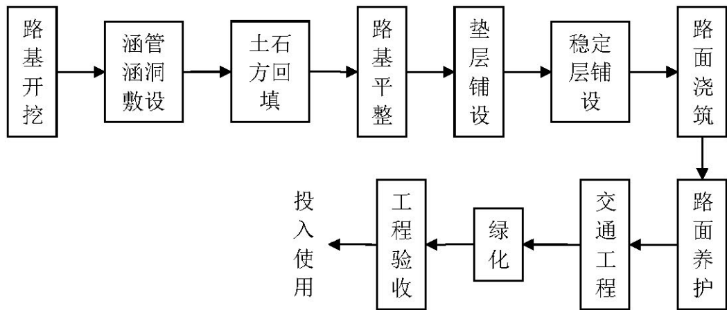
图 4 道路建设项目工艺流程图
