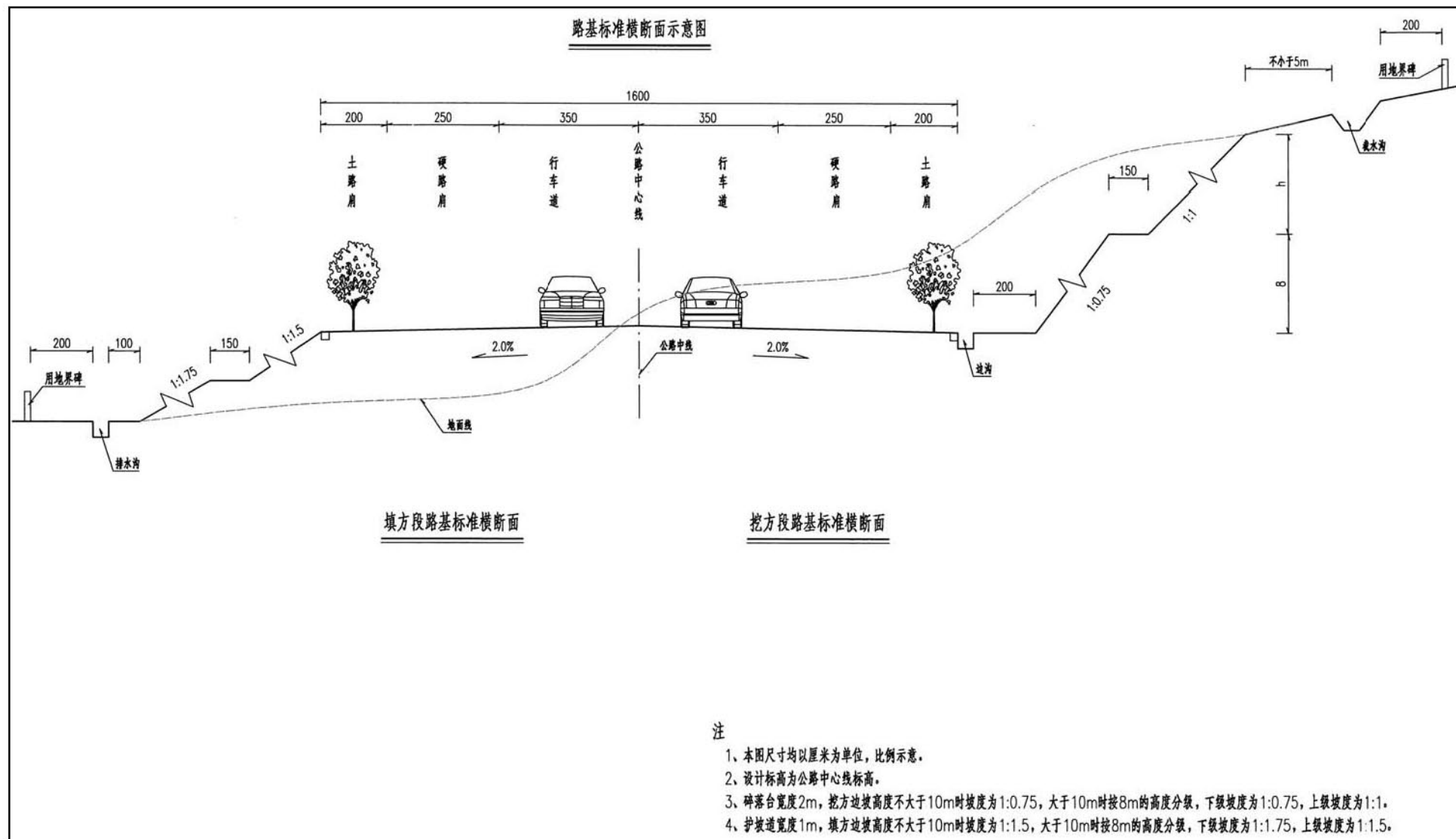
图2 南韶高速公路总甫口至心泉谷公路改建工程横断面设计图
