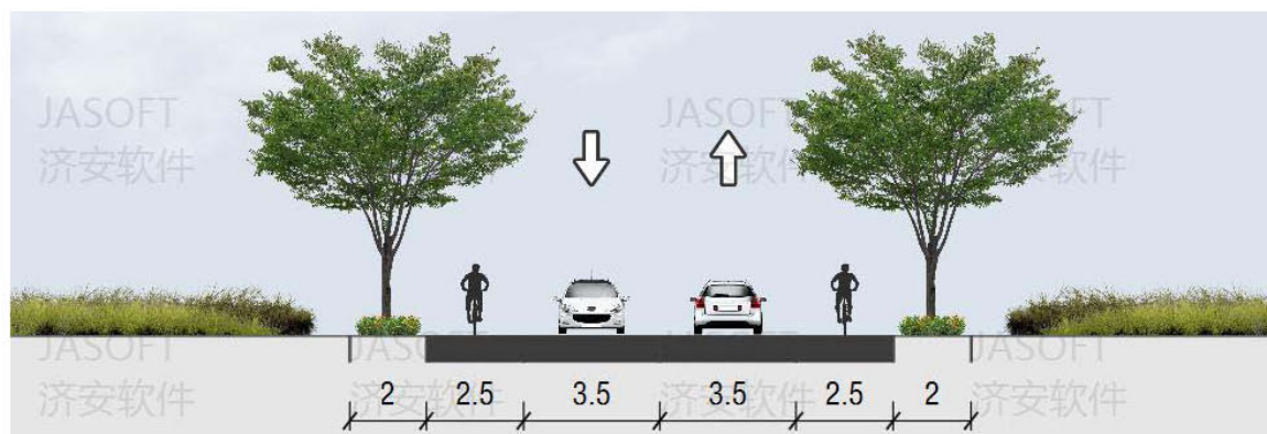
图1 标准横断面效果图
