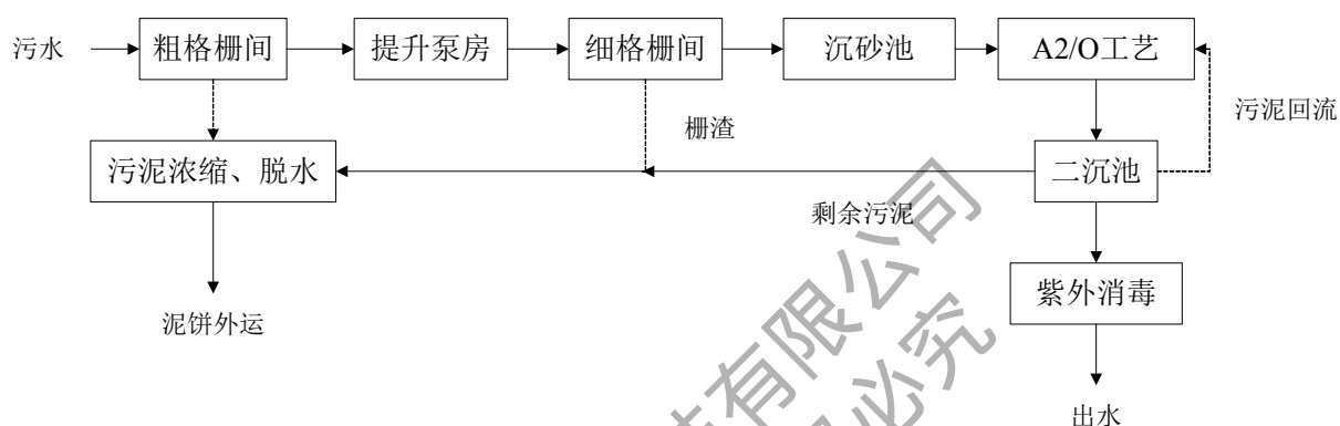
图 7-3 始兴县污水处理厂工艺流程图
