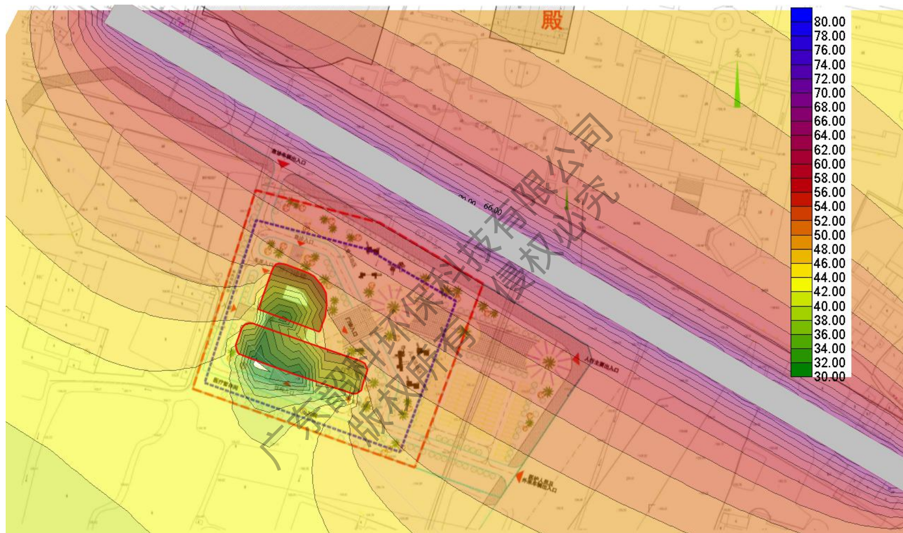
图 6-2 省道 343 线本项目构筑物噪声预测图（夜间 dB（A））
