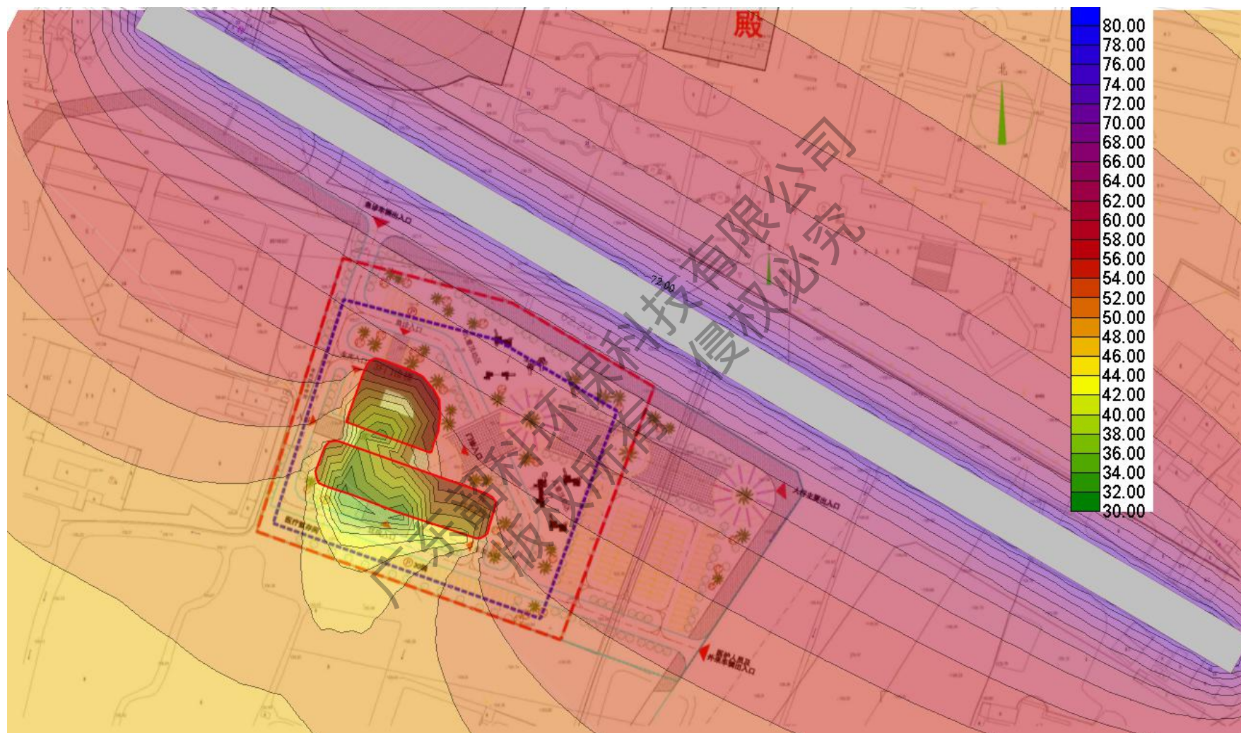
图 6-1 省道 343 线到本项目构筑物噪声预测图（昼间 dB（A））
