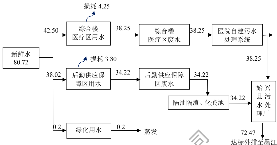
图 3-7 医院水平衡图 (单位: \text{m}^3/\text{d} )
