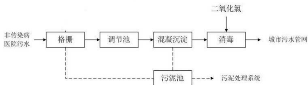
图 7-1 本项目污水处理系统处理工艺流程
