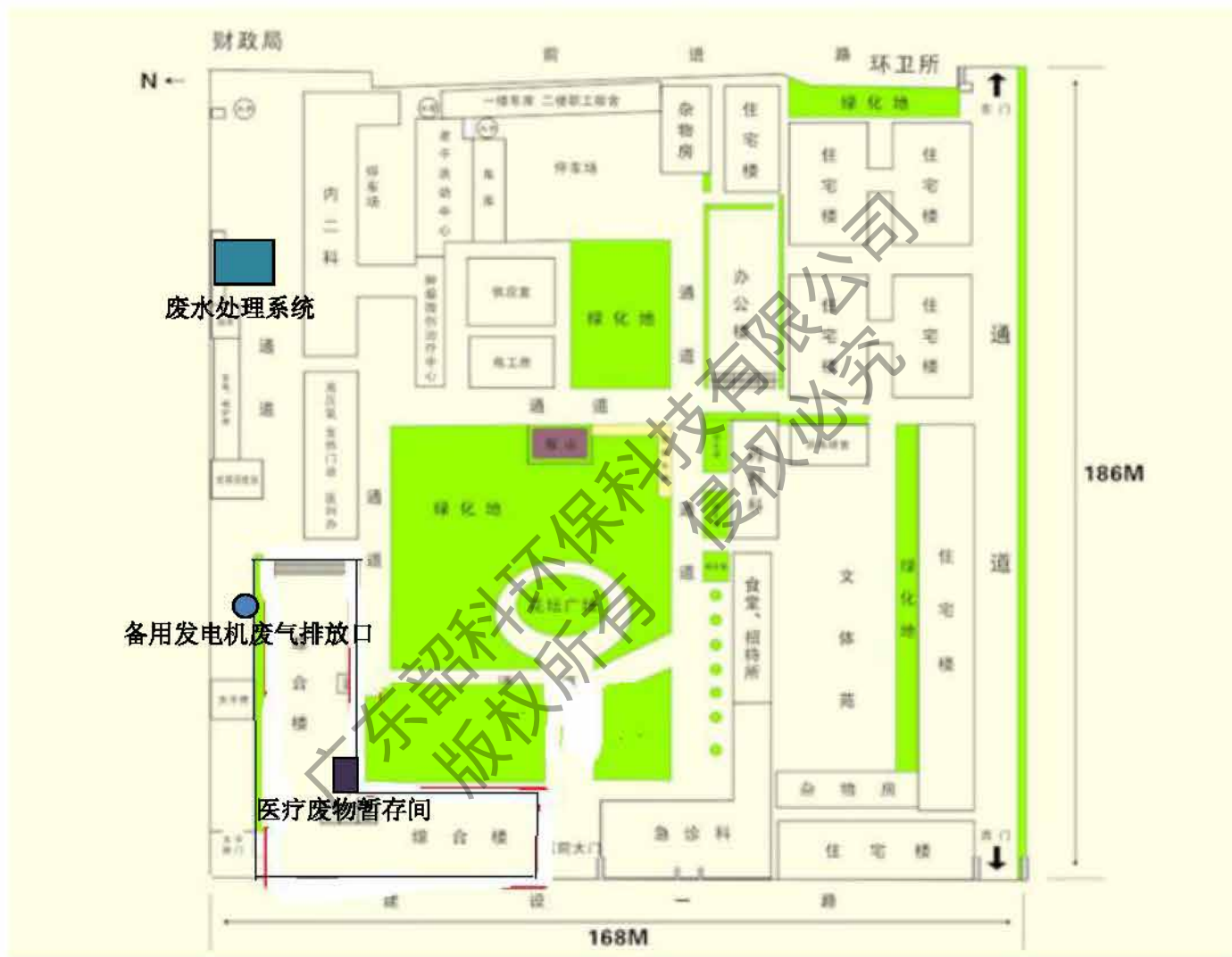
图4 现有工程平面布置图
