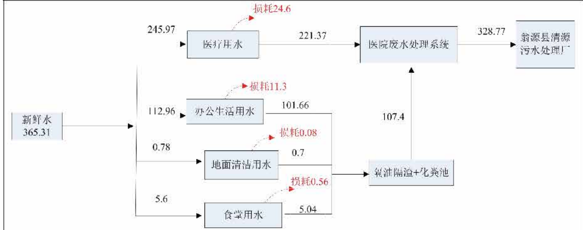
图10 现有工程水平衡图 (单位: m³/d)
