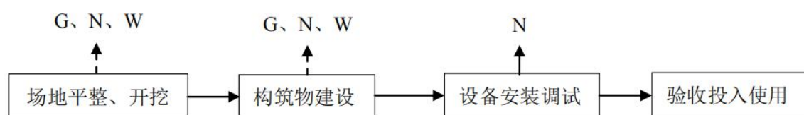
图 5-2 净水厂、取水坡头 施工工艺及产污节点图
