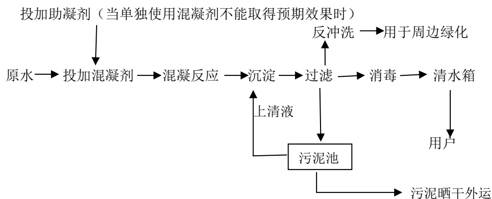
图 5-3 净水厂净水工艺
