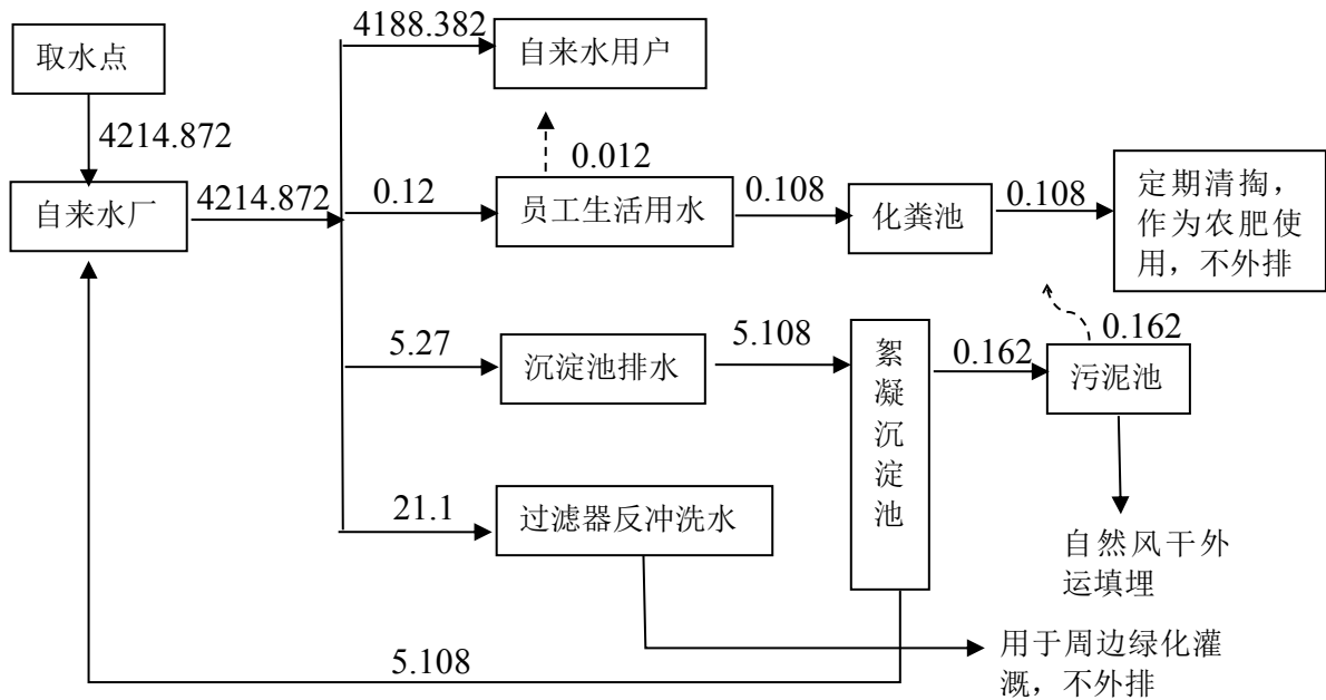
(3) 本项目水平衡图
