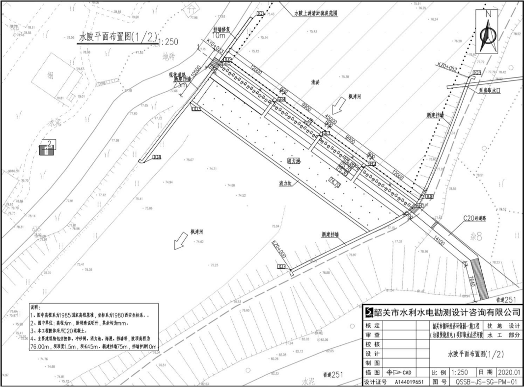
图 2 拦河水陂平面布置图 (a)
