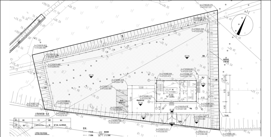
图 1 取水泵站平面布置图
