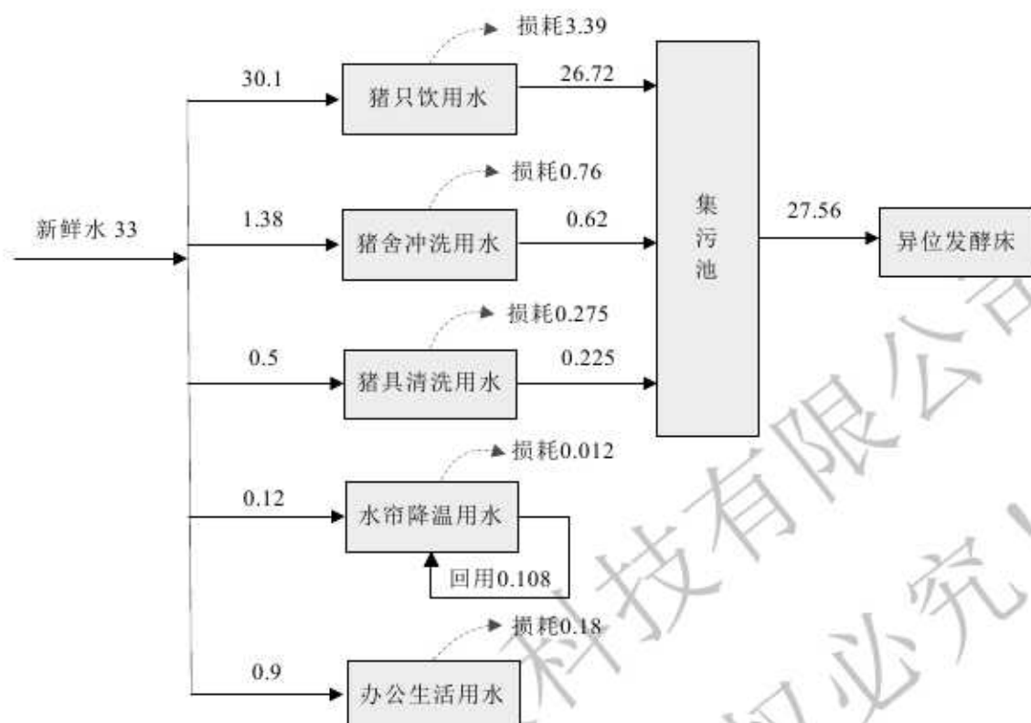
图 4-3 项目水平衡图 (单位: \text{m}^3/\text{d} )
