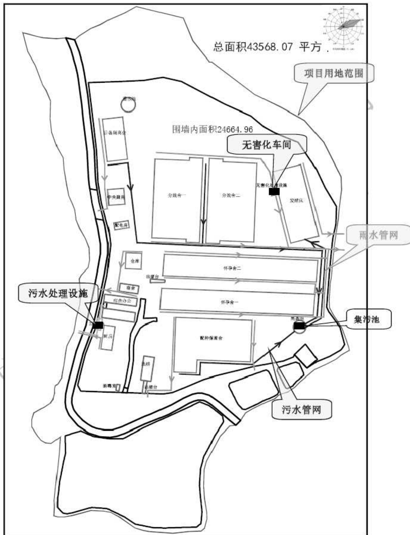
图 4-2 项目总体平面布置图
