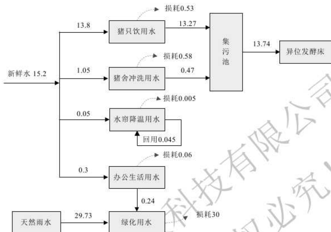
图 3-2 项目水平衡图 (单位: \text{m}^3/\text{d} )
