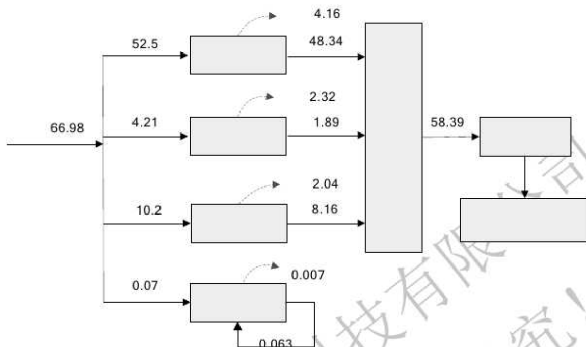
图 3-2 项目水平衡图 (单位: \text{m}^3/\text{d} )
