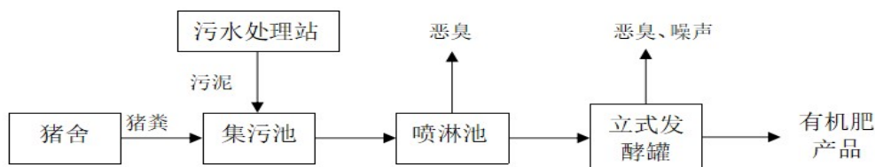
图 4-5 猪粪、污泥处理工艺流程及产污环节图
