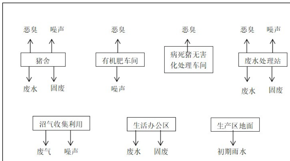
图 4-9 项目产污节点图
