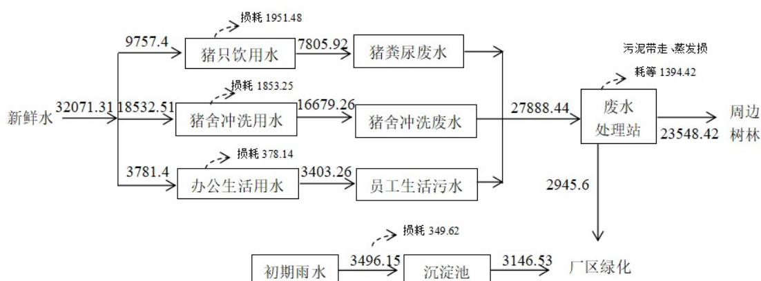
图 3-4 水平衡图 (单位: m 3 /a)
