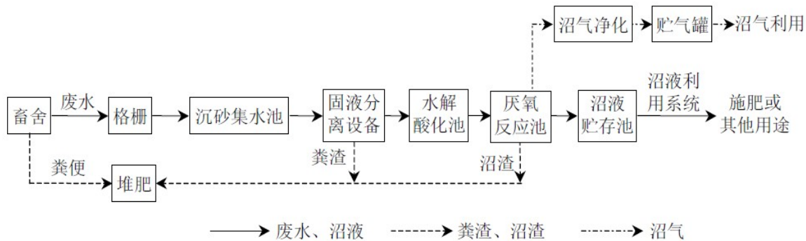
图 8-3 模式 II 工艺基本流程
