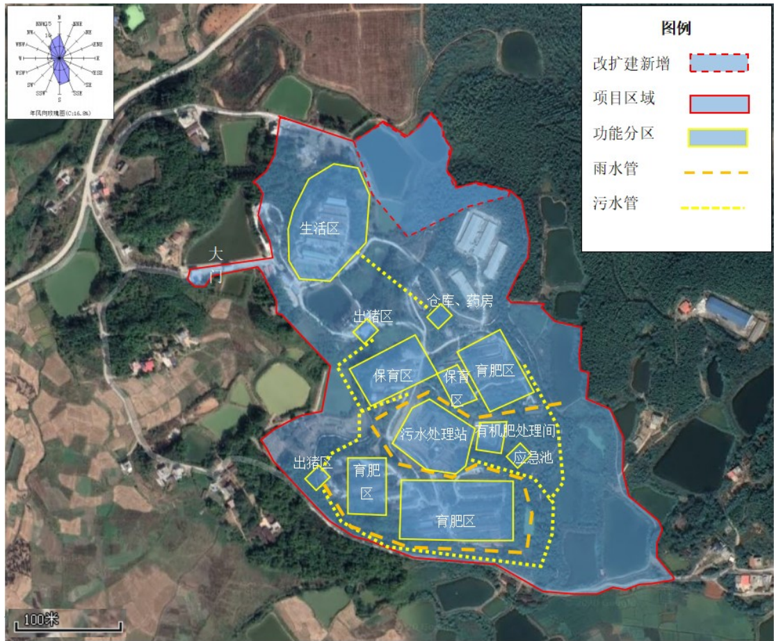
图 4-2 项目平面布置及雨污管网图
