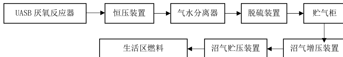
图 8-5 沼气收集系统工艺流程图
