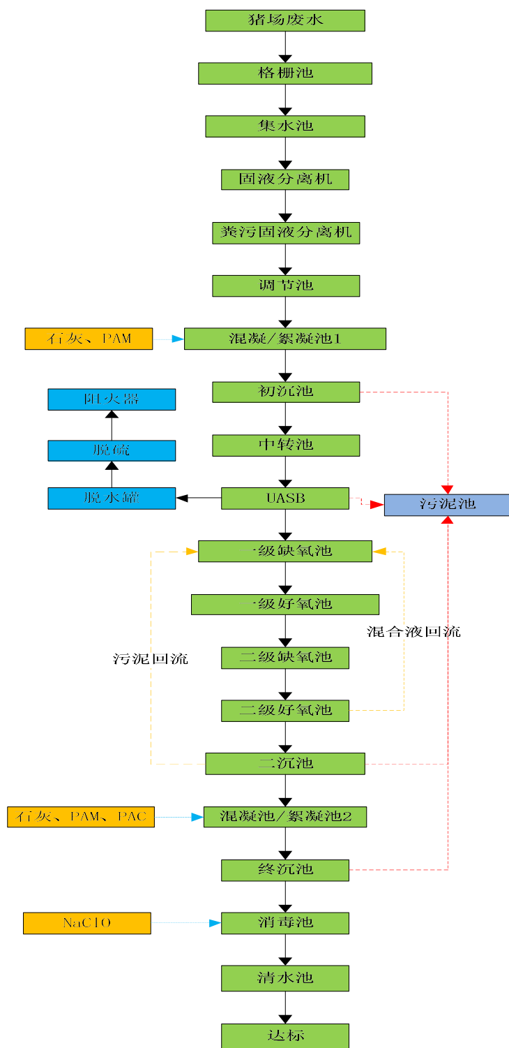
图 4-11 废水处理站工艺流程图
