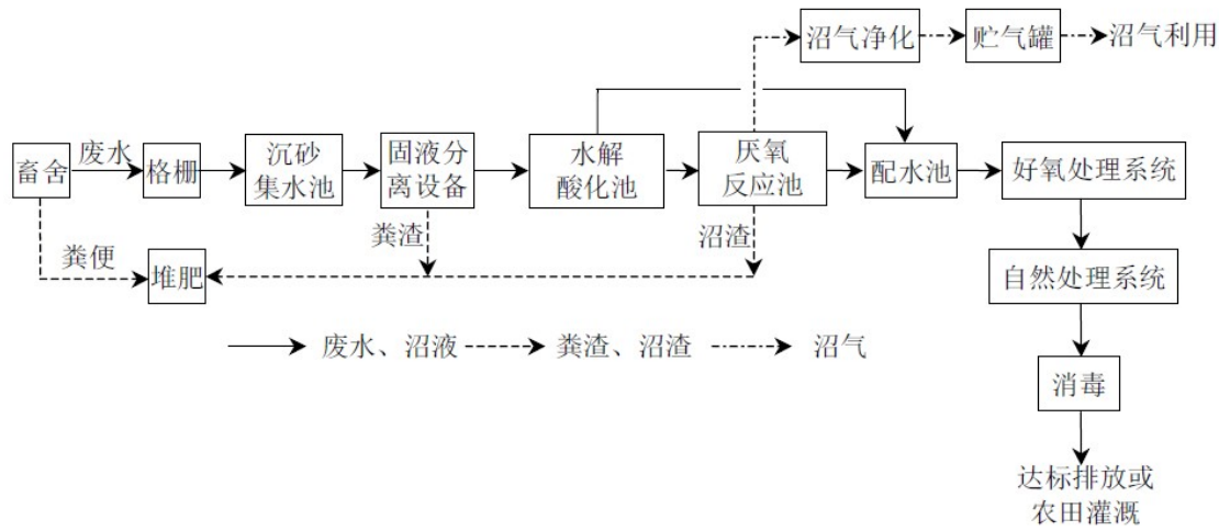
图 8-4 模式 III 工艺基本流程
