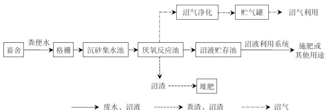
图 8-2 模式 I 工艺基本流程
