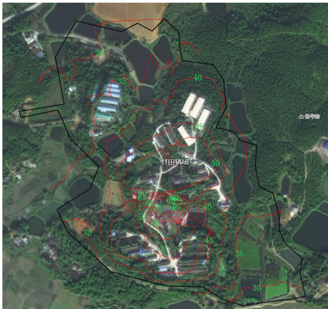
图 7-3 项目噪声昼间预测等声级线图
