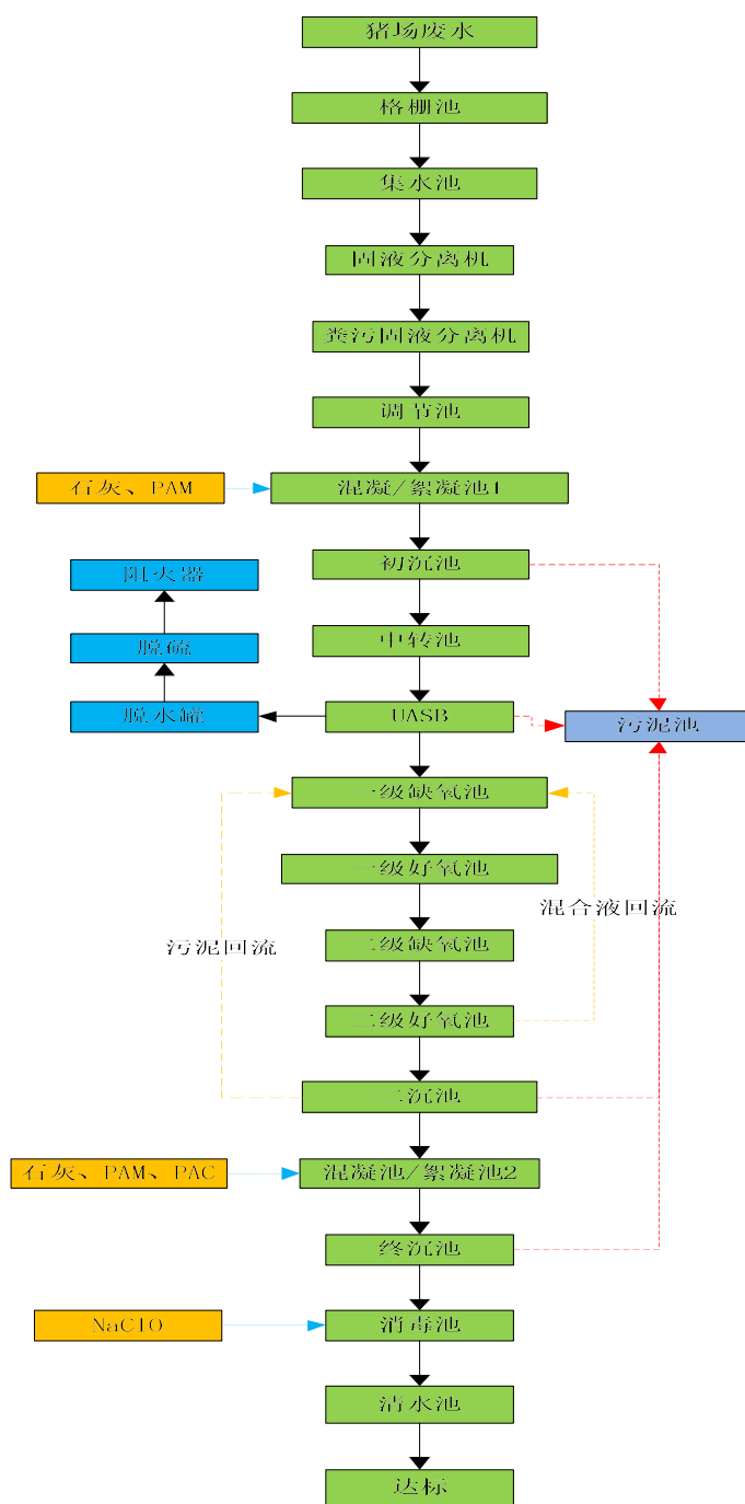
图 3-5 现有项目污水处理工艺
