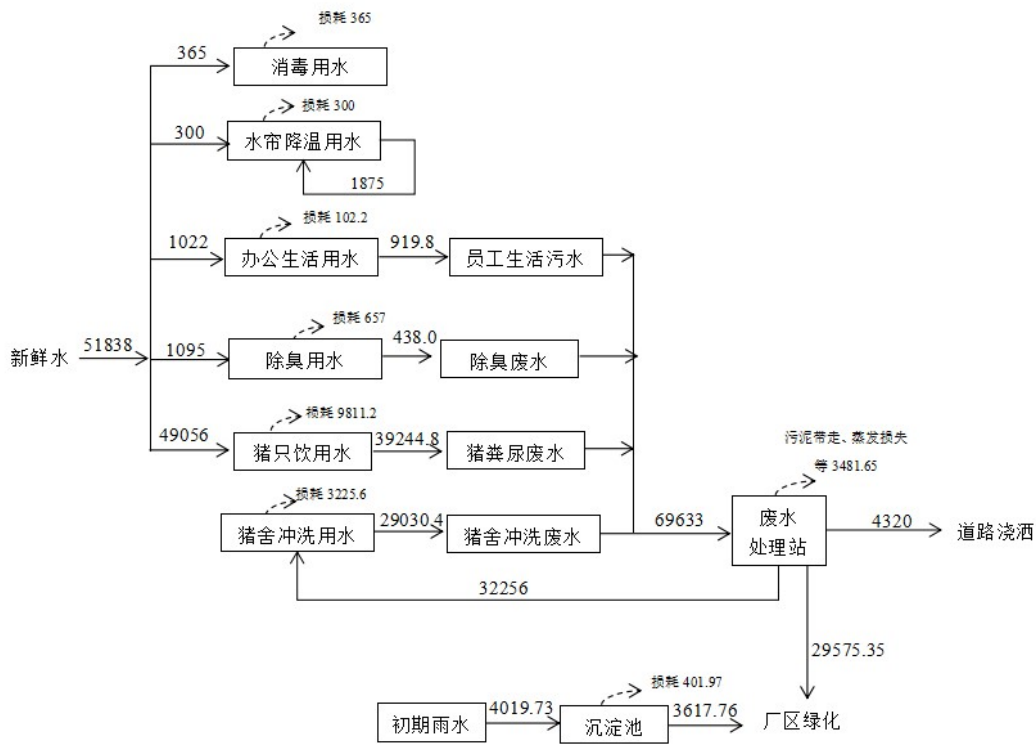
图 4-10 水平衡图 (单位: m³/a)
