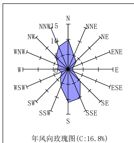
图 7-1 韶关气象站风玫瑰图 (1997~2016 年)
