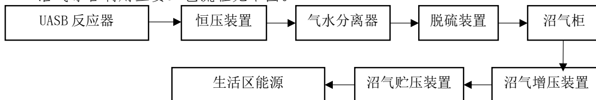
图 4-7 沼气收集利用工艺流程图
