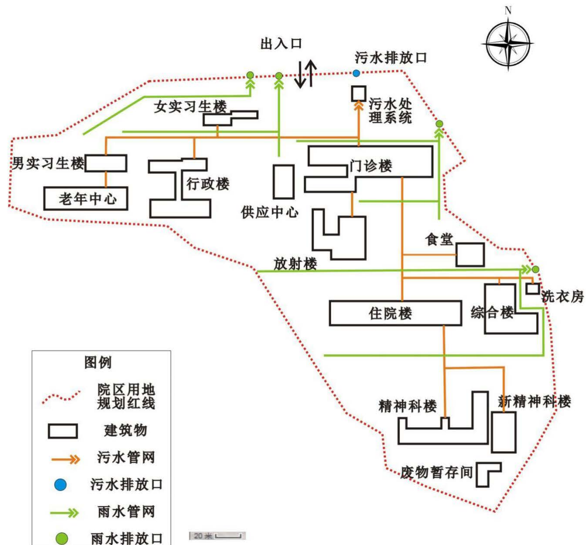
图 4 项目平面布置图
