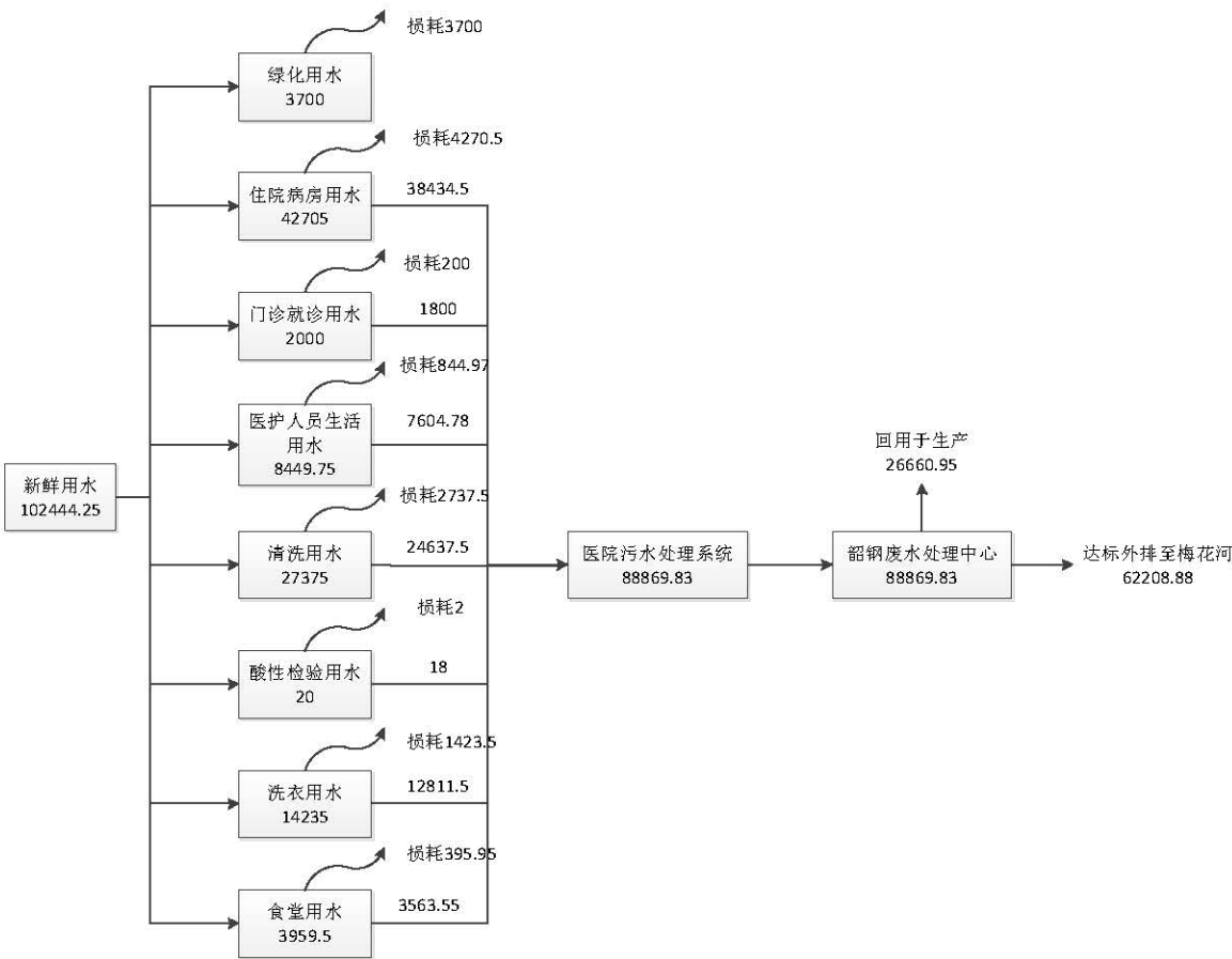
图 5 项目水平衡图（单位：m 3 /a）
