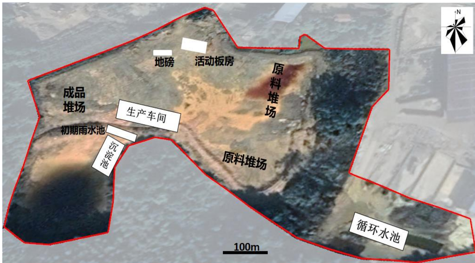
图 4 项目厂区平面布置图
