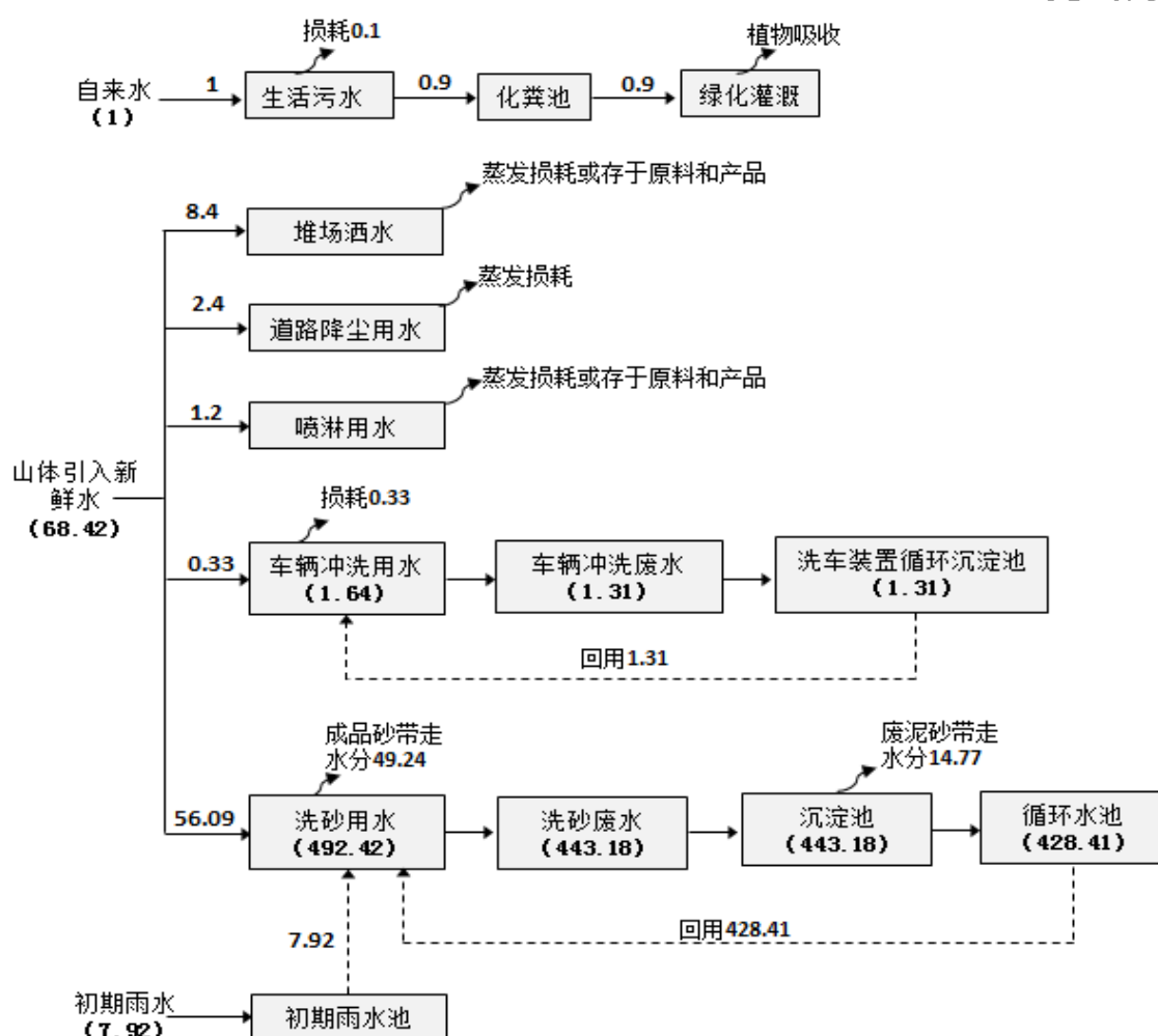
图 5 本项目水平衡图 (m 3 /d)
