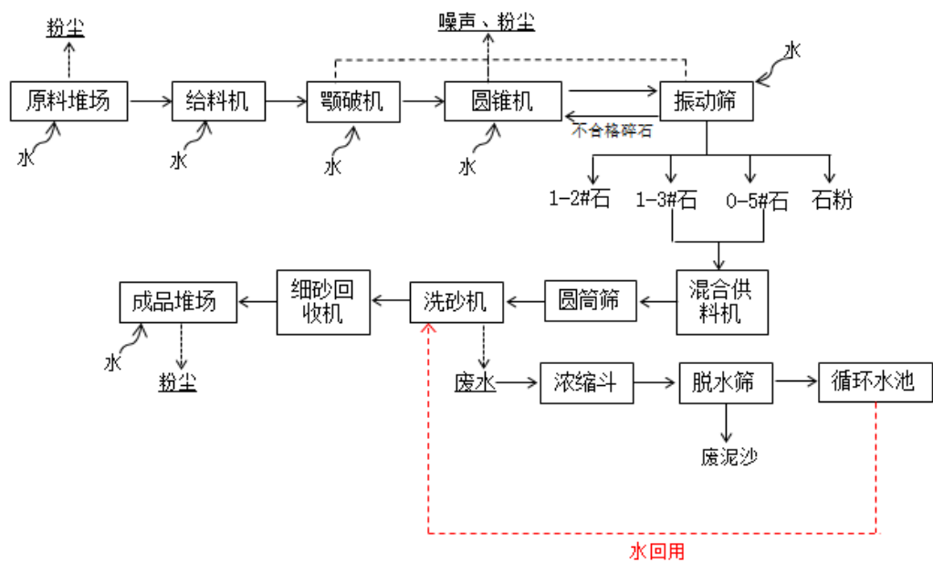
图 8 本项目生产工艺流程及产污环节图
