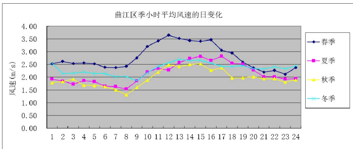
图 6.3-4 2018 年曲江季小时平均风速日变化曲线
