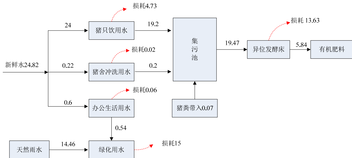
图 4.5-2 本项目扩建完成后水量平衡图 单位: m³/d
