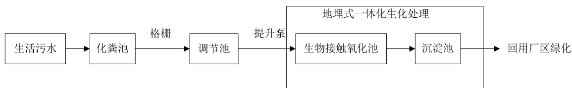
图 7.1-3 项目生活污水处理工艺流程图
