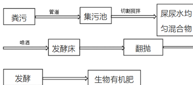
图 4.6-3 发酵床工艺流程图
