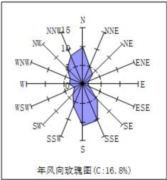
图 6.3-1 气象站年风向玫瑰图
