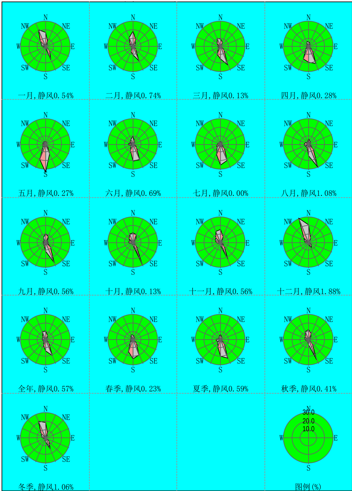
图 6.3-5 2018 年曲江区各季度及全年风向玫瑰图
