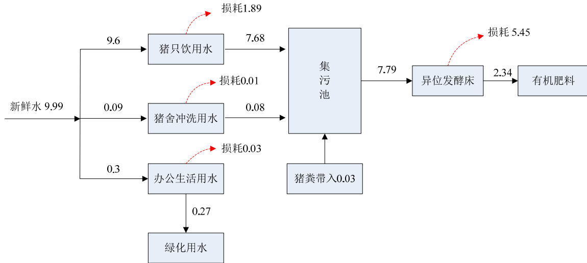
图 4.5-1 本项目水量平衡图 单位: m³/d
