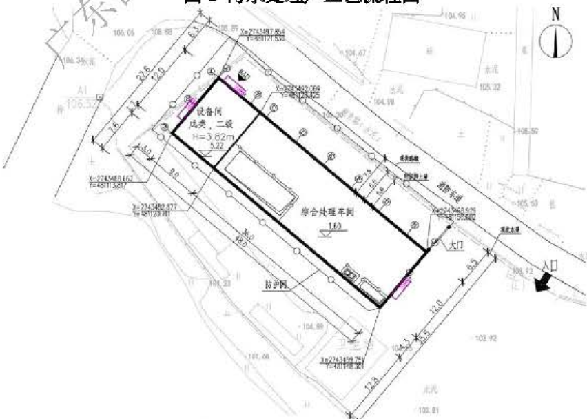
图 2 污水处理厂平面布置图
