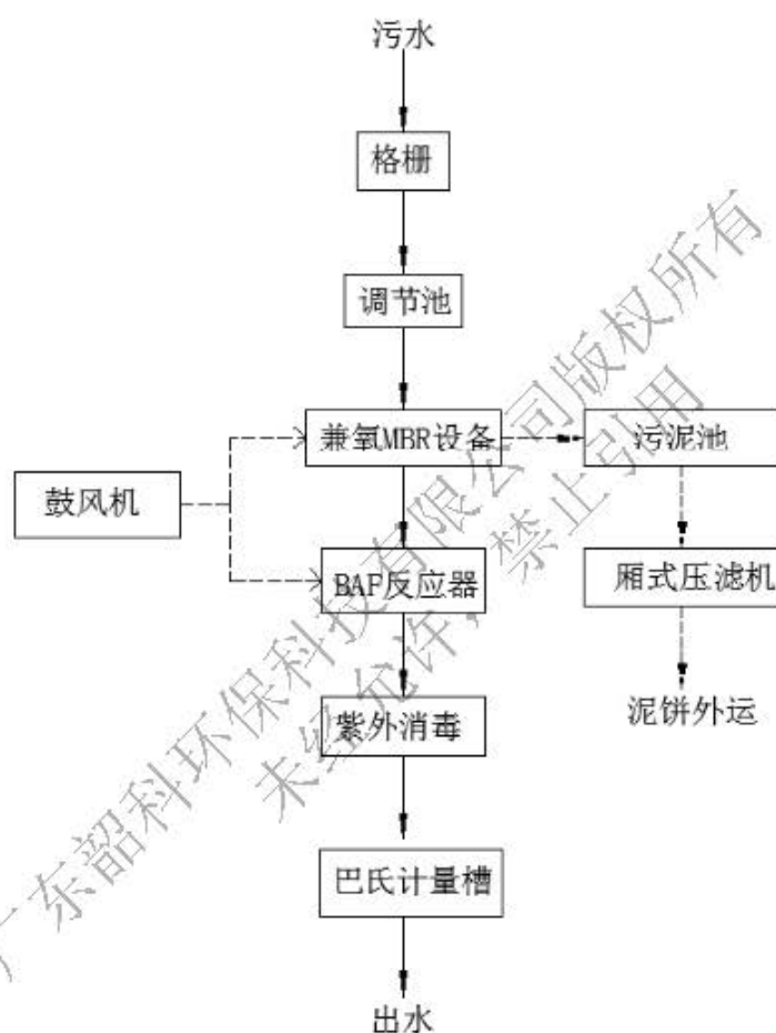
图 11 污水处理工艺流程图
