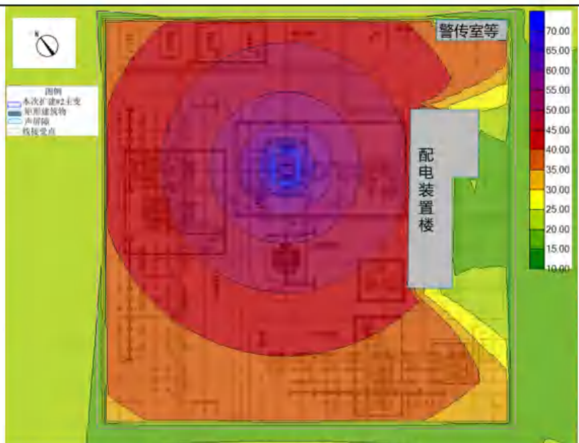
图 4-1 噪声贡献值等声值线图
