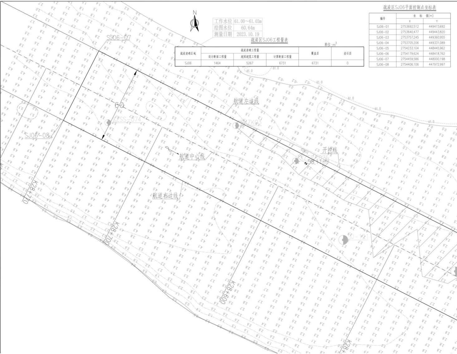
图2.5-37 疏浚区SJ06平面布置图 (c)
