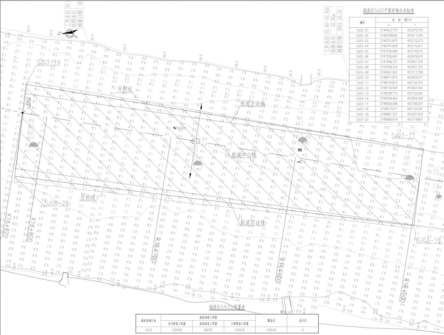
图2.5-28 疏浚区SJ03平面布置图 (h)
