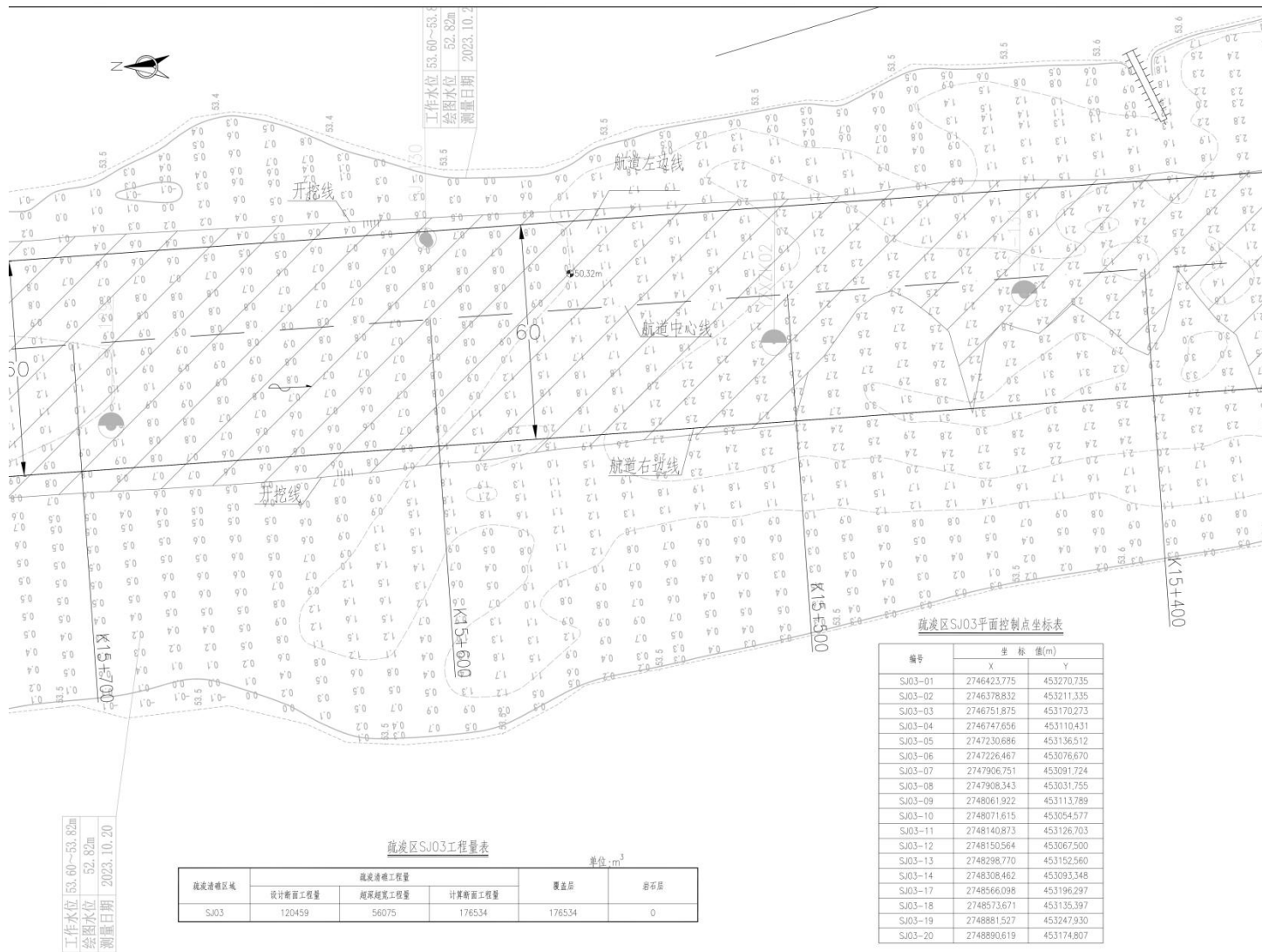
图2.5-24 疏浚区SJ03平面布置图（d）
