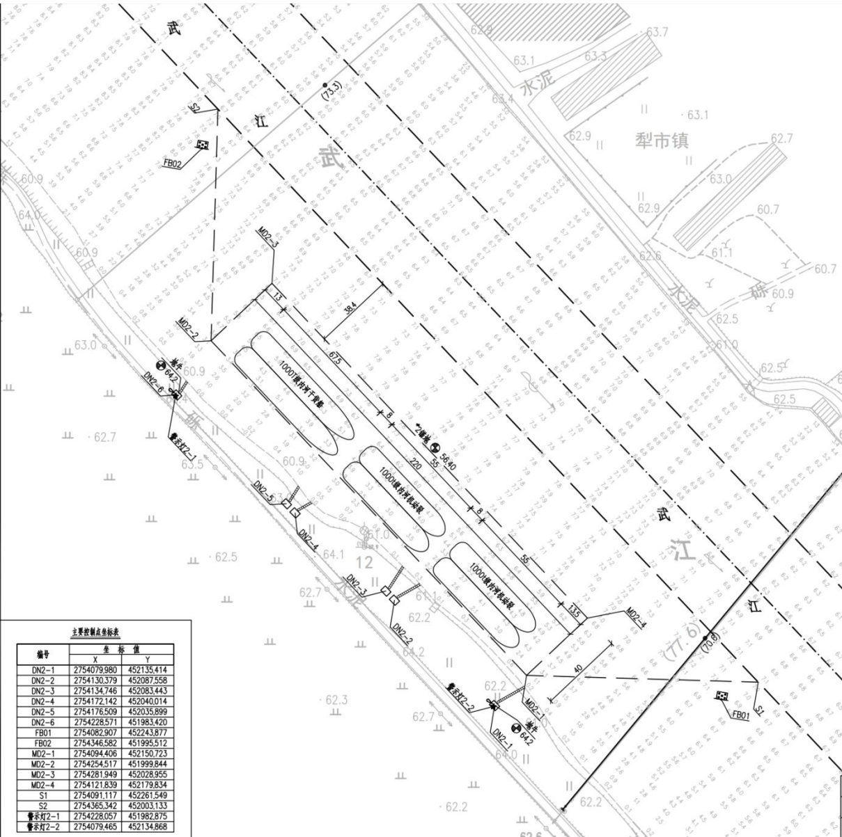
图2.5-61 2#锚地平面图
