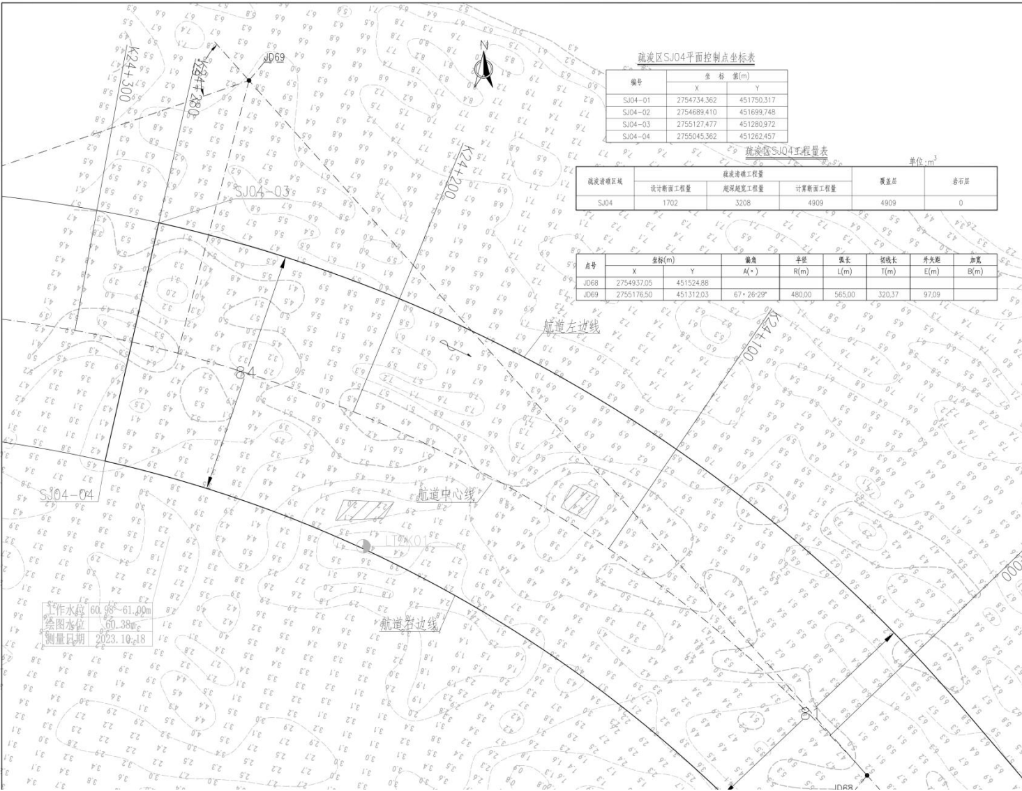
图2.5-31 疏浚区SJ04平面布置图（c）
