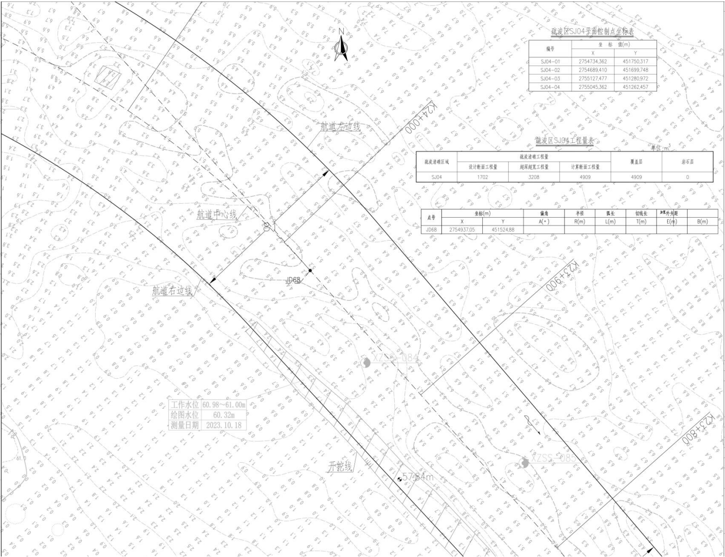
图2.5-30 疏浚区SJ04平面布置图（b）
