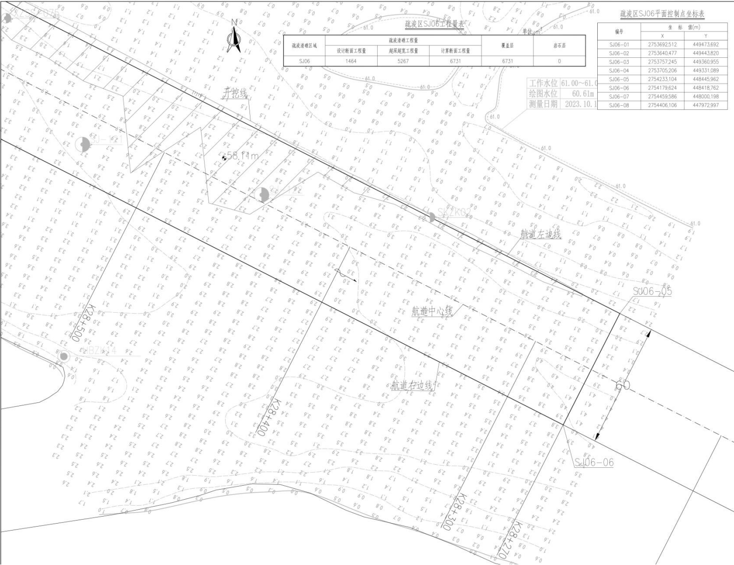
图2.5-36 疏浚区SJ06平面布置图（b）
