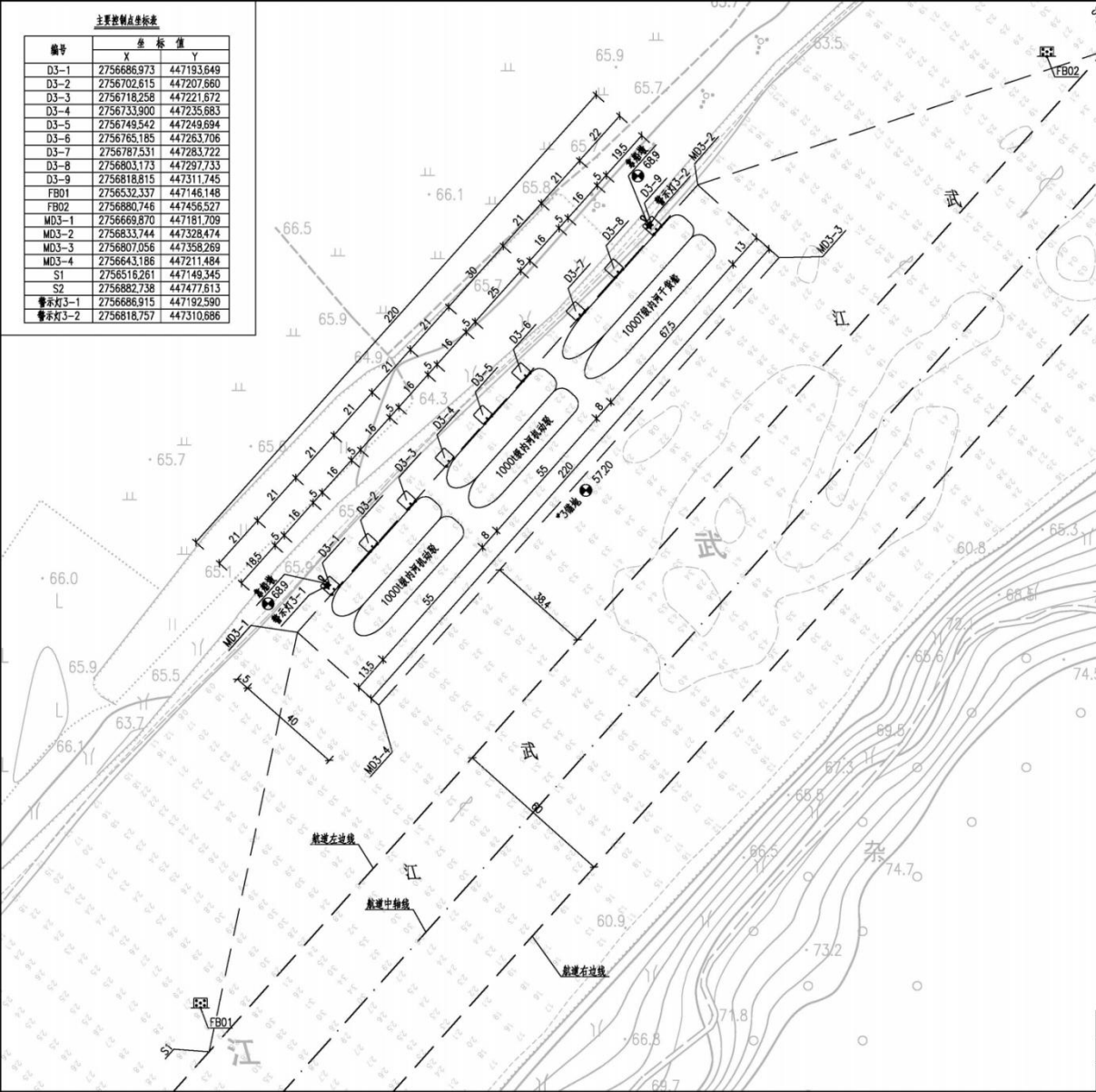
图2.5-62 3#锚地平面图
