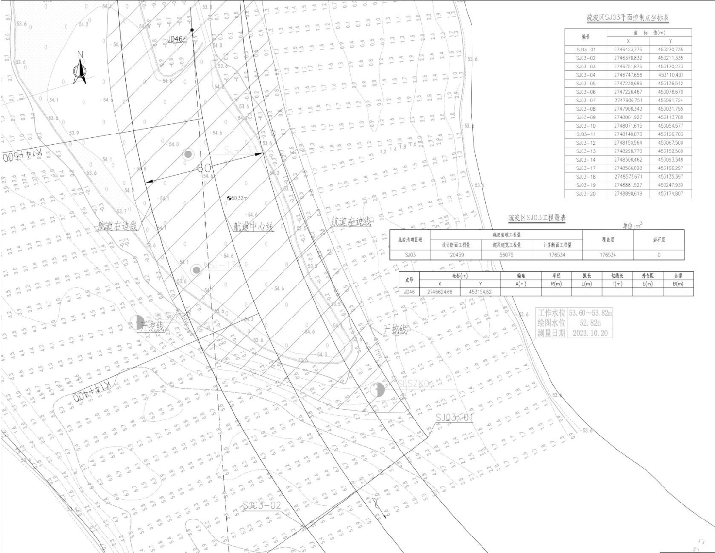
图2.5-21 疏浚区SJ03平面布置图（a）
