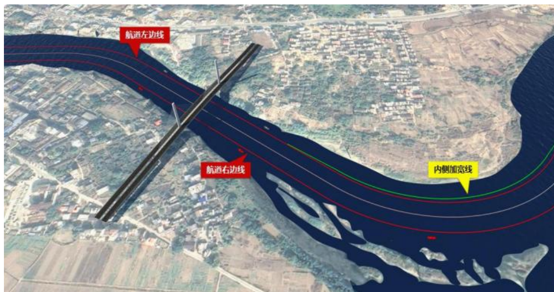
图2.5-9 桂头大桥桥区航道线路图
