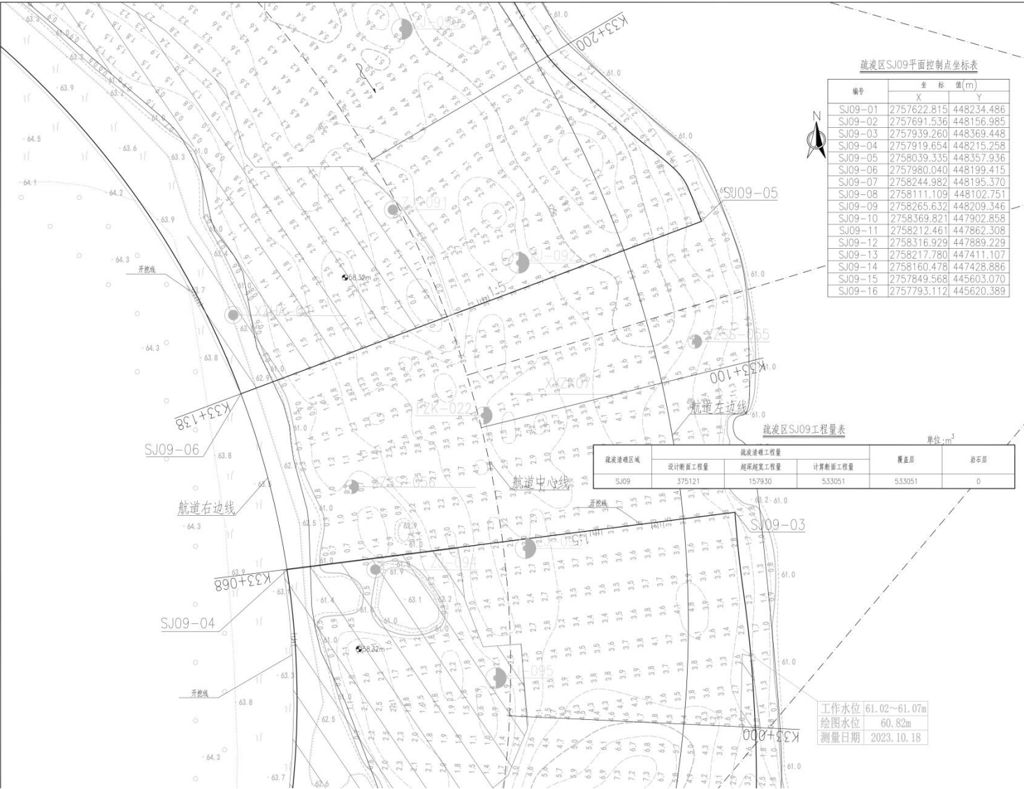
图2.5-47 疏浚区SJ09平面布置图（b）
