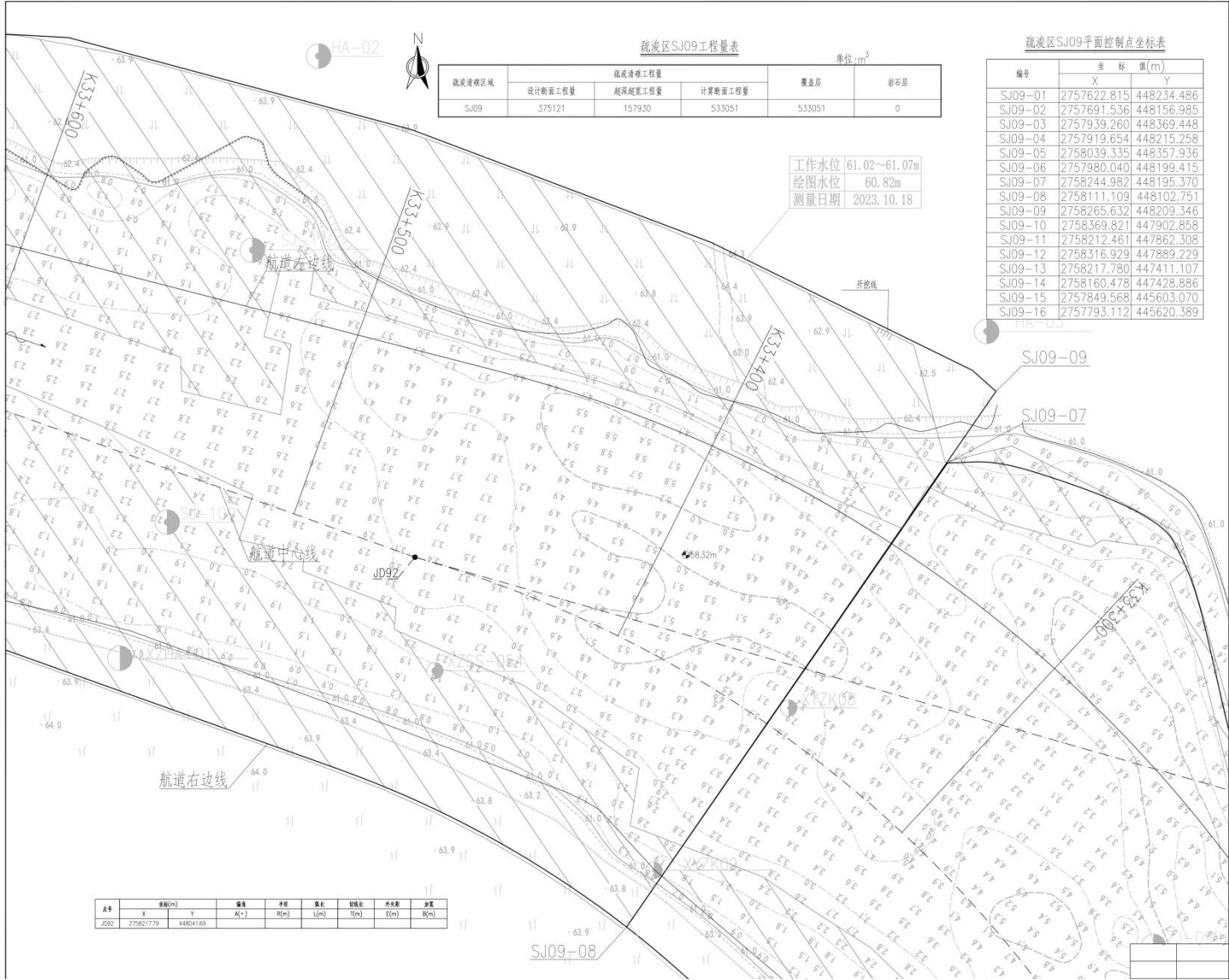
图2.5-49 疏浚区SJ09平面布置图（d）
