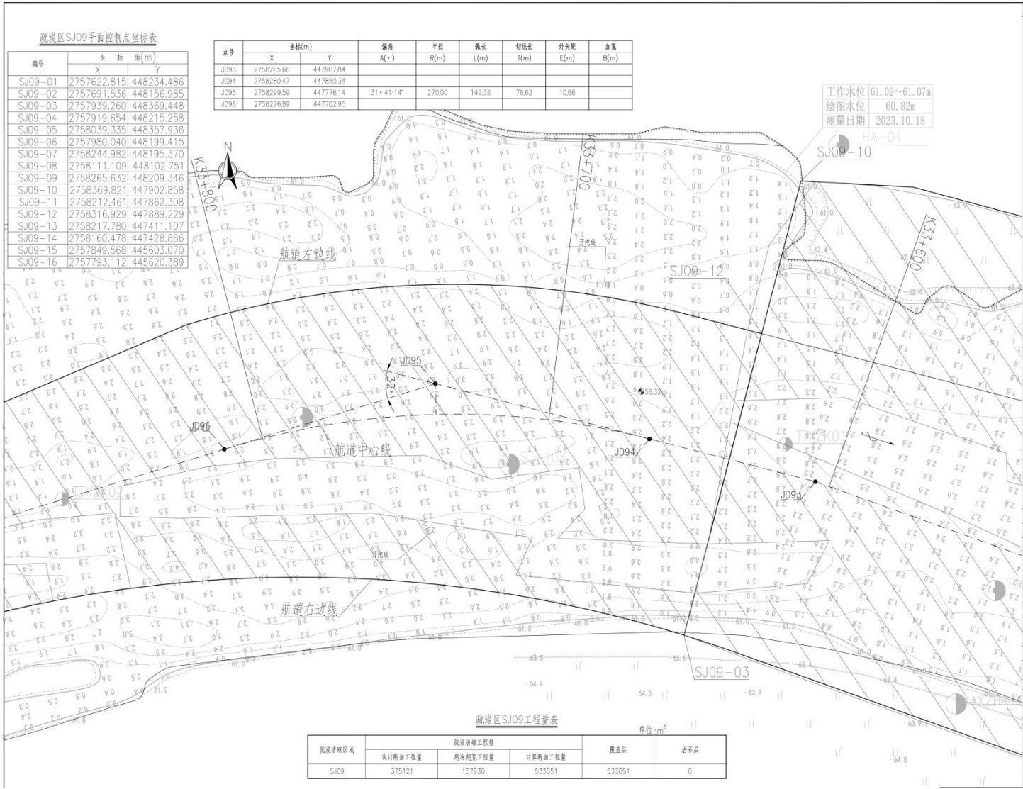
图2.5-50 疏浚区SJ09平面布置图（e）
