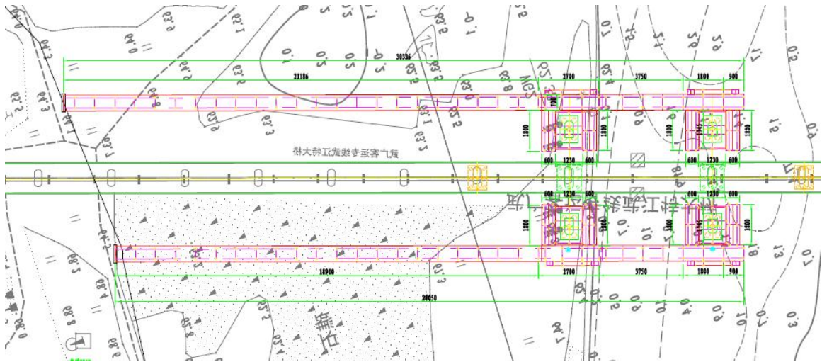
图2.5-17 武广客运专线武江特大桥防撞墩栈桥与平台平面布置图
