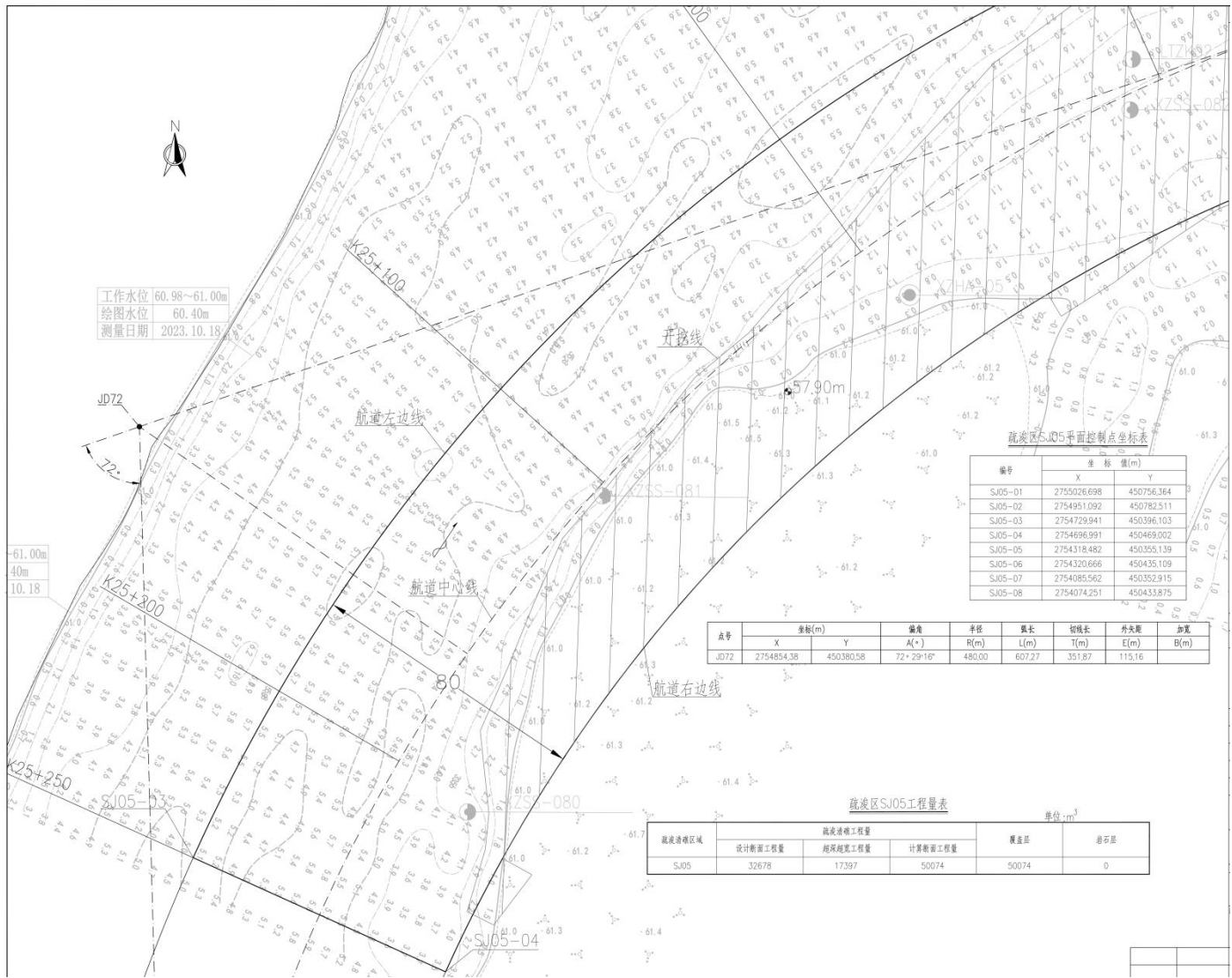
图2.5-33 疏浚区SJ05平面布置图（b）
