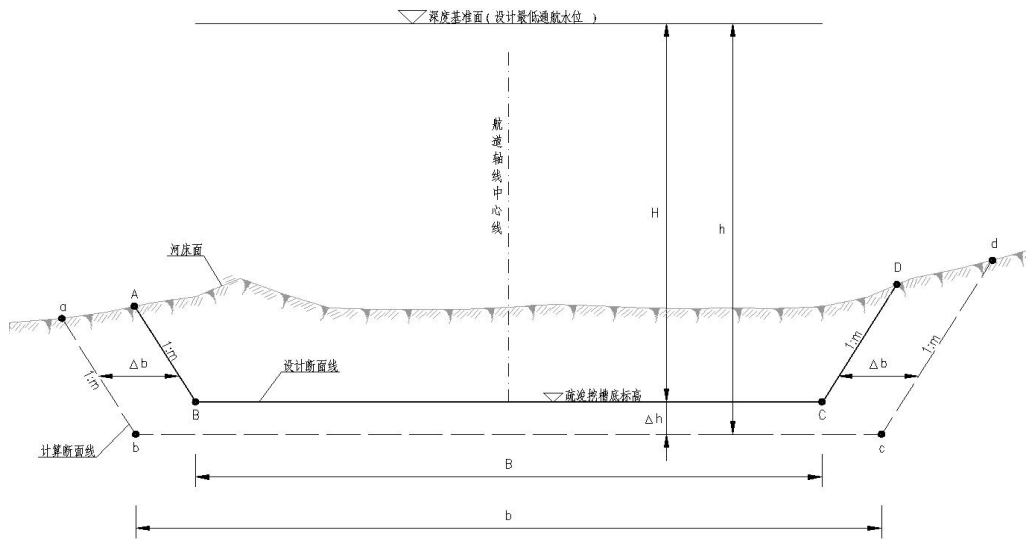
图2.5-14 挖槽设计标准断面图
