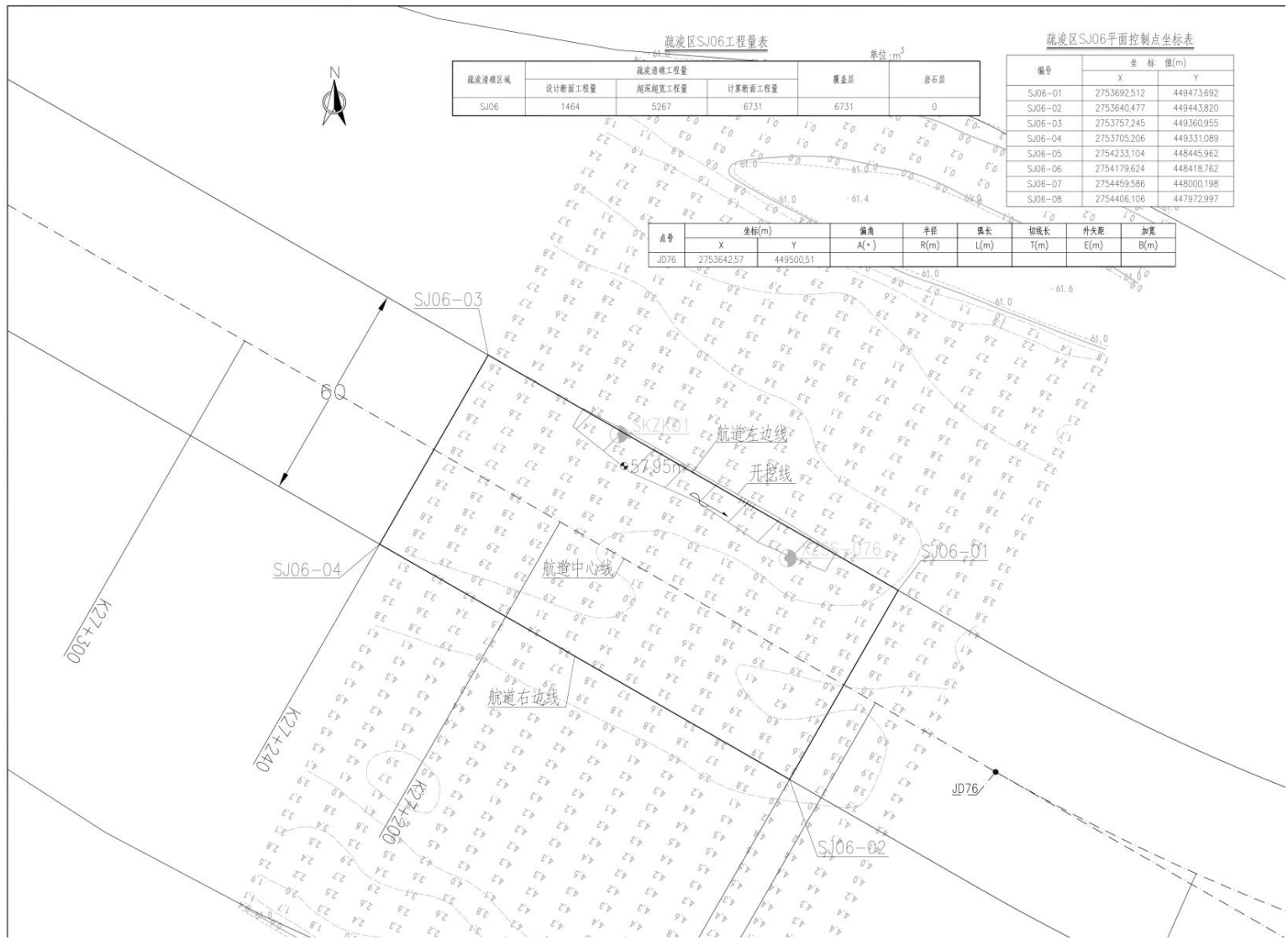
图2.5-35 疏浚区SJ06平面布置图 (a)
