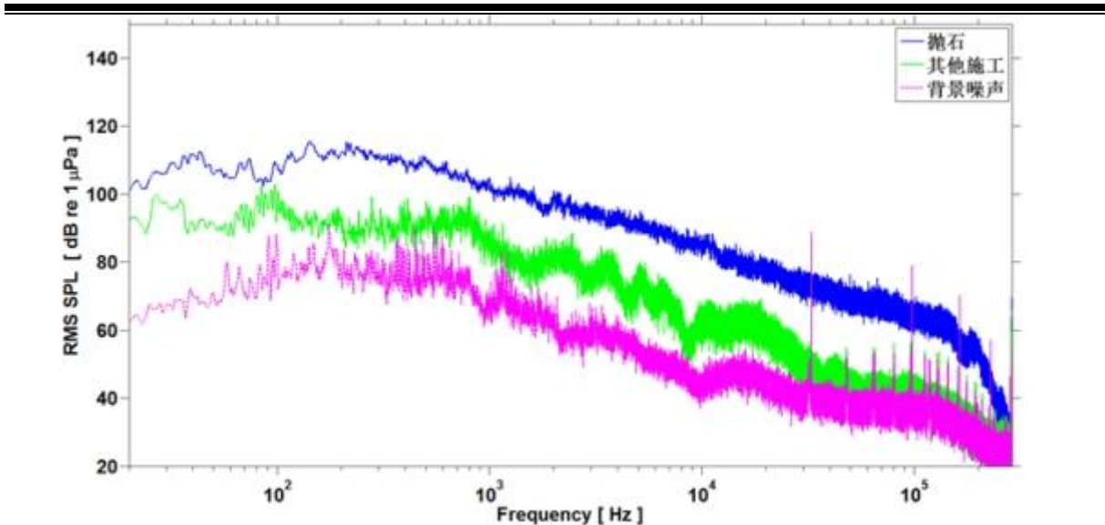
图5.2-1 不同类型航道整治施工噪声的均方根声压级对比
