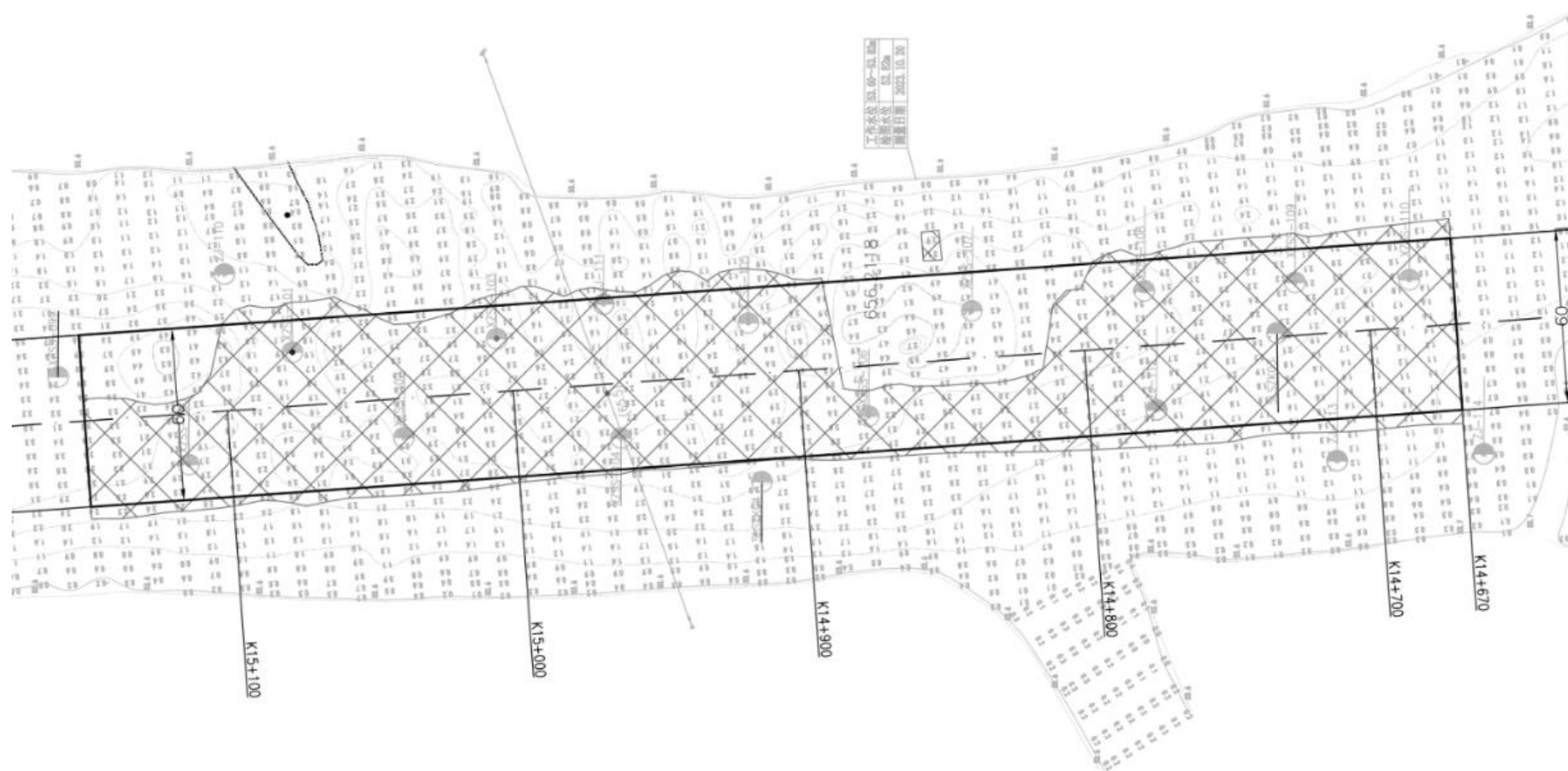
图 2.5-54 清淤区 QJ01 平面布置图
