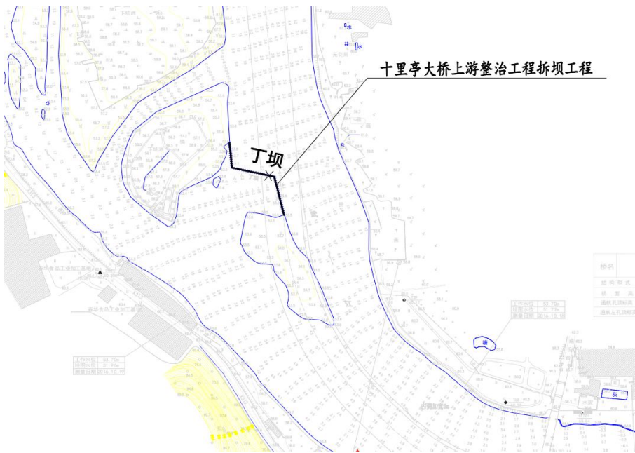
图2.5-58 十里亭大桥上游整治方案平面图
