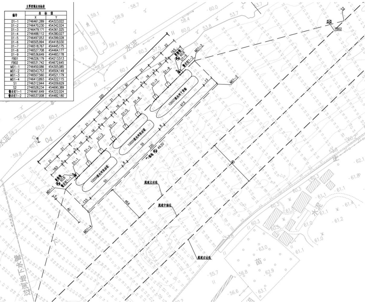
图2.5-60 1#锚地平面图
