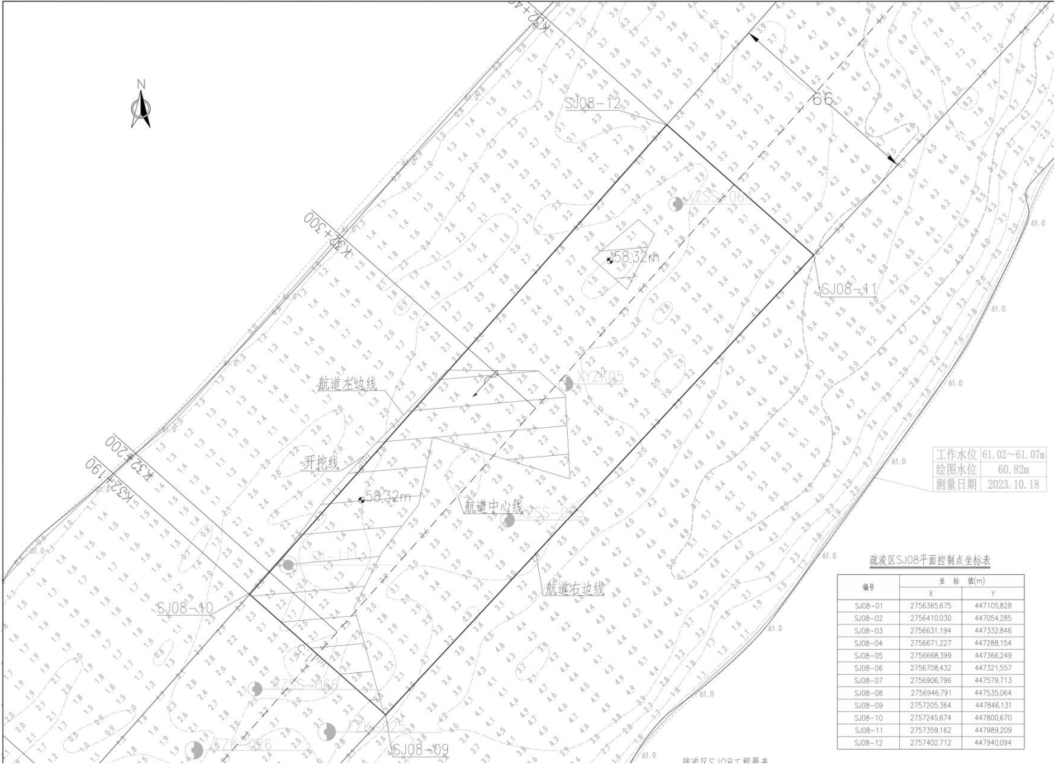
图2.5-45 疏浚区SJ08平面布置图（d）
