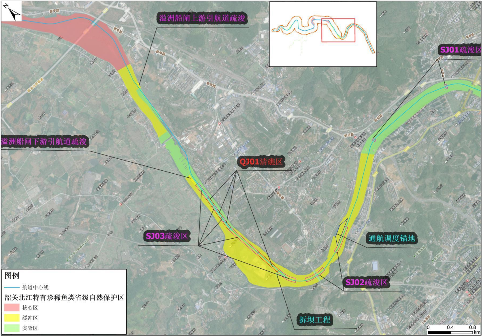
图 1.7-6 工程与韶关北江特有珍稀鱼类省级自然保护区（现状）位置关系示意图（c）
