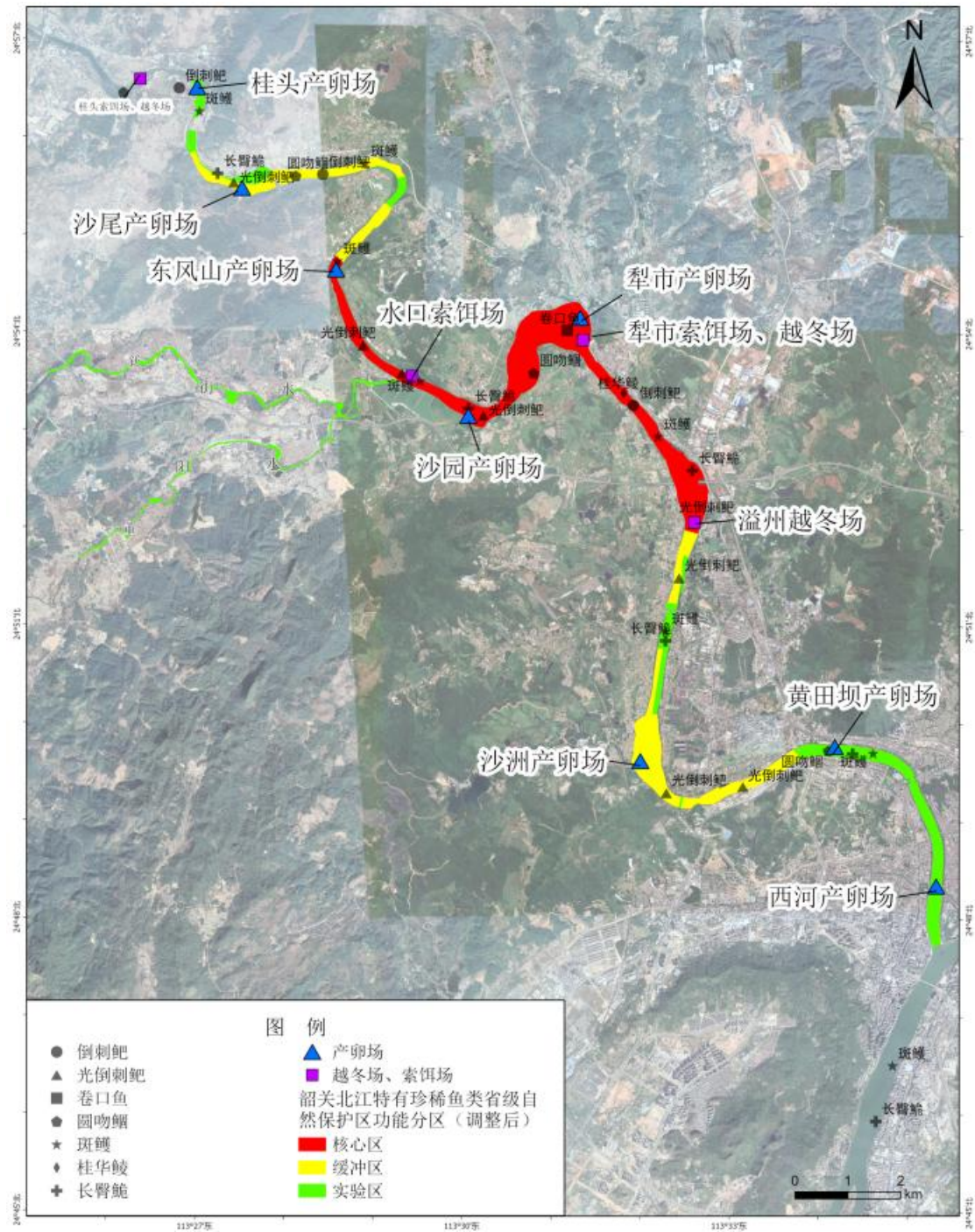
图 4.3-1 评价范围内鱼类三场分布
