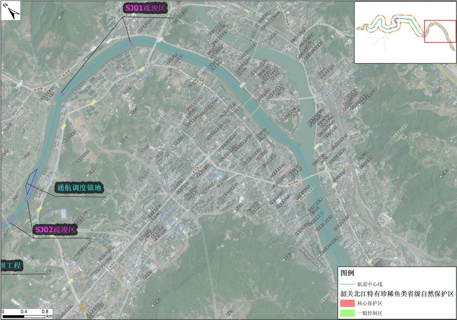
图 1.7-12 工程与韶关北江特有珍稀鱼类省级自然保护区（整合优化调整后）位置关系示意图（d）
