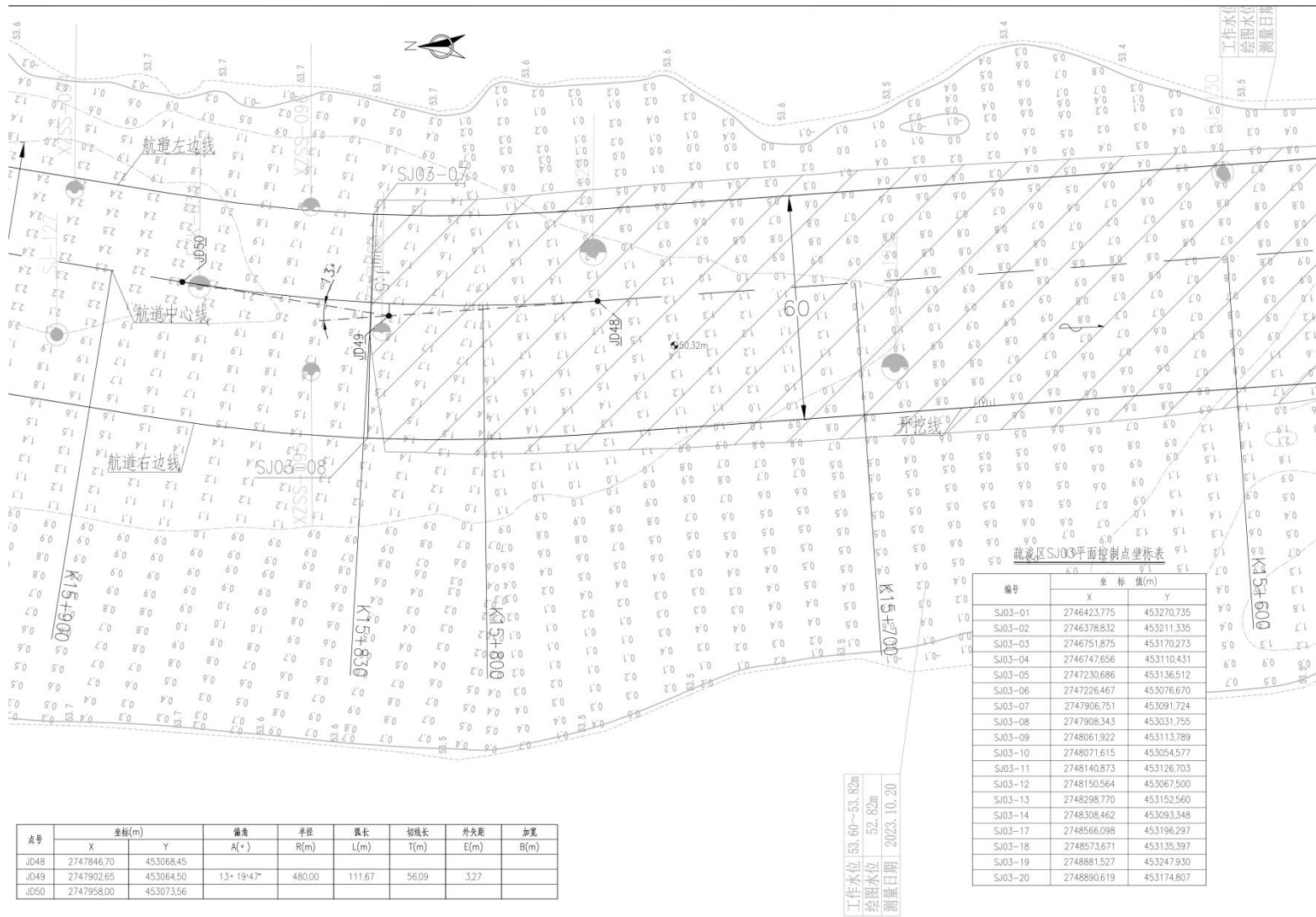
图2.5-25 疏浚区SJ03平面布置图 (e)
