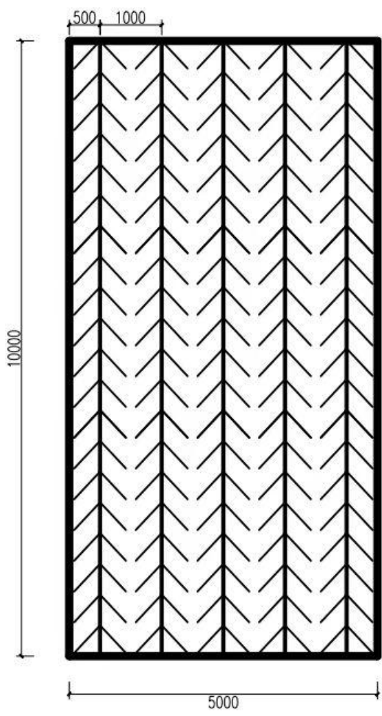
图 7.2-1 单件人工鱼巢布置（单位：mm）
