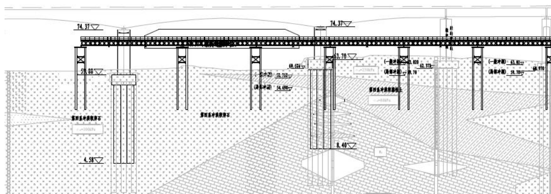
图2.5-18 武广特大桥栈桥断面图
