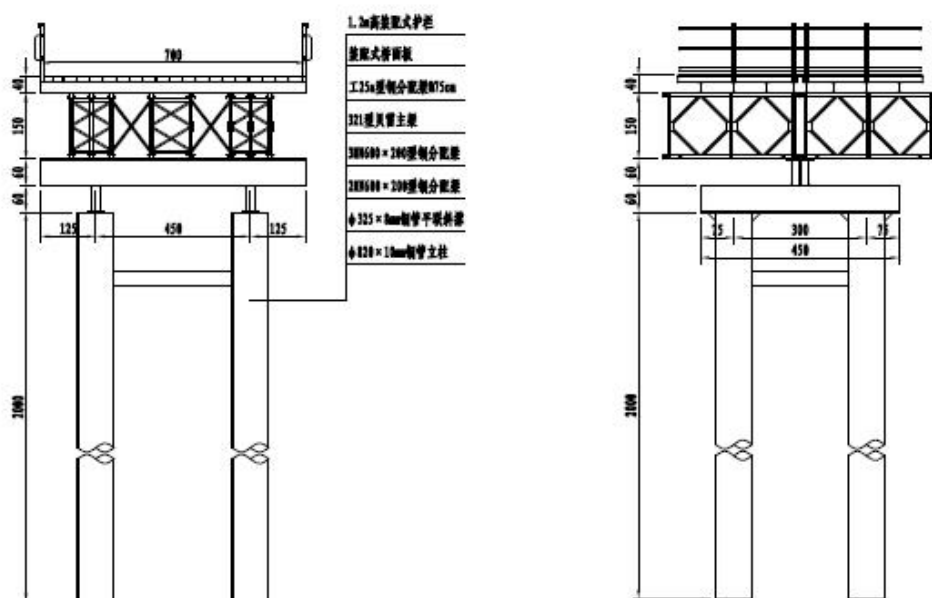
图2.5-20 栈桥标准横断面图
