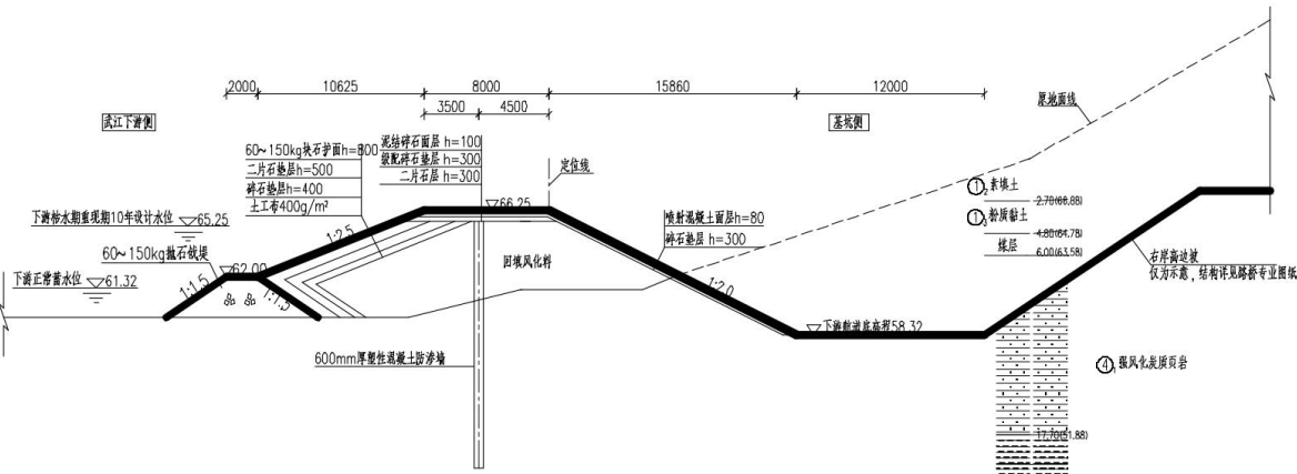
图2.5-16 下游枯水围堰断面图
