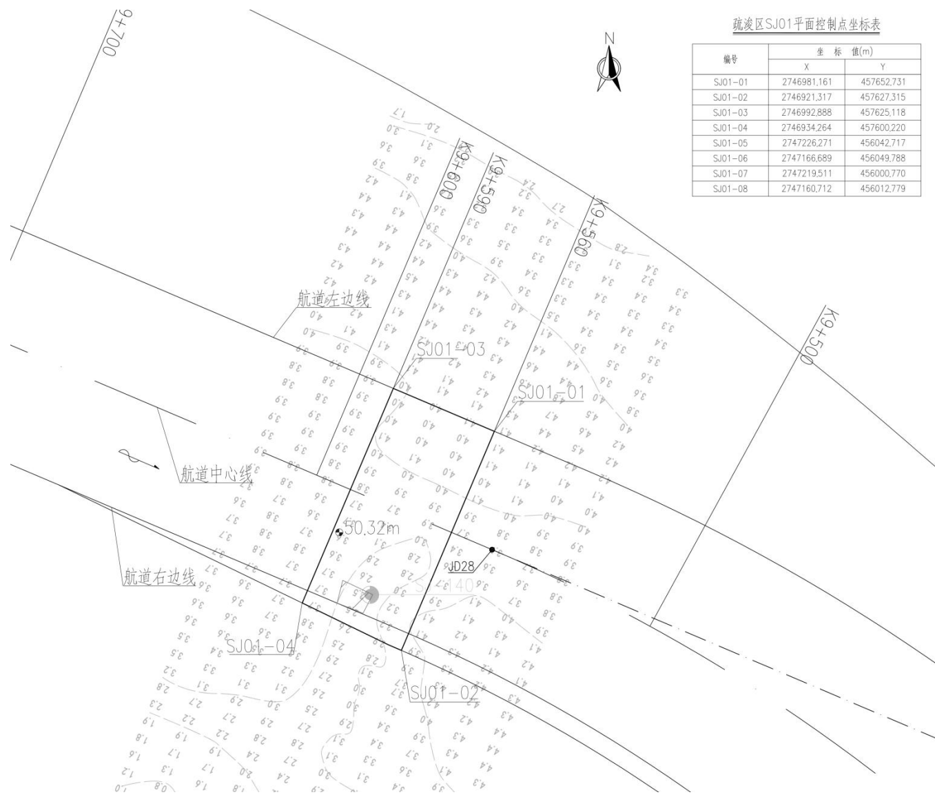
图2.5-15 疏浚区SJ01平面布置图（a）
