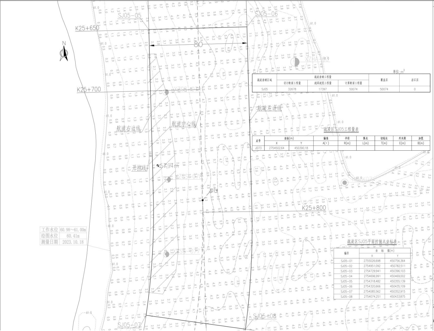
图2.5-34 疏浚区SJ05平面布置图 (c)
