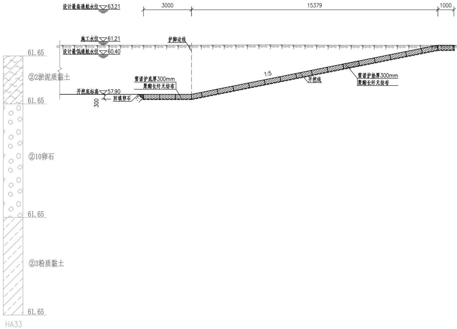
图 2.5-65 莲塘河段切滩及护岸工程断面图
