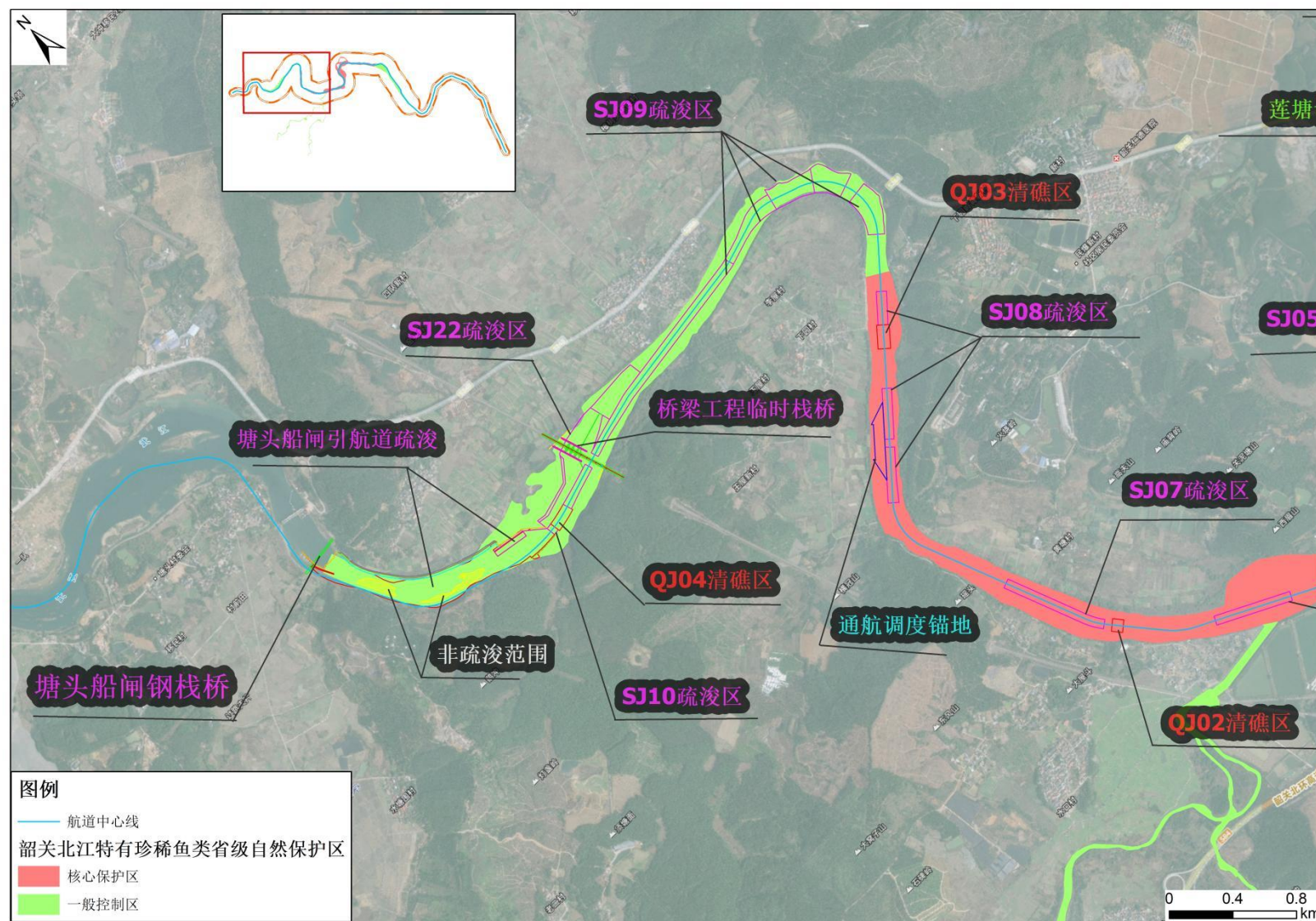
图 1.7-9 工程与韶关北江特有珍稀鱼类省级自然保护区（整合优化调整后）位置关系示意图（a）
