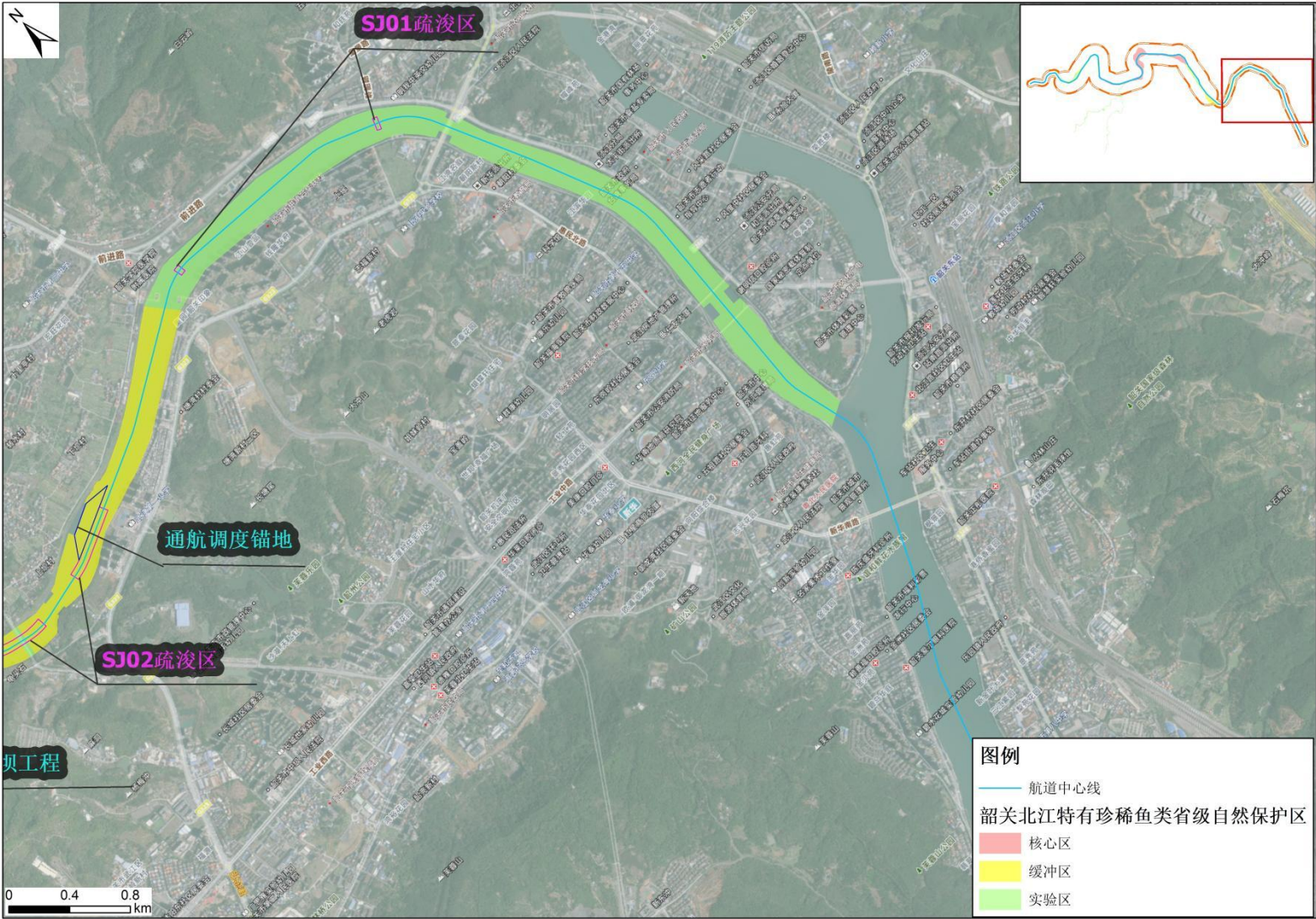
图 1.7-7 工程与韶关北江特有珍稀鱼类省级自然保护区（现状）位置关系示意图（d）
