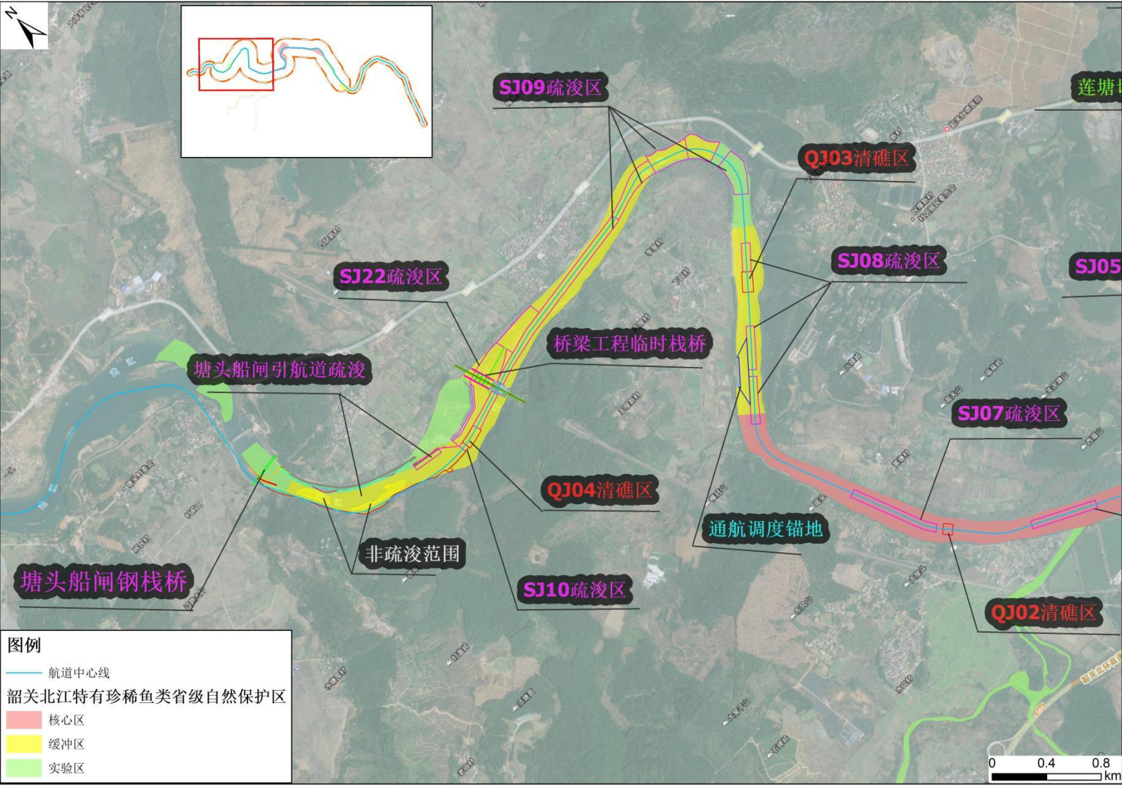
图 1.7-4 工程与韶关北江特有珍稀鱼类省级自然保护区（现状）位置关系示意图（a）
