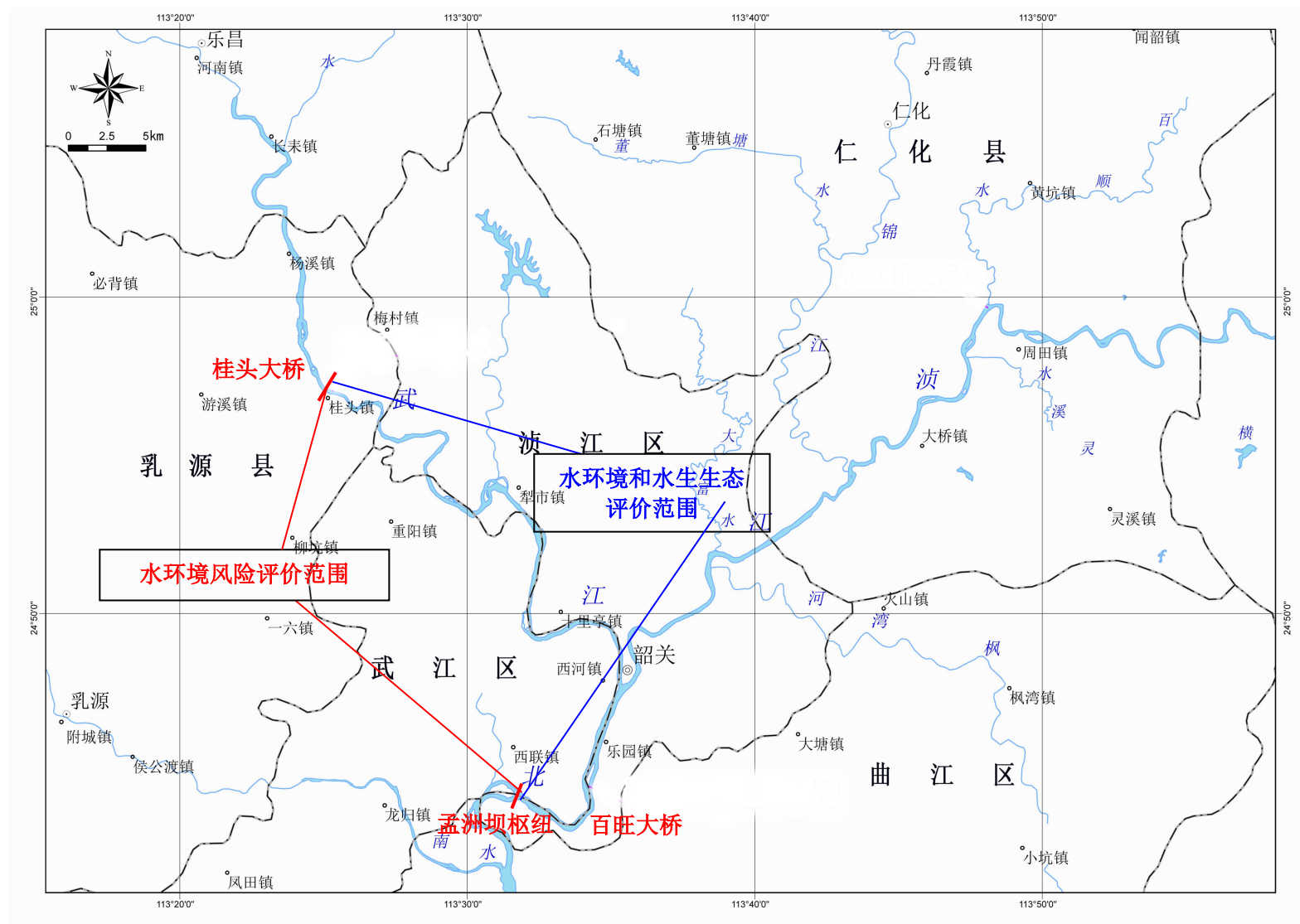
图 1.5-1 本工程水生生态、水环境及水环境风险评价范围示意图
