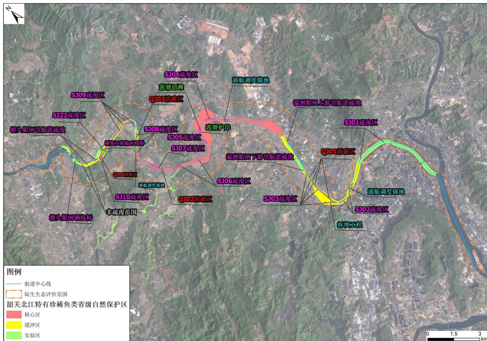
图 1.7-3 工程与韶关北江特有珍稀鱼类省级自然保护区（现状）位置关系示意图（总图）
