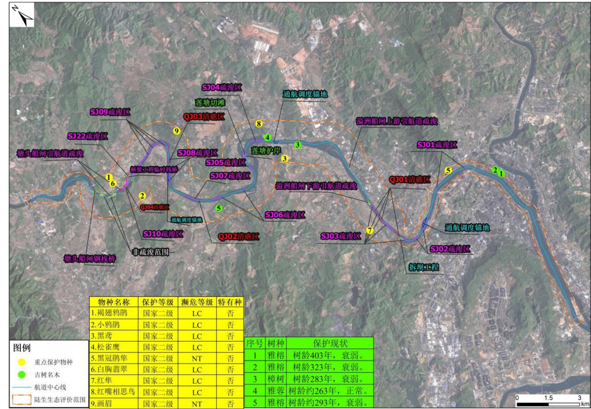
图 1.7-15 工程生态评价范围古树和国家重点保护野生动物分布图
