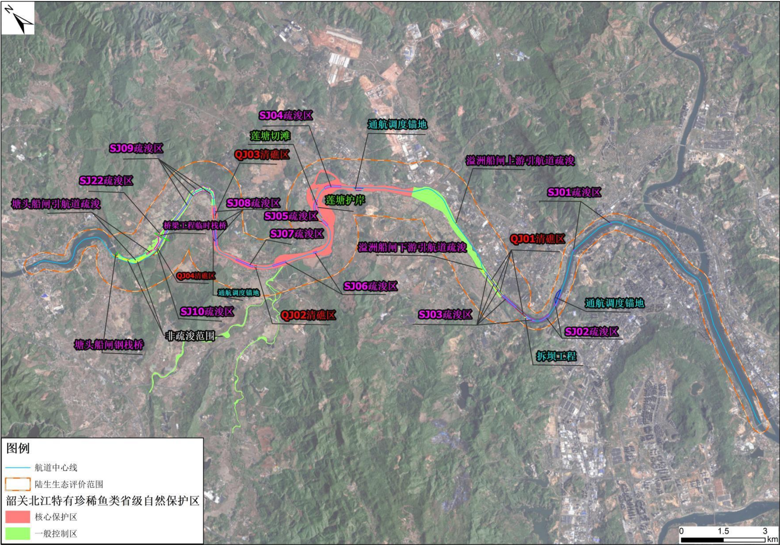
图 1.7-8 工程与韶关北江特有珍稀鱼类省级自然保护区（整合优化调整后）位置关系示意图（总图）
