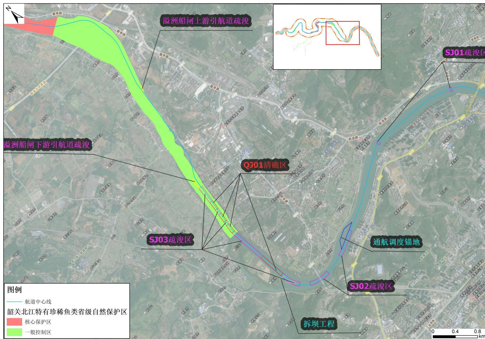
图 1.7-11 工程与韶关北江特有珍稀鱼类省级自然保护区（整合优化调整后）位置关系示意图（c）
