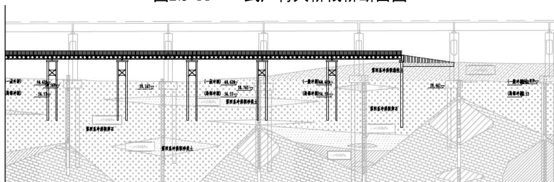
图2.5-19 武广特大桥栈桥立面布置图
