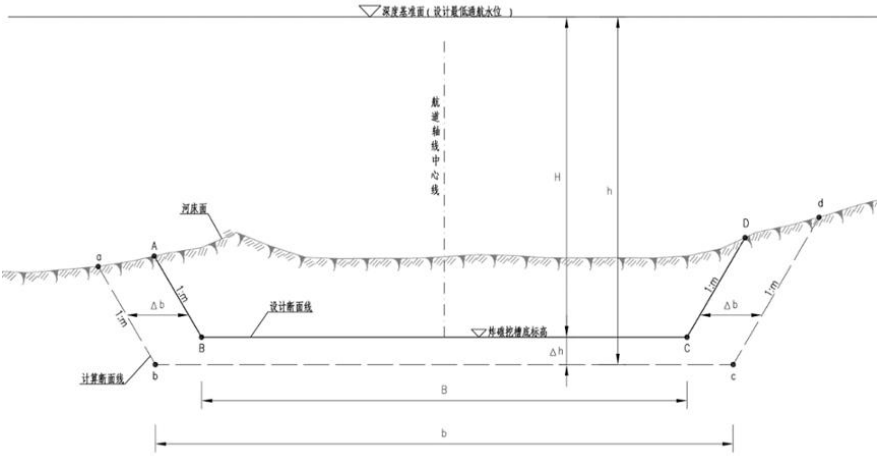
图2.5-13 清礁设计标准断面图
