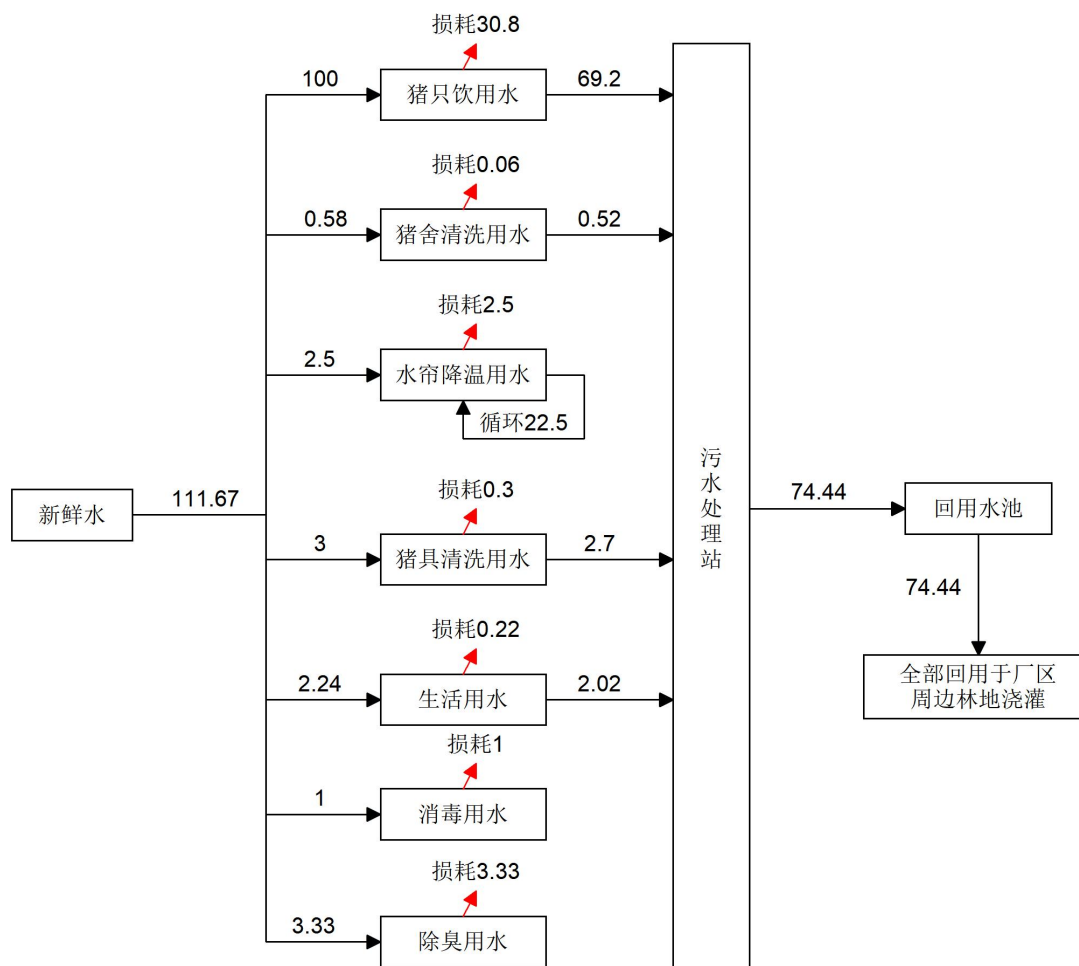
图 3.2-1 项目水平衡图（单位：m³/d）
