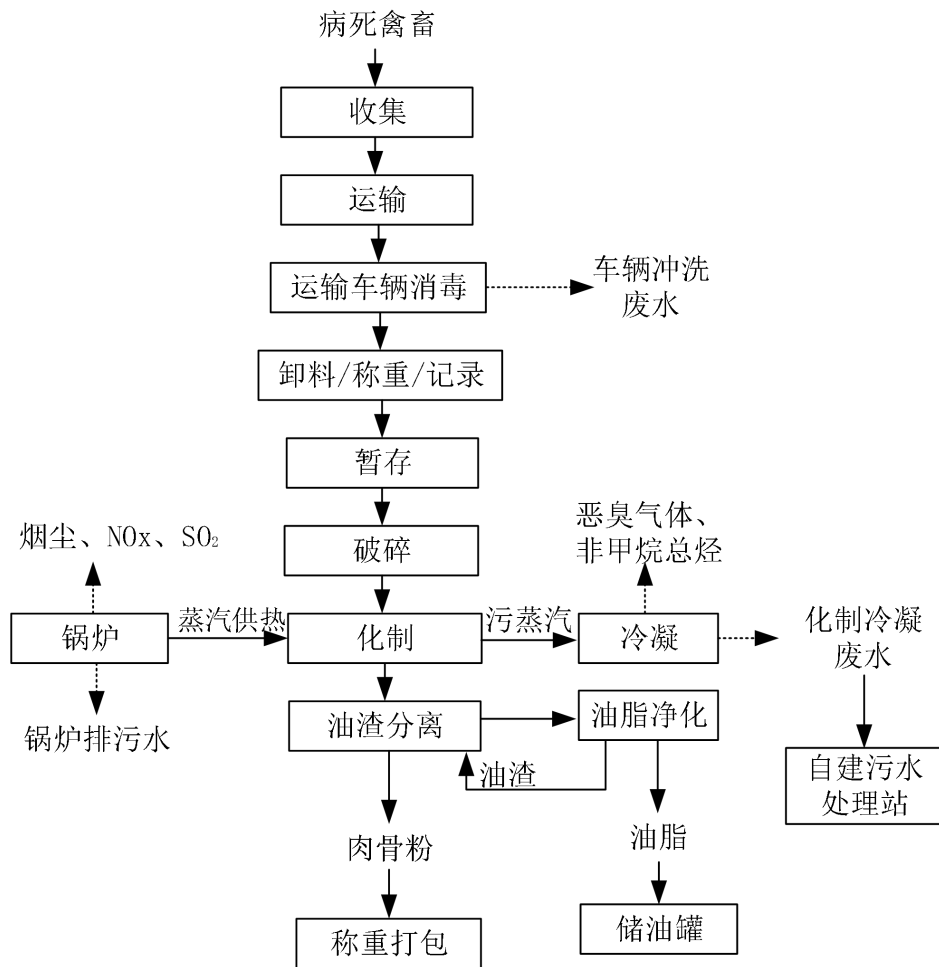
图 3.3-5 瀚蓝生态资源科技（韶关）有限公司病死畜禽处理工艺
