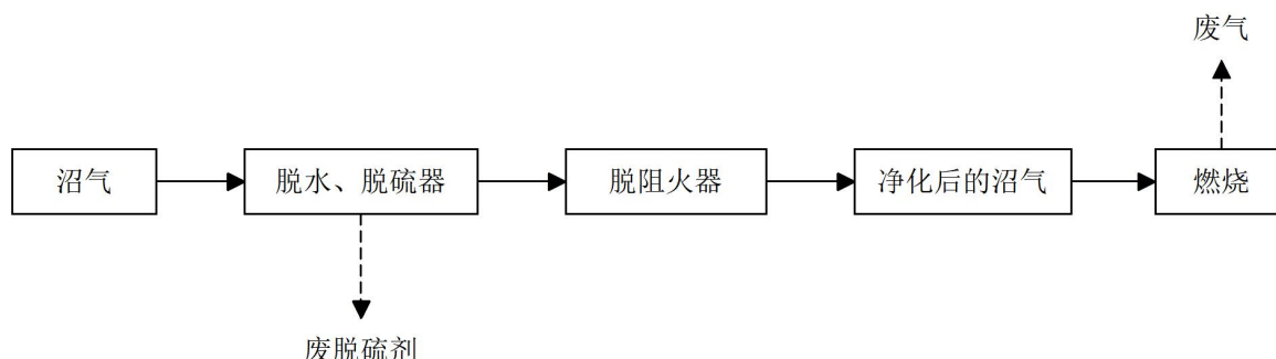
图 3.3-3 沼气燃烧工艺流程图
