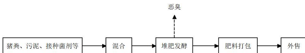
图 3.3-4 有机肥工艺流程图
