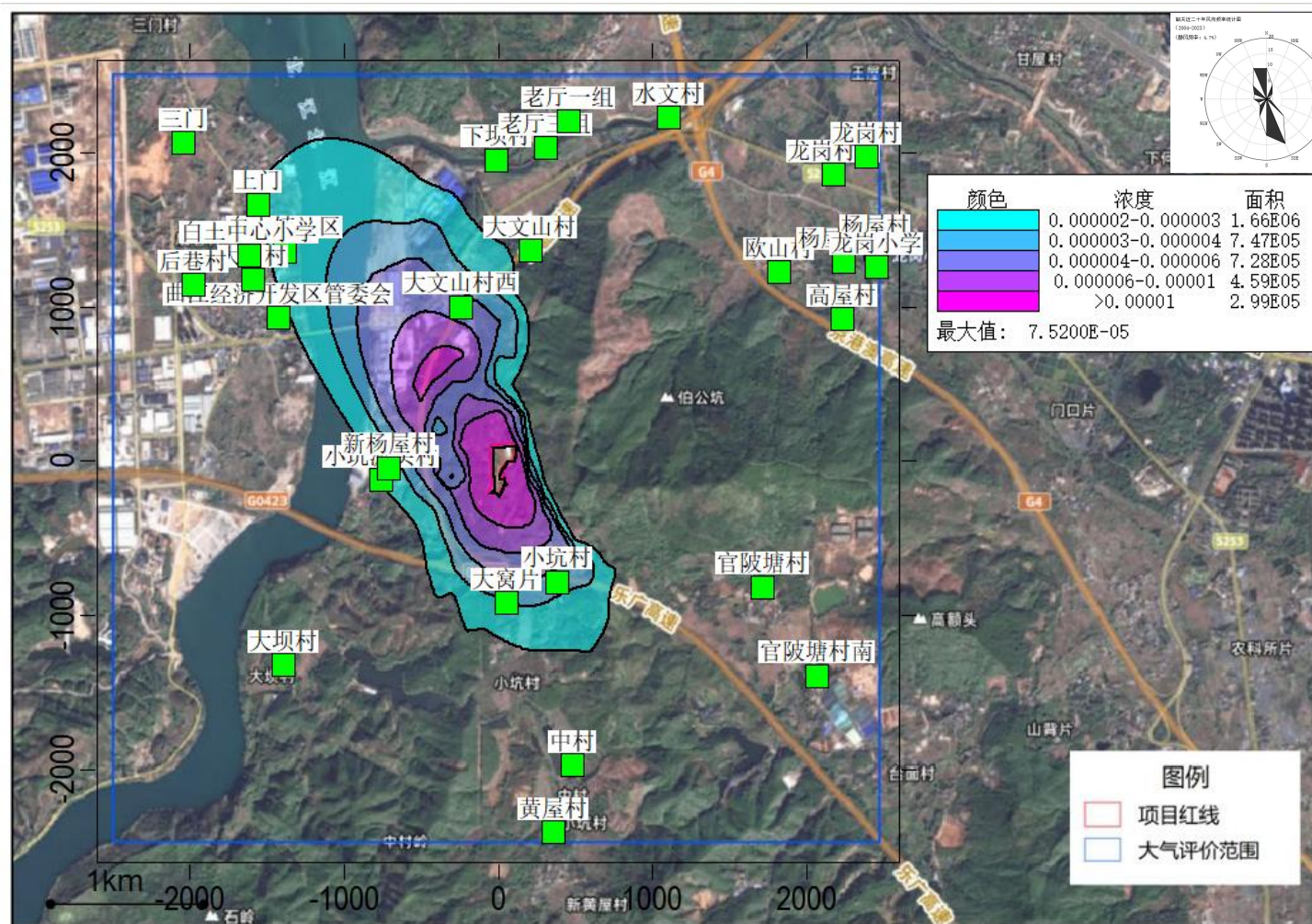
图 5.3-15 正常排放 PM_{10} 年均浓度各点贡献高值分布图 ( mg/m^3 )
