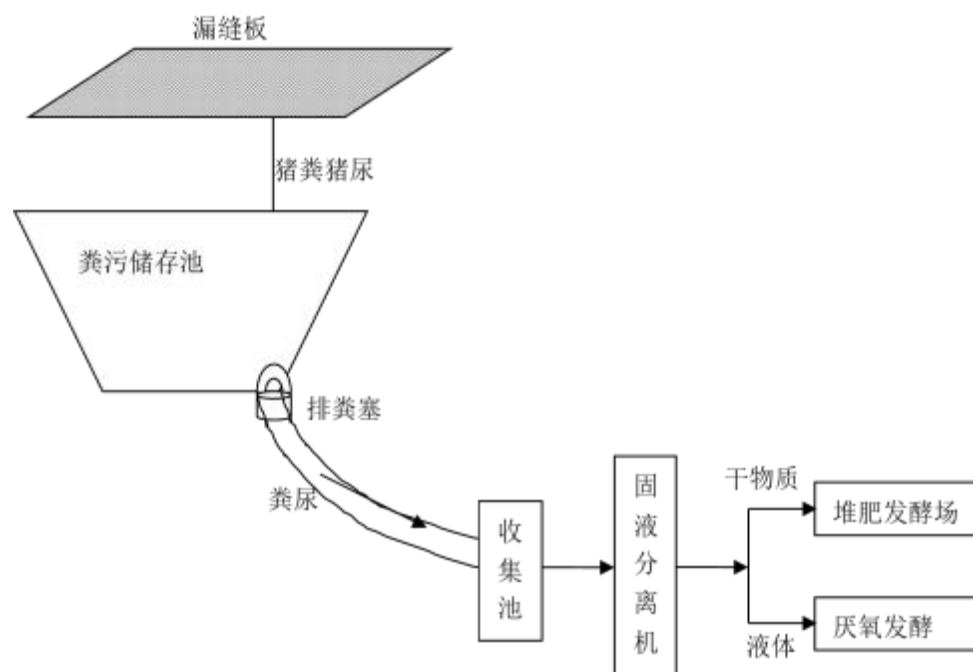
图 3.3-2 粪污处理工艺流程图
