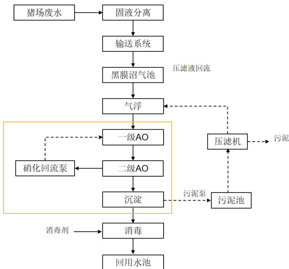
图 6.1-1 废水处理工艺流程图
