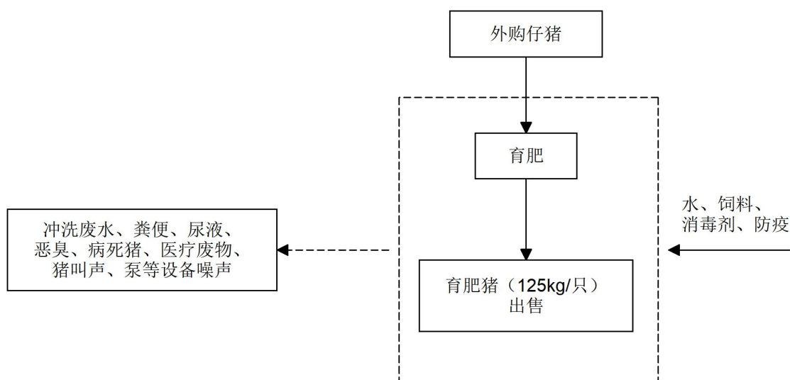
图 3.3-1 建设项目猪场饲养工艺流程图
