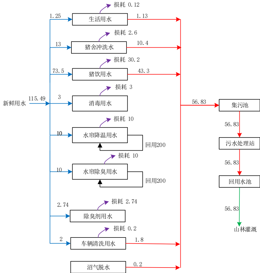
图 2.1-5 项目高温季节日最大水平衡图 (单位: \text{m}^3/\text{d} )
