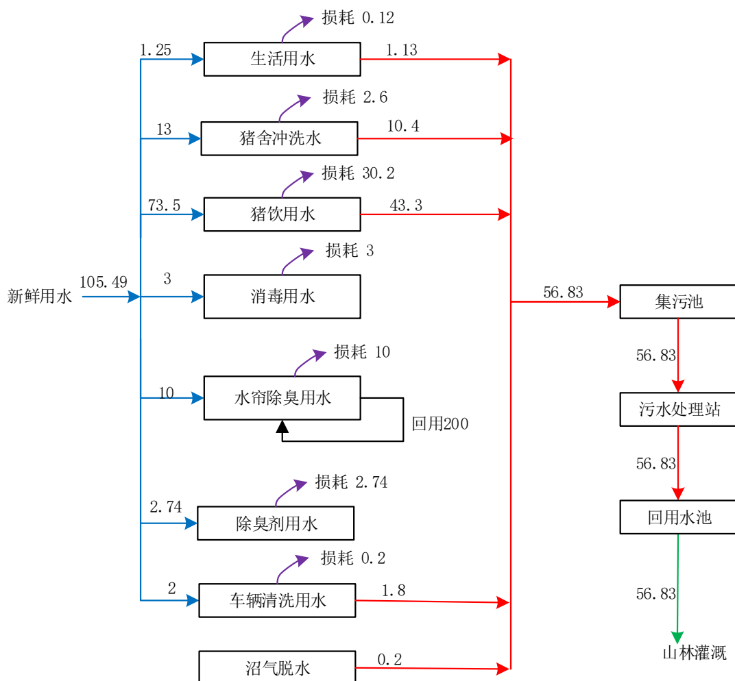
图 2.1-7 项目非高温季节日最大水平衡图（单位：m³/d）
