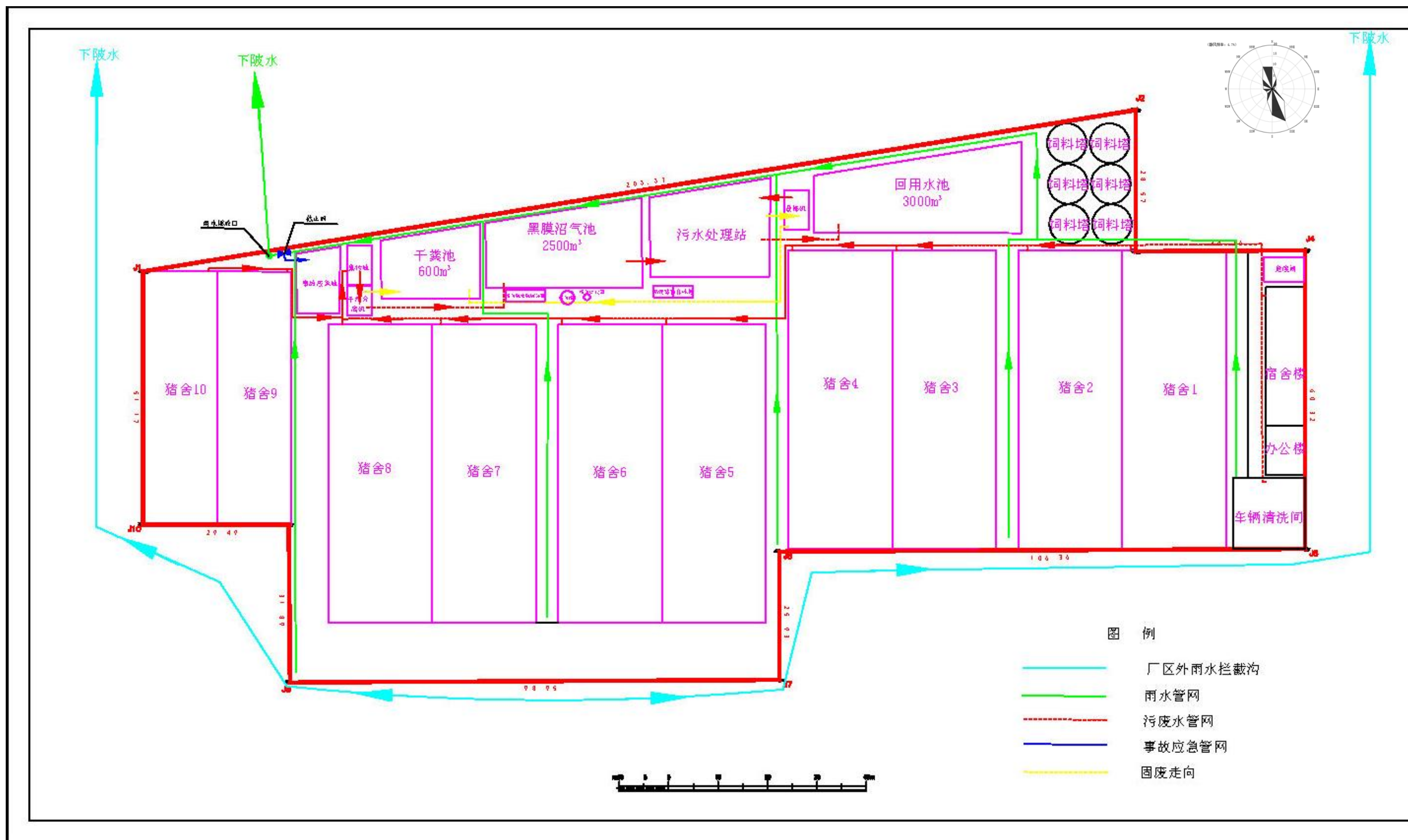
图 2.1-4 项目雨污水管网布设图
