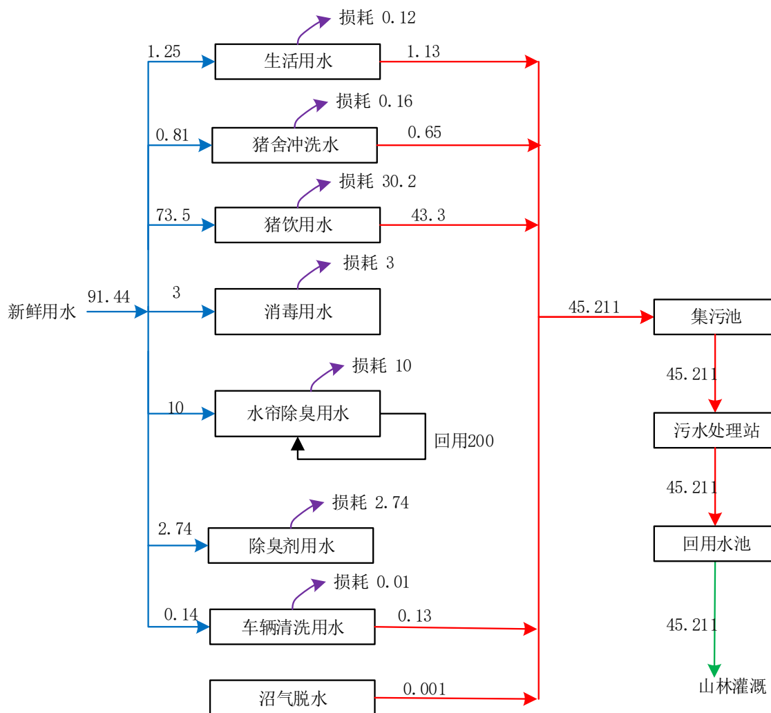
图 2.1-8 项目非高温季节日平均水平衡图 (单位: m³/d)
