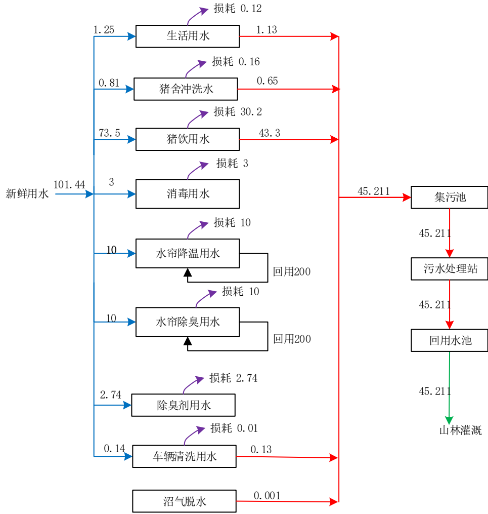
图 2.1-6 项目高温季节日平均水平衡图 (单位: \text{m}^3/\text{d} )
