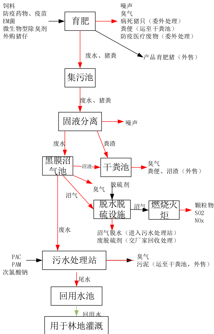
图 2.2-2 项目运营期生产工艺流程图
