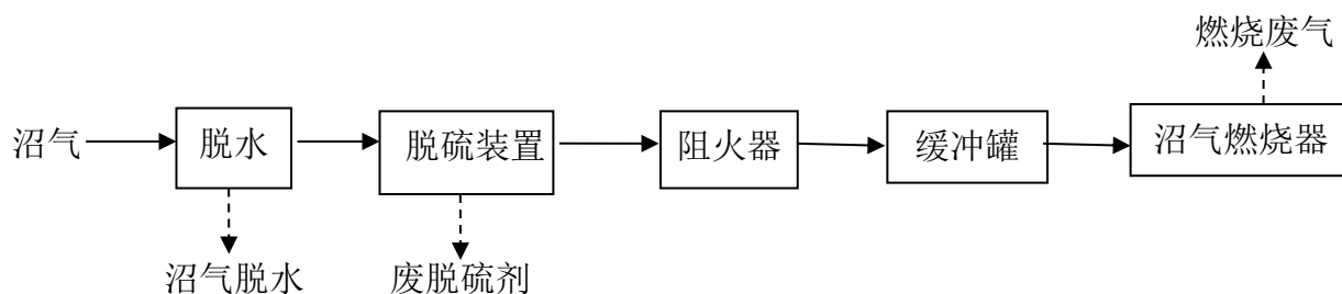
图 2.2-4 项目运营期沼气处理流程及产污环节图
