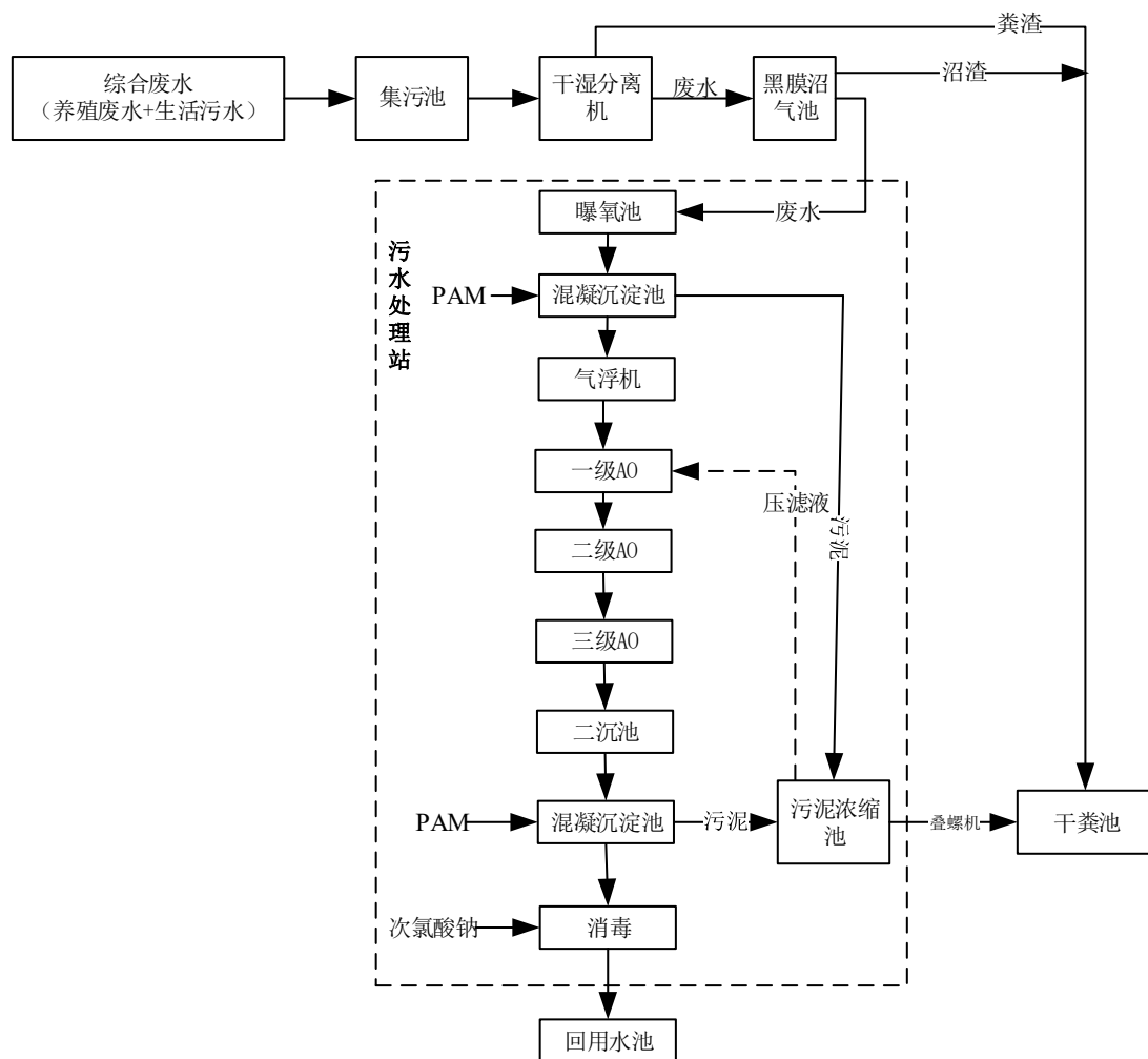
图 4.2-26 废水处理工艺流程图-
