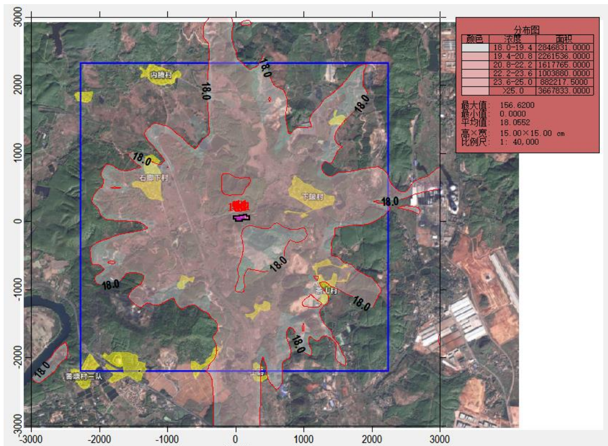
图 4.2-6 正常排放条件下 NH 3 最大 1h 平均浓度叠加值等值线图 (单位: \mu\text{g}/\text{m}^3 )
