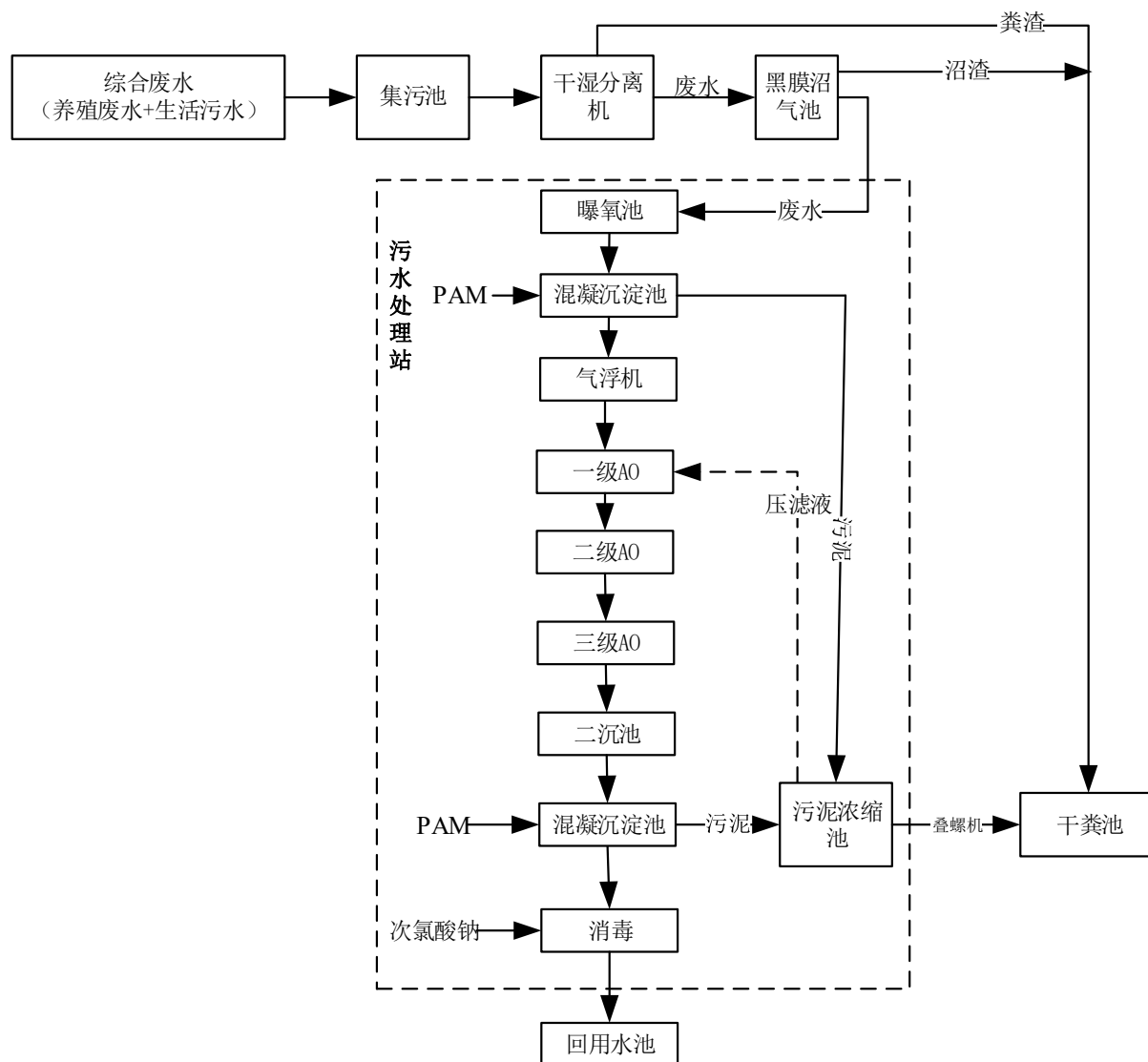
图 6.2-3 项目污水处理工艺流程图
