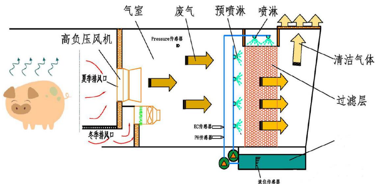
图 6.2-1 猪舍负压抽风除臭系统工作原理示意图
