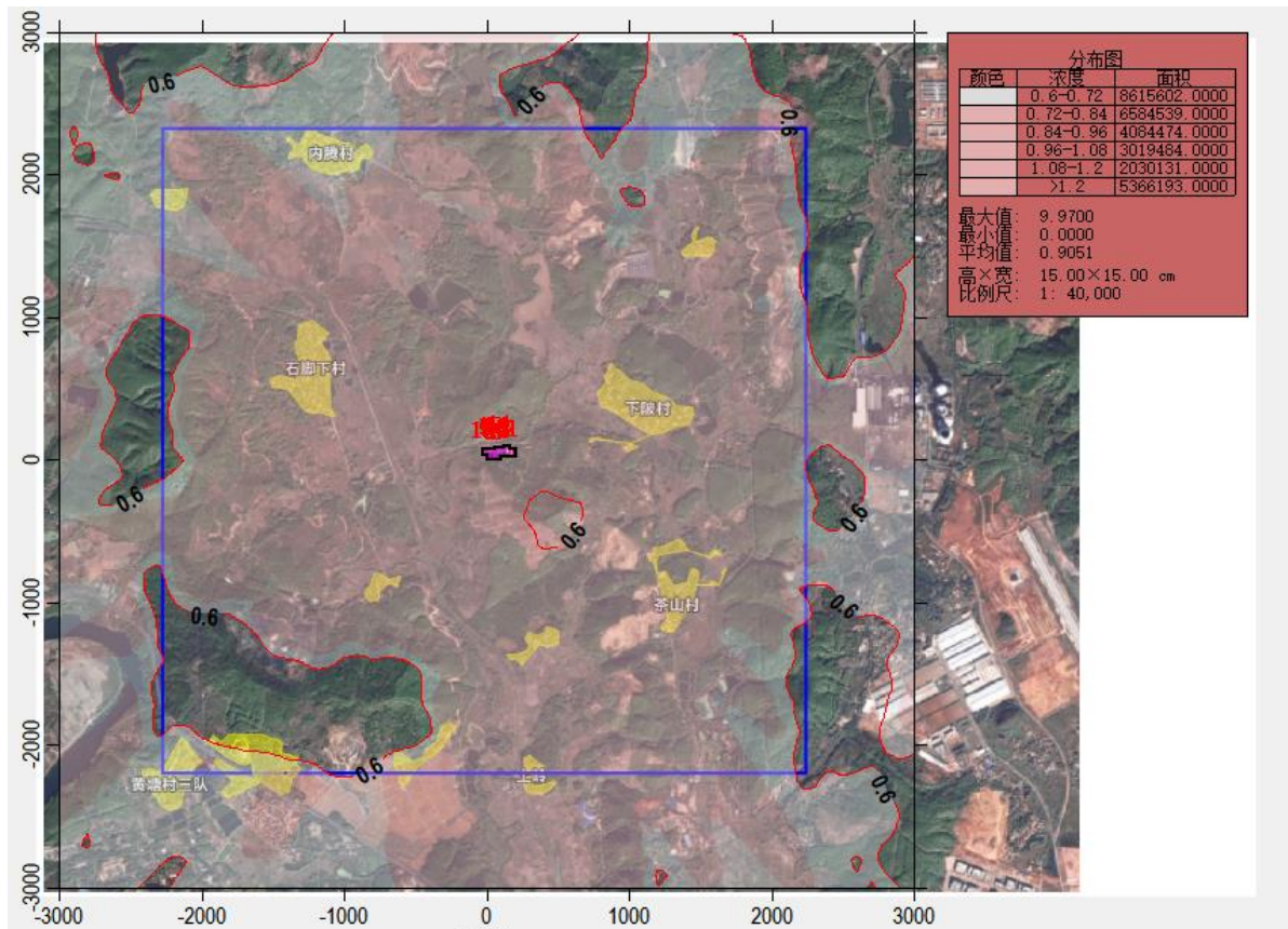
图 4.2-7 正常排放条件下 H 2 S 最大 1h 平均浓度叠加值等值线图 (单位: \mu\text{g}/\text{m}^3 )
