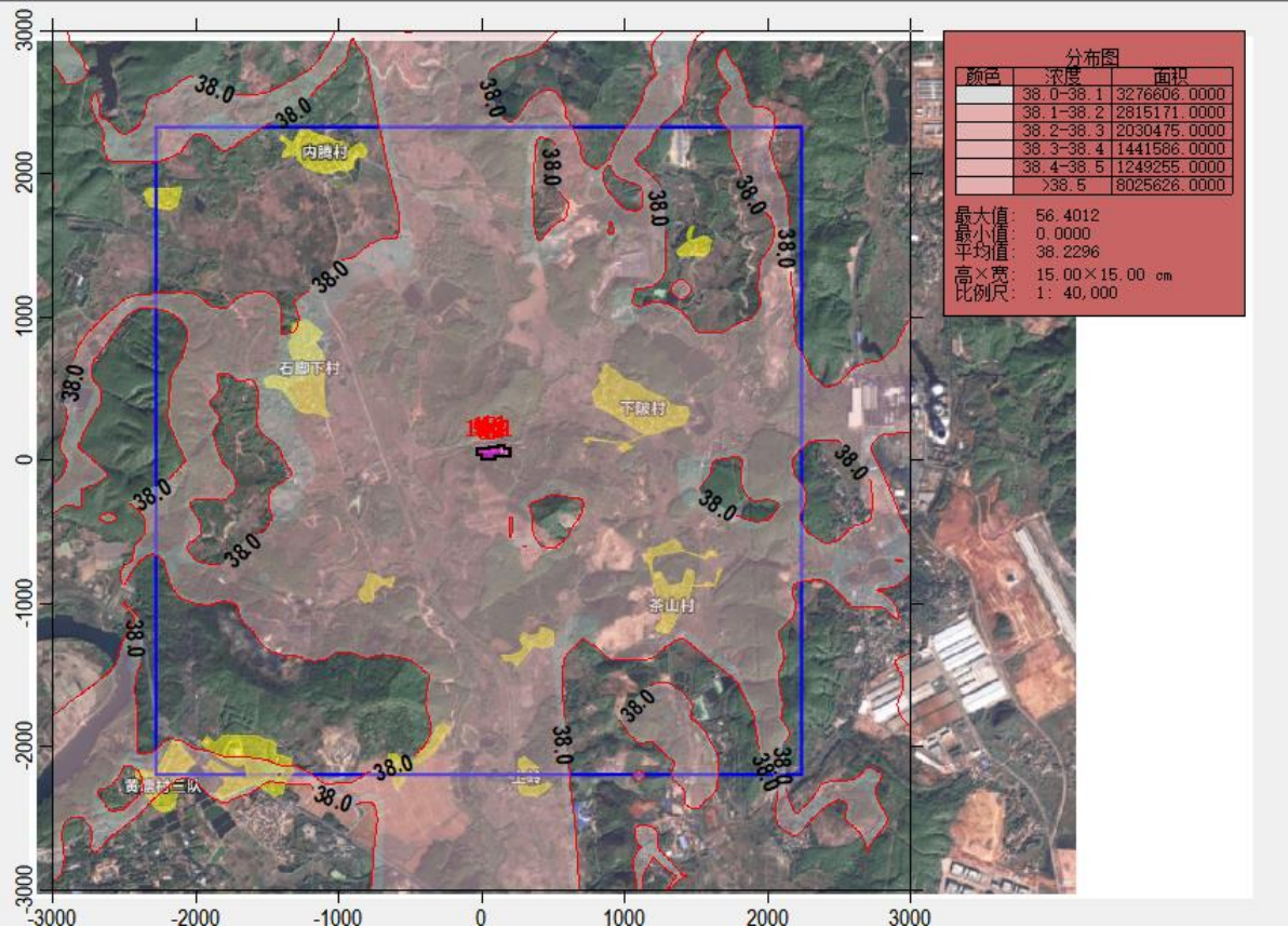
图 4.2-12 正常排放条件下 NO x 最大 1h 平均浓度叠加值等值线图 (单位: \mu\text{g}/\text{m}^3 )
