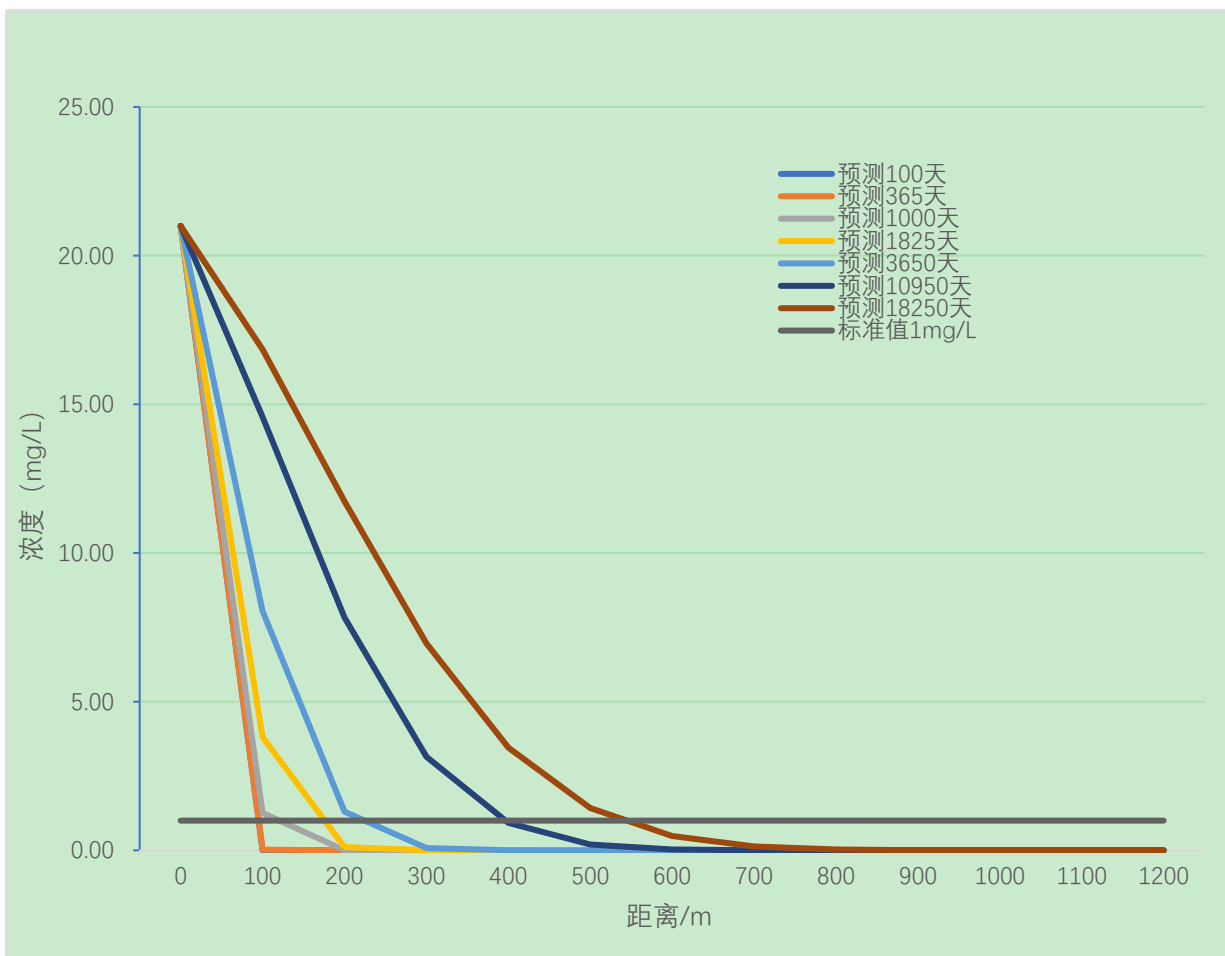
图 4.2-31 非正常工况下锌运移范围预测结果图
