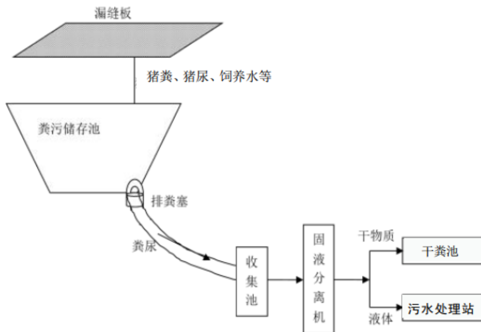
图 2.2-3 项目运营期生产工艺流程图
