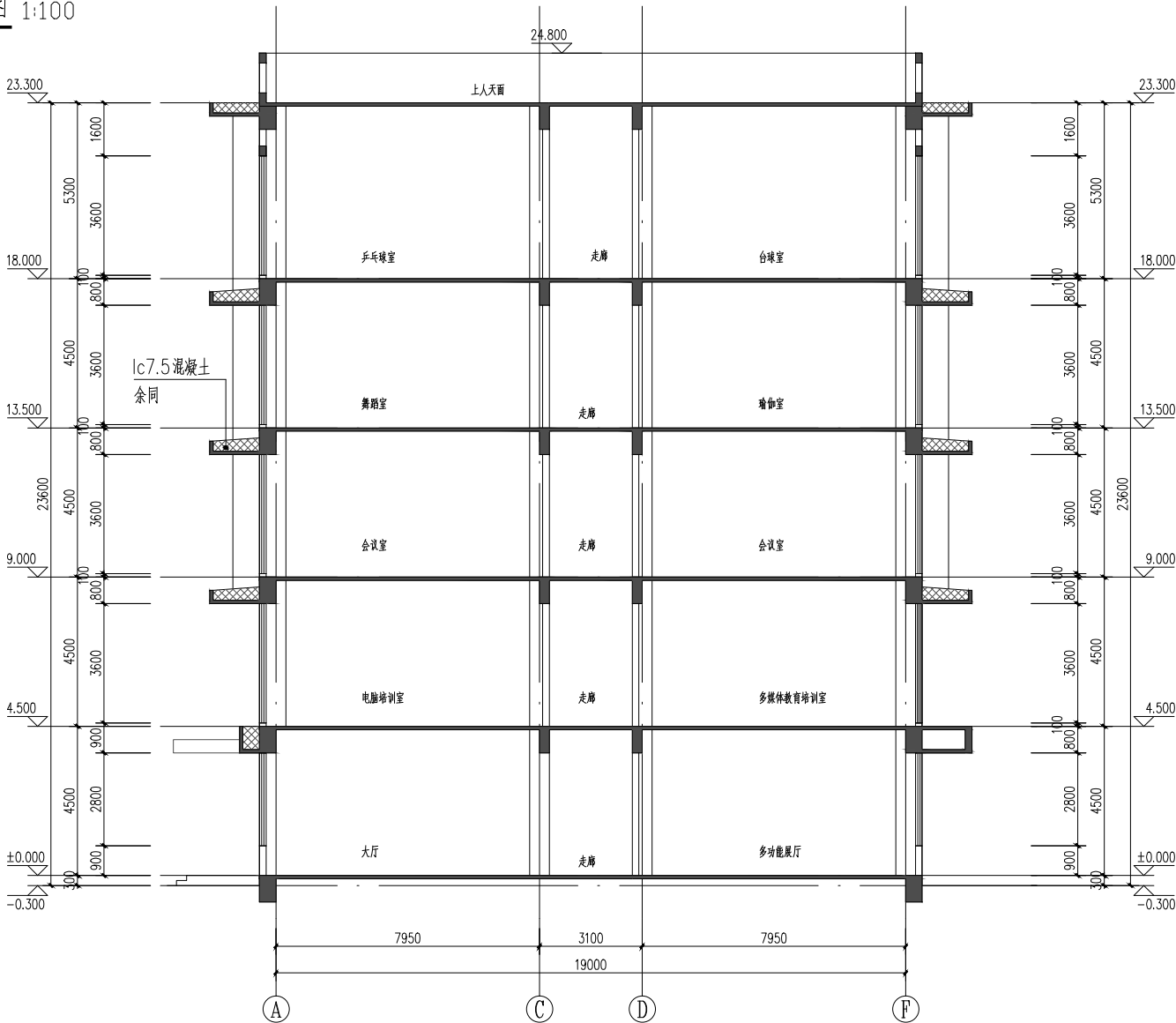
1-1 剖面图 1:100
