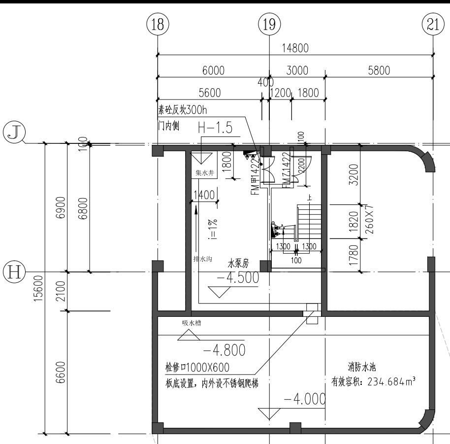
地下层平面图 1:200
