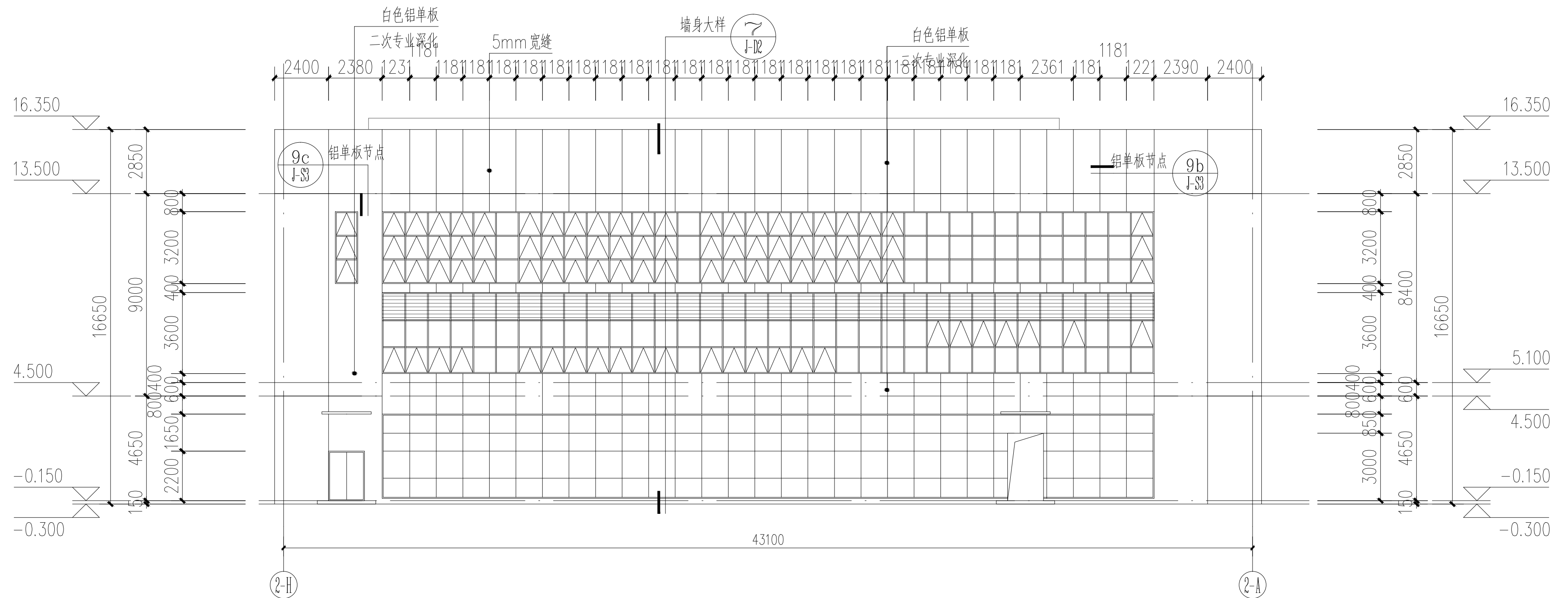
②A~②H轴立面图 1:200
