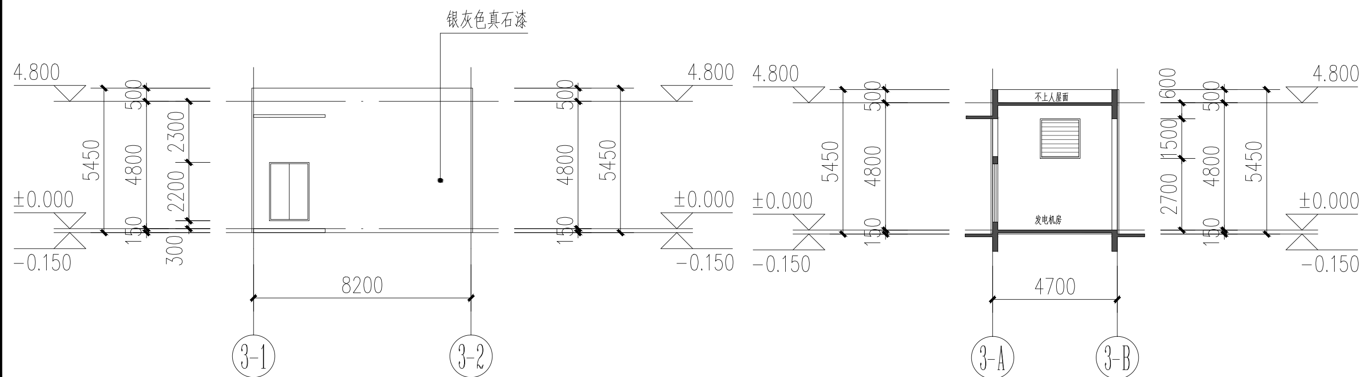
发电机房③~②轴立面图 1:200
