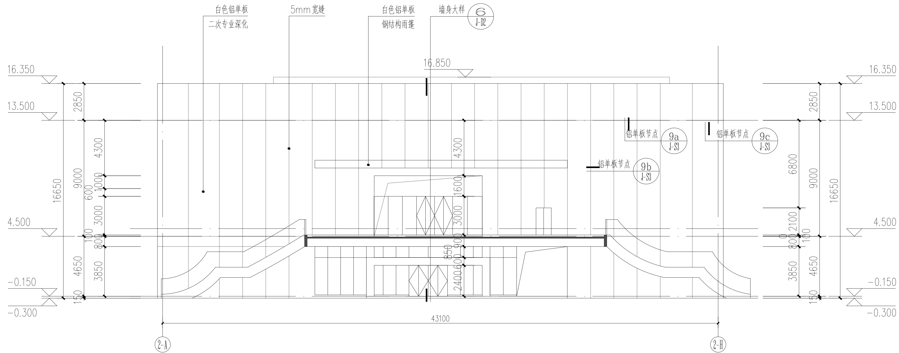
②A~②H轴立面图 1:200
