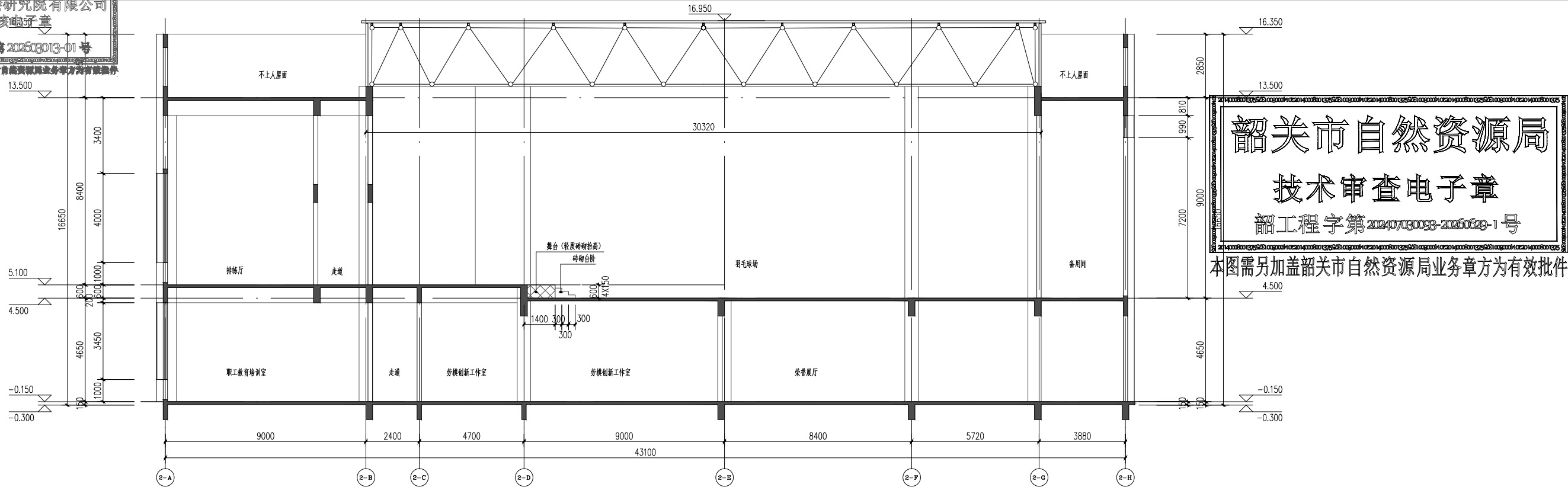
1-1 剖面图 1:100
