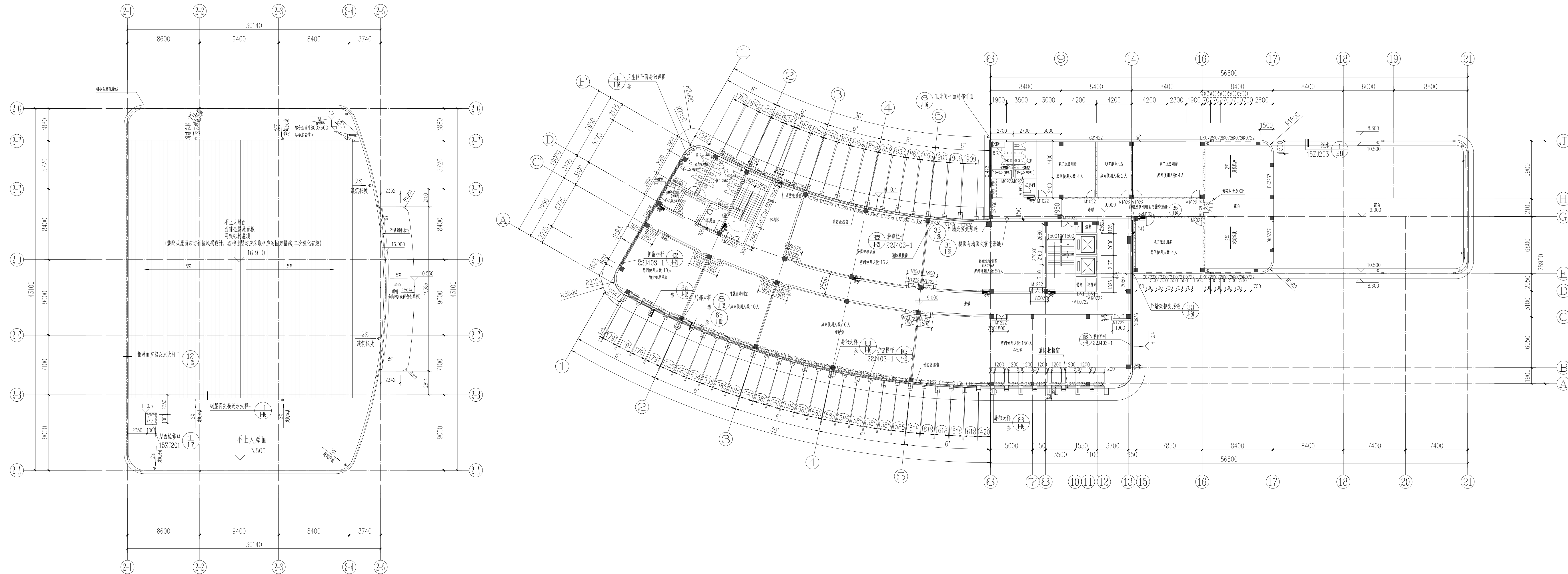
三层平面图 1:200
