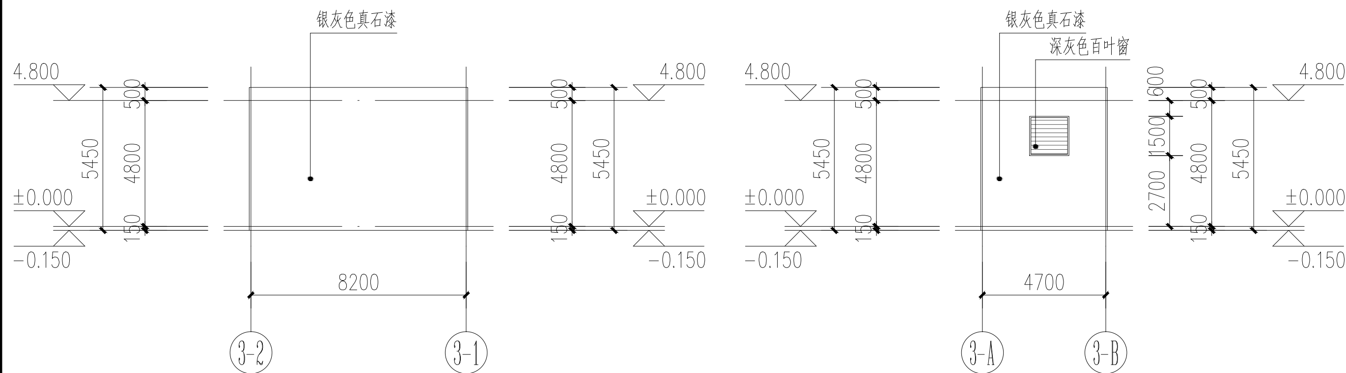
发电机房③~①轴立面图 1:200
