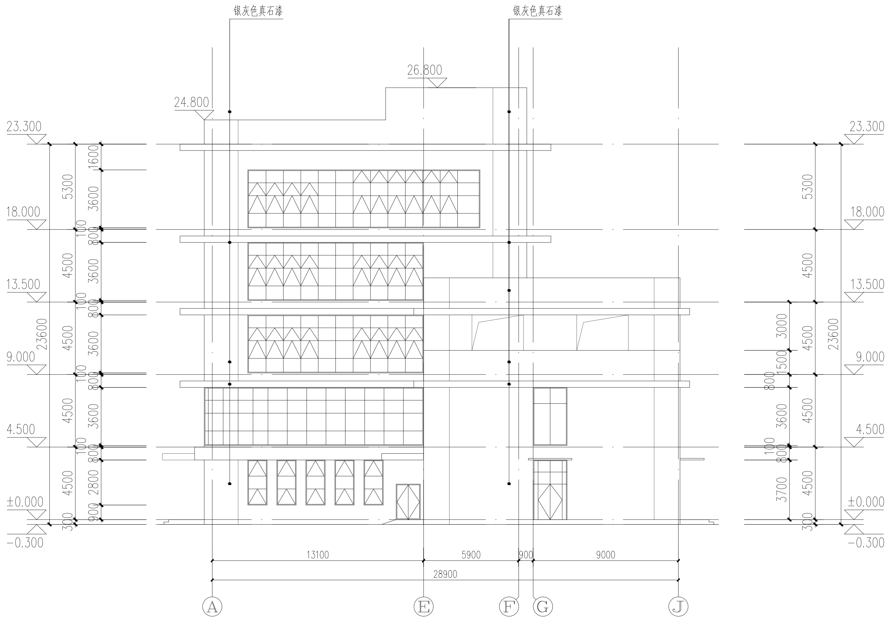
①~③轴立面图 1:200
