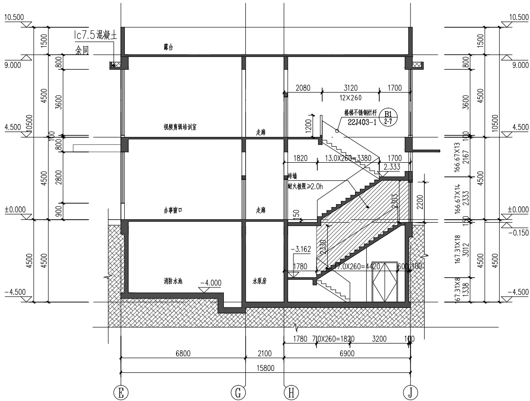
3-3 剖面图 1:100
