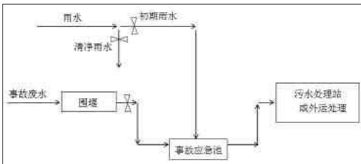
图 7.5-1 事故废水截流、收集及处理流程图
