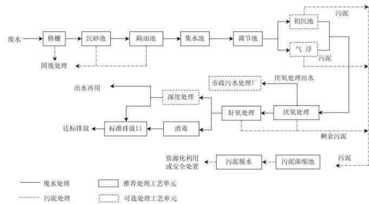
图 8.2-2 屠宰与肉类加工废水治理工程典型工艺流程图
