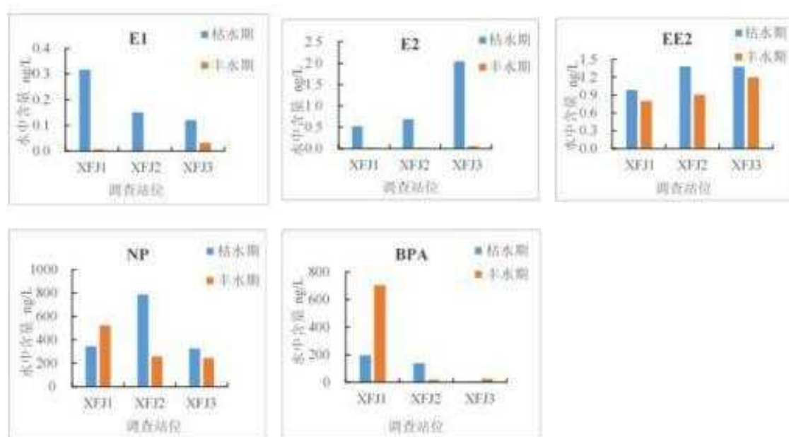
图 4.6-7 2023 年新丰江国家级水产种质资源保护区水体 EDCs 含量
