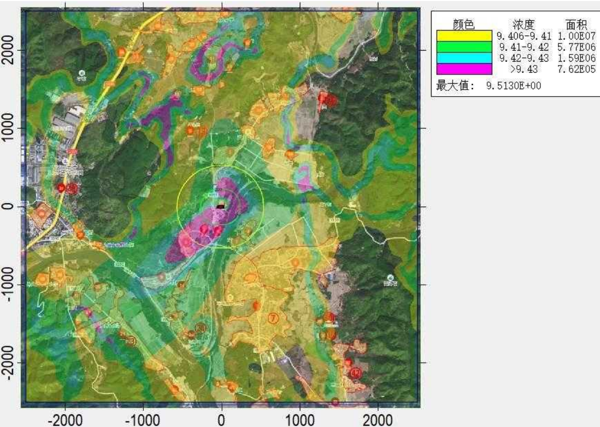
图 6.3-12b NO 2 叠加现状值后年均质量浓度分布图 (单位 \mu\text{g}/\text{m}^3 )
