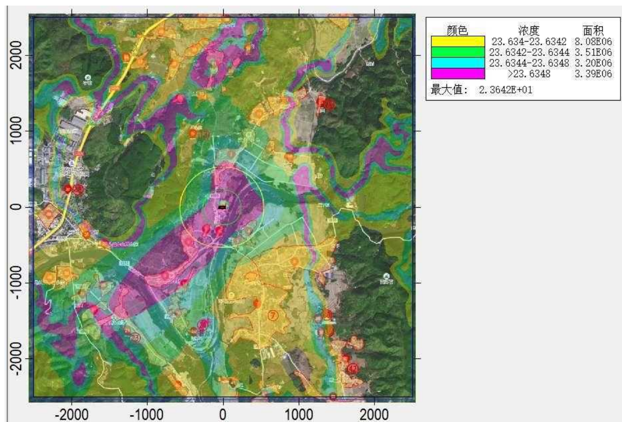
图 6.3-14b PM 2.5 叠加现状值后年均质量浓度分布图 (单位 \mu\text{g}/\text{m}^3 )
