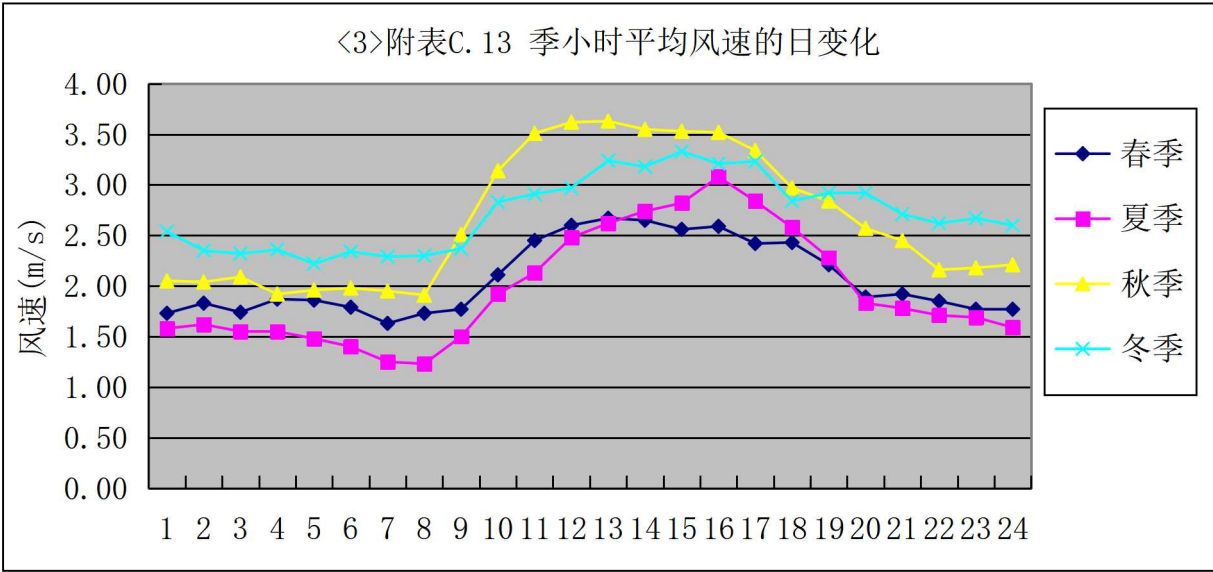
图 6.3-4 区域季小时平均风速的日变化图
