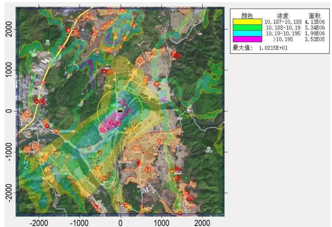
图 6.3-11b SO 2 叠加现状值后年均质量浓度分布图 (单位 \mu\text{g}/\text{m}^3 )
