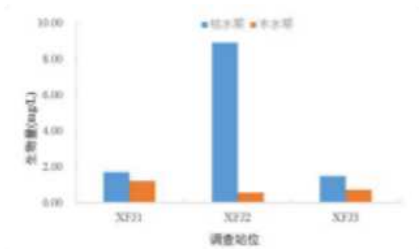
图 4.6-11 2023 年新丰江国家级水产种质资源保护区浮游植物生物量
