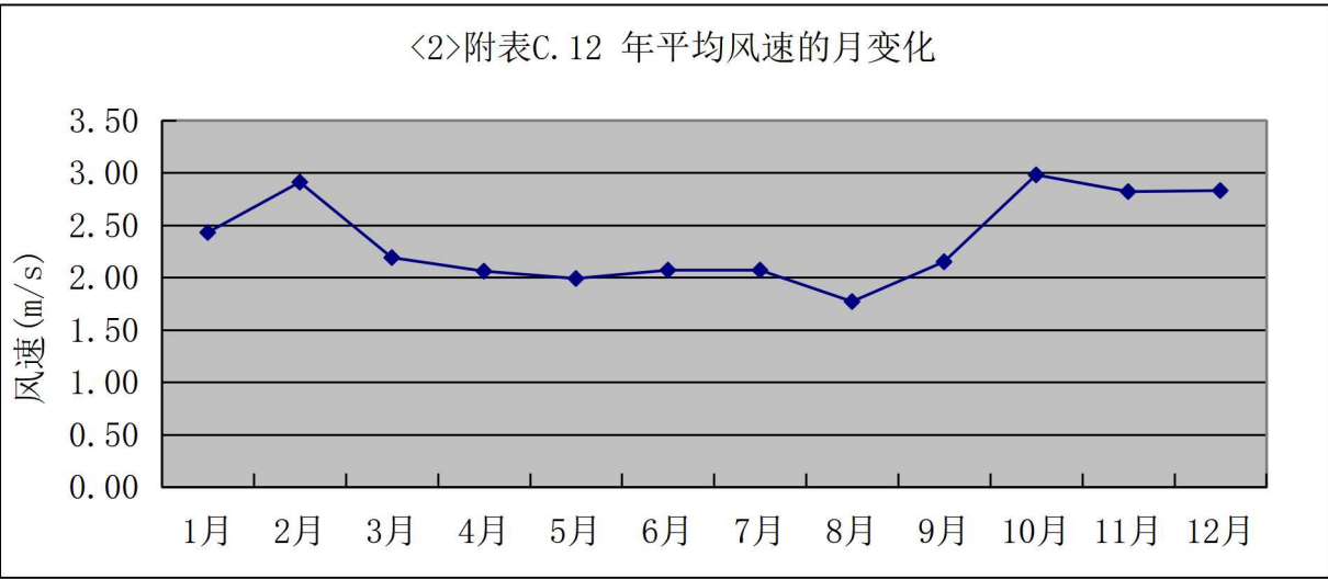
图 6.3-3 区域月平均风速变化图
