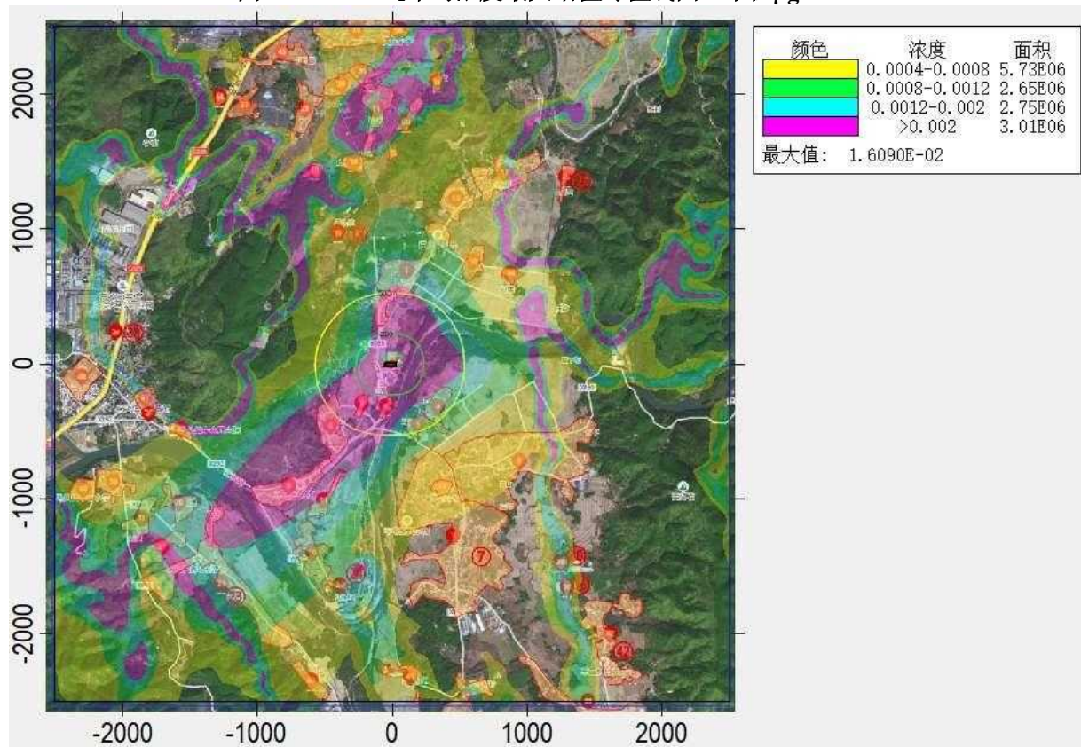
图6.3-10c PM 10 年均浓度最大增值等值线图 (单位 \mu\text{g}/\text{m}^3 )
