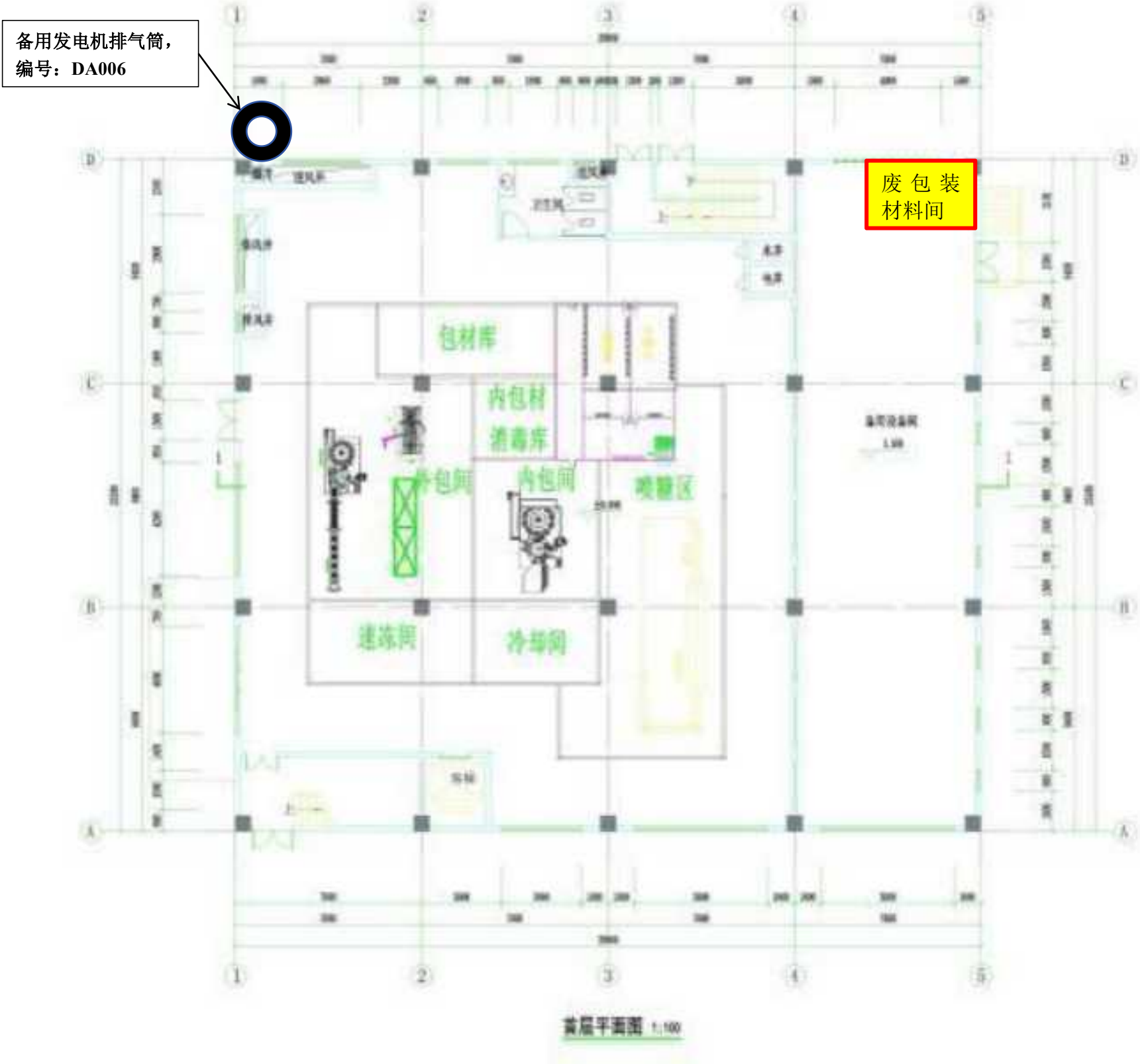
图 3.1-4b (2 号)厂房平面布置图 (1 层)
