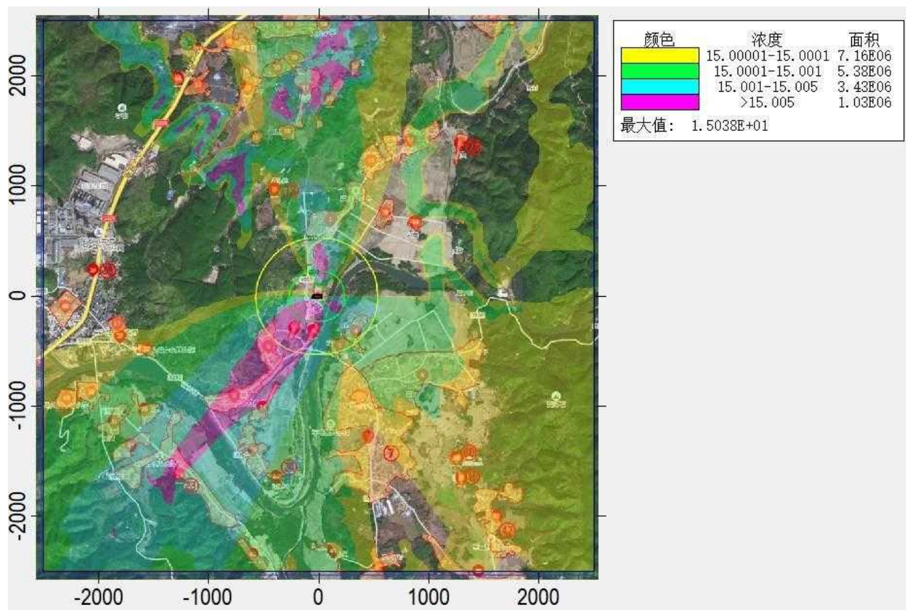
图 6.3-11a SO 2 叠加现状值后 98%保证率日均质量浓度分布图 (单位 \mu\text{g}/\text{m}^3 )
