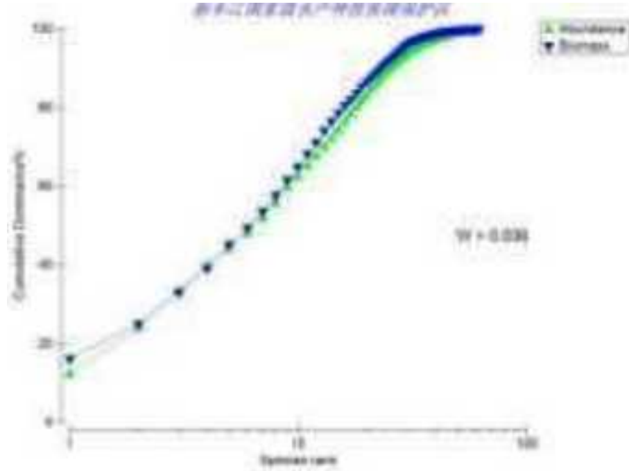
图 4.6-19 新丰江国家级水产种质资源保护区鱼类群落稳定性 abc 曲线图
