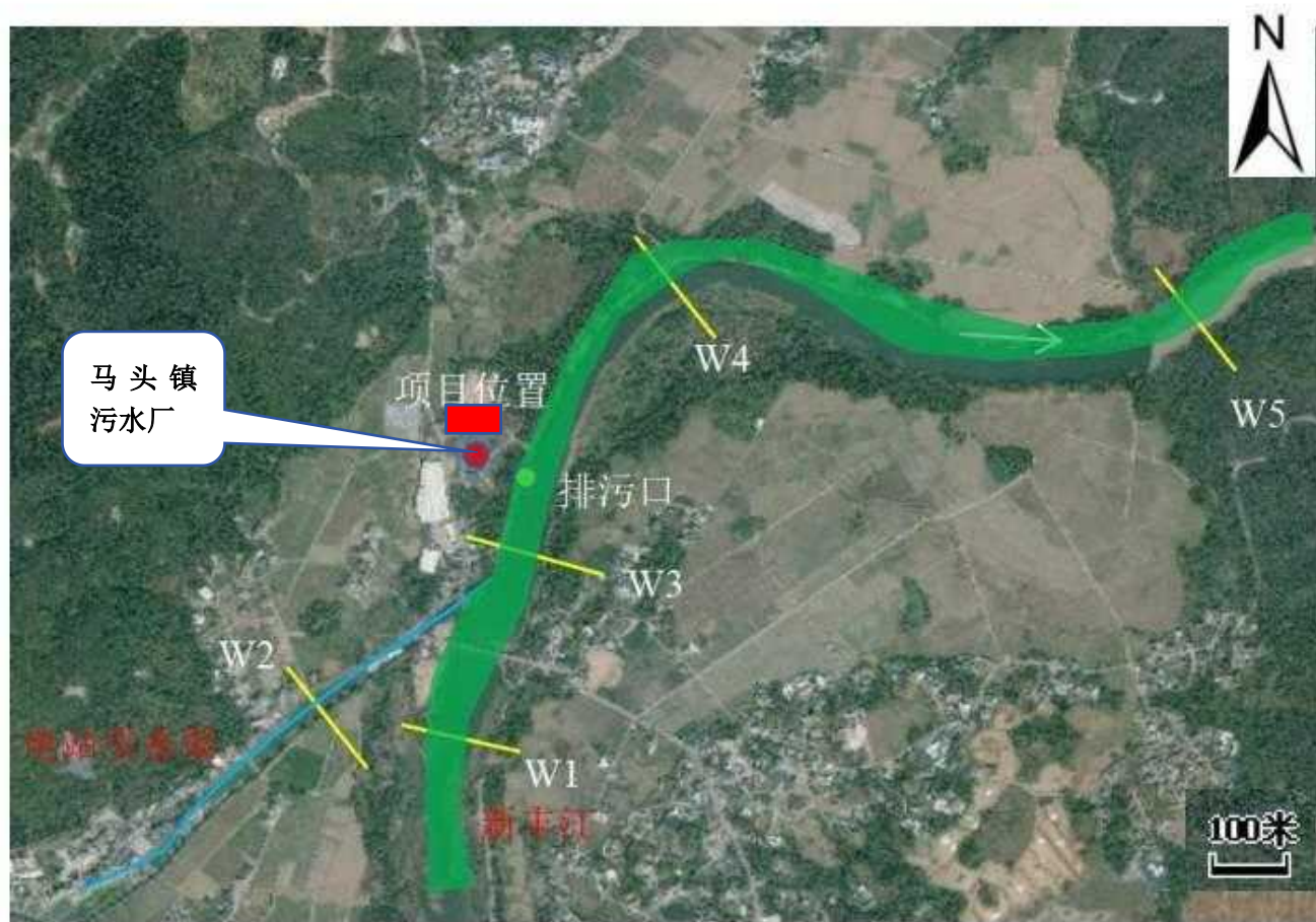
图 4.3-2b 引用报告（枯水期）地表水环境质量监测点位图
