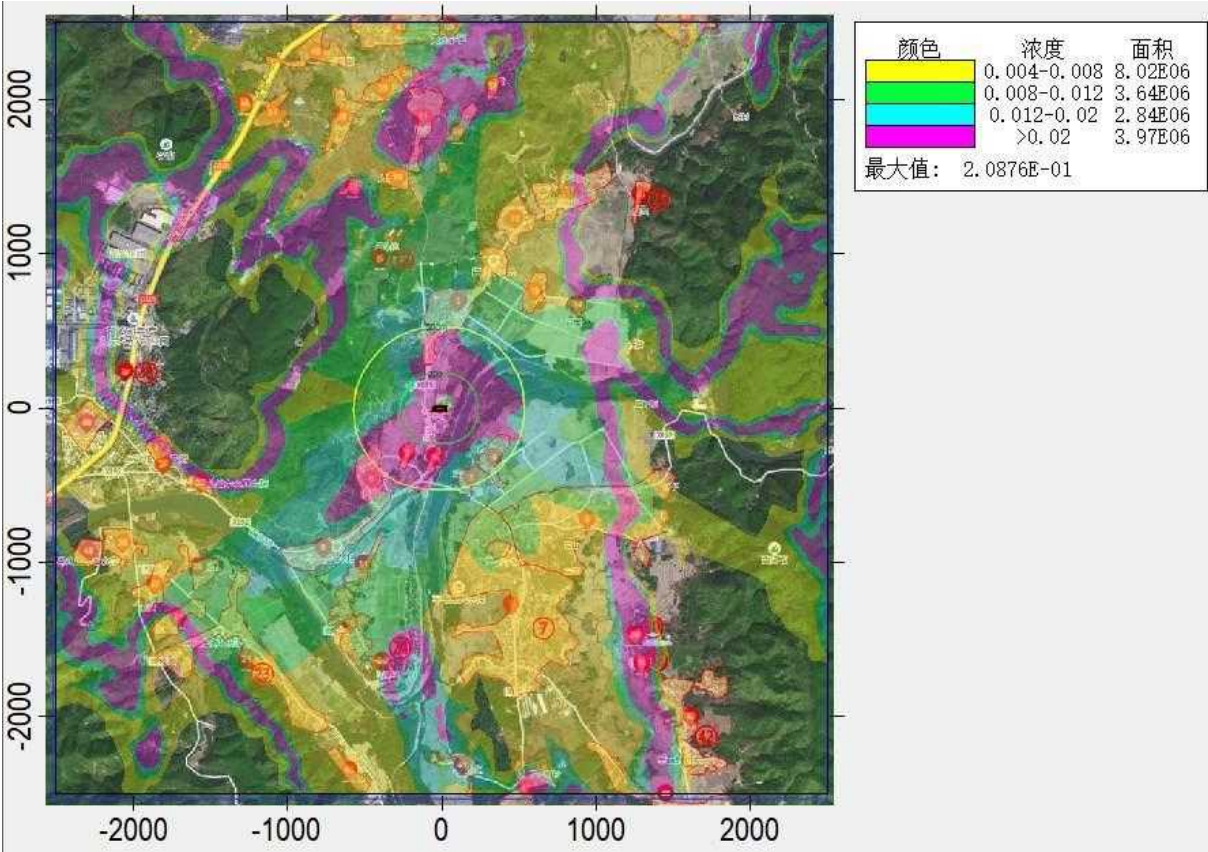
图 6.3-9c PM 10 日均浓度最大增值等值线图 (单位 \mu\text{g}/\text{m}^3 )
