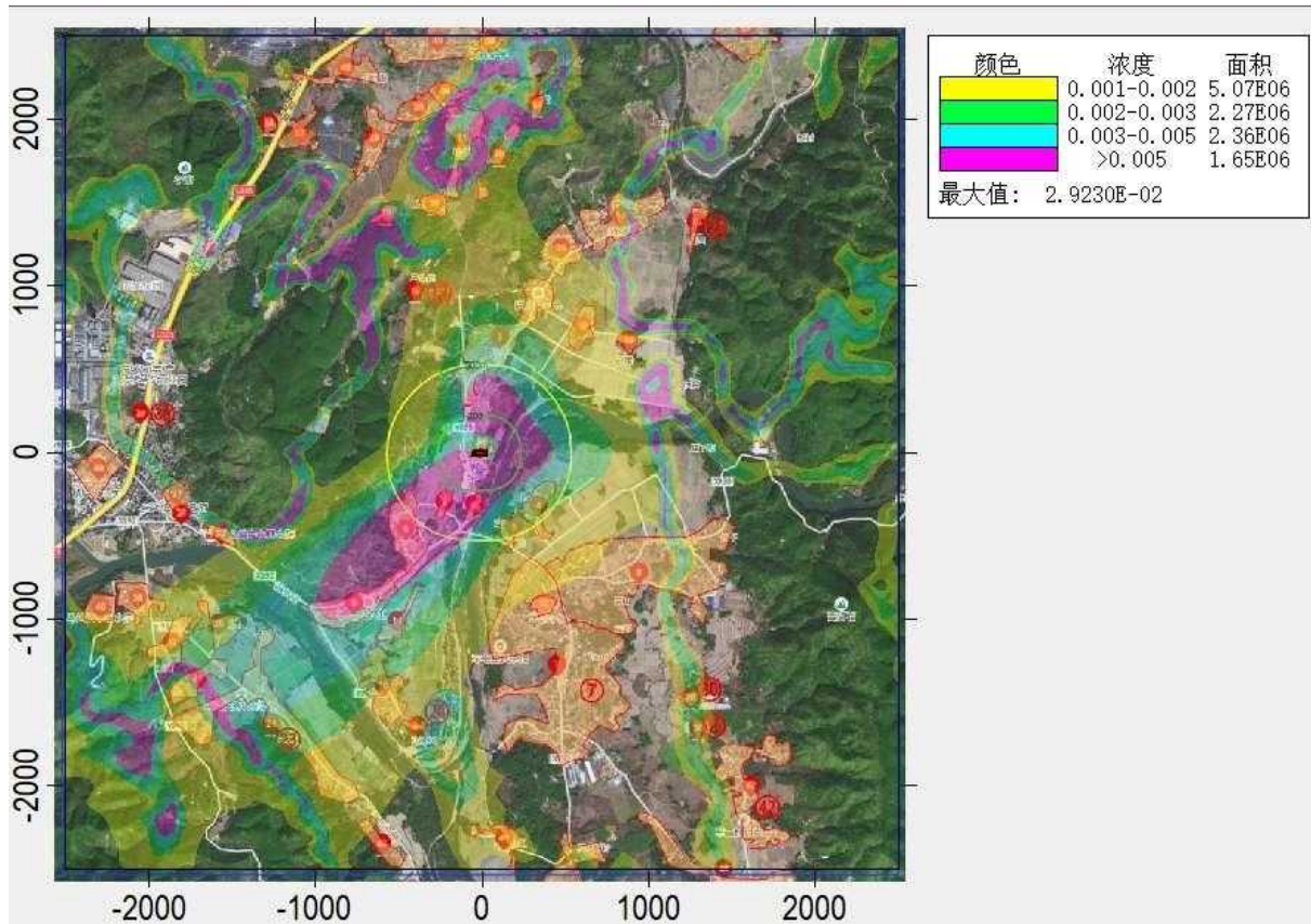
图6.3-10a SO 2 年均浓度最大增值等值线图 (单位μg/m 3 )
