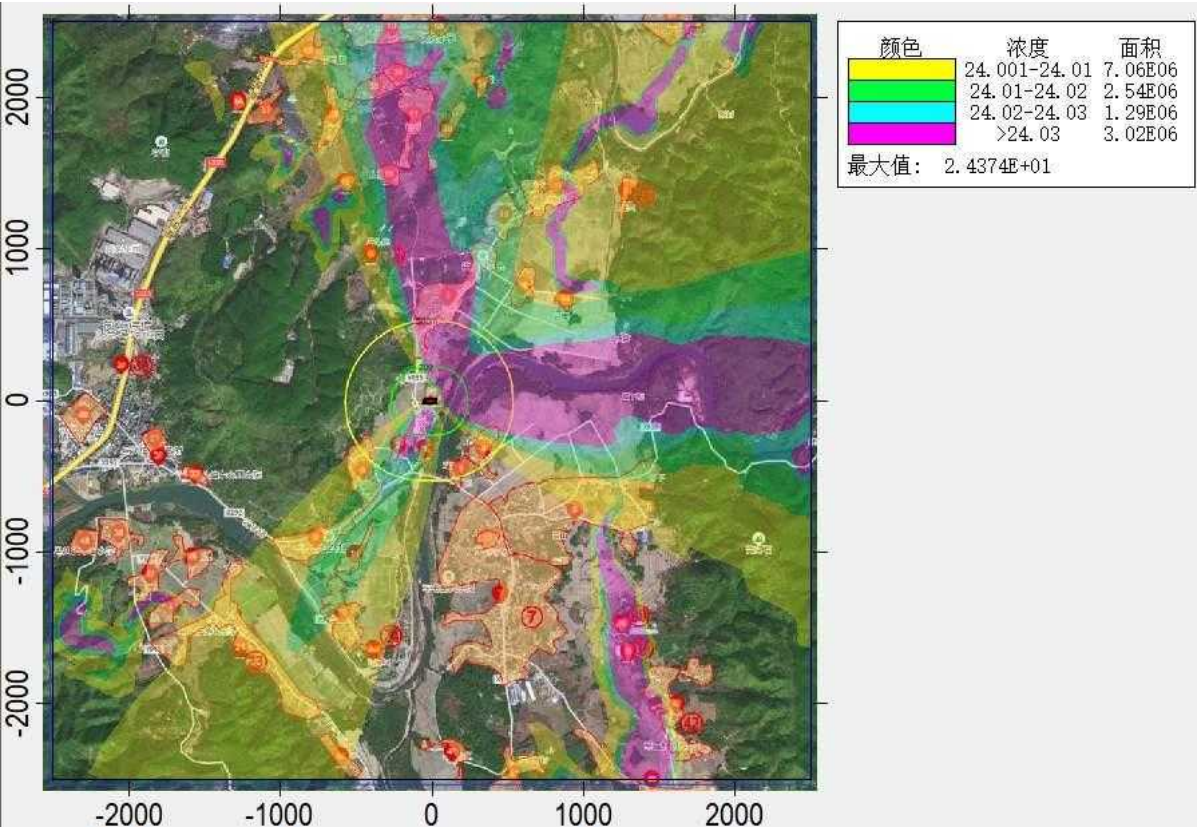
图 6.3-12a NO 2 叠加现状值后 98%保证率日均质量浓度分布图 (单位 \mu\text{g}/\text{m}^3 )
