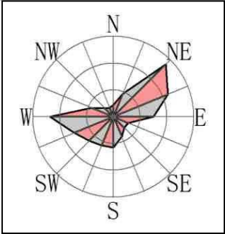
图6.3-1 累年各季风向玫瑰图（统计年限：2005-2024年）
