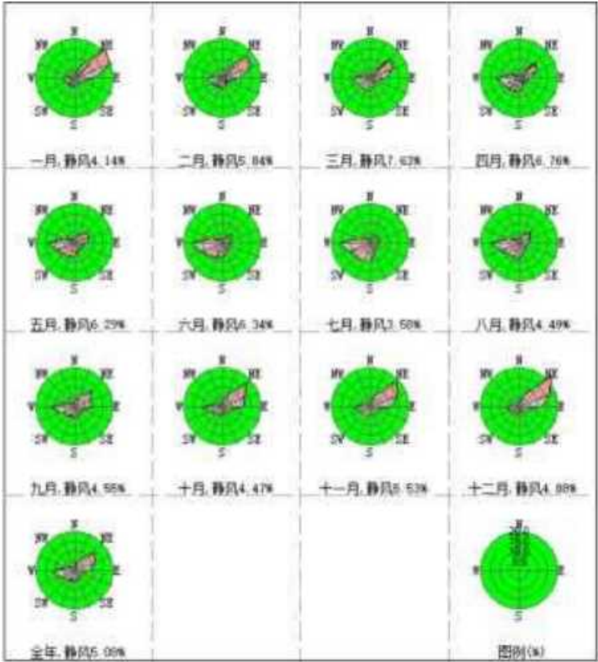
图 6.3-5 新丰 2024 年风玫瑰图
