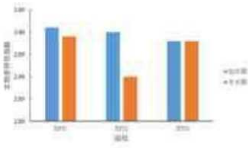
图 4.6-15 2023 年新丰江国家级水产种质资源保护区浮游动物生物多样性指数分布
