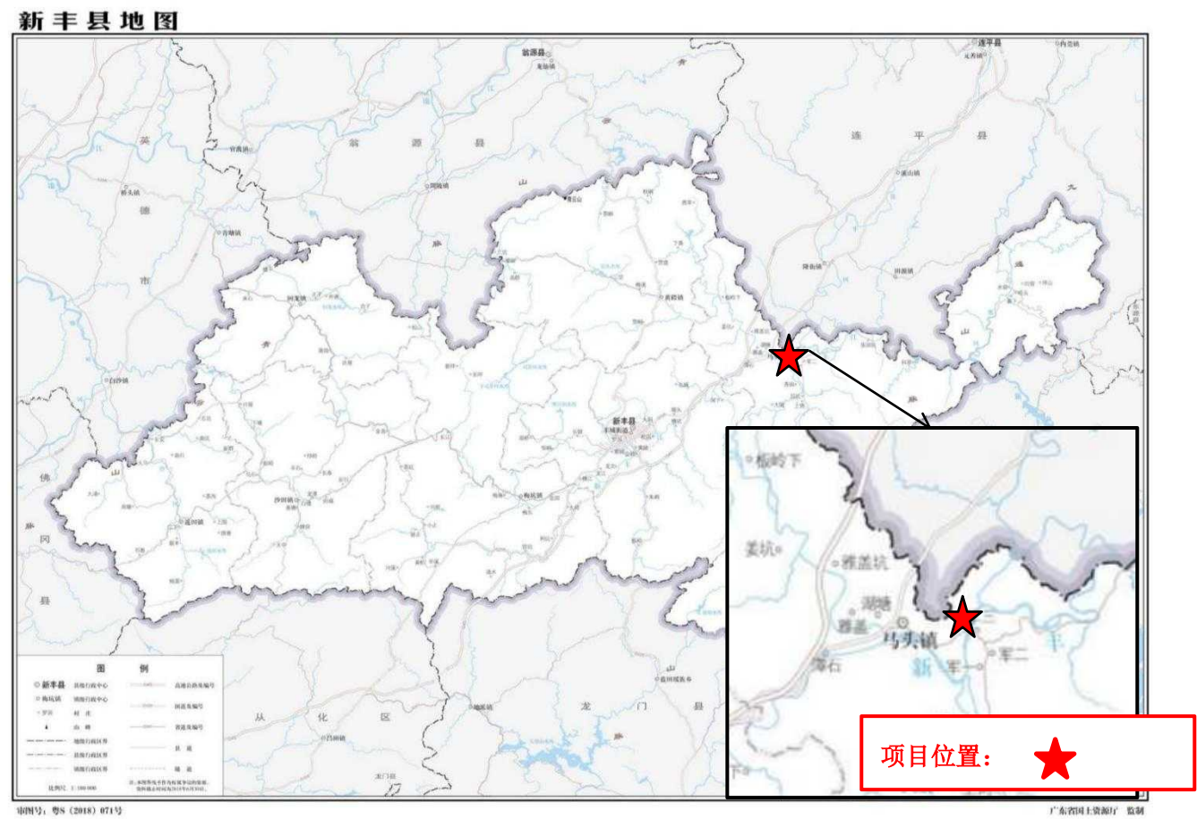
图 1.1-1 项目地理位置图
