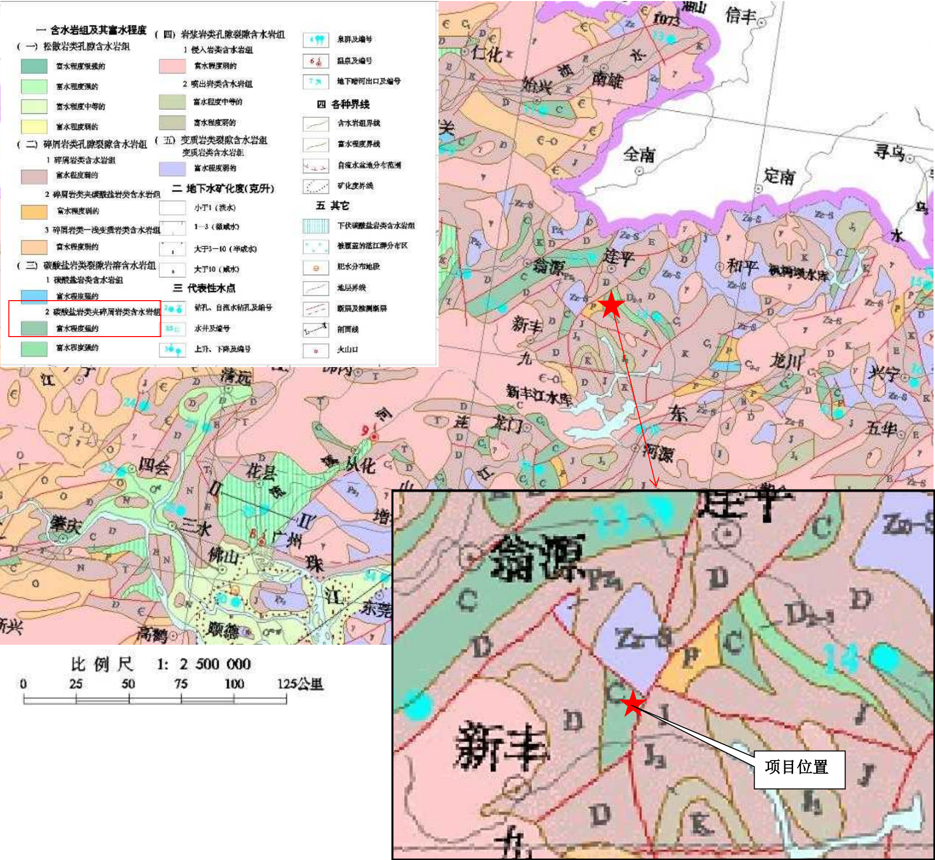
图 6.2-1 广东省水文地质图
