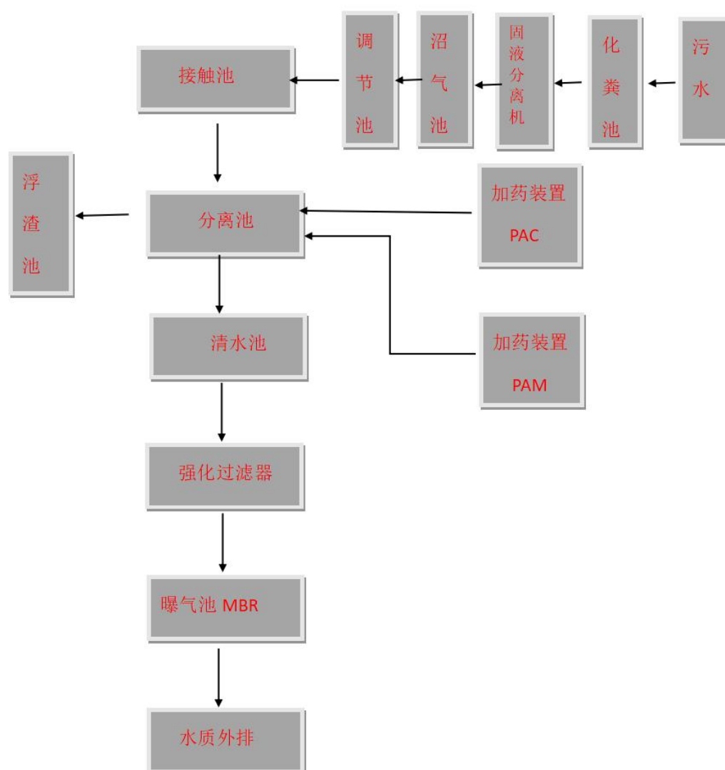
图 8.2-1 养殖废水处理工艺流程图
