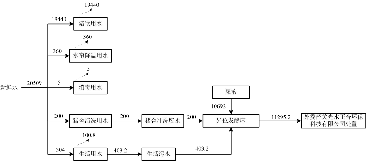
图 4.1-2 项目水平衡图单位：m³/a
