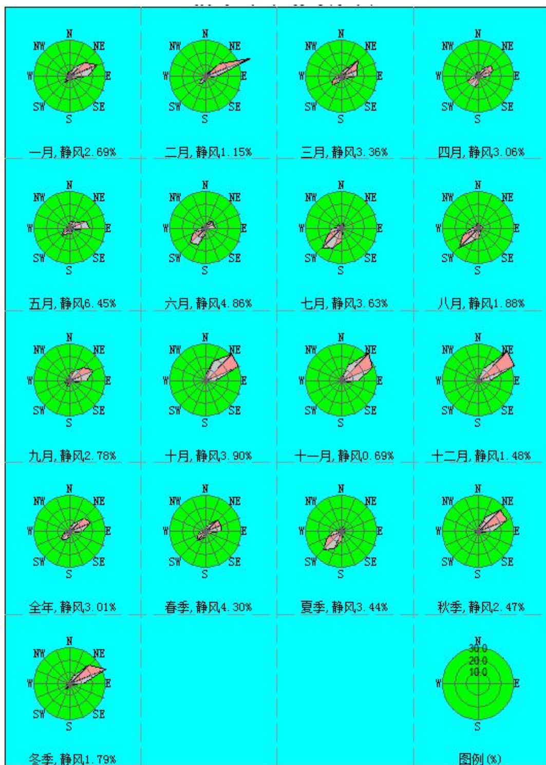
图 6.2-6 南雄 2024 全年各季风频玫瑰图
