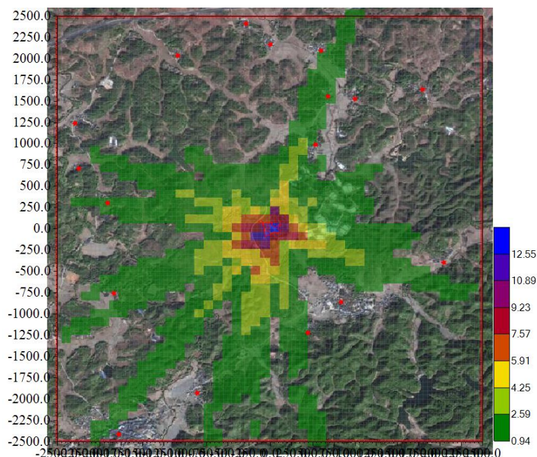
图 6.2-8 本项目 \text{H}_2\text{S} 最大小时浓度影响 ( \mu\text{g}/\text{m}^3 )
