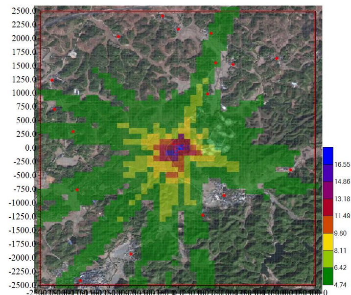
图 6.2-10H 2 S1 小时平均浓度叠加预测等值线图
