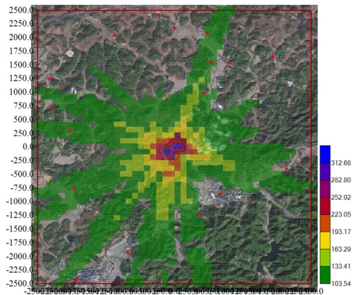
图 6.2-9NH 3 1 小时平均浓度叠加预测等值线图
