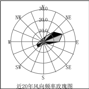
图 6.2-1 南雄气象站近 20 年(2005-2024)风向频率玫瑰图
