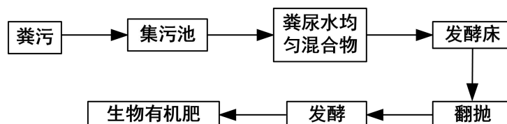
图3.2-2猪粪处理工艺图
