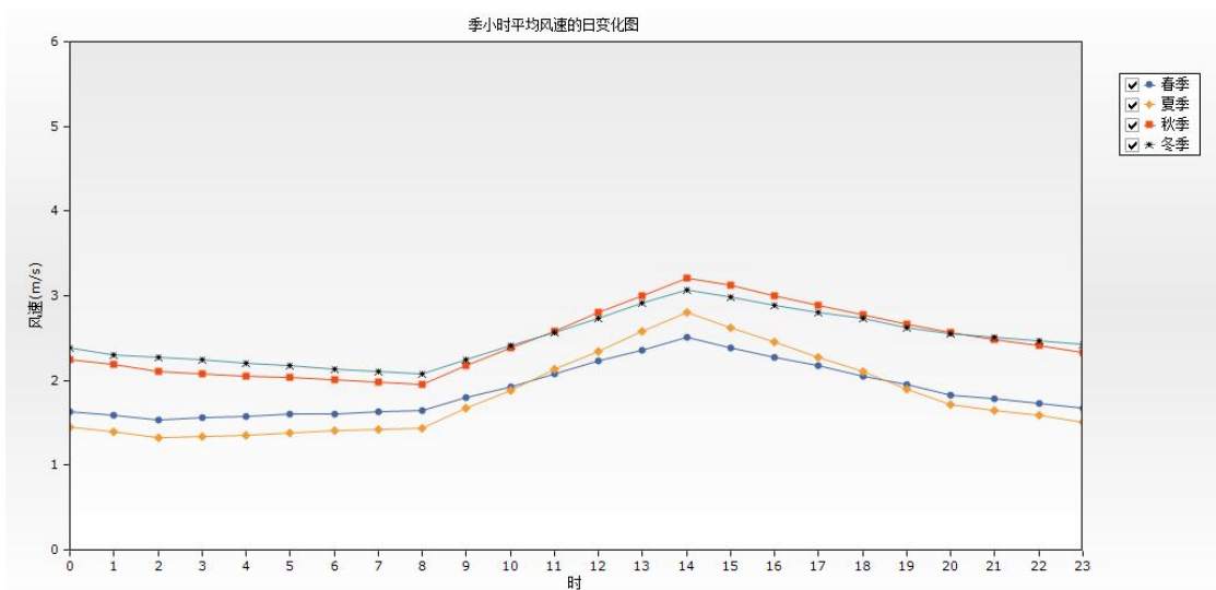
图 6.2-5 各季平均风速日变化曲线图
