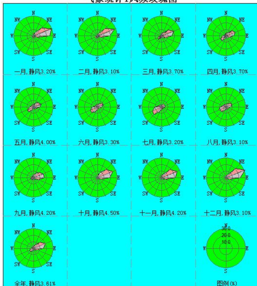
图 6.2-2 南雄气象站近 20 年(2005-2024)风向频率玫瑰图
