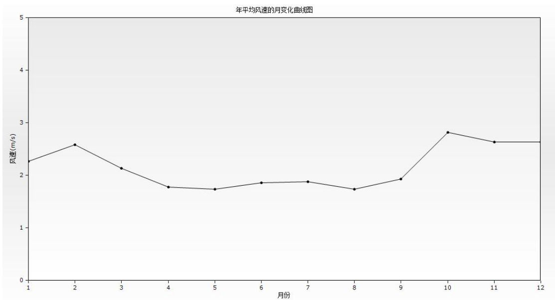
图 6.2-4 年平均风速的月变化图
