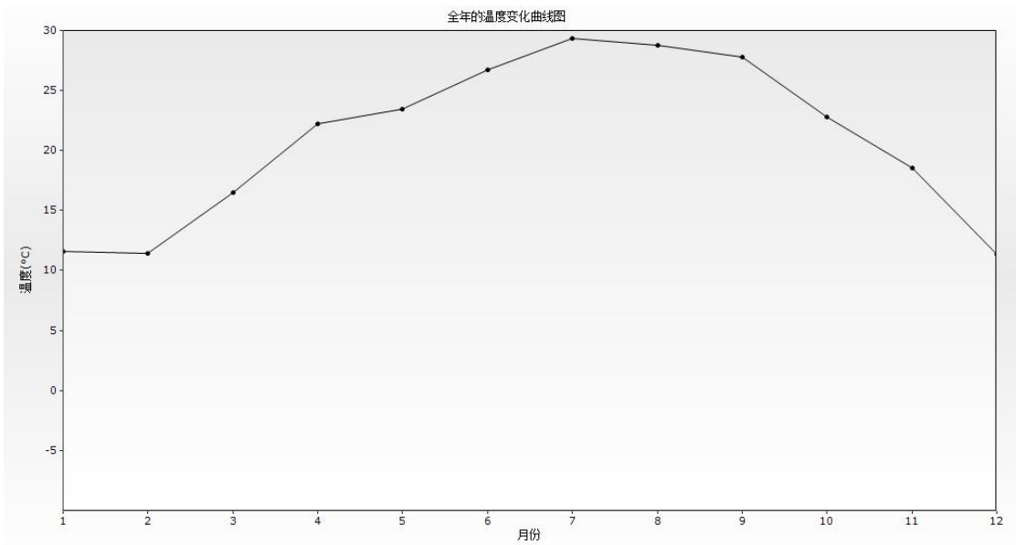
图 6.2-32024 年平均温度的月变化曲线图
