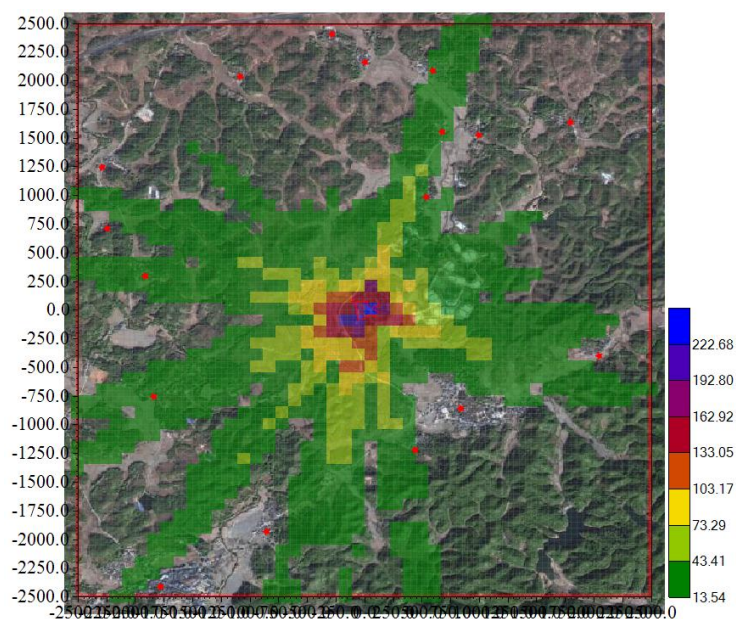
图 6.2-7 本项目 \text{NH}_3 最大小时浓度影响 ( \mu\text{g}/\text{m}^3 )
