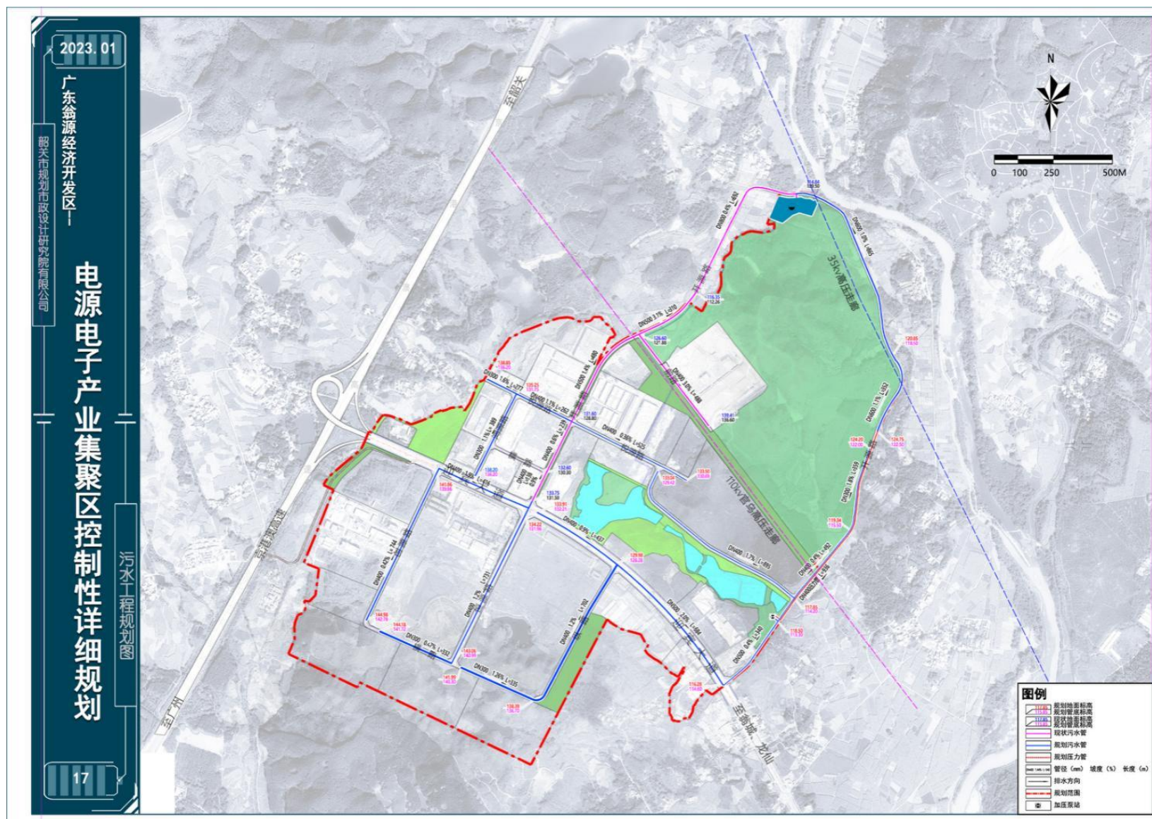
图 4.3.2-4 电源电子集聚区污水工程规划图
