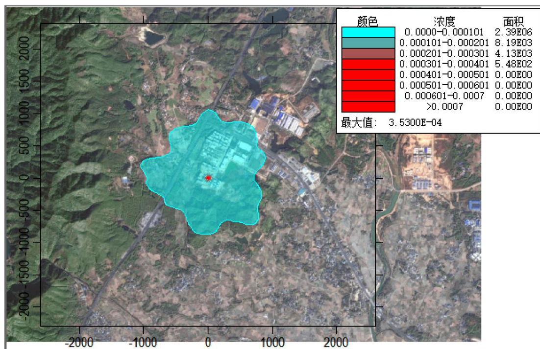
图 5.4.12-3 新增源 PM 2.5 日均值贡献浓度分布 (单位: mg/m 3 )
