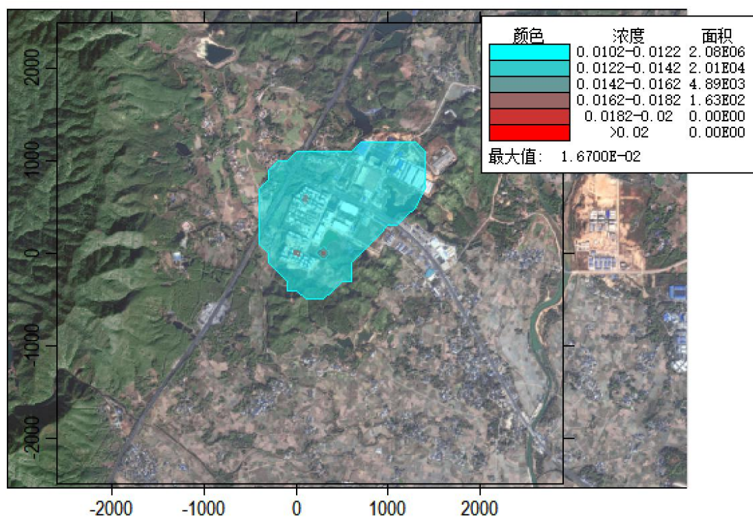
图 5.4.12-12 污染源叠加的 PM 2.5 年均值浓度分布
