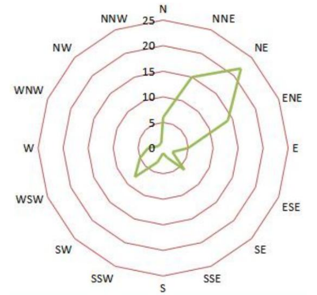
图 4.1-2 翁源气象站累年各季风向玫瑰图（统计年限：2004-2023 年）
