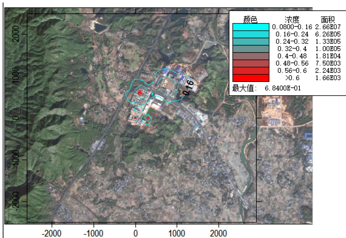
图 5.4.12-14 污染源叠加的非甲烷总烃 1 小时值浓度分布
