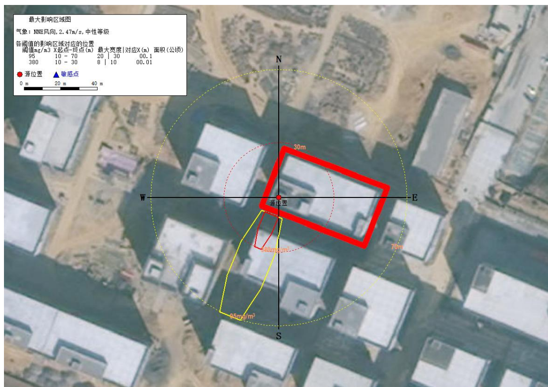
图 6.4-3 常见气象条件下 CO 浓度超过阈值范围的最大影响范围图
