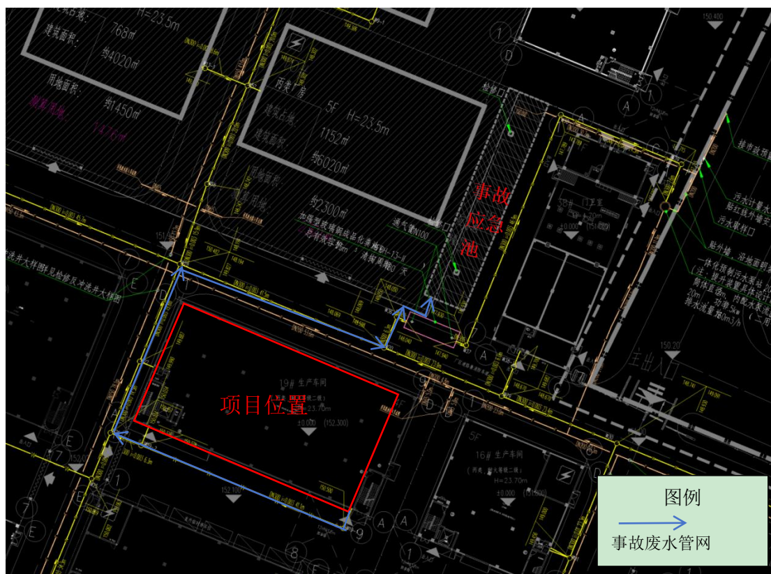
图 6.5-1 项目事故废水收集管网示意图
