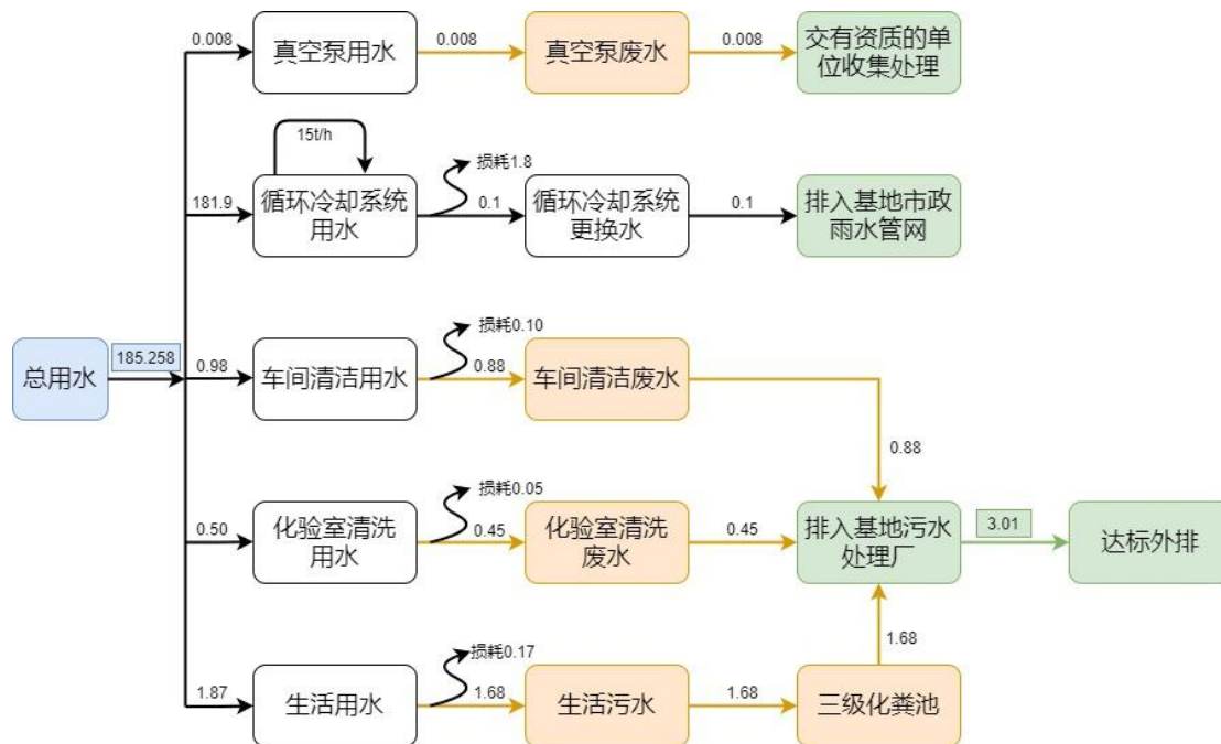
图 3.3.2-1 项目水平平衡图 (m³/d)
