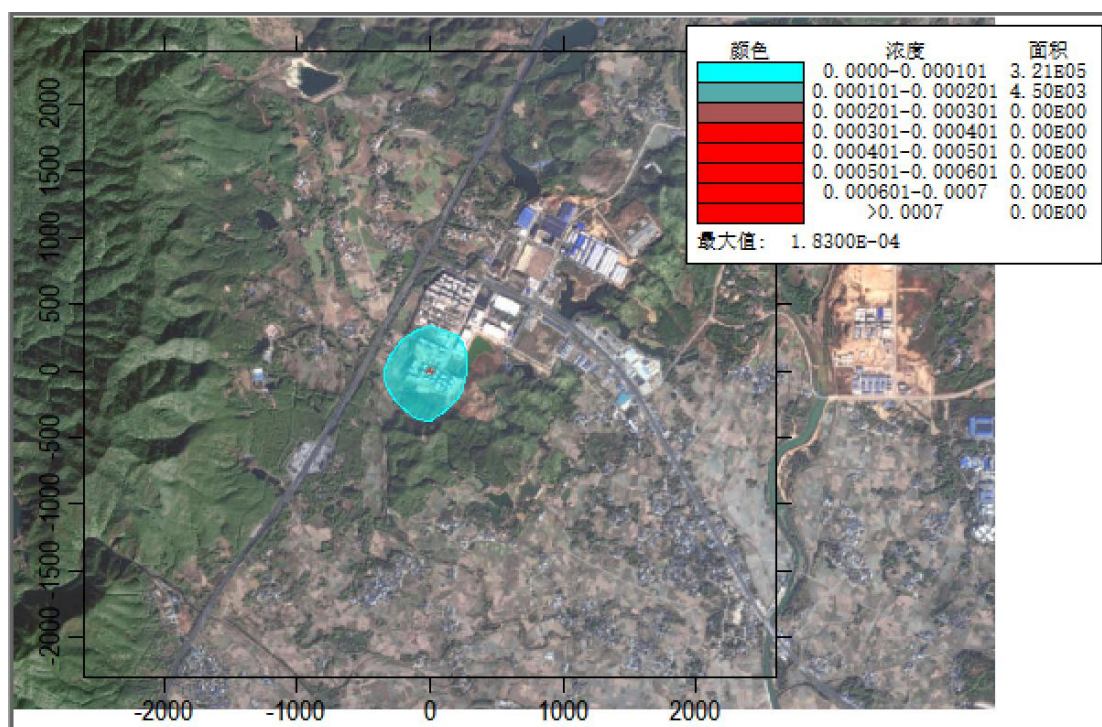
图 5.4.12-4 新增源 PM 2.5 年均值贡献浓度分布 (单位: mg/m 3 )
