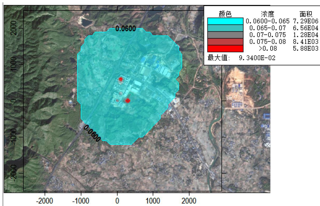
图 5.4.12-16 污染源叠加的 TSP 月均值浓度分布
