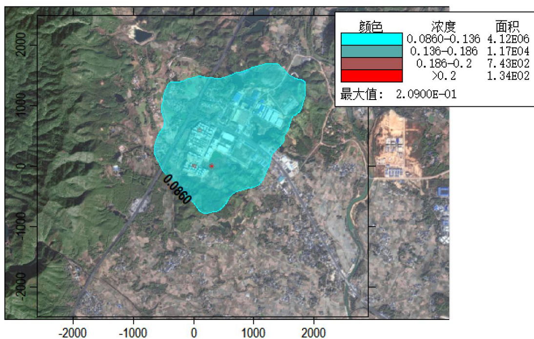
图 5.4.12-15 污染源叠加的 TSP 日均值浓度分布
