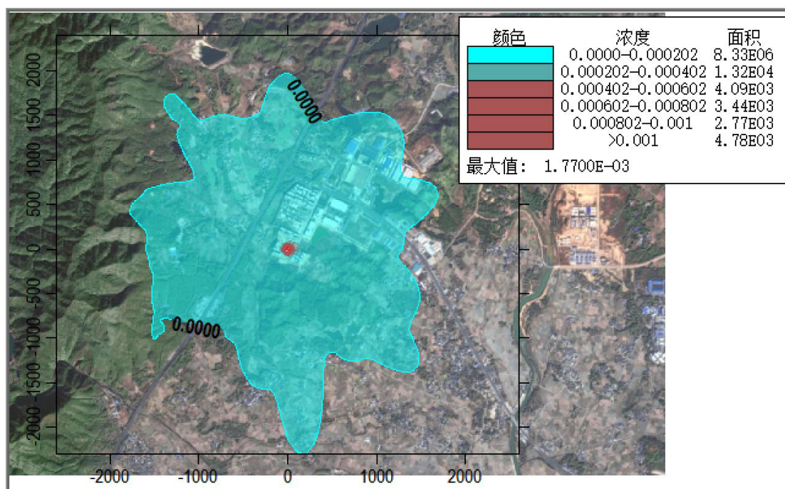
图 5.4.12-7 新增源 TSP 日均值贡献浓度分布 (单位: \text{mg}/\text{m}^3 )
