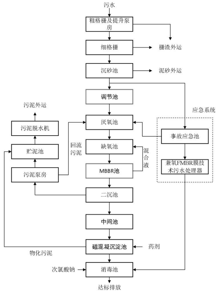
图 4-1 乌泥角污水处理厂处理工艺流程图
