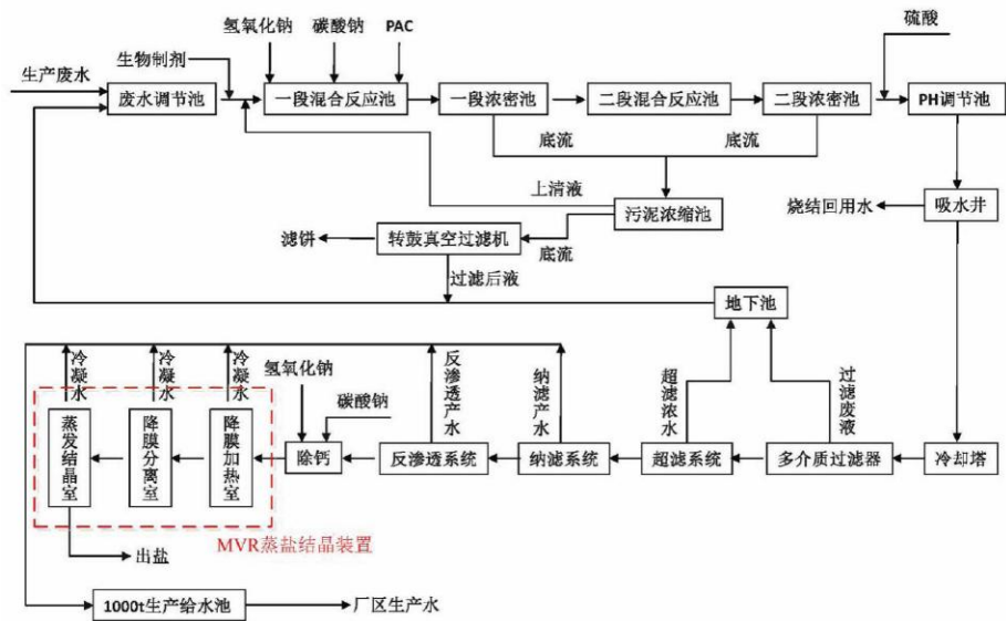
图4-1 现有的深度污水处理站废水处理工艺流程
