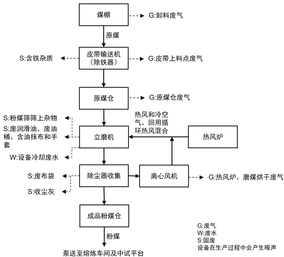
图 2-2 磨煤工艺流程及产污节点图
