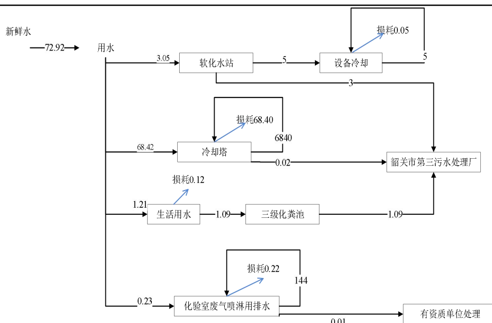
图 2-1 项目水平衡图 (t/d)
