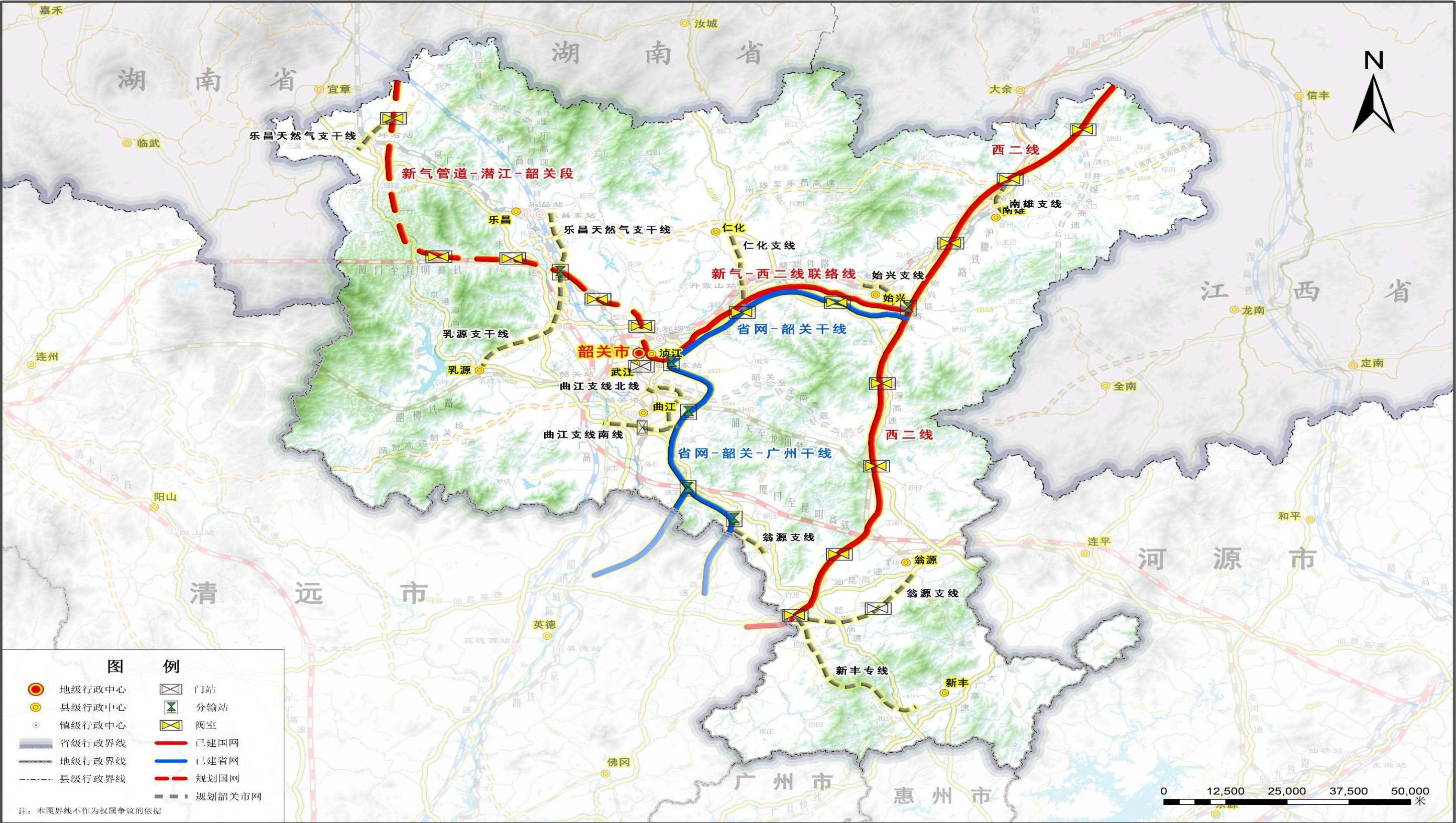
附图 10 韶关市油气管道布局示意图
