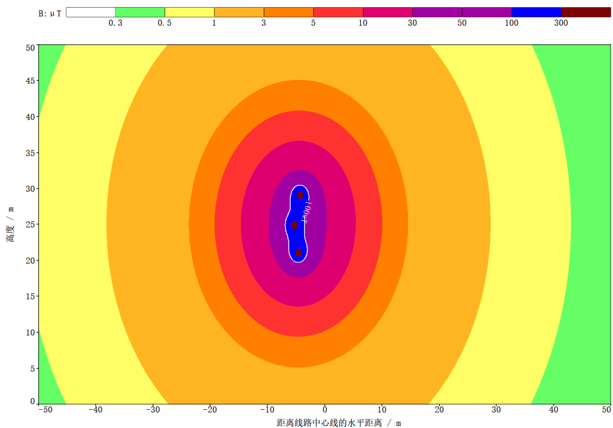
图 7 110kV 同塔双回挂单边线路工频磁感应强度空间分布图
