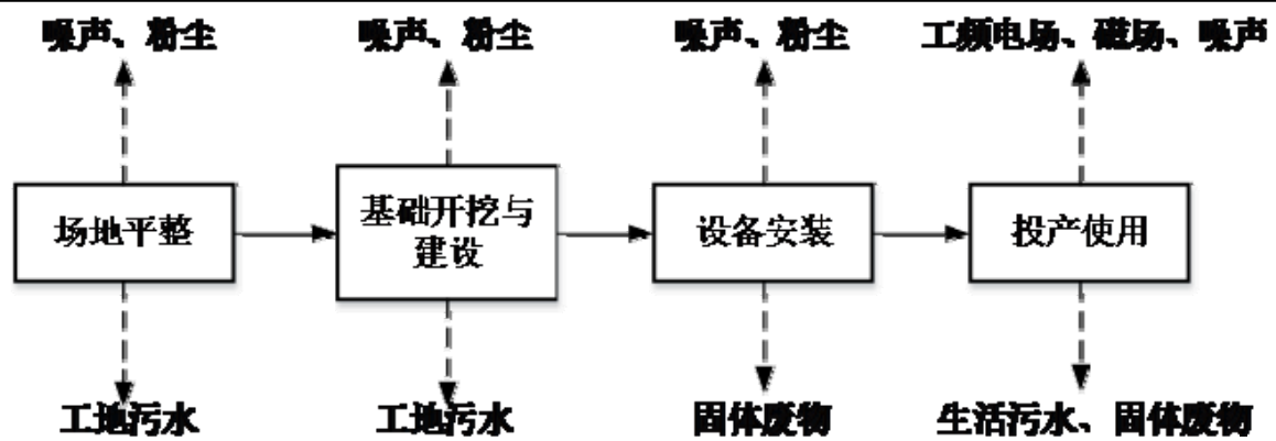
图 2.11-1 变电站工程工艺流程及产污环节
