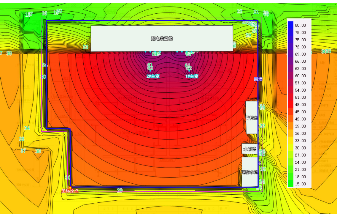
图 4.9-1 噪声贡献值等值线图 表 4.9-3 本工程厂界噪声贡献值计算结果
