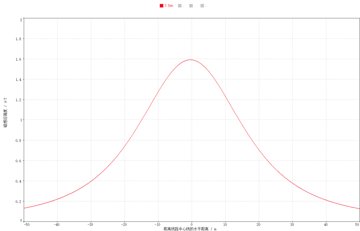
图 14 110kV 同塔双回架空线路工同塔双回挂单边线路结果衰减趋势图
