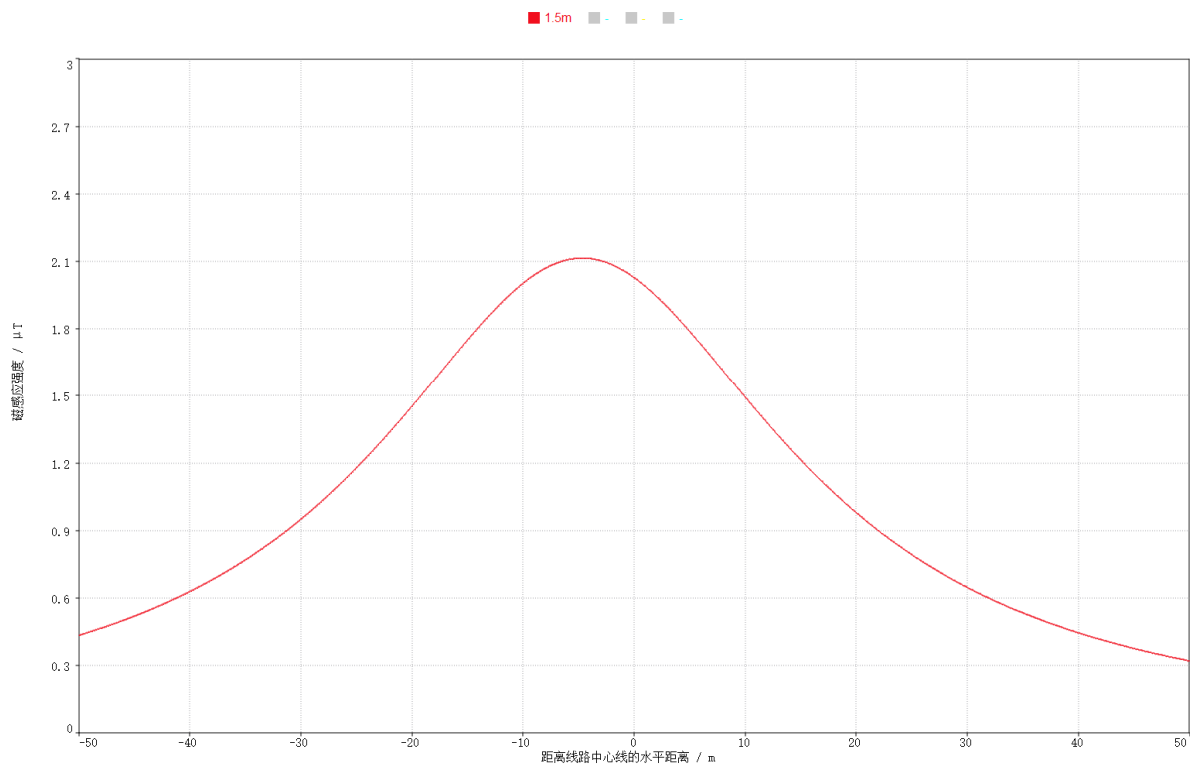
图 13 110kV 同塔双回挂单边线路工频磁场预测结果衰减趋势图
