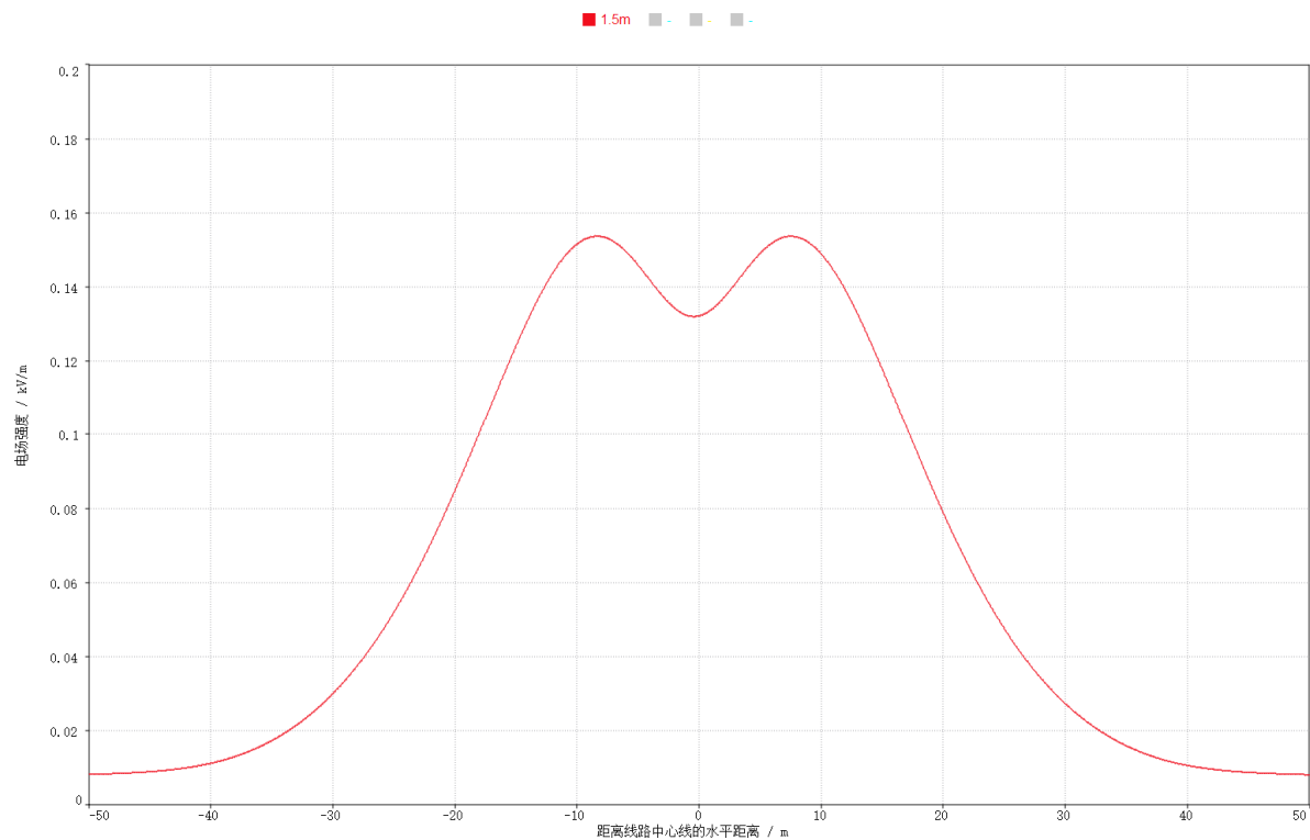
图 11 110kV 同塔双回架空线路工频电场预测结果衰减趋图
