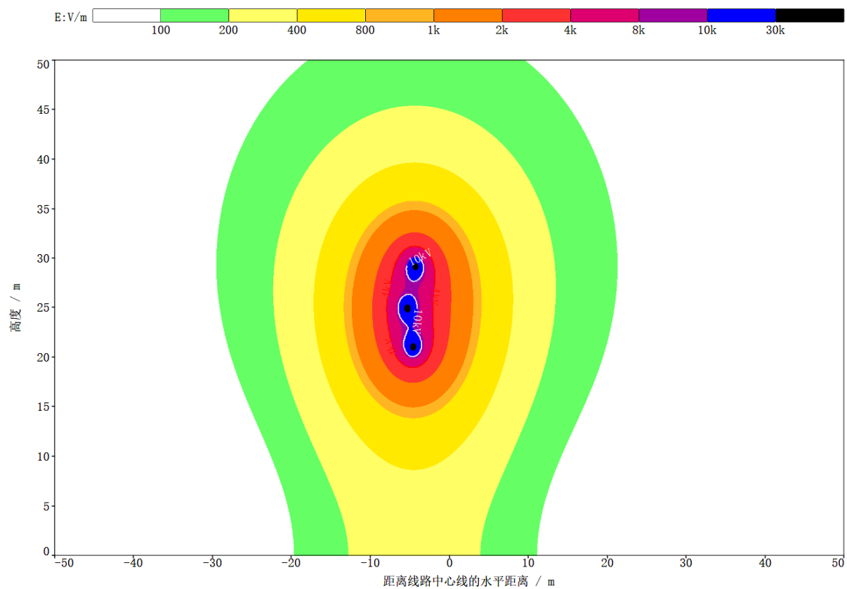
图 4 110kV 同塔双回挂单边线路工频电场强度空间分布图
