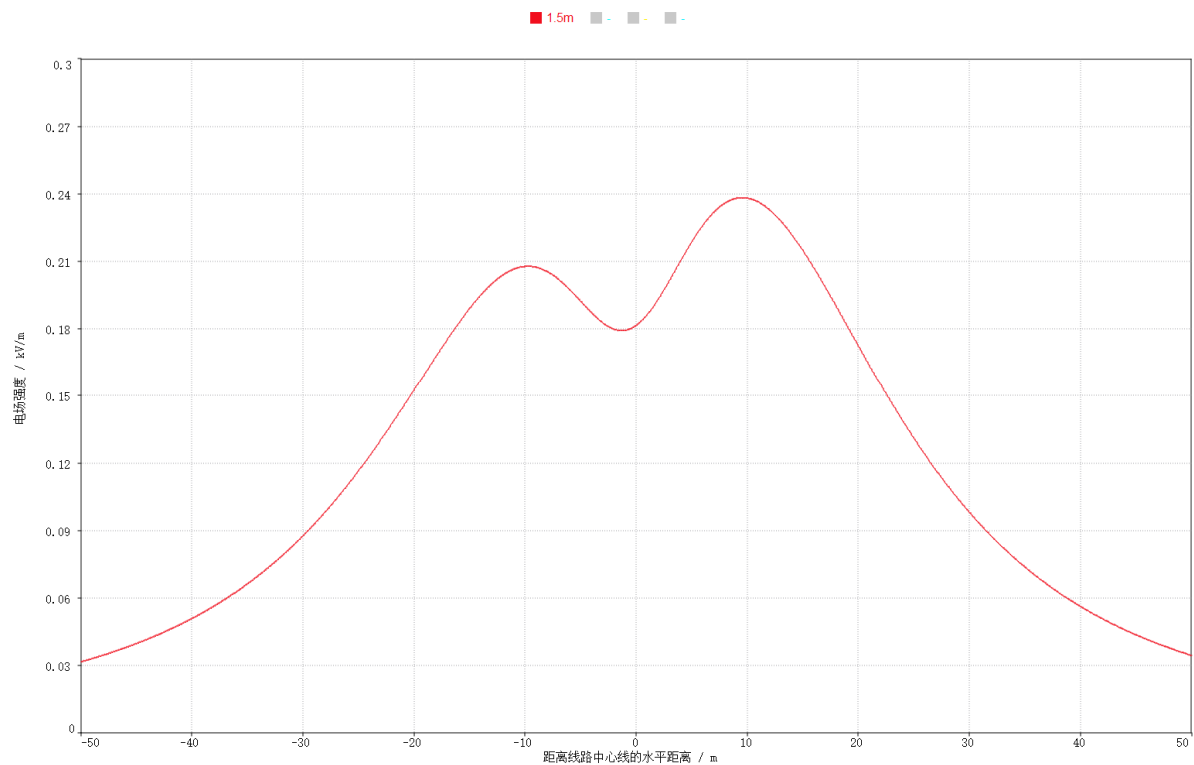
图 9 110kV 单回架空线路工频电场预测结果衰减趋势图
