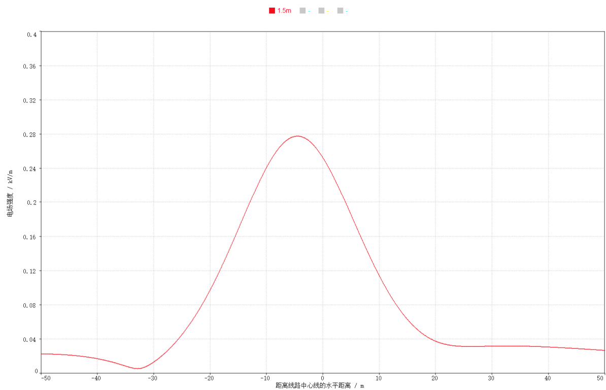
图 10 110kV 同塔双回挂单边线路工频电场预测结果衰减趋势图
