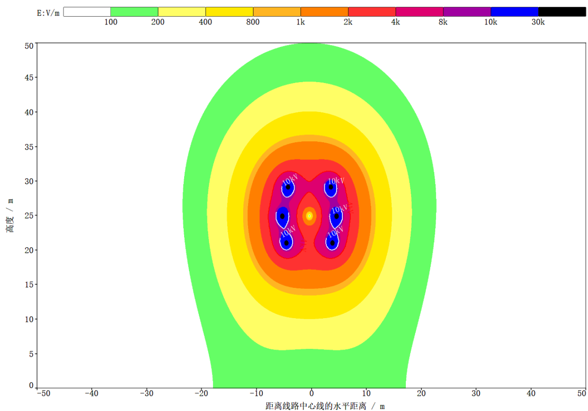
图 5 110kV 同塔双回架空线路工频电场强度空间分布图
