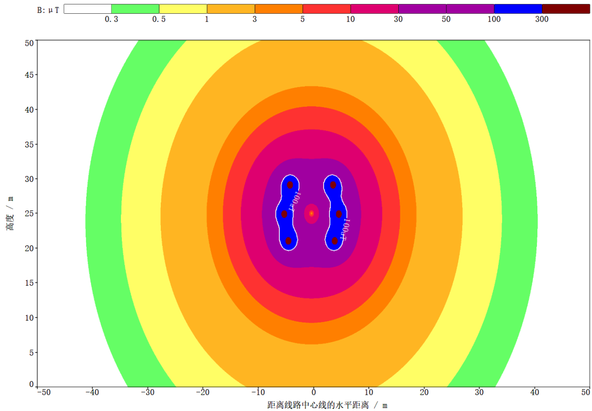
图 8 110kV 同塔双回架空线路工频磁感应强度空间分布图
