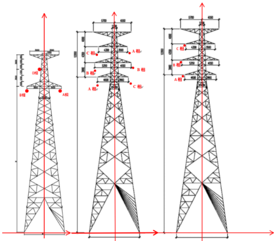
图 2 拟建 110kV 架空线路工频电场、工频磁场预测建立的直角坐标系
