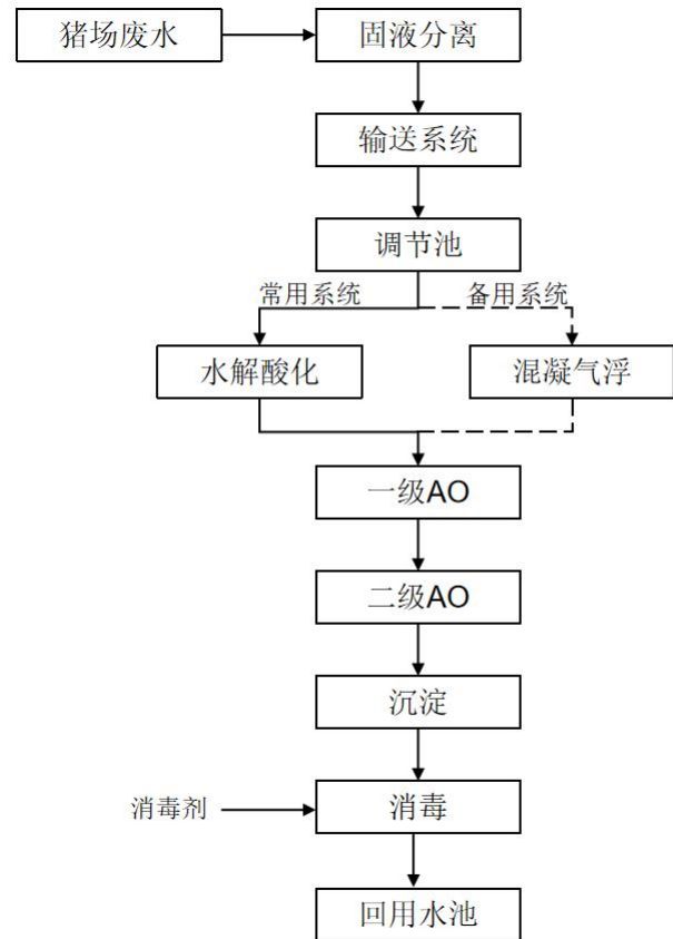
图 7.2-1 项目污水处理站处理工艺流程图
