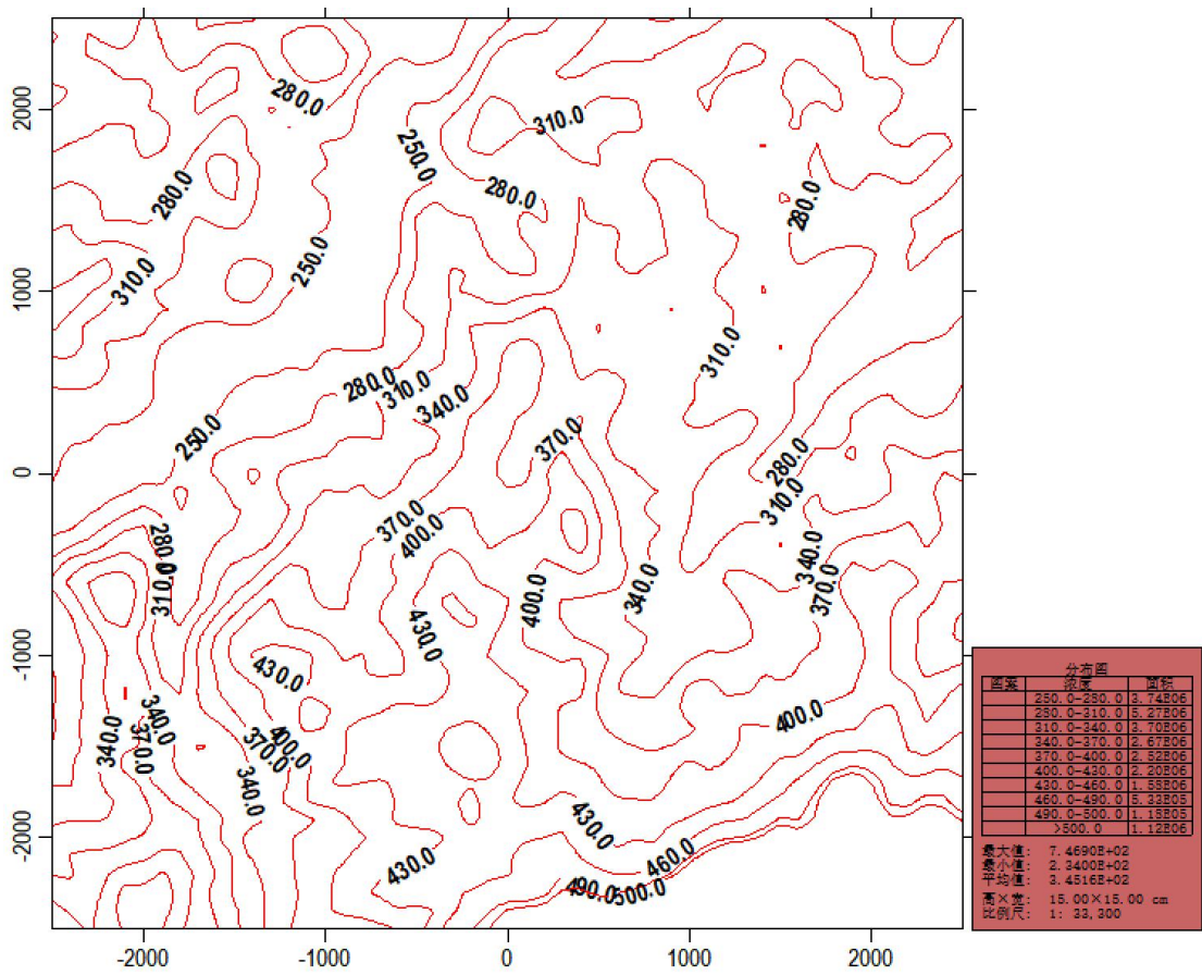
图 5.2-6 项目预测范围内地面高程图
