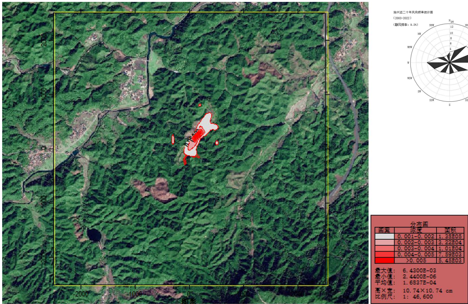
图 5.2-8 正常排放 H 2 S 小时平均浓度各点贡献值分布图 (mg/m 3 )
