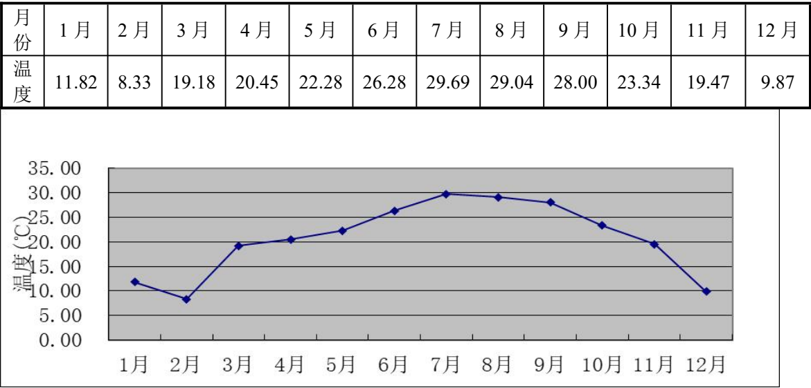
图5.2-2 始兴气象站2022年平均温度的月变化图
