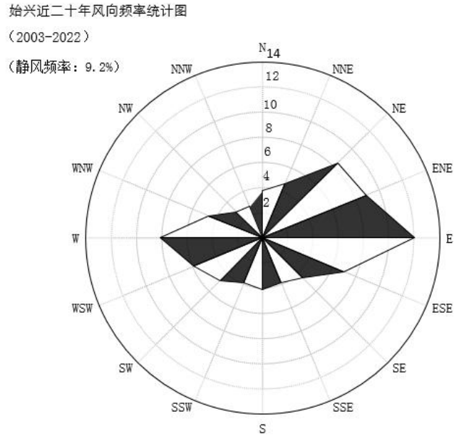
图5.2-1 始兴县气象站风向玫瑰图 (统计年限2003年~2022年)
