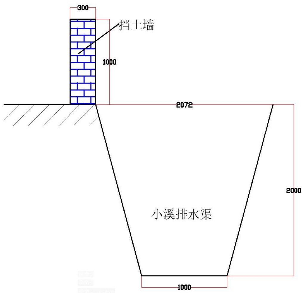
图 3.1-2 无名小溪改造方案示意图
