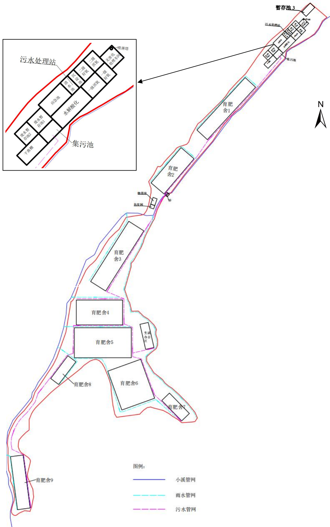
图 3.1-4 项目平面布置及雨污管网分布图
