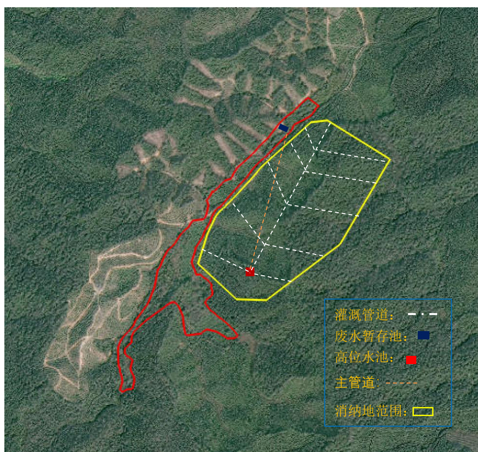
图 7.2-2 项目灌溉管网分布示意图
