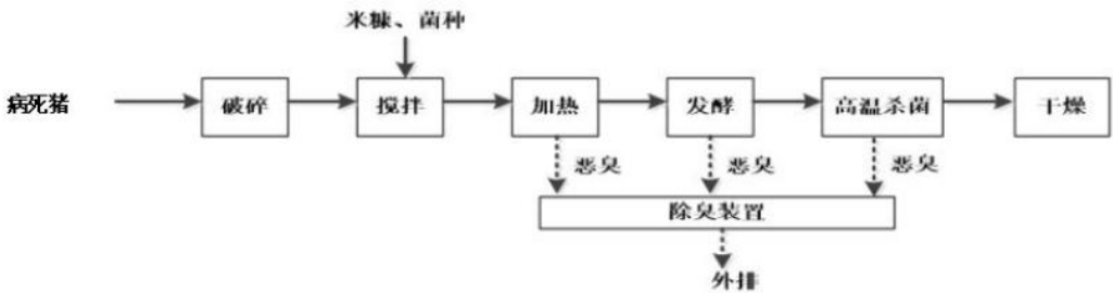
图 3.2-3 项目无害化降解处理机工艺流程图
