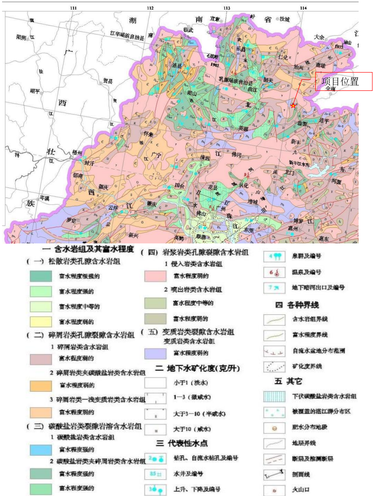
图 5.2-7 项目所在区域水文地质状况图
