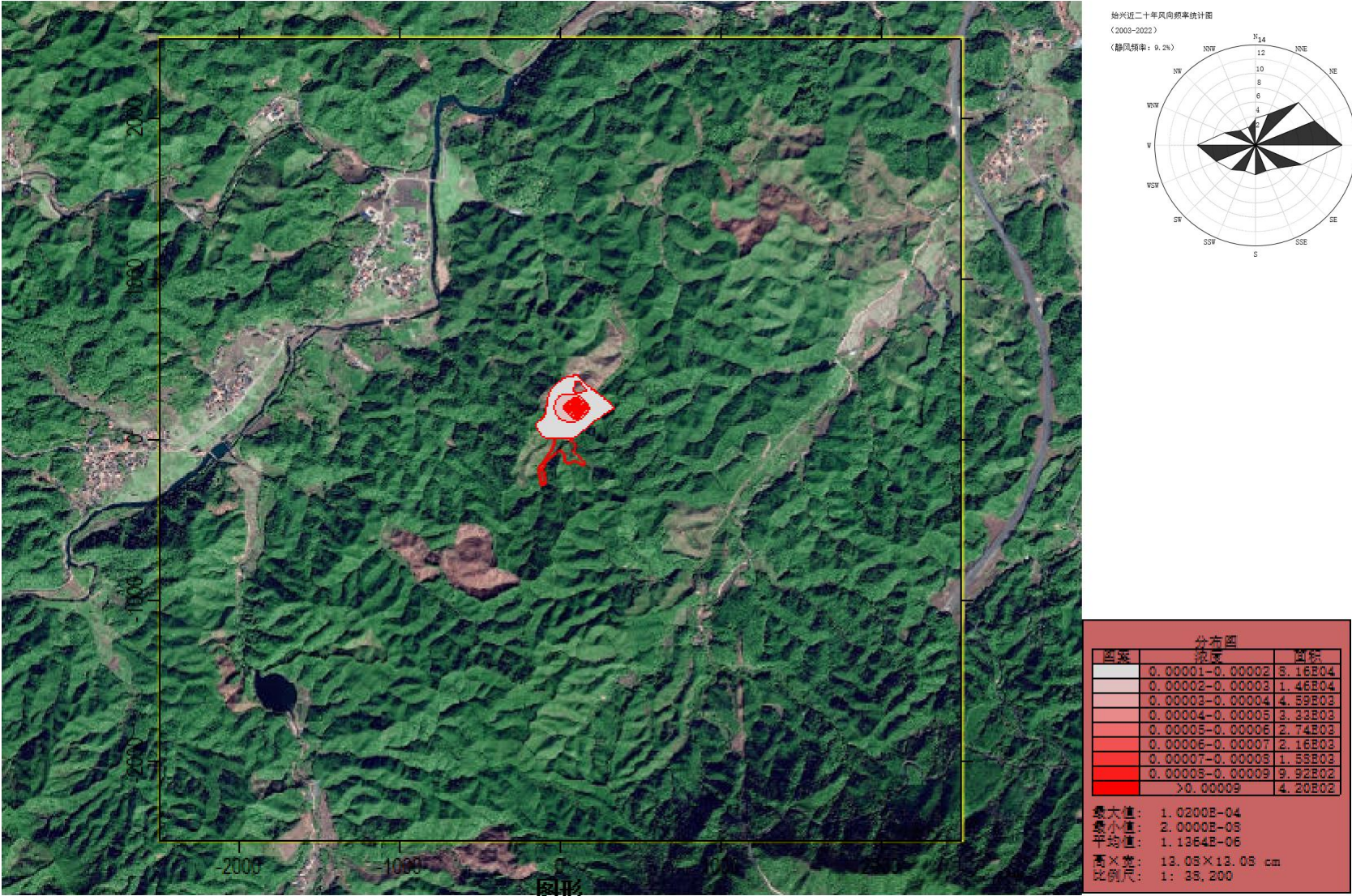
图 5.2-10 正常排放 SO 2 日均浓度各点贡献值分布图 (mg/m 3 )
