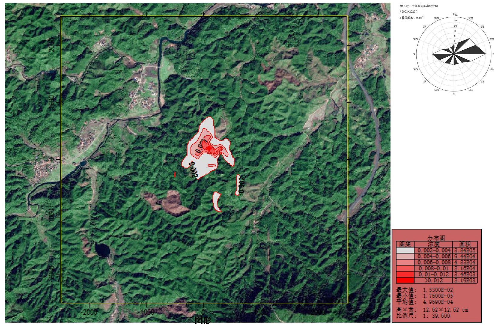
图 5.2-12 正常排放 NO 2 小时平均浓度各点贡献值分布图 (mg/m 3 )
