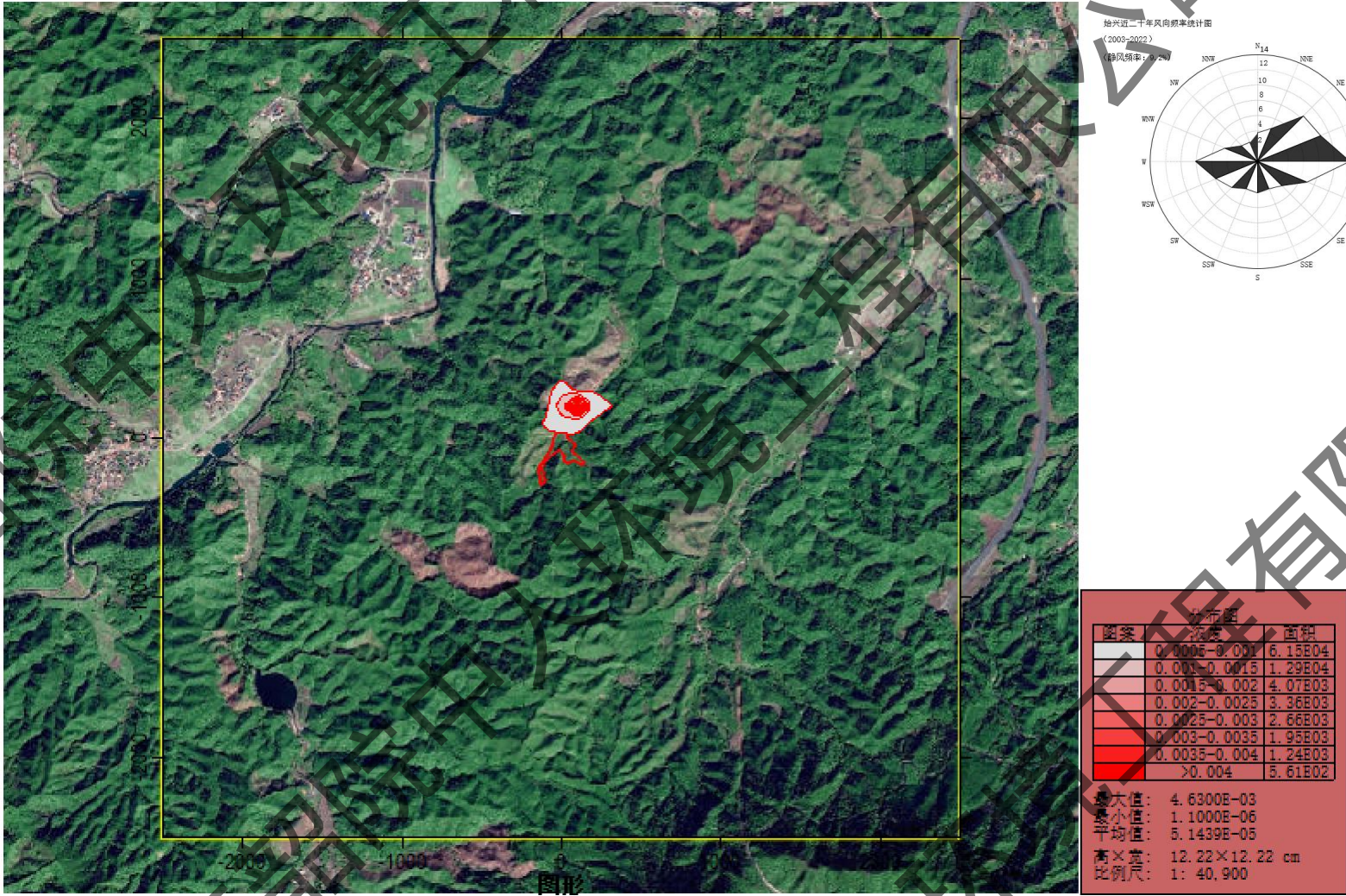
图 5.2-13 正常排放 NO 2 日均浓度各点贡献值分布图 (mg/m 3 )
