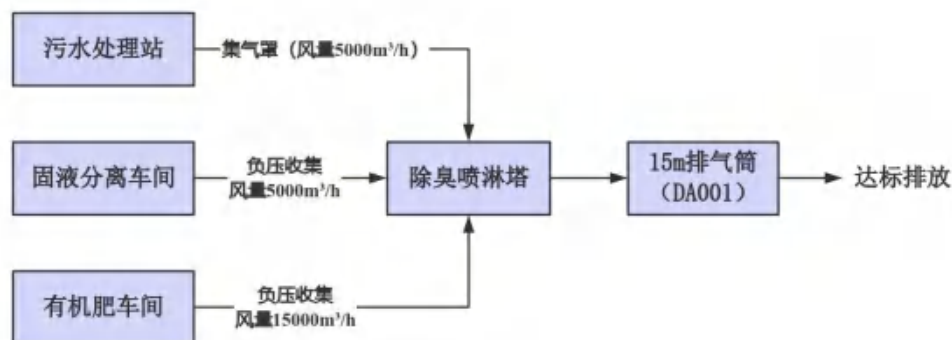
图3.4.2-1 污水站、固液分离车间及有机肥车间恶臭气体收集及处置措施流程图
