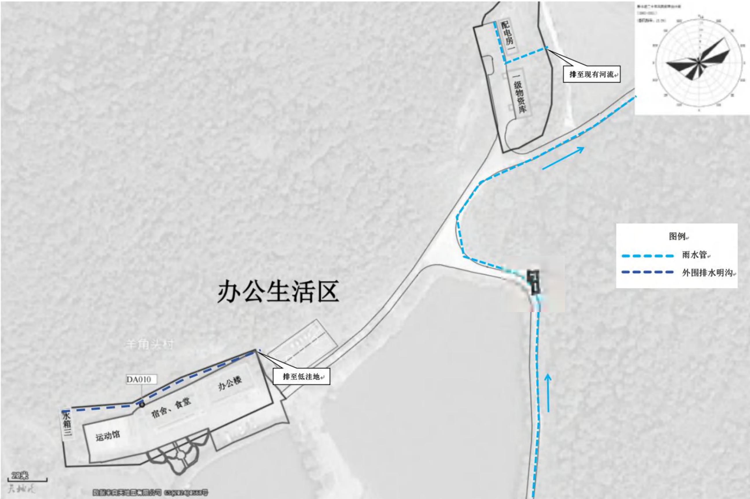
图3.2.2-13 雨水管网布置图
