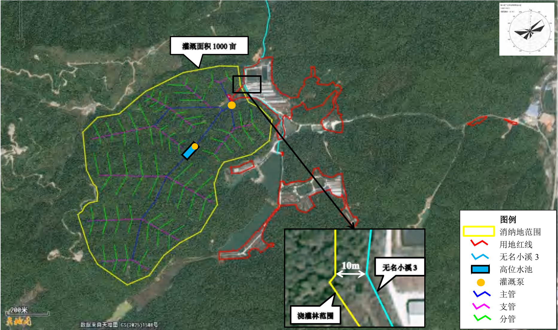
图 7.2.2-6 灌溉林地管网布设图
