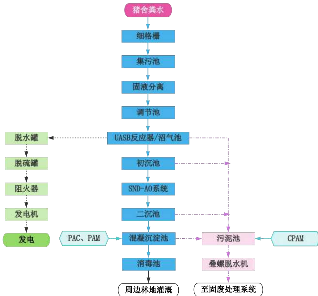
图3.3.2-4 污水处理工艺流程图
