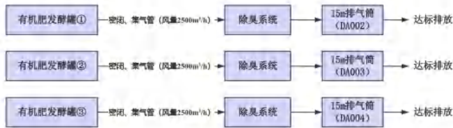
图3.4.2-2 有机肥发酵恶臭气体收集及处置措施流程图
