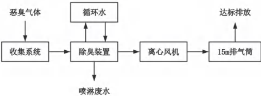
图7.2.1-1 除臭系统工艺流程 表7.2.1-1 除臭系统清单一览表
