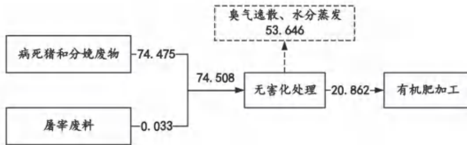
图3.2.8-7 改扩建后项目无害化处理物料平衡图（单位t/a）
