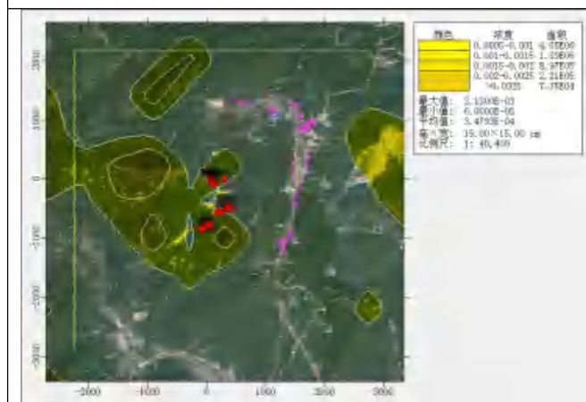
SO 2 1 小时平均浓度预测值分布图
