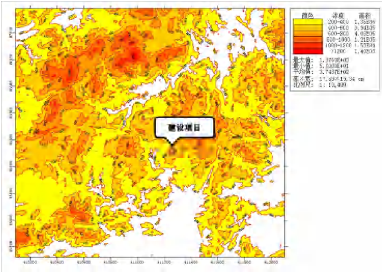
图 5.2.1-19 项目周边地形高程分布图
