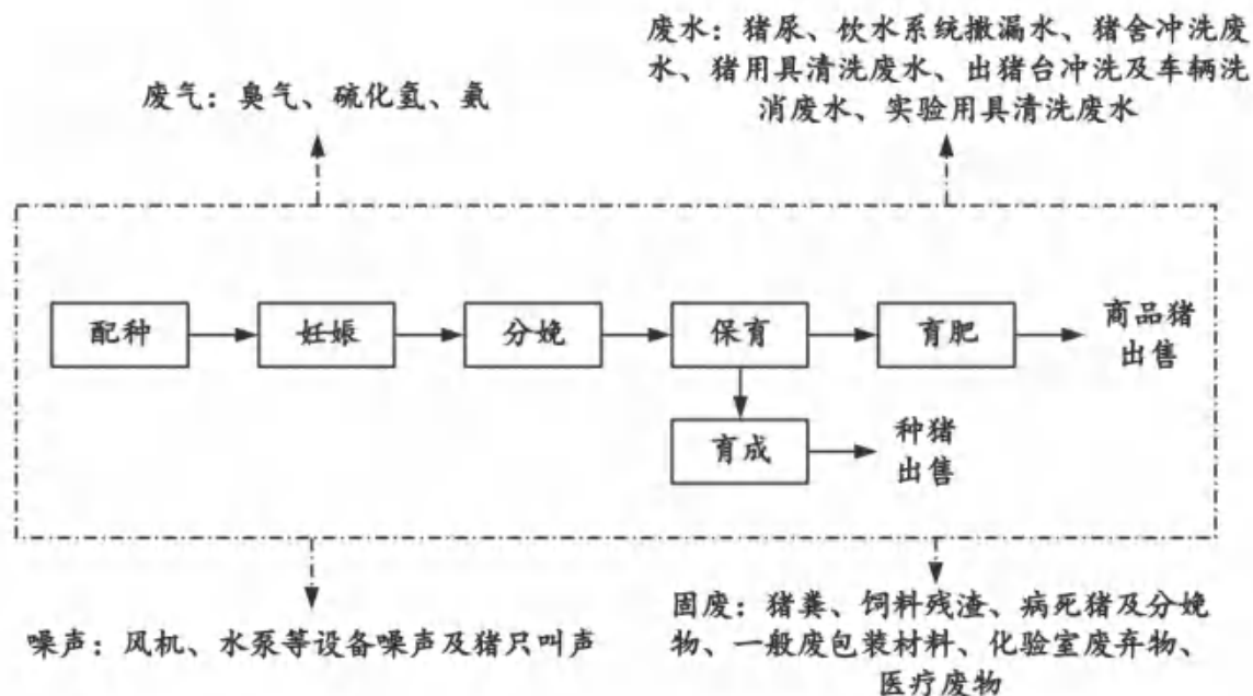
图3.3.2-1 养殖工艺流程图
