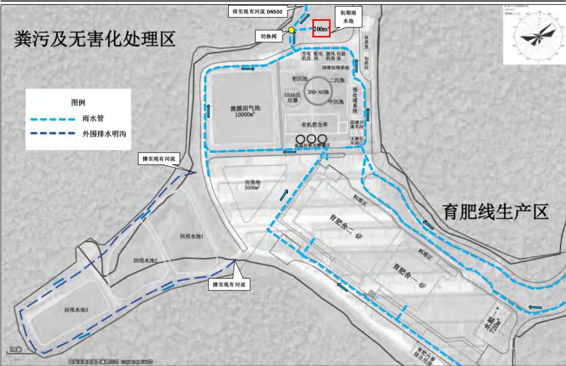
图7.2.2-5 粪污处理区雨水管网图
