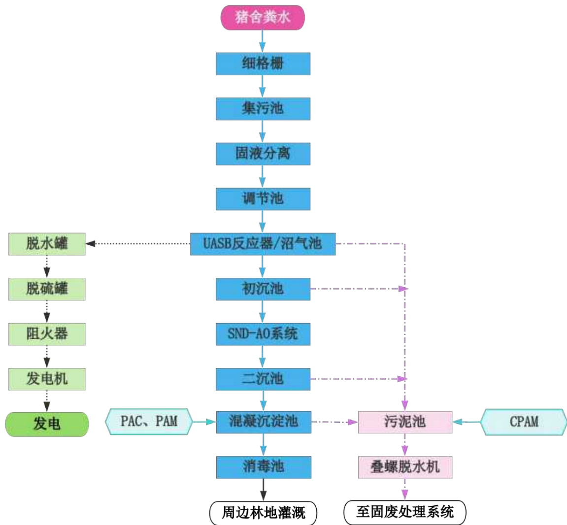
图7.2.2-1 污水处理工艺流程图1
