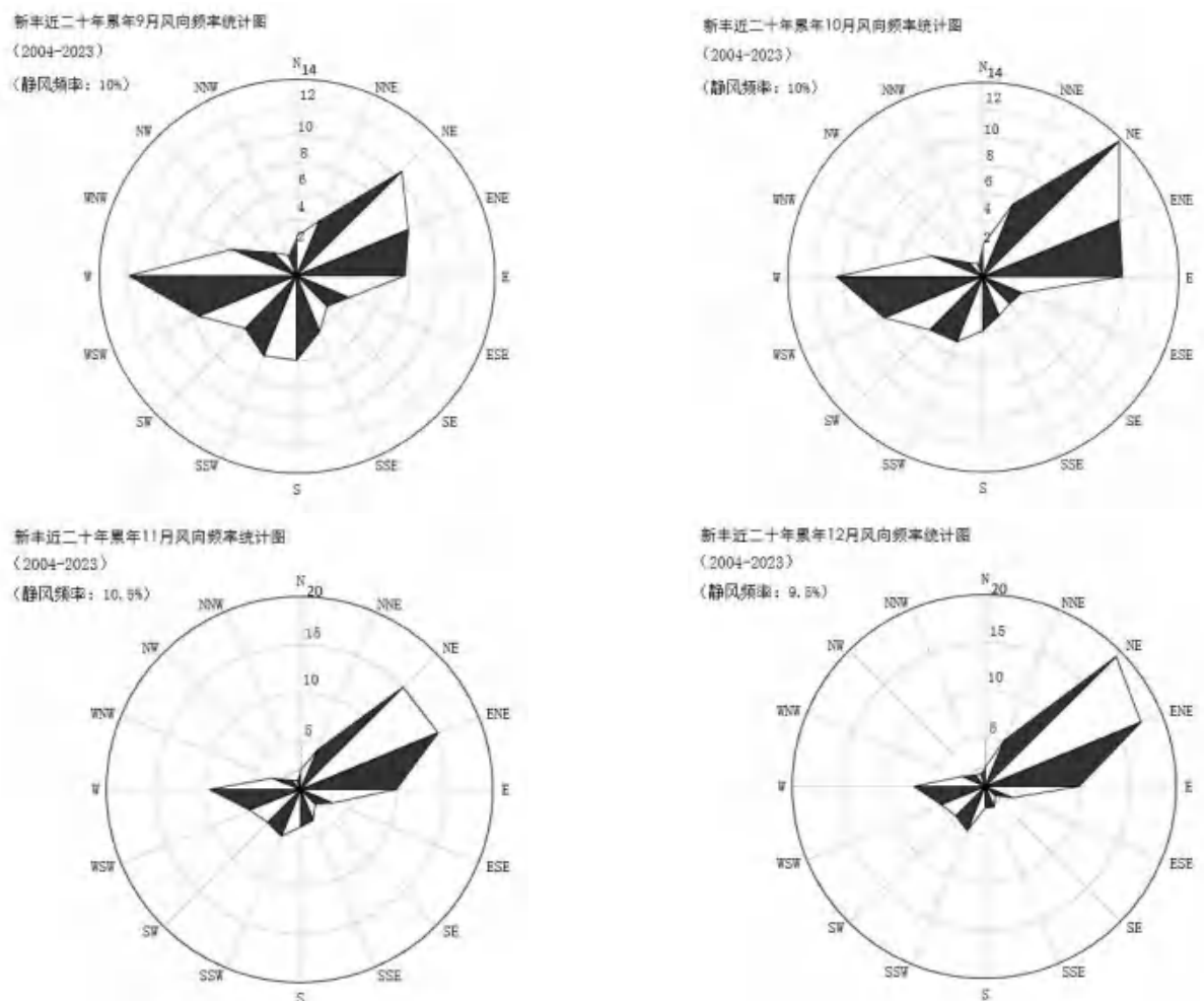
图5.2.1-2 新丰月风向玫瑰图
