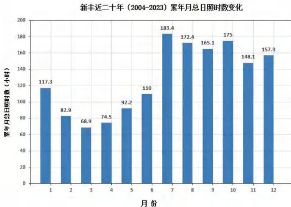
图5.2.1-8 新丰月日照时数（单位：小时）
