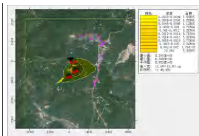
NMHC 1 小时平均浓度预测值分布图
