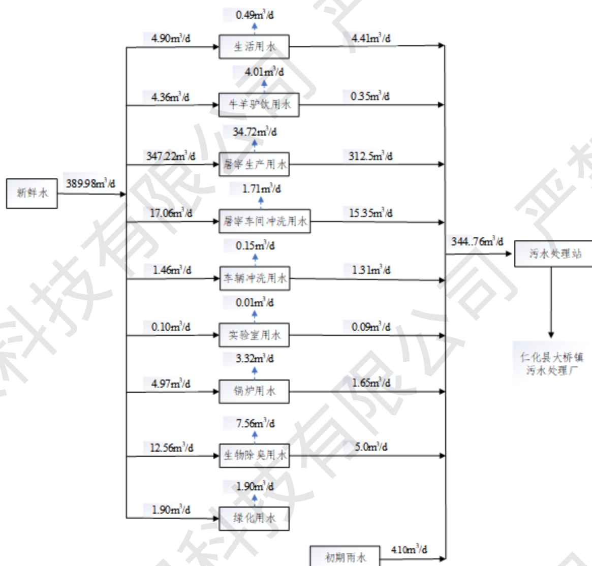
图 3-4 项目水平衡图 (单位: \text{m}^3/\text{d} )
