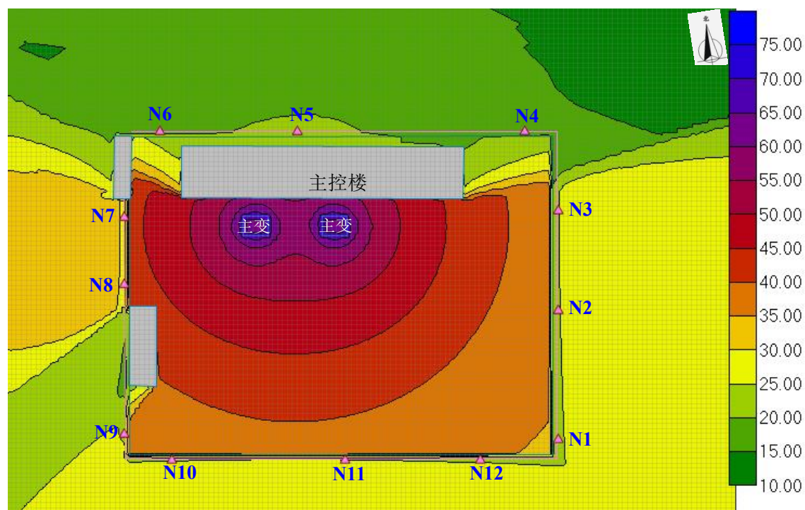
图 4.4-2 噪声贡献值等值线图
