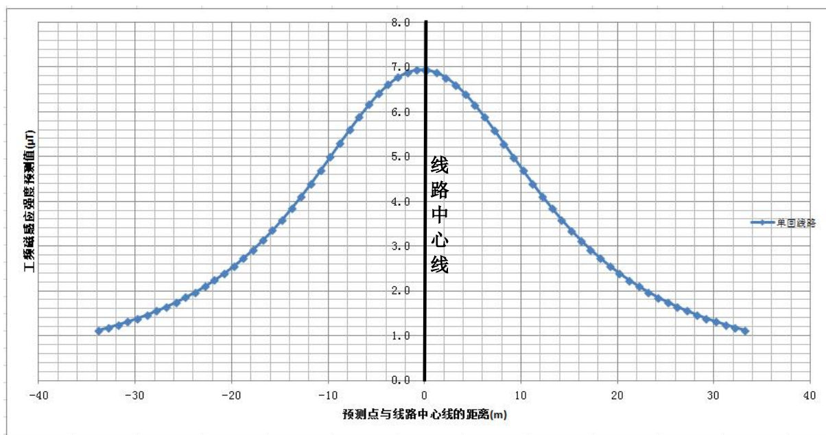
图 4 110kV 单回架空线路工频磁场预测结果衰减趋势图
