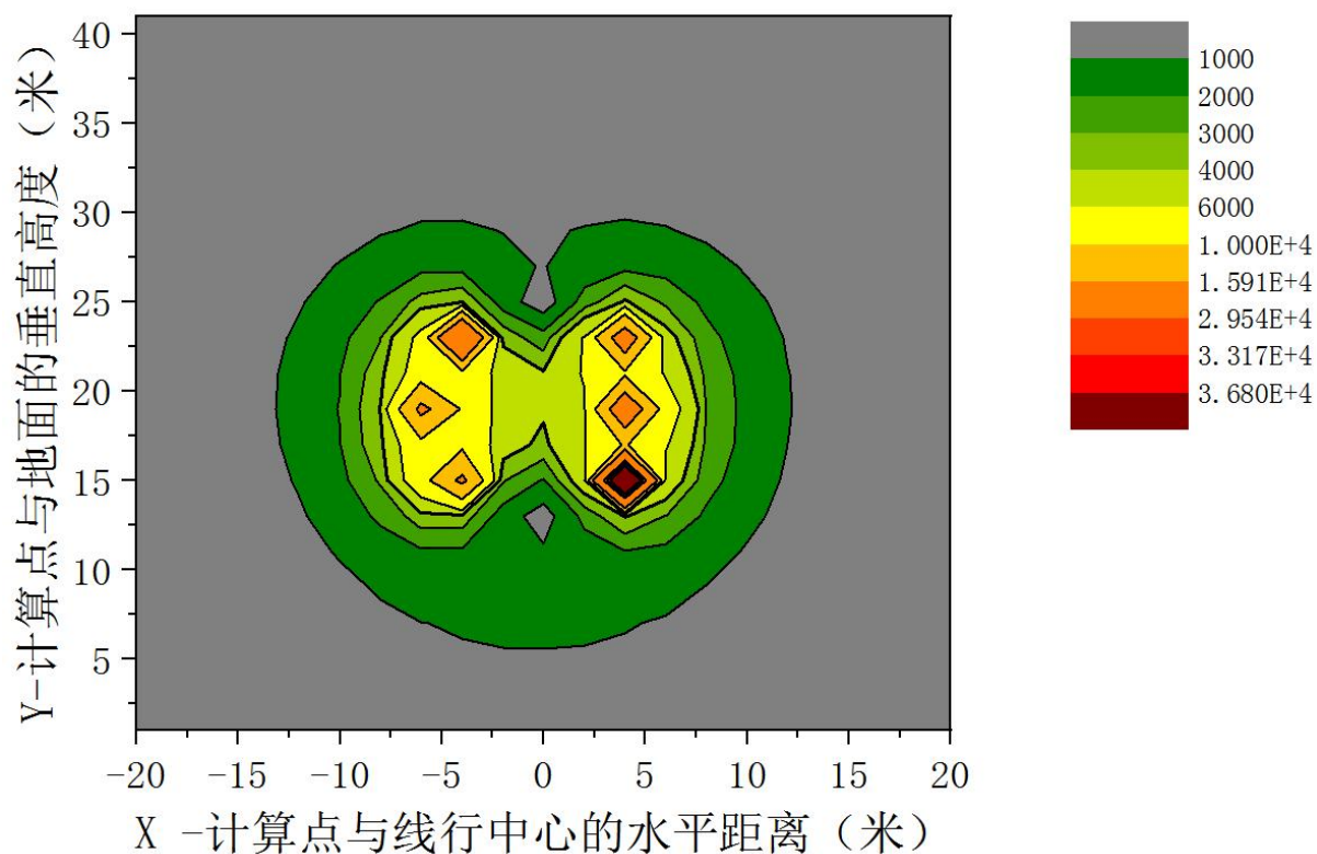
图 9 110kV 同塔双回架空输电线路工频电场强度空间分布（电场单位为 V/m）
