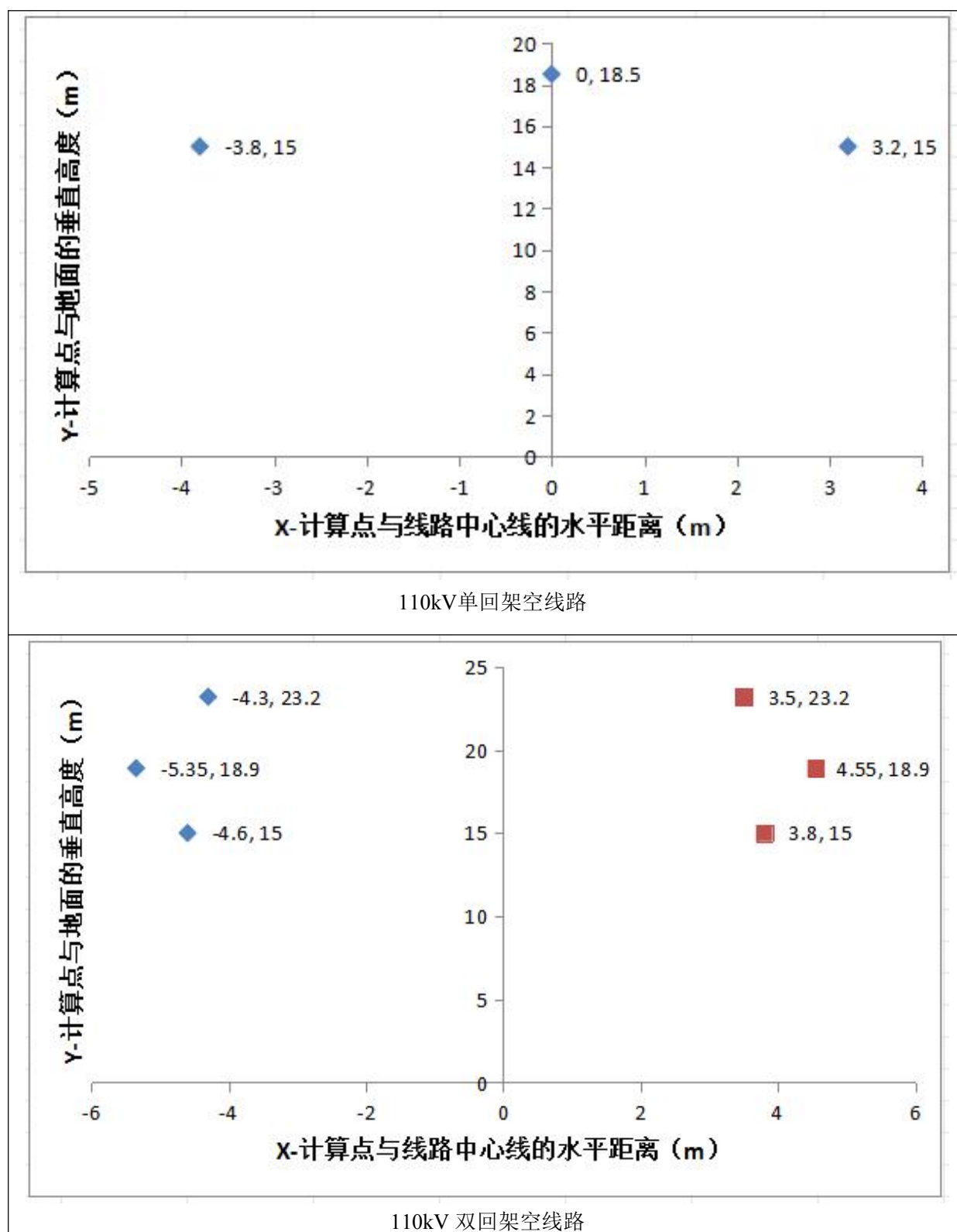
图 2 工频电磁场预测建立的直角坐标系
