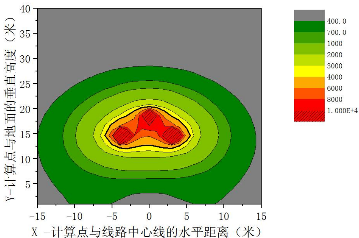
图 5 110kV 单回架空输电线路工频电场强度空间分布（电场单位为 V/m）
