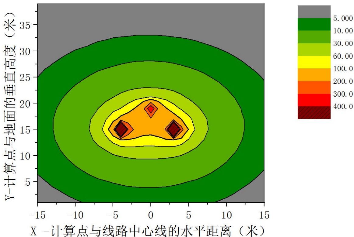
图 6 110kV 单回架空输电线路工频磁场强度空间分布图（磁场单位为 \mu\text{T} ）
