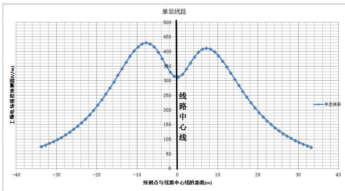
图 3 110kV 单回架空线路工频电场预测结果衰减趋势图
