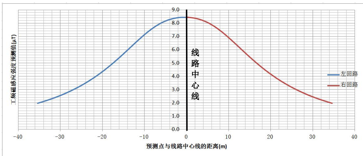
图 8 110kV 同塔双回架空线路工频磁场预测结果衰减趋势图
