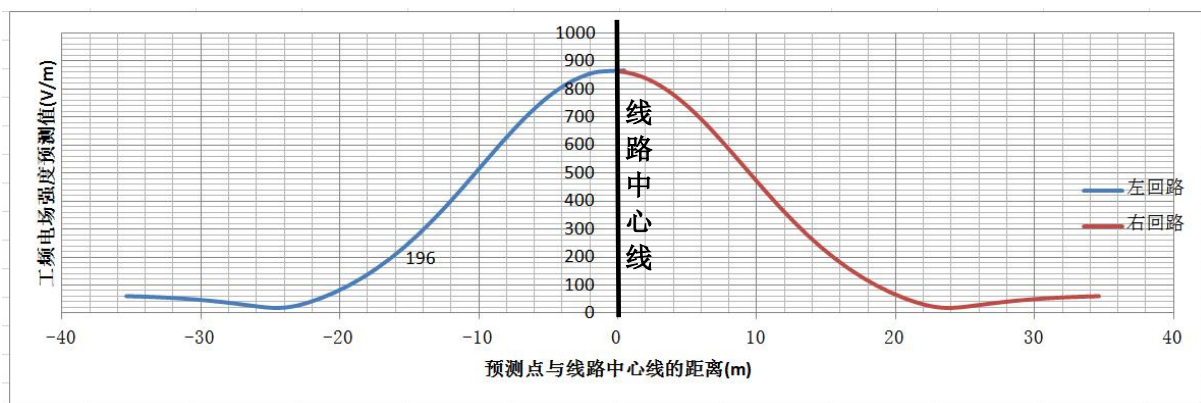
图 7 110kV 同塔双回架空线路工频电场预测结果衰减趋势图
