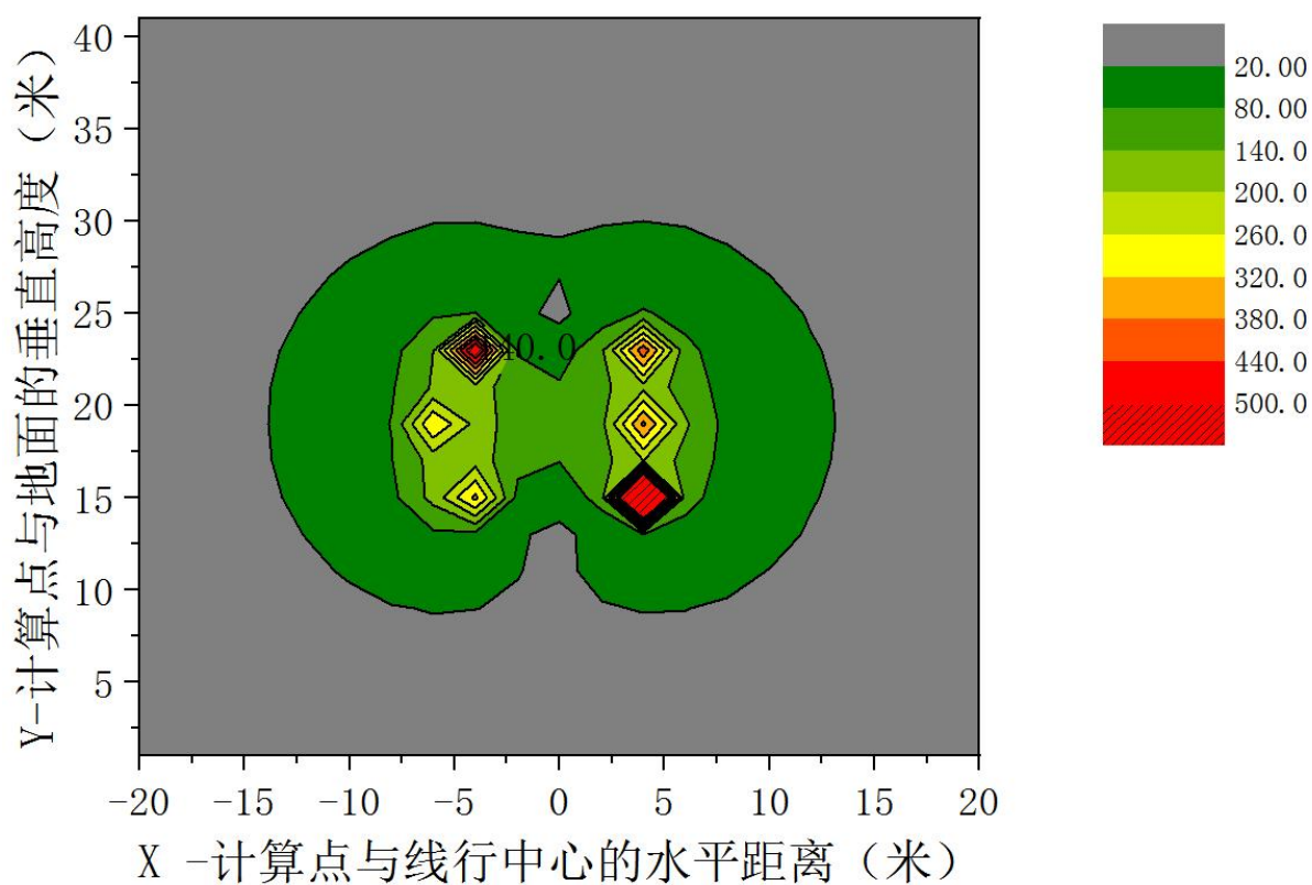
图 10 110kV 同塔双架空输电线路工频磁场强度空间分布图（磁场单位为 \mu\text{T} ）
