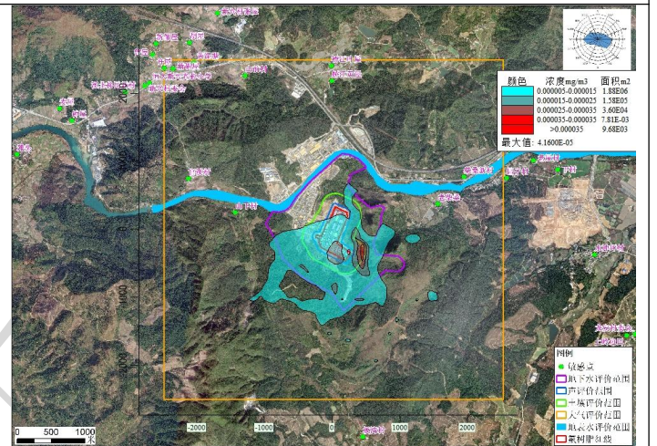
氟化氢日均浓度贡献值分布图
