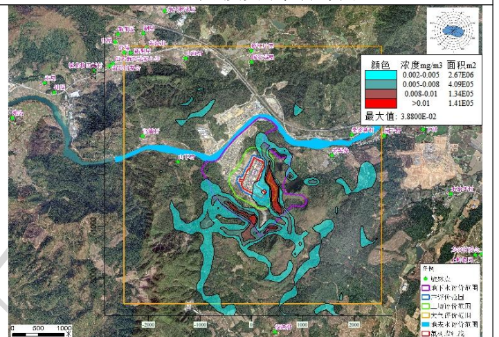
NO 2 小时浓度贡献值分布图
