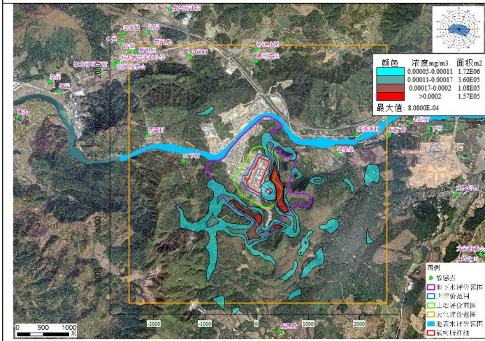
氟化氢小时浓度贡献值分布图
