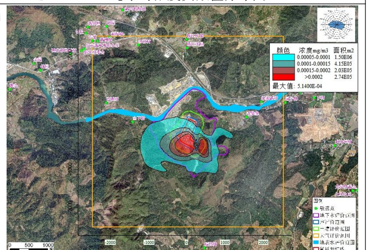
NO 2 年均浓度贡献值分布图
