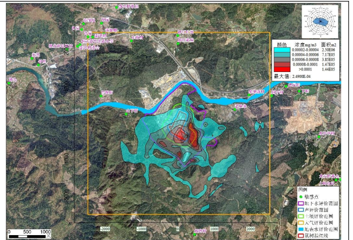
氯化氢日均浓度贡献值分布图
