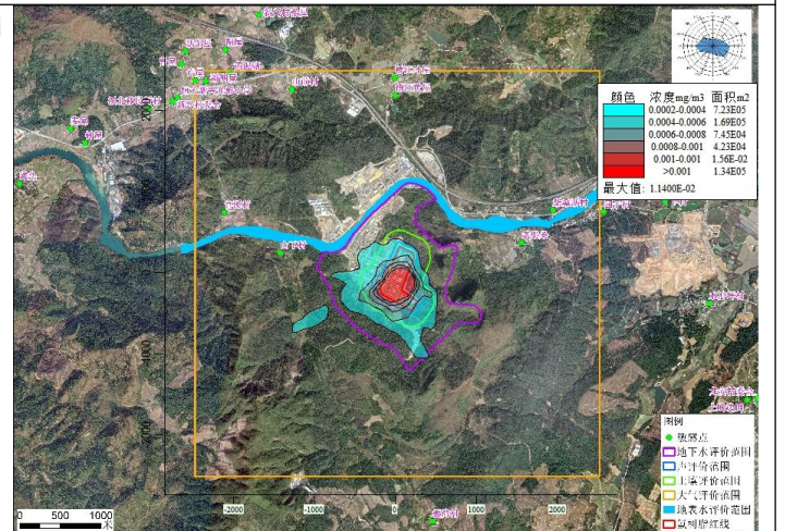
TVOC 8 小时浓度贡献值分布图
