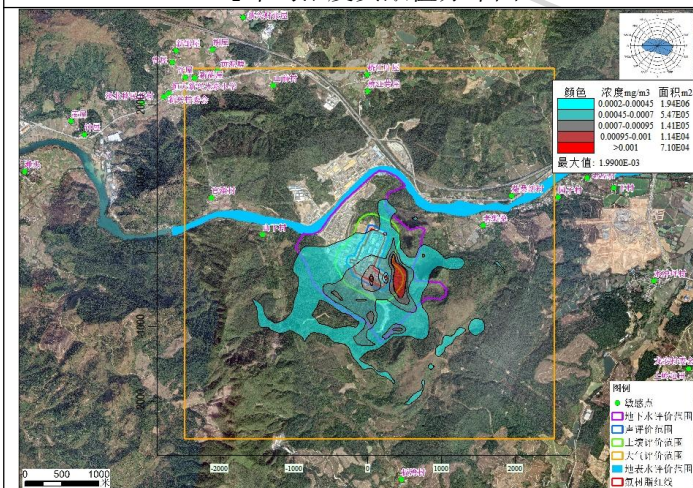
NO 2 日均浓度贡献值分布图
