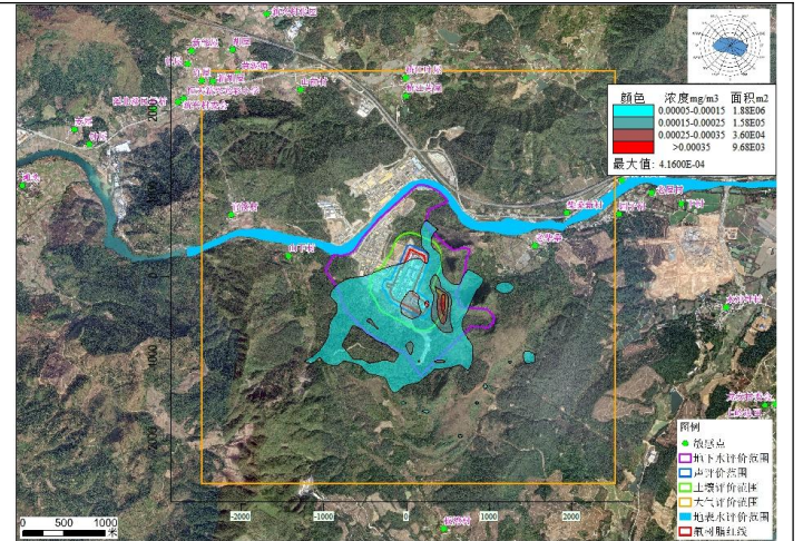
SO 2 日均浓度贡献值分布图
