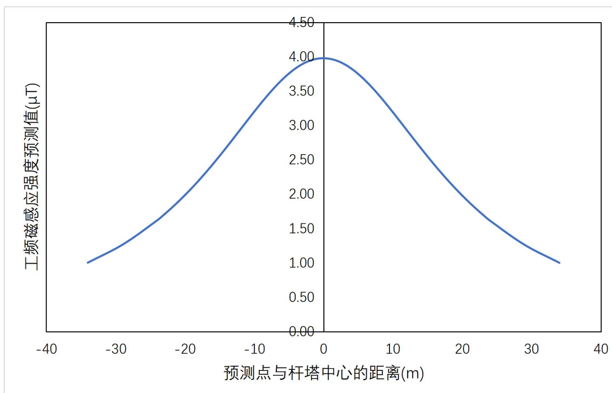
图 8 新建 110kV 单回架空线路离地 1.5m 处工频磁场预测结果衰减趋势图
