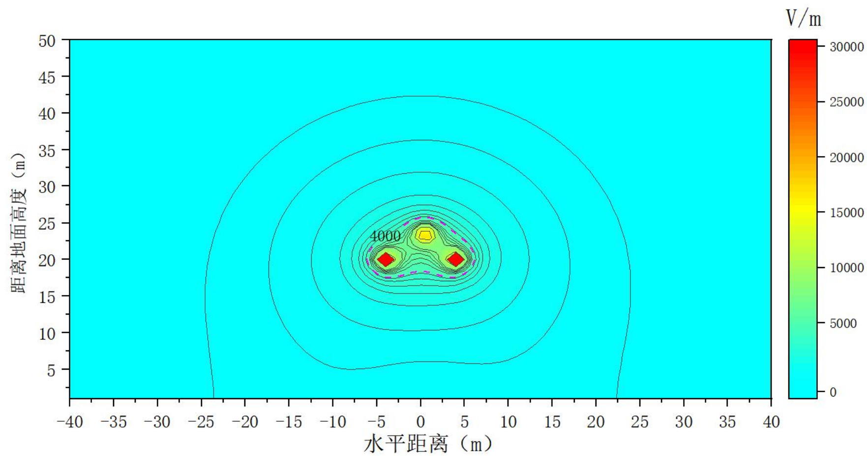
图 2 新建 110kV 单回架空线路工频电场强度空间分布图
