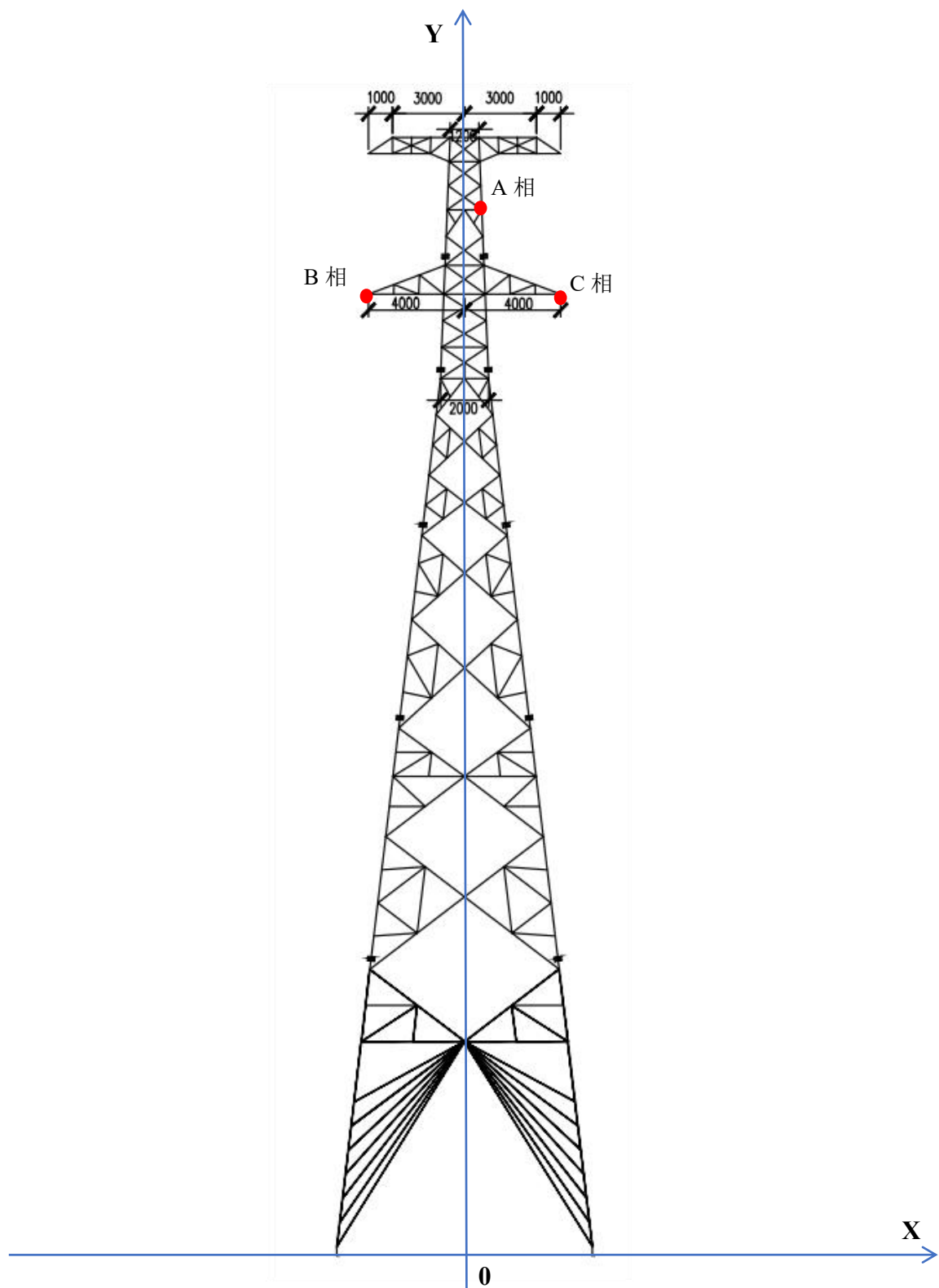
图 1 本项目新建 110kV 单回架空线路工频电场、工频磁场预测建立的直角坐标系
