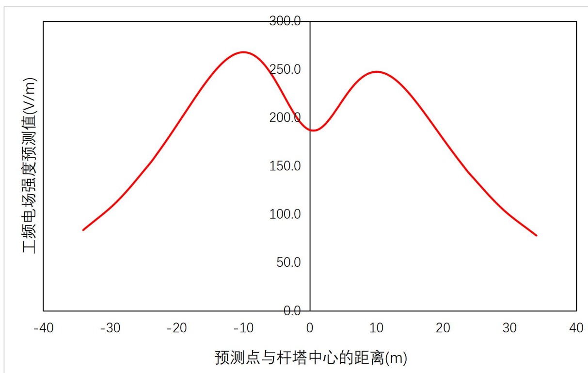
图 7 新建 110kV 单回架空线路离地 1.5m 处工频电场预测结果衰减趋势图
