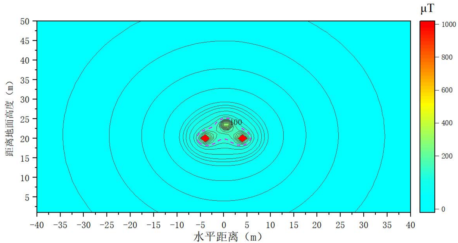
图 3 新建 110kV 单回架空线路工频磁感应强度空间分布图
