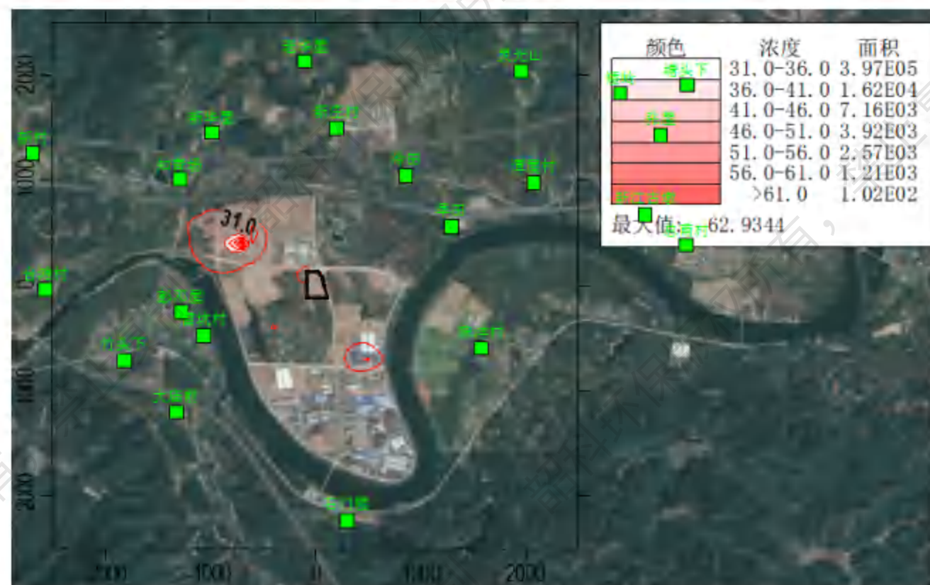
图 6.1-9b 排放磷酸铁锂电芯破碎烘干分选废气情景时正常排放条件下叠加现状浓度后 PM_{10} 年均浓度分布图
