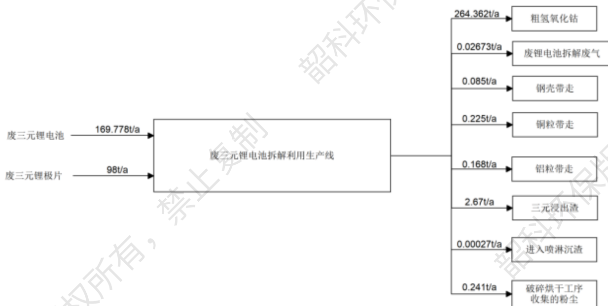
图3.5-4 本项目钴平衡图
