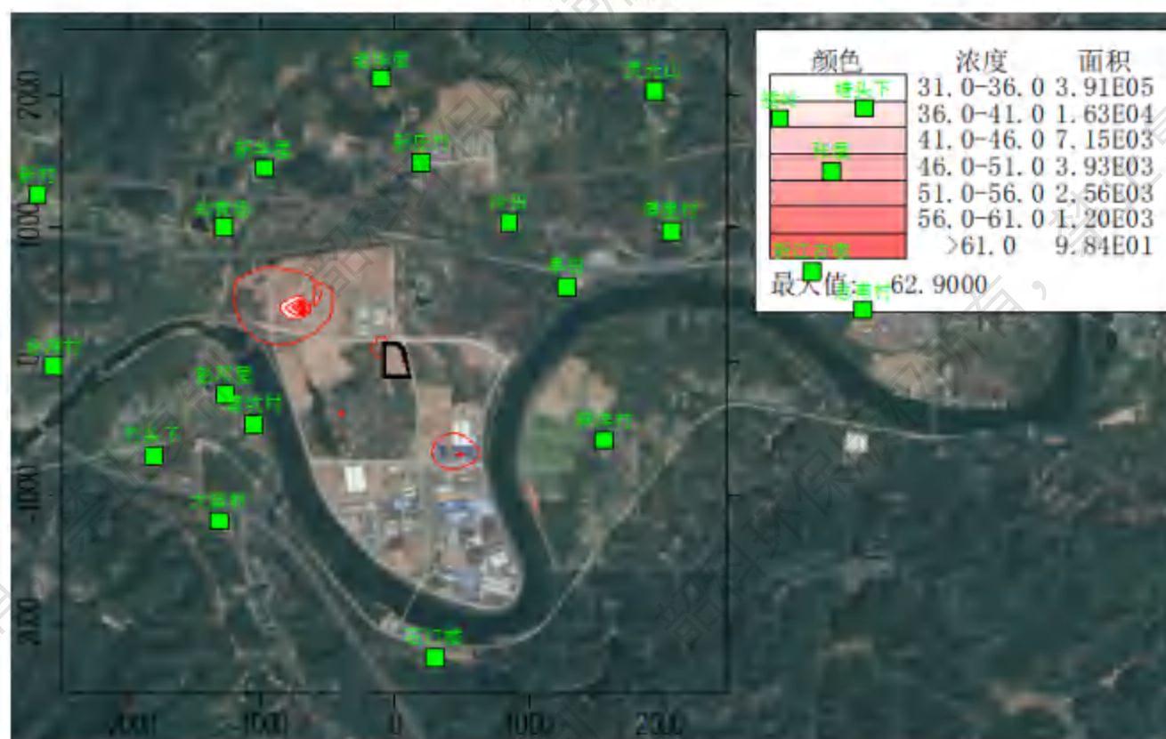
图 6.1-8b 排放三元锂电芯破碎烘干分选废气情景时正常排放条件下叠加现状浓度后 PM_{10} 年均浓度分布图
