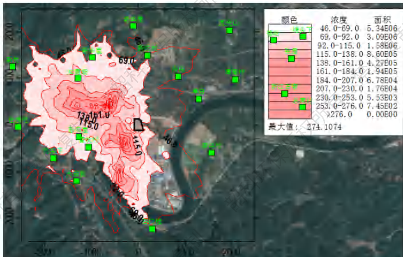
图 6.1-17 正常排放条件下叠加后硫酸小时浓度分布图
