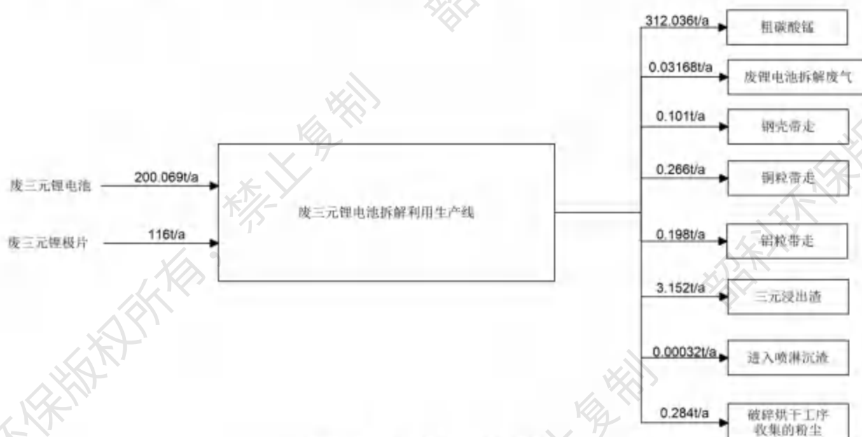
图3.5-3 本项目锰平衡图
