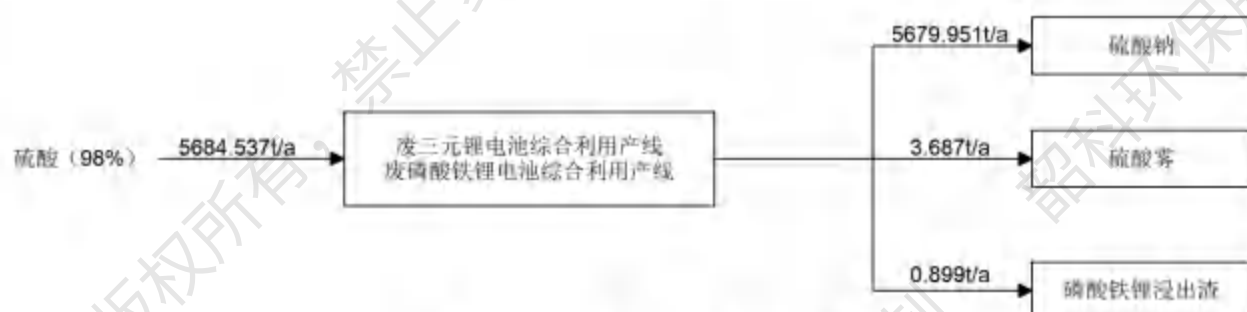
图3.5-7 本项目硫酸根平衡图
