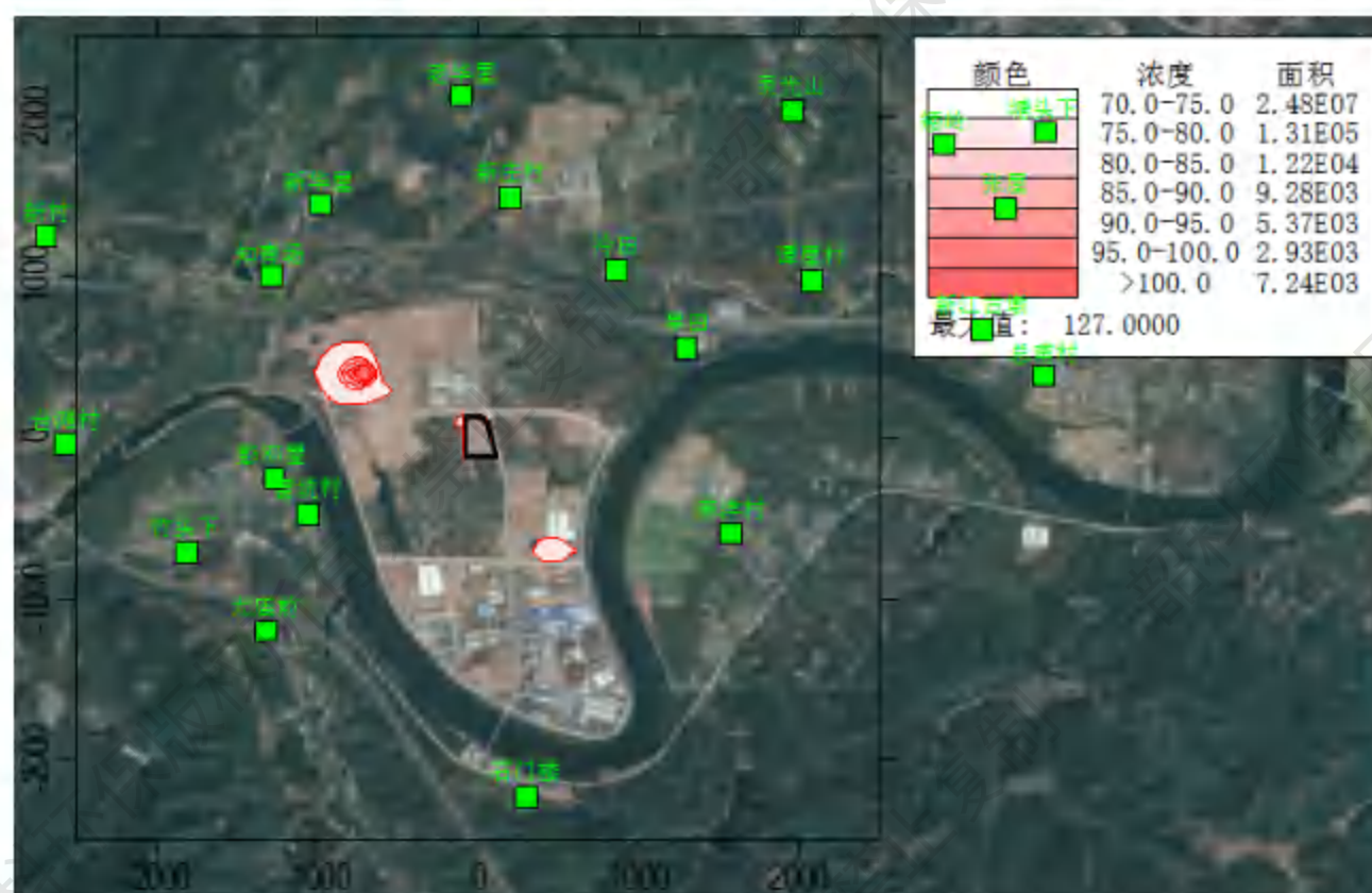
图 6.1-8a 排放三元锂电芯破碎烘干分选废气情景时正常排放条件下叠加现状浓度后 PM_{10} 保证率日均浓度分布图
