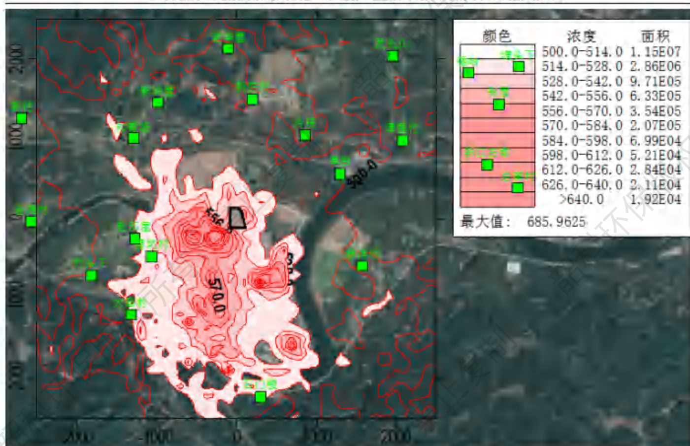
图 6.1-16 正常排放条件下叠加后 NMHC 小时浓度分布图
