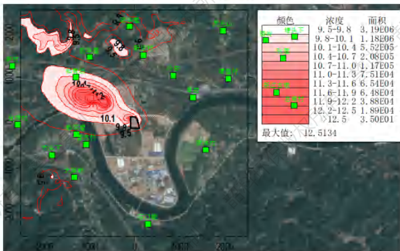
图 6.1-15 正常排放条件下叠加现状浓度后 \text{NO}_2 年均浓度分布图
