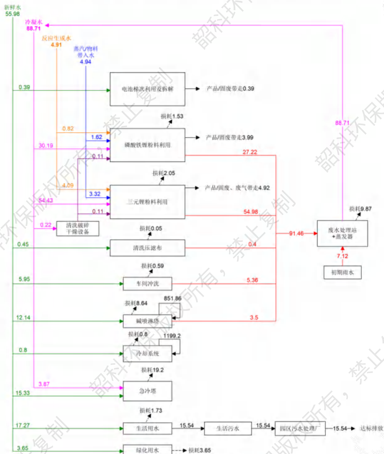
图 3.5-1 本项目水平衡图 (单位: \text{m}^3/\text{d} )
