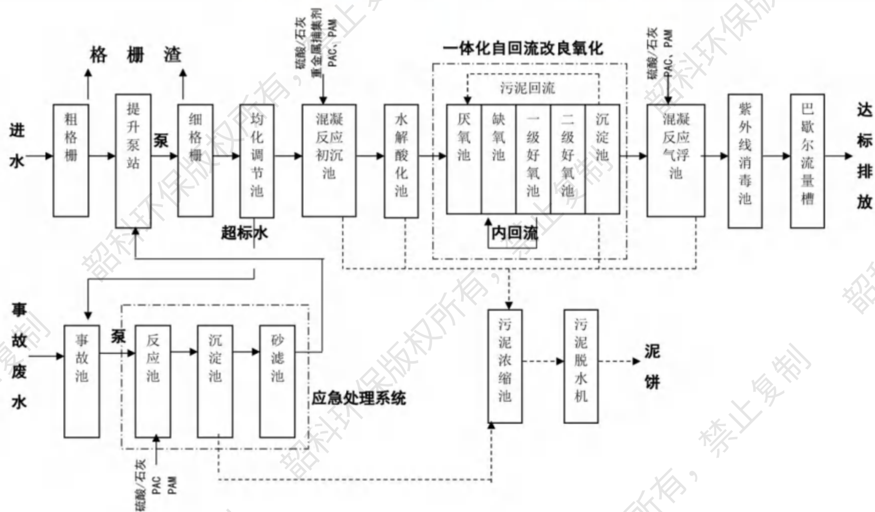
图 8.1-2 园区污水处理厂处理工艺流程图
