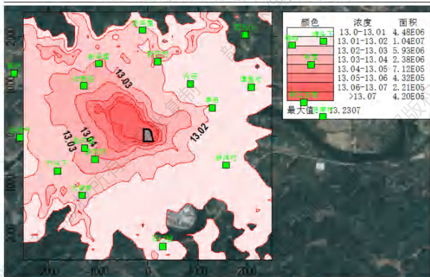
图 6.1-12 正常排放条件下叠加现状浓度后 SO 2 保证率日均浓度分布图
