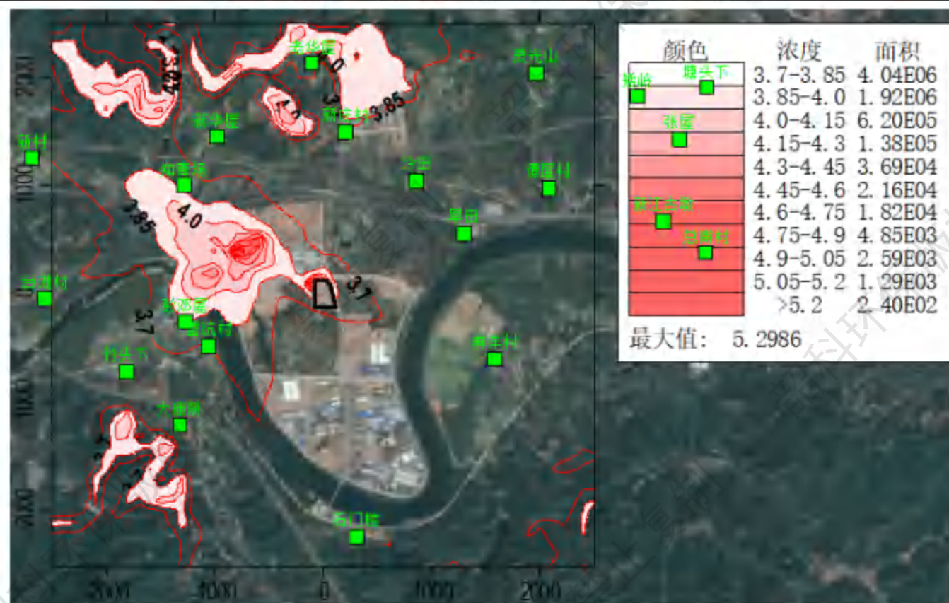
图 6.1-22 正常排放条件下叠加后氟化物日均浓度分布图
