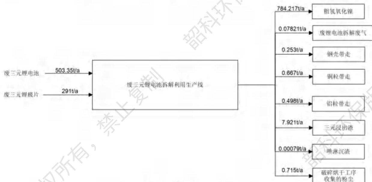
图3.5-5 本项目镍平衡图
