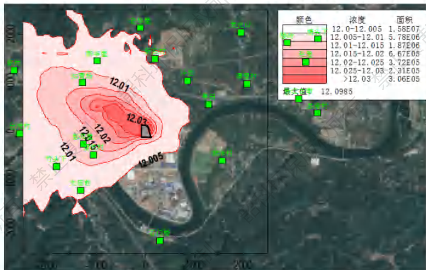
图 6.1-13 正常排放条件下叠加现状浓度后 SO 2 年均浓度分布图
