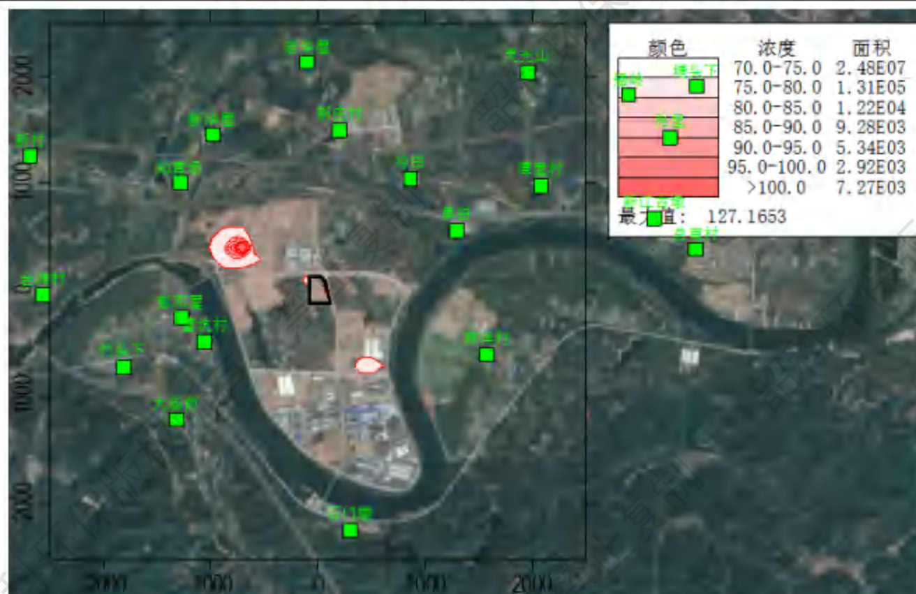
图 6.1-9a 排放磷酸铁锂电芯破碎烘干分选废气情景时正常排放条件下叠加现状浓度后 PM_{10} 保证率日均浓度分布图
