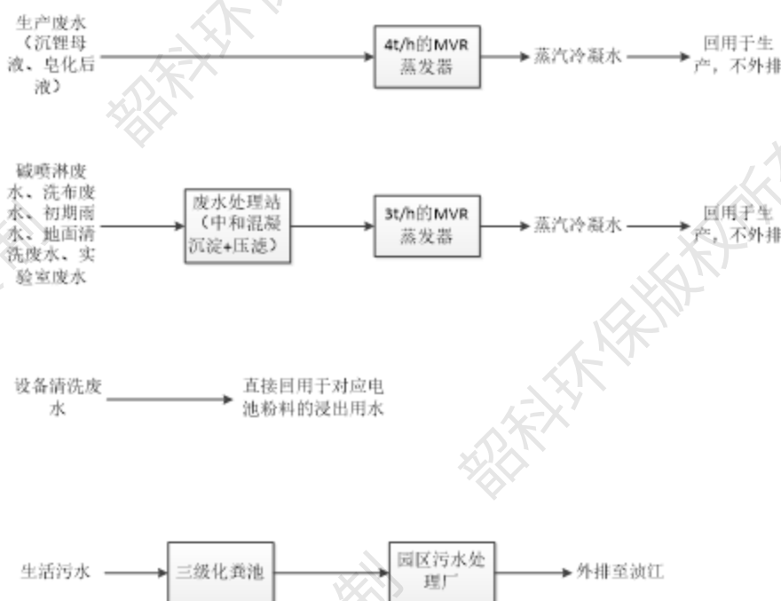
图8.1-1 废水处理工艺流程图
