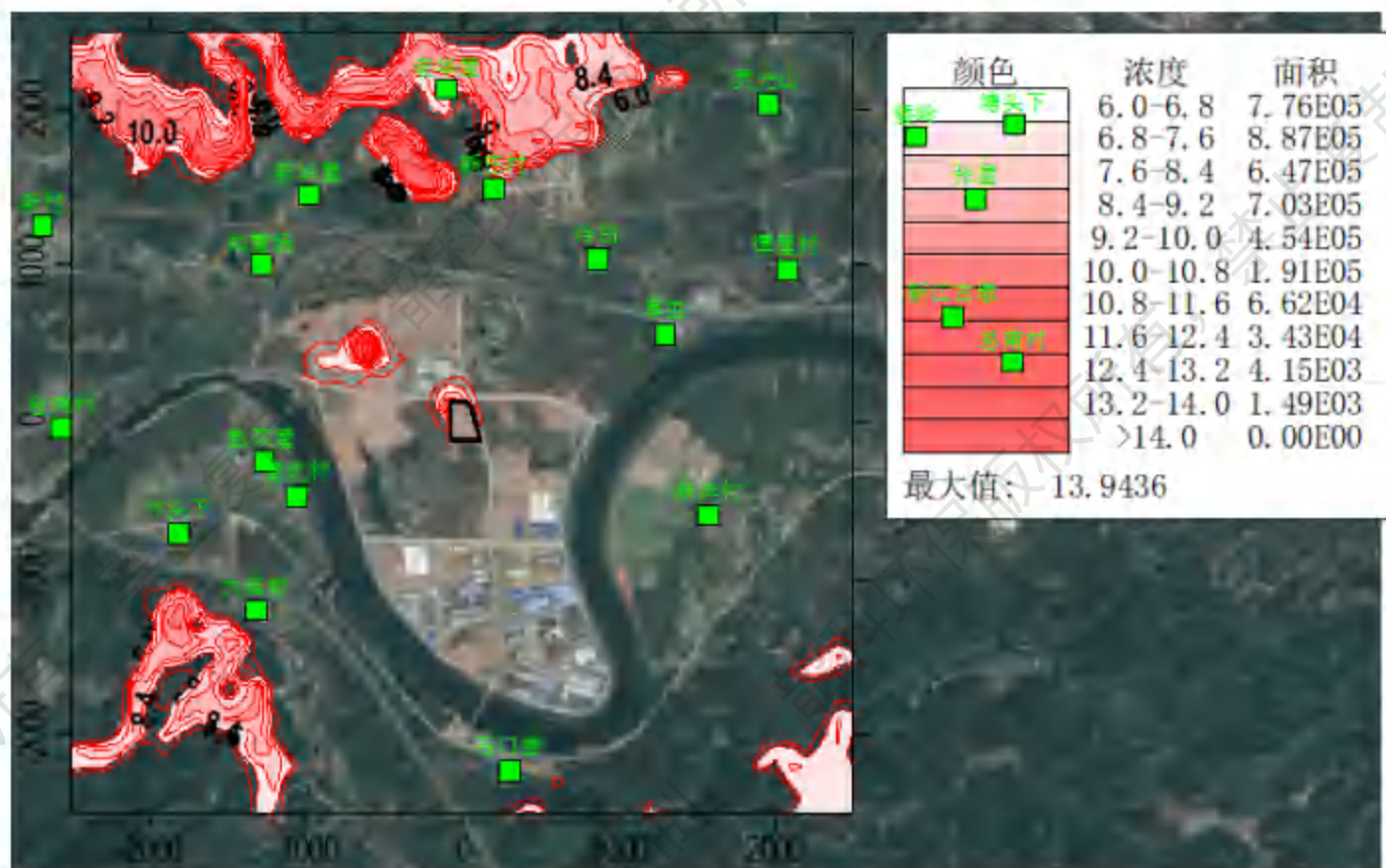
图 6.1-21 正常排放条件下叠加后氟化物小时浓度分布图
