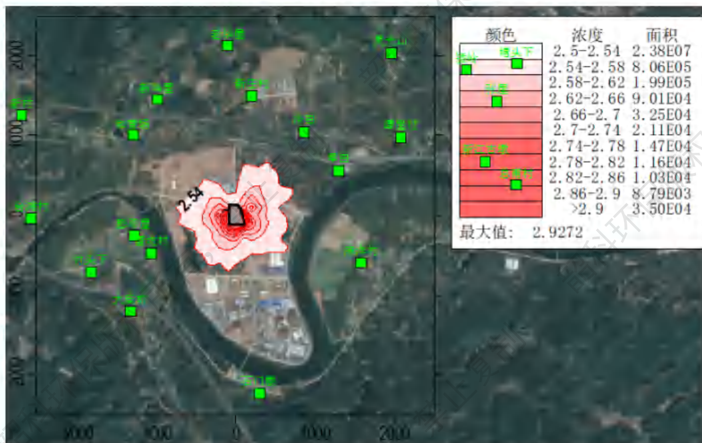
图 6.1-20 正常排放条件下叠加后氯化氢日均浓度分布图
