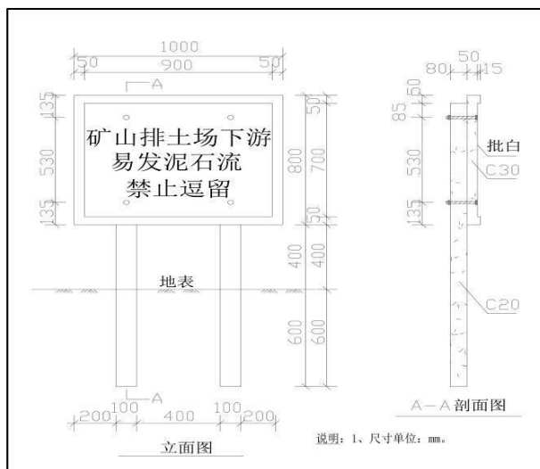
图 5-2 排土场警示牌工程
