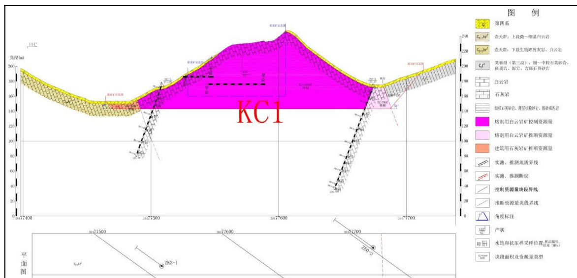
图2-3 典型地质剖面图
