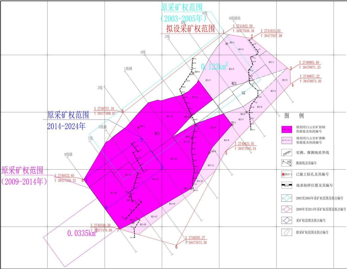
图2-2 熔剂用白云岩矿体分布图
