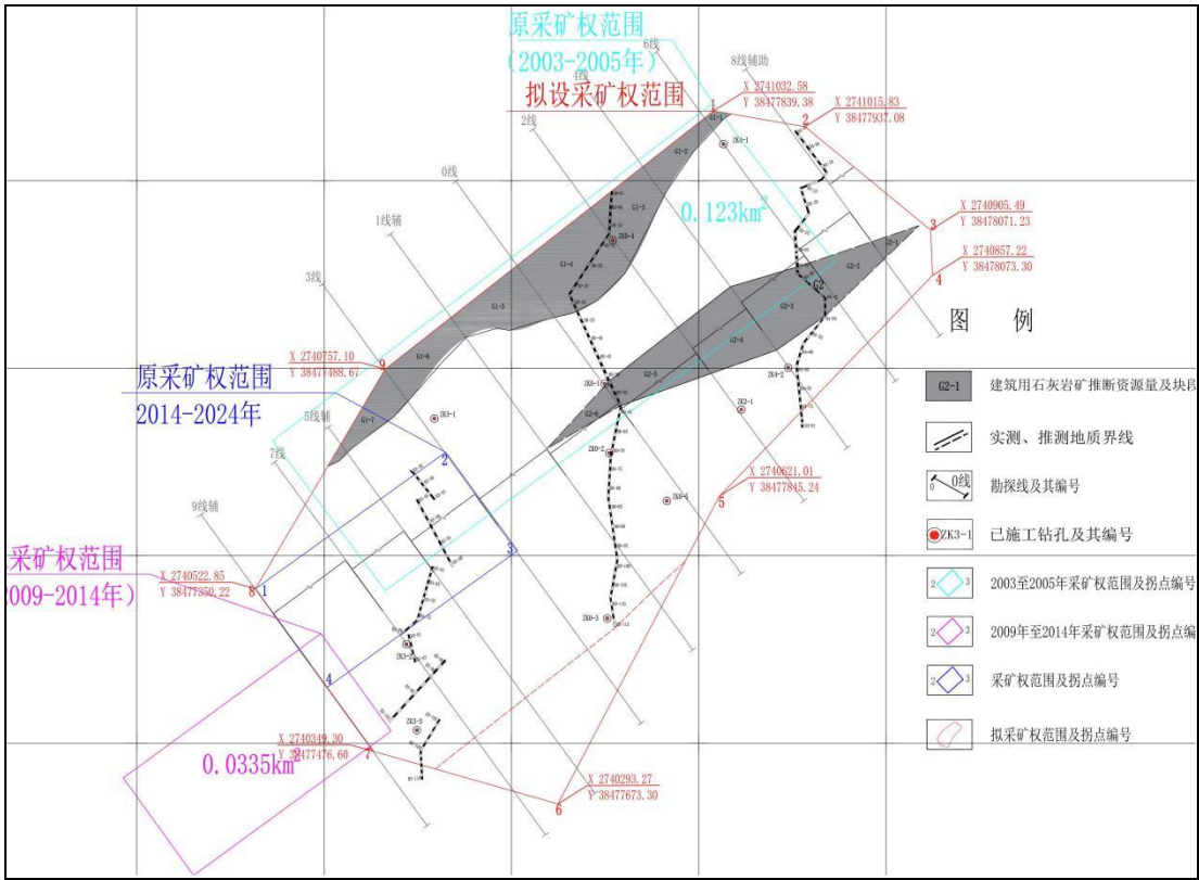
图2-4 建筑用灰岩矿体分布图
