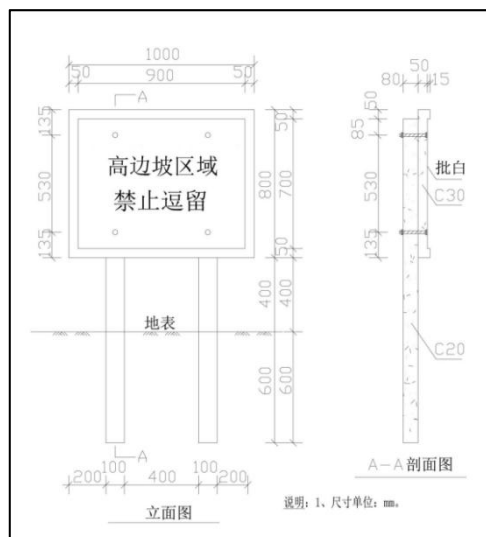
图5-1 边坡警示牌工程
