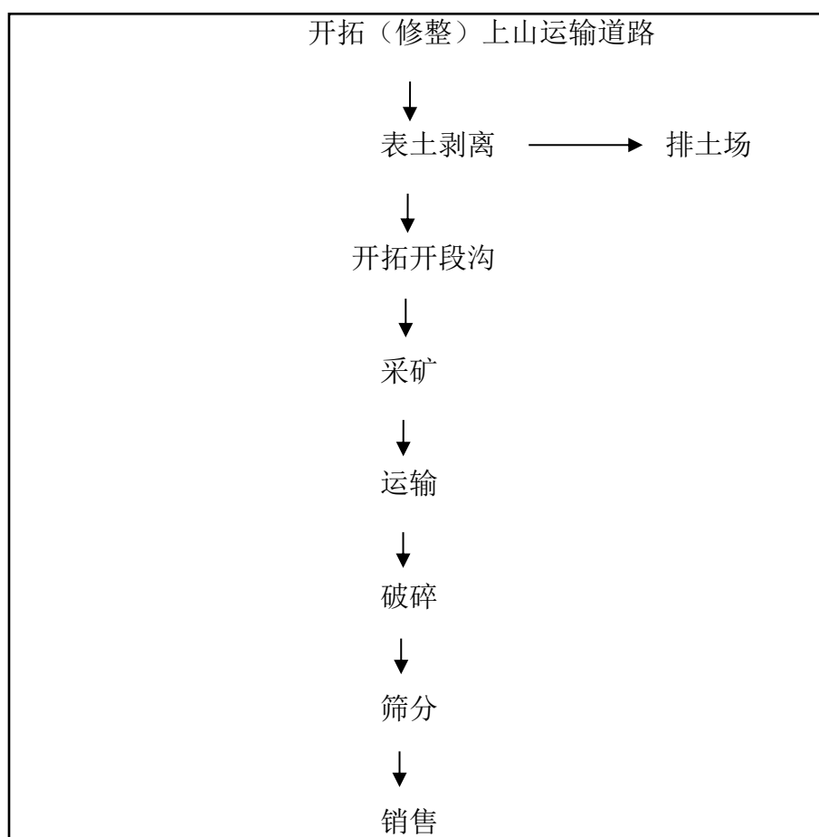
图1-4 矿山生产工艺流程示意图
