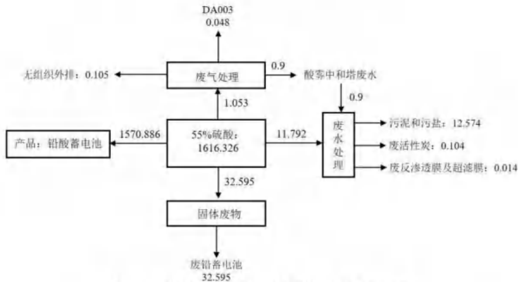
图 2.5-3 项目硫酸平衡图 (以硫酸根 \text{SO}_4^{2-} 计, t/a)
