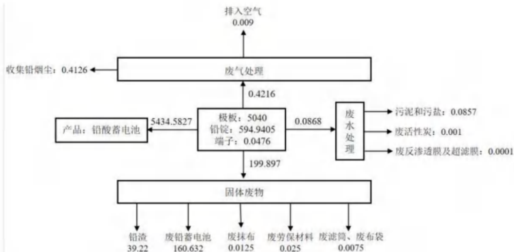
图 2.5-2 项目铅元素平衡图 (t/a)
