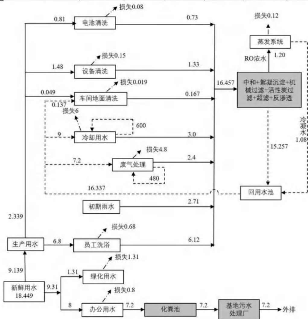
图 2.5-4 项目水平衡图 (m³/d)
