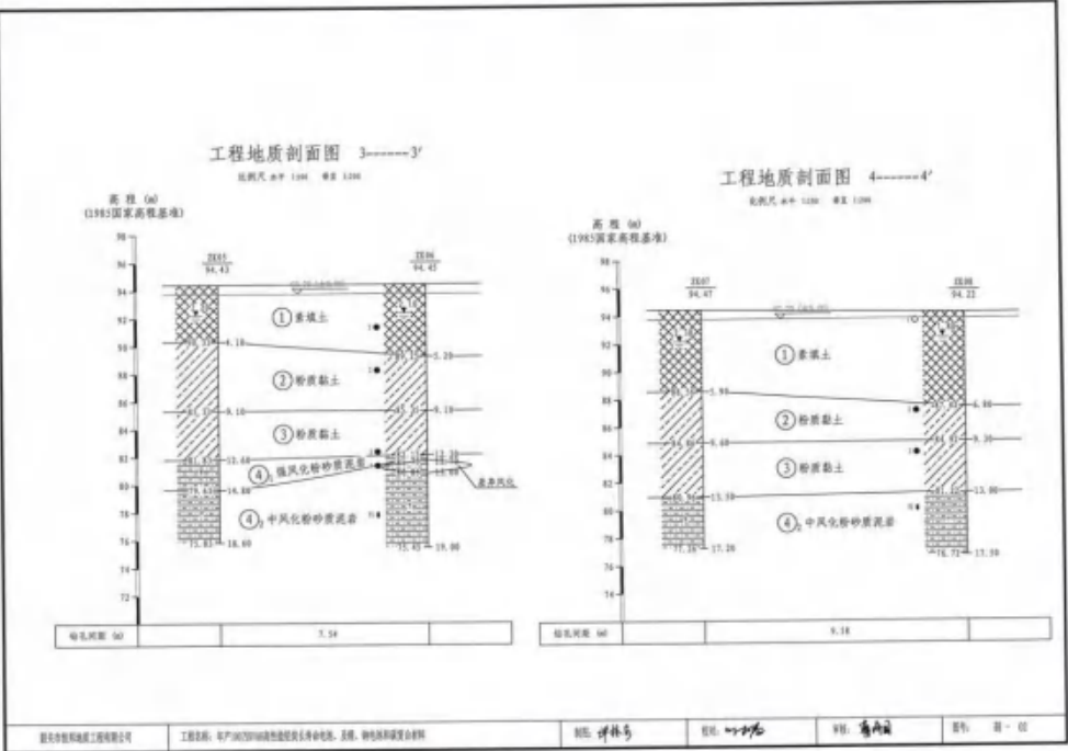
图 4.3-2b 工程地质剖面图 (剖面 3-3' 4-4')
