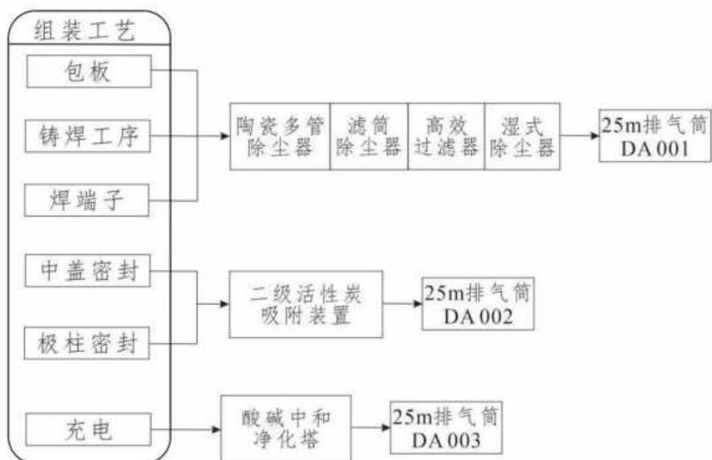
图 2.4-3 项目废气收集处理示意图
