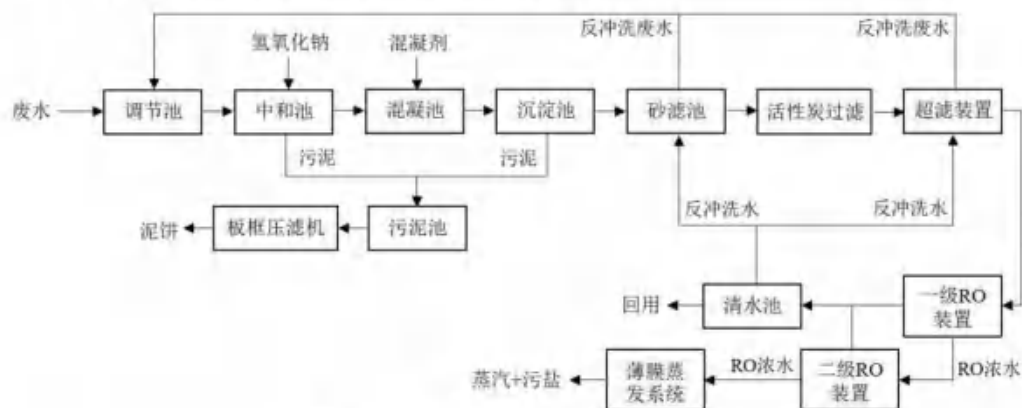
图 6.1-1 项目铅酸废水处理系统工艺流程图
