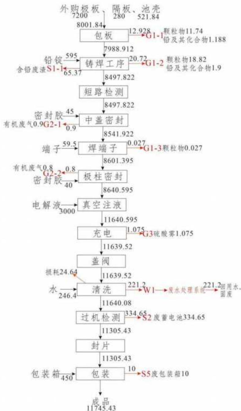
图 2.5-1 项目总物料平衡图 (t/a)
