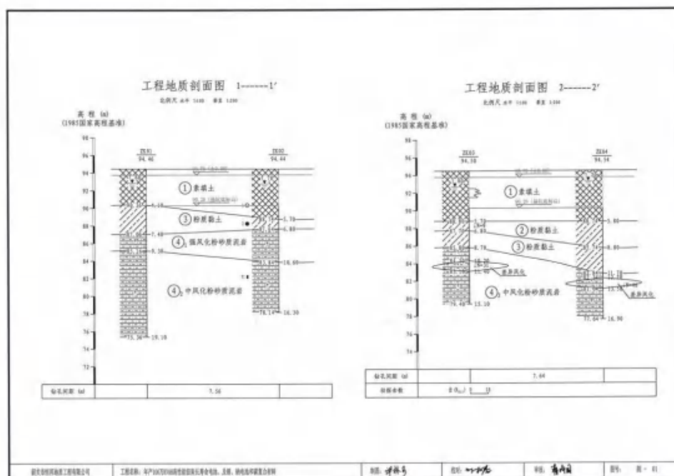
图 4.3-2a 工程地质剖面图 (剖面 1-1' 2-2')
