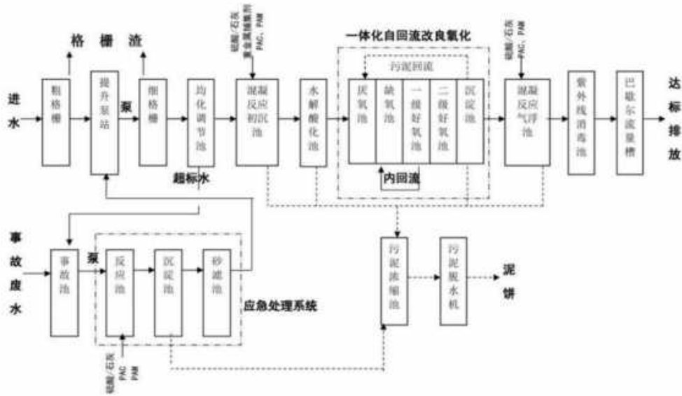
图 6.1-2 基地污水处理厂处理工艺流程图
