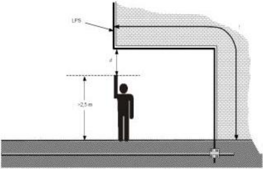
图 5-2 具有悬臂部件的建筑物的 LPS 设计
