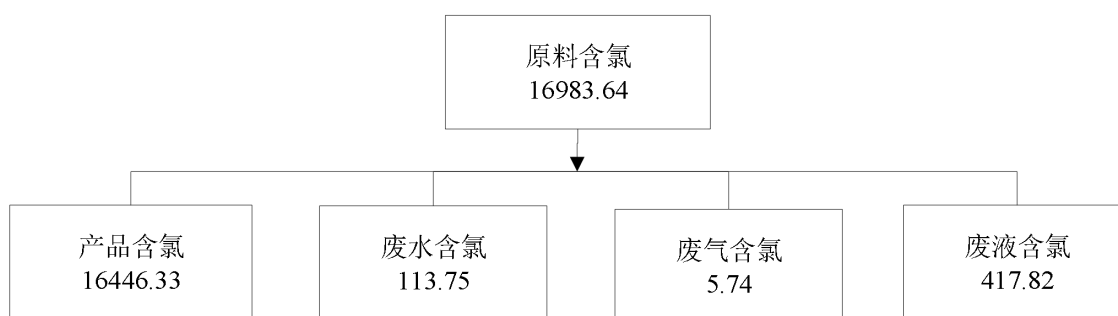
图 3.1-8 已验收投产项目氯平衡图（单位：t/a）
