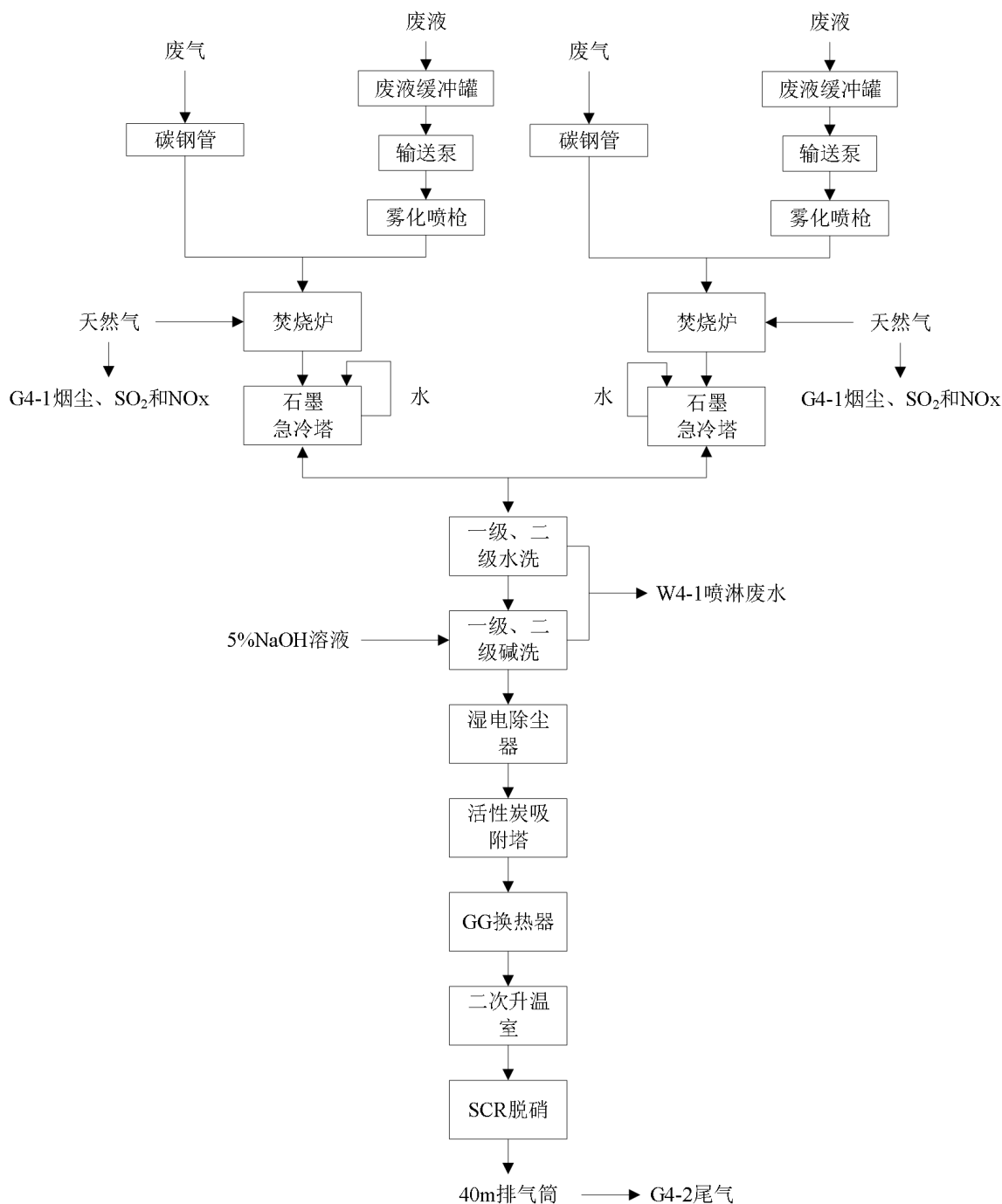
图7.2-6 焚烧炉焚烧工艺流程及产污环节
