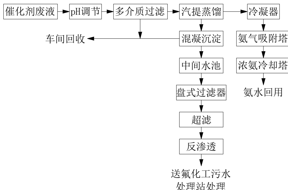
图 5.2-5 催化剂废水处理工艺流程图
