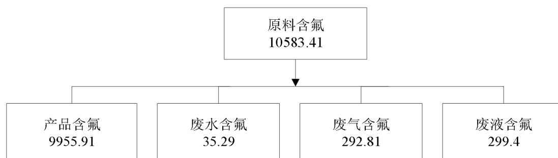
图 3.1-9 已验收投产项目氟平衡图（单位：t/a）
