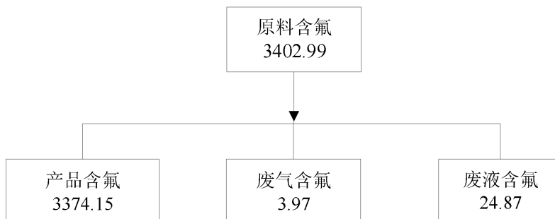
图 4.8-8 VDF 装置升级改造后氟平衡图（单位：t/a）
