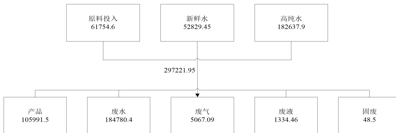
图 3.2-3 在建项目工艺物料平衡图 (单位: t/a)
