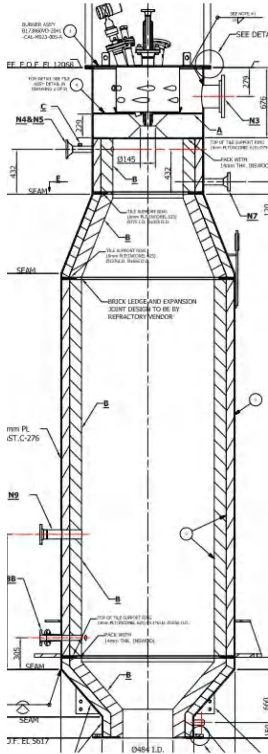
图 7.2-5 焚烧炉炉膛示意图
