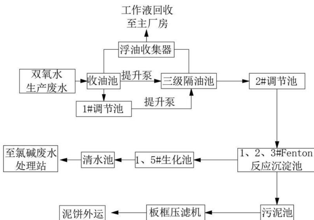
图 5.2-2 双氧水废水的处理工艺流程
