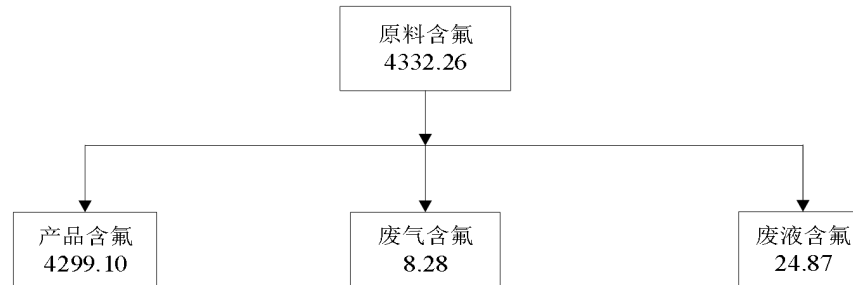
图 4.8-15 技改项目工艺氟平衡图 (单位: t/a)
