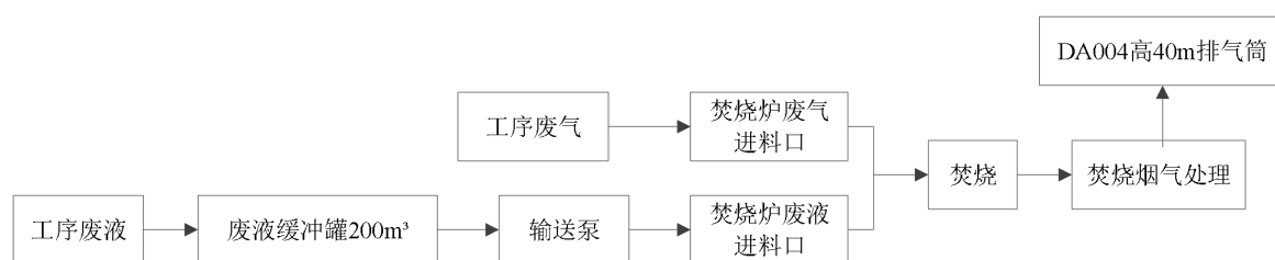
图 7.2-3a 焚烧物料进料工艺流程示意图
