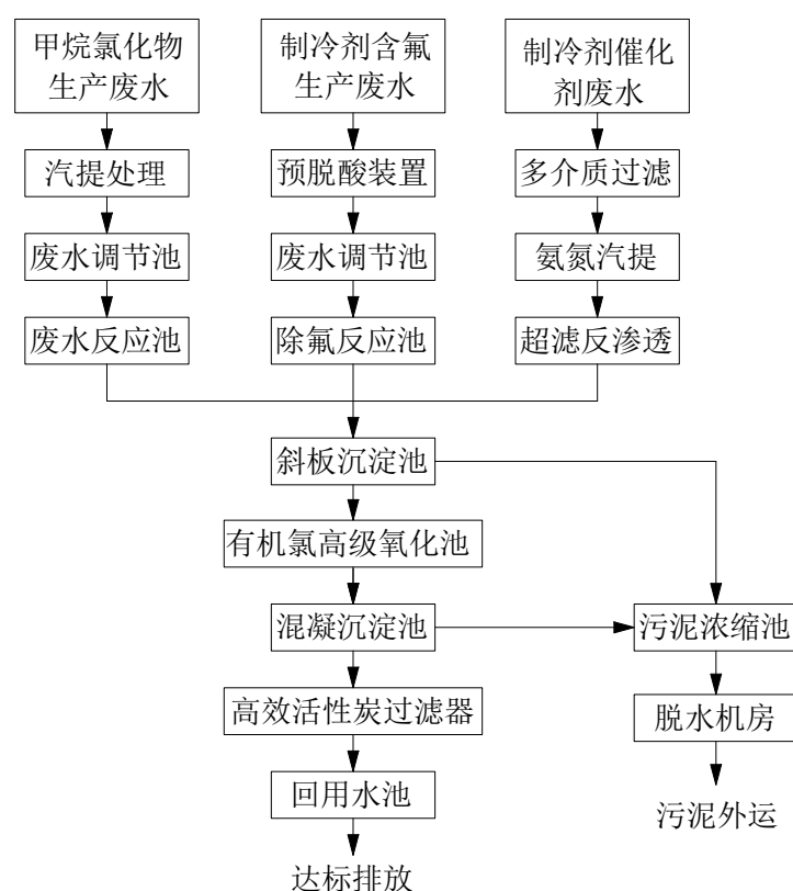
图 5.2-6 氟有限废水处理站处理工艺流程图
