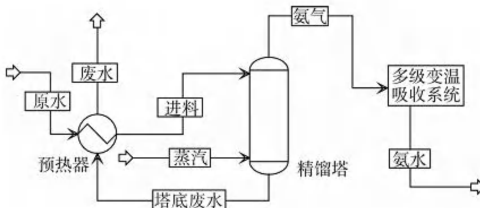
图 5.2-4 催化剂废水汽提脱氨工艺流程图
