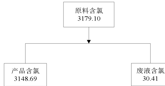
图 4.8-14 技改项目工艺氯平衡图 (单位: t/a)
