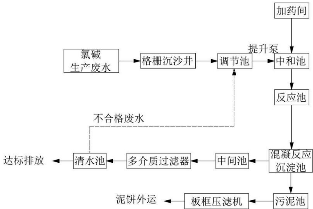
图 5.2-1 氯碱废水处理站处理工艺流程图
