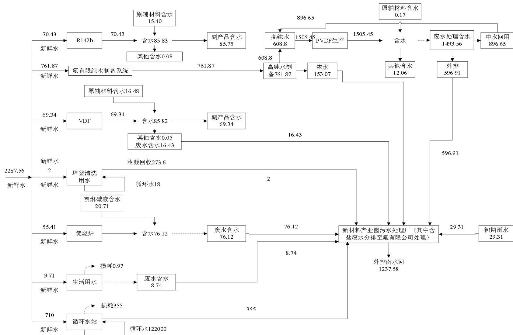
图 3.1-10 已验收投产项目水平衡图 (单位: m^3/d )
