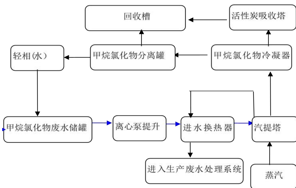
图 5.2-3 甲烷氯化物废水汽提工艺流程简图
