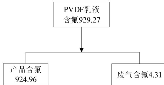
图 4.8-11 后处理喷雾干燥生产工序氟平衡图 (单位: \text{t/a} )
