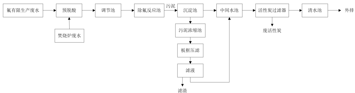
图 3.1-11 氟有限公司生产废水处理工艺
