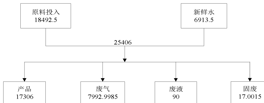
图 4.8-12 技改项目工艺物料平衡图（单位：t/a）
