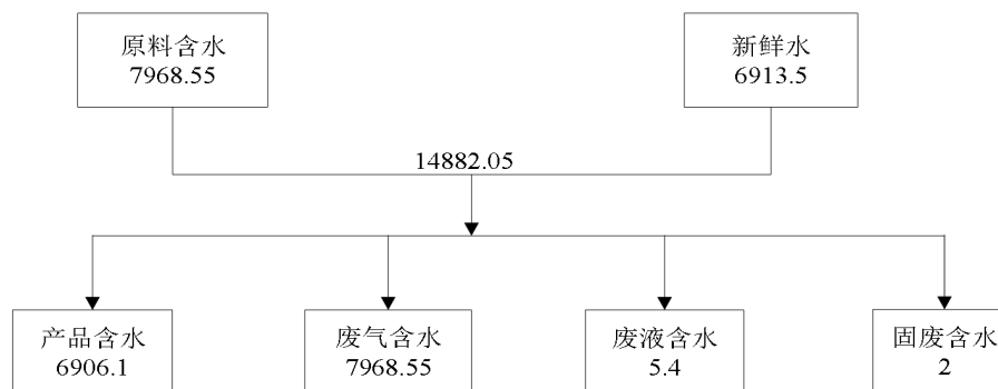
图 4.8-13 技改项目工艺水平衡图（单位：m³/a）
