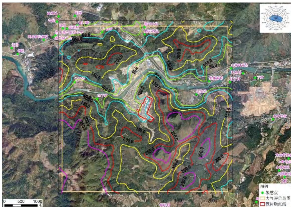
图 6.4-6 预测区域等高线示意图
