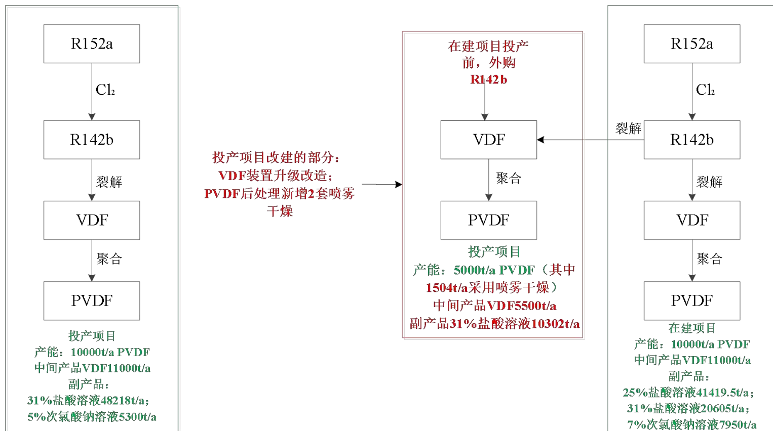
图4.8-1 氟树脂有限公司总体工艺路线示意图
