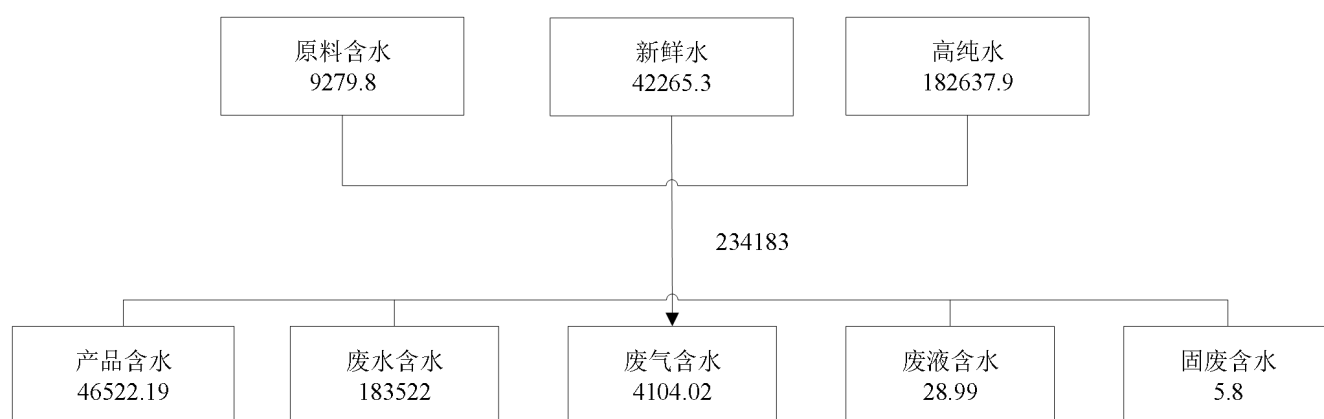
图 3.1-7 已验收投产项目工艺水平衡图（单位：m³/a）
