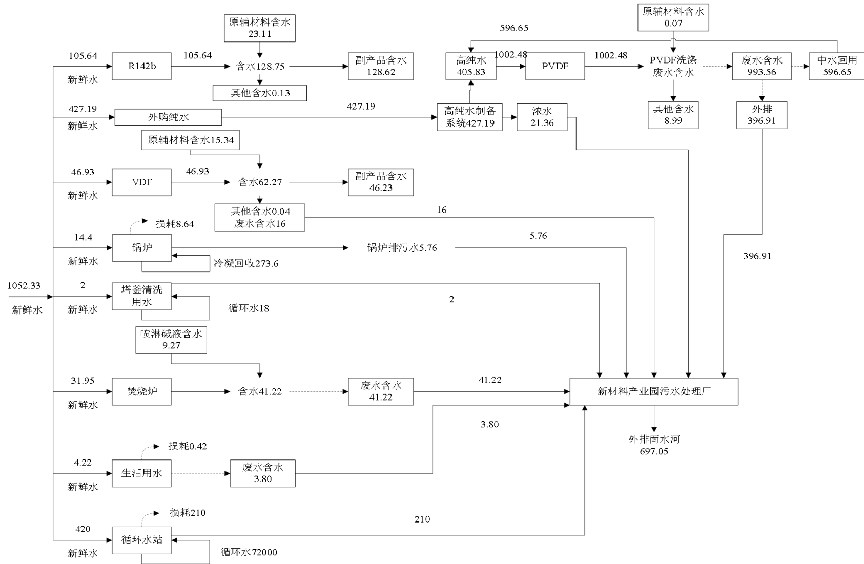
图 3.2-4 在建项目水平衡图 (单位: m³/d)
