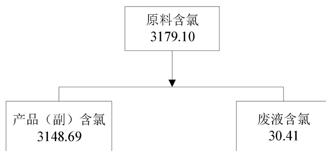
图 4.8-7 VDF 装置升级改造后氯平衡图（单位：t/a）
