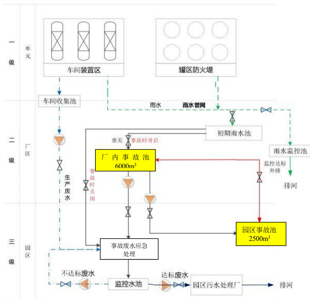
图 6.8-12 环境风险三级防控系统图
