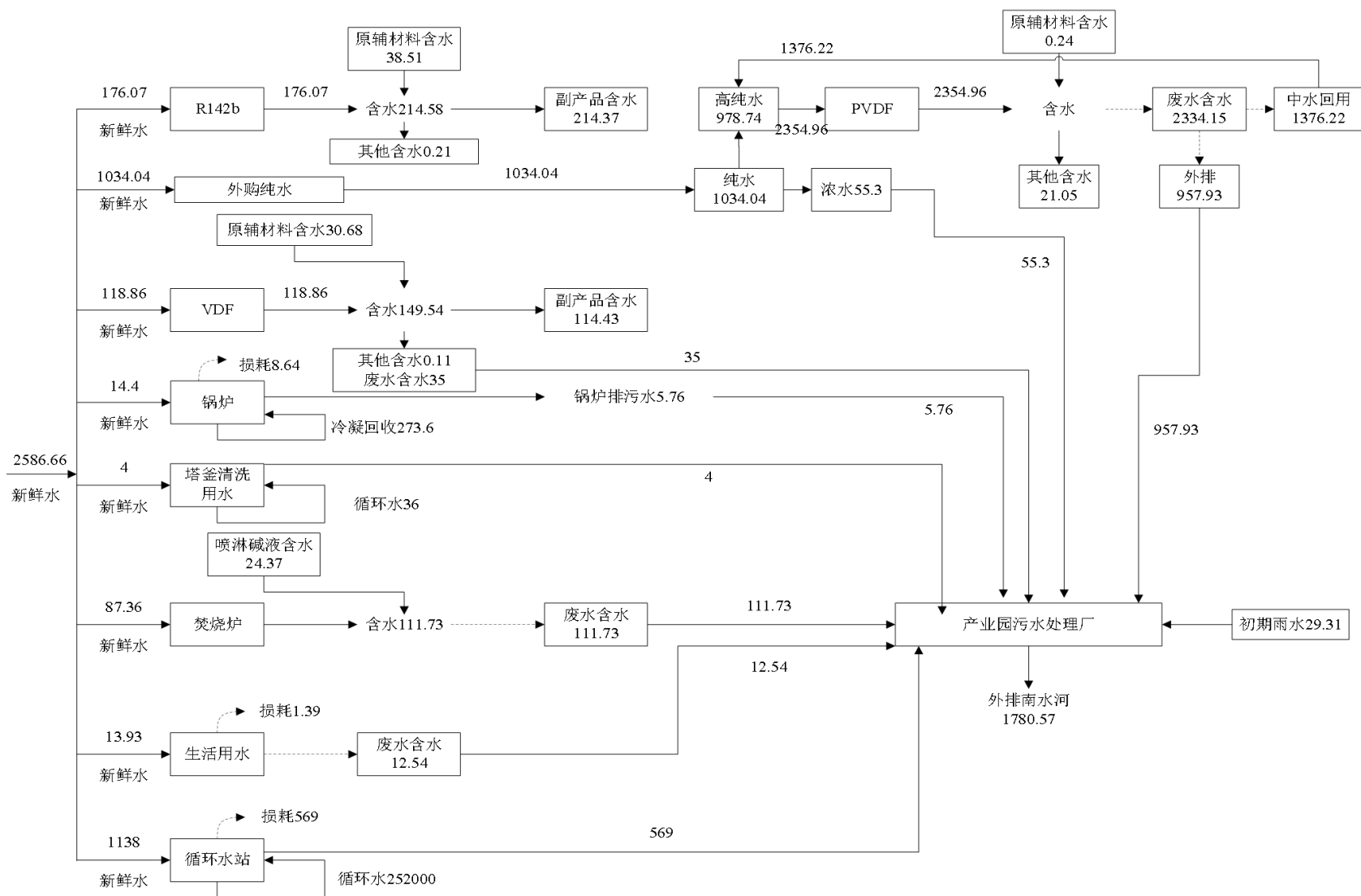
图 4.8-17 技改项目实施后全厂水平衡图 (单位: \text{m}^3/\text{d} )
