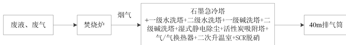
图 7.2-4 焚烧炉烟气处理工艺流程示意图
