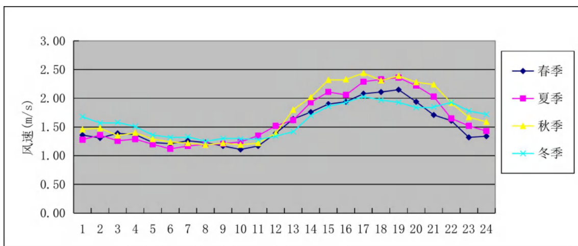
图 6.4-4 季小时平均风速日变化图
