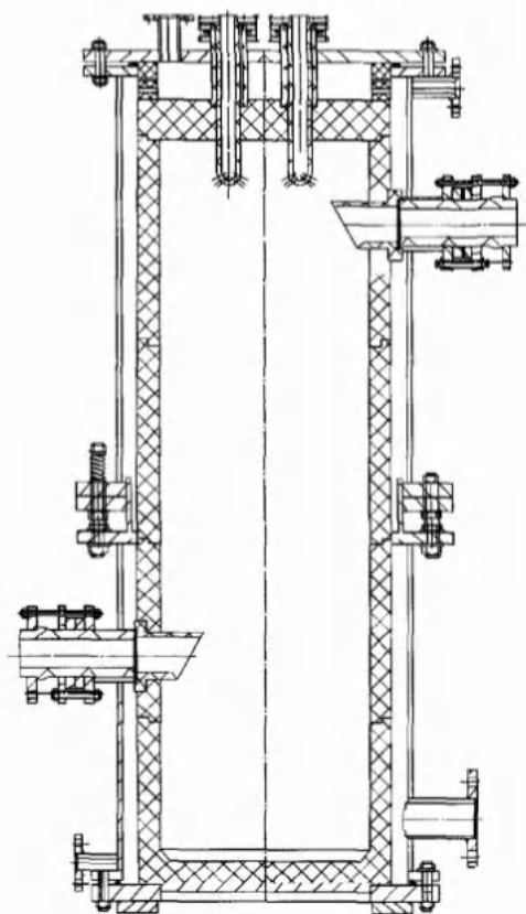
图 7.2-7 石墨急冷塔的结构图
