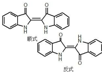
靛蓝分子式
