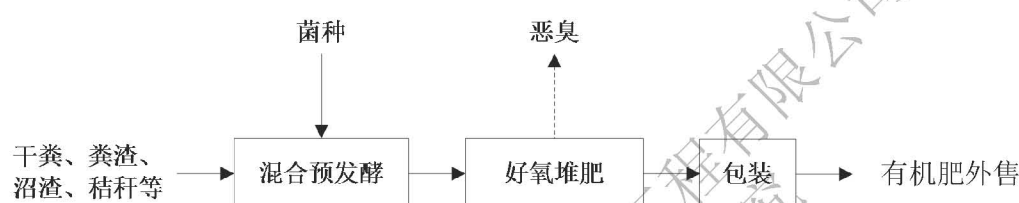
图3-9 粪渣等制作有机肥料工艺流程图
