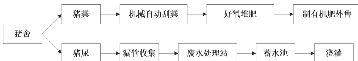
图 3-7 粪污处理工艺流程图
