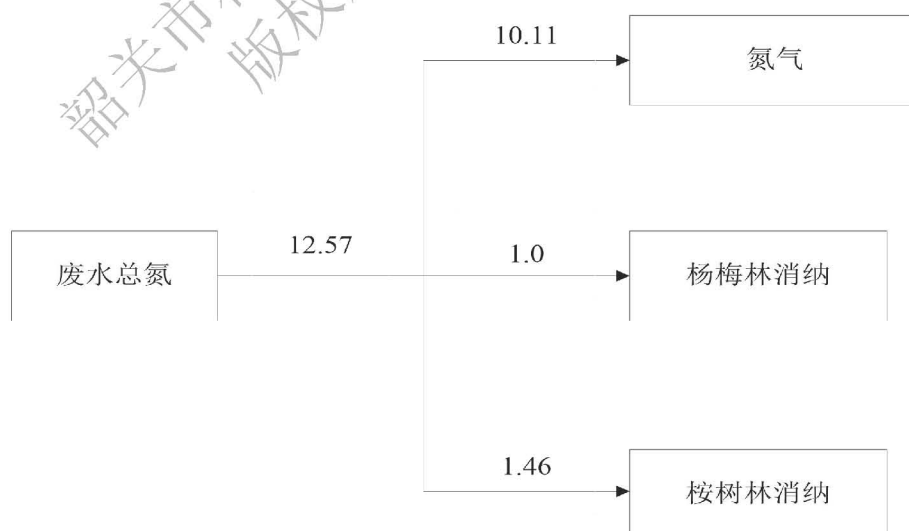
图 3-12 本项目总氮平衡图 (t/a)
