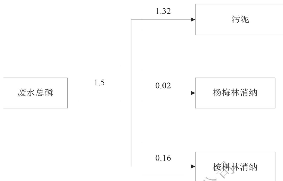
图 3-13 本项目总磷平衡图 (t/a)
