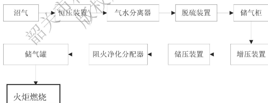
图 3-8 沼气燃烧工艺流程图
