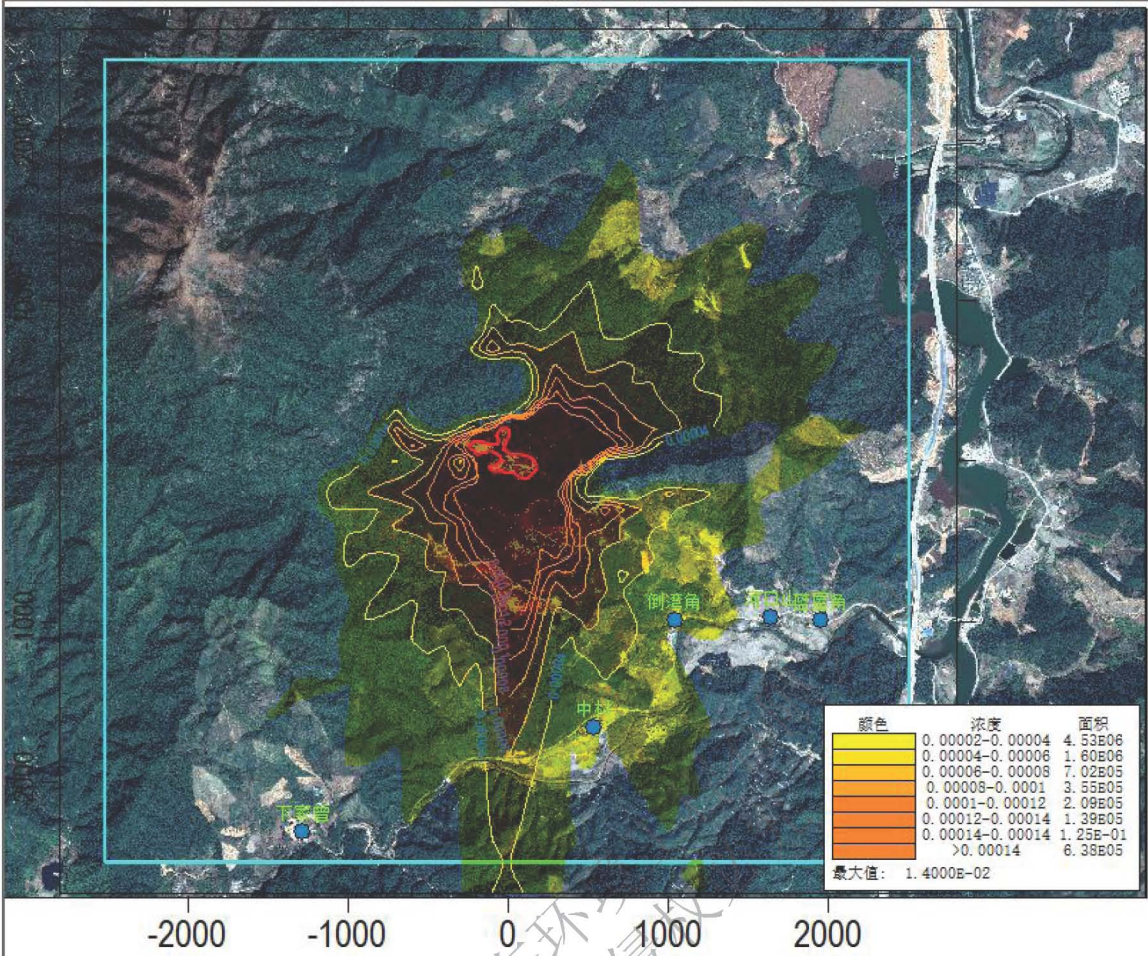
图 5-12 正常工况 NO 2 日均浓度贡献值分布图 (mg/m 3 )
