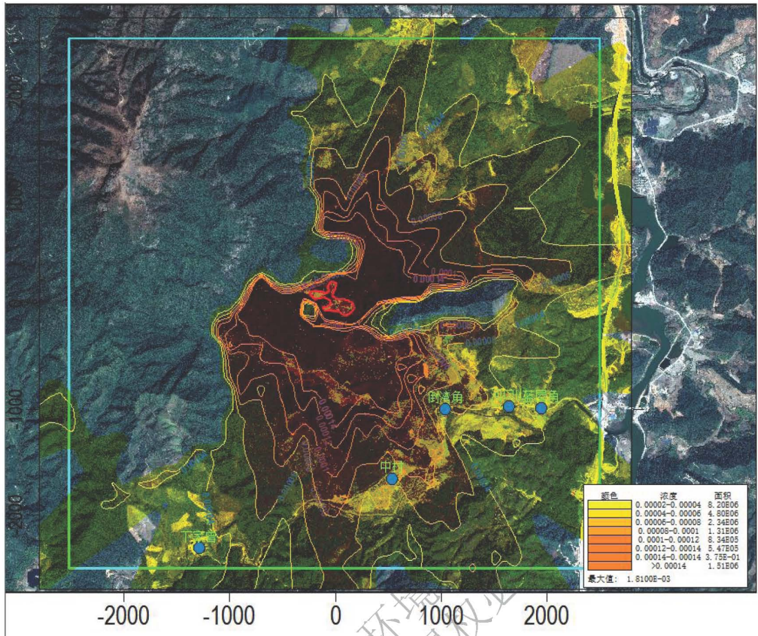
图 5-9 正常排放情况下新增污染源 H_2S 小时平均浓度最大值分布图
