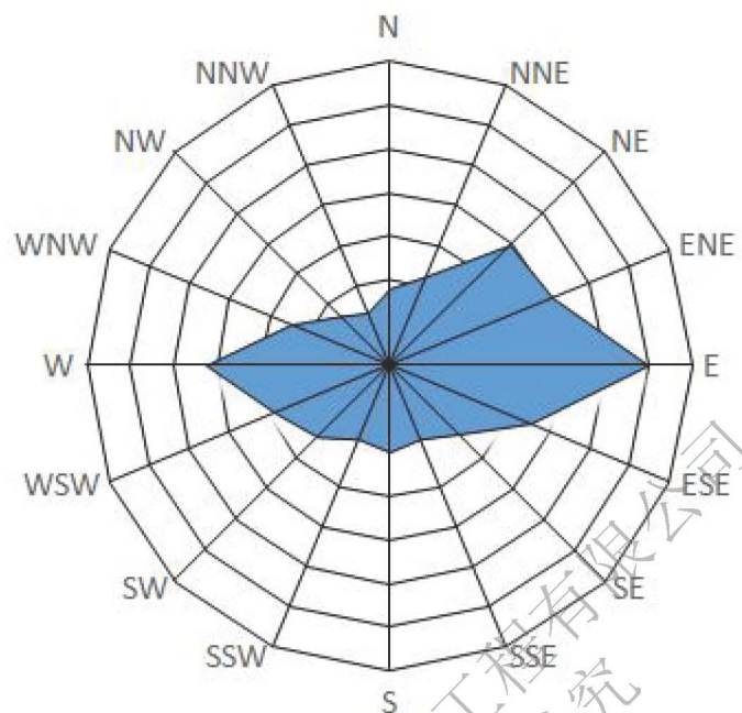
图 5-2 始兴气象站风向玫瑰图（统计年限：2002-2021）
