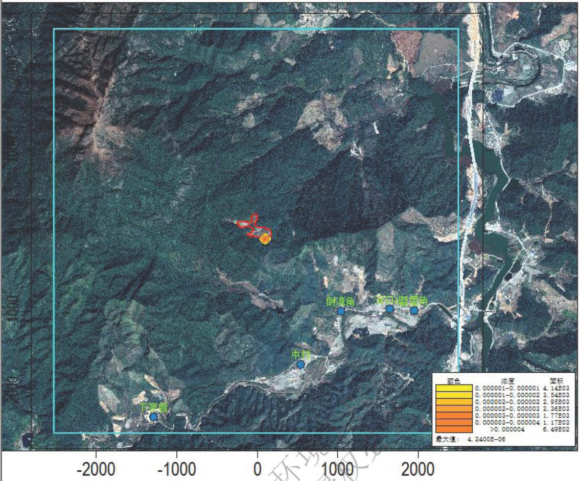
图 5-11 正常工况 SO 2 年均浓度贡献值分布图 (mg/m 3 )
