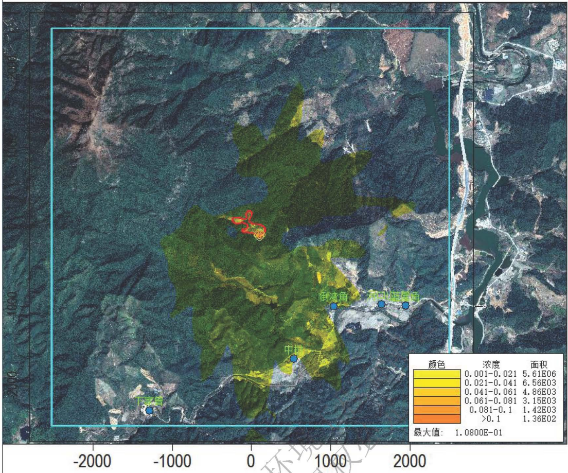
图 5-8 正常排放情况下新增污染源 \text{NH}_3 小时平均浓度最大值分布图
