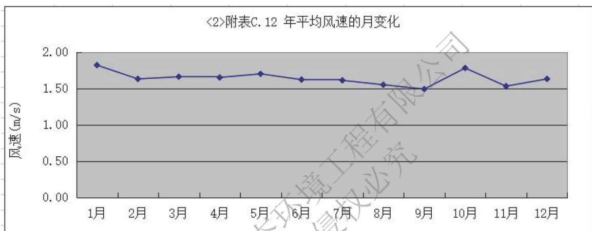
图 5-4 年平均风速的月变化曲线图
