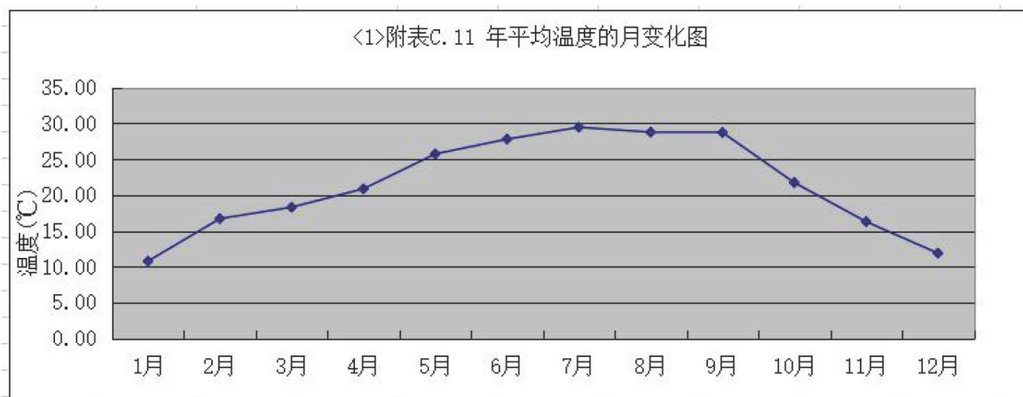
图 5-3 年平均温度的月变化曲线图
