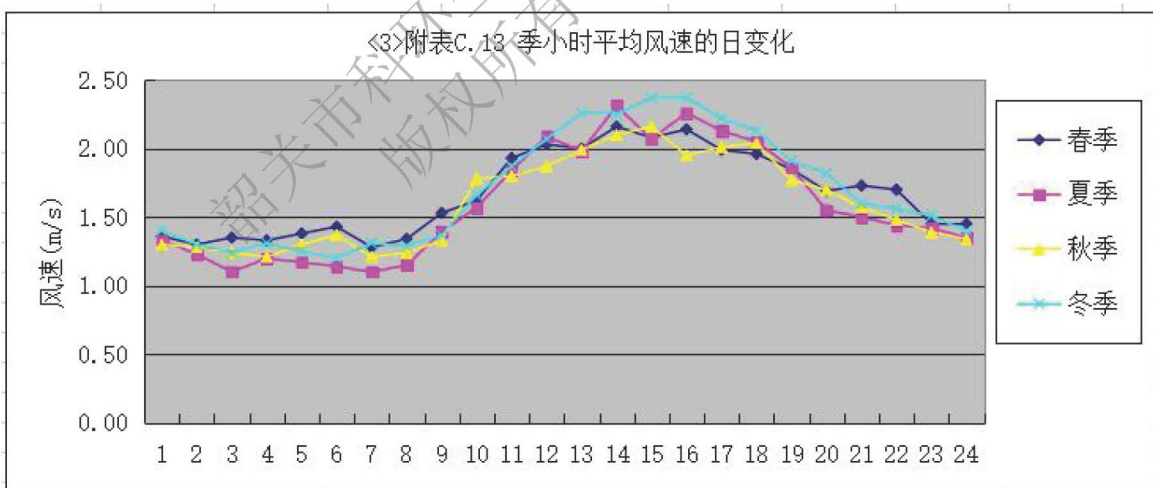
图 5-5 季小时平均风速的日变化曲线图
