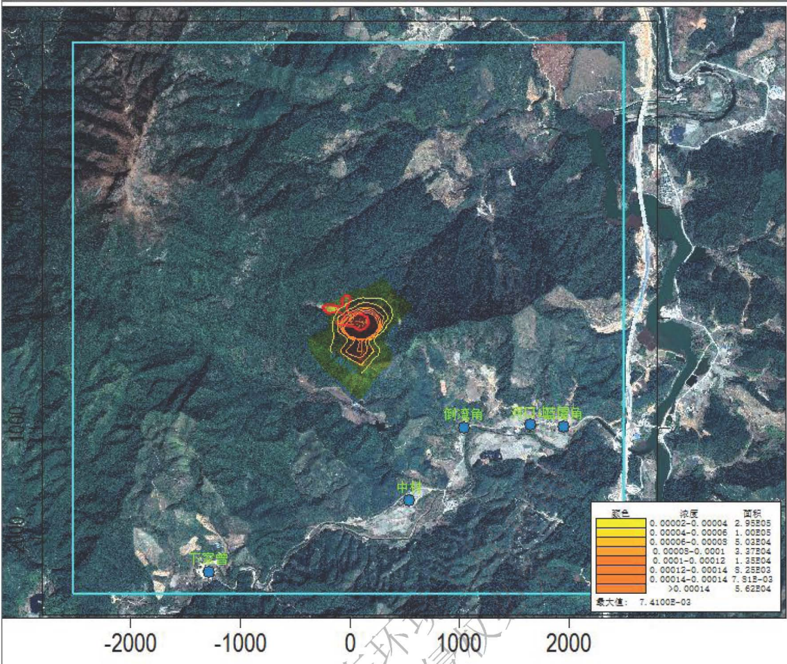
图 5-13 正常工况 \text{NO}_2 年均浓度贡献值分布图 ( \text{mg}/\text{m}^3 )
