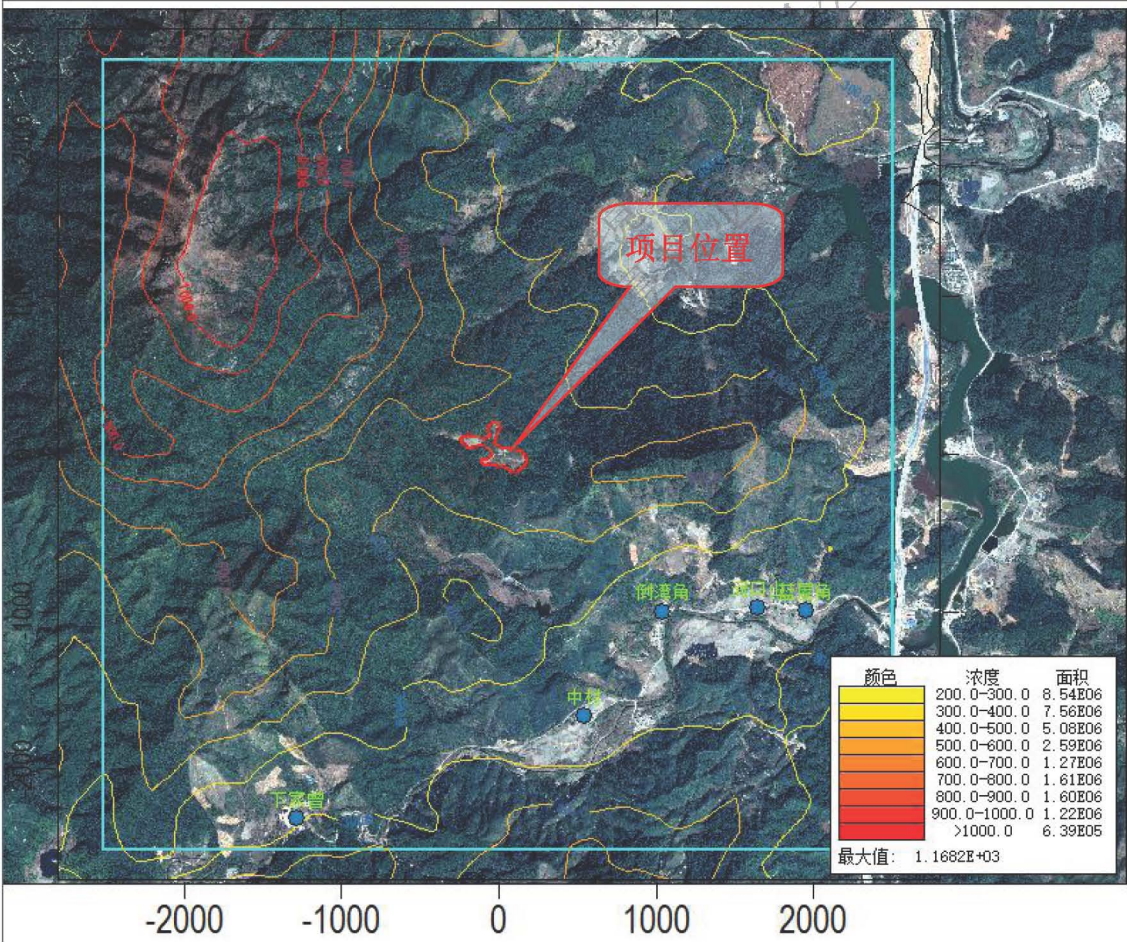
图 5-7 项目区域地形高程图
