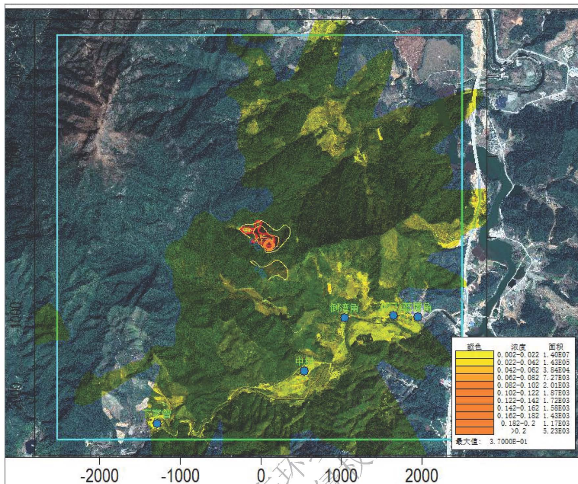
图 5-16 非正常排放情况下新增污染源 \text{NH}_3 小时平均浓度最大值分布图
