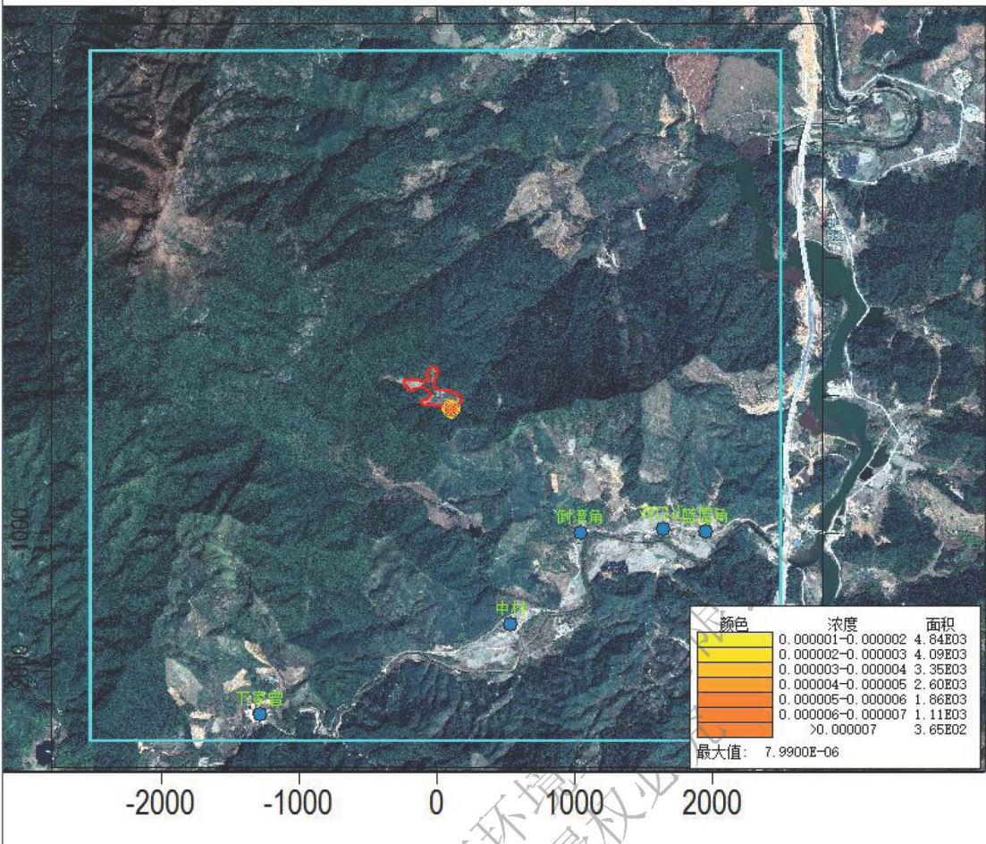
图 5-10 正常工况 SO 2 日均浓度贡献值分布图 (mg/m 3 )
