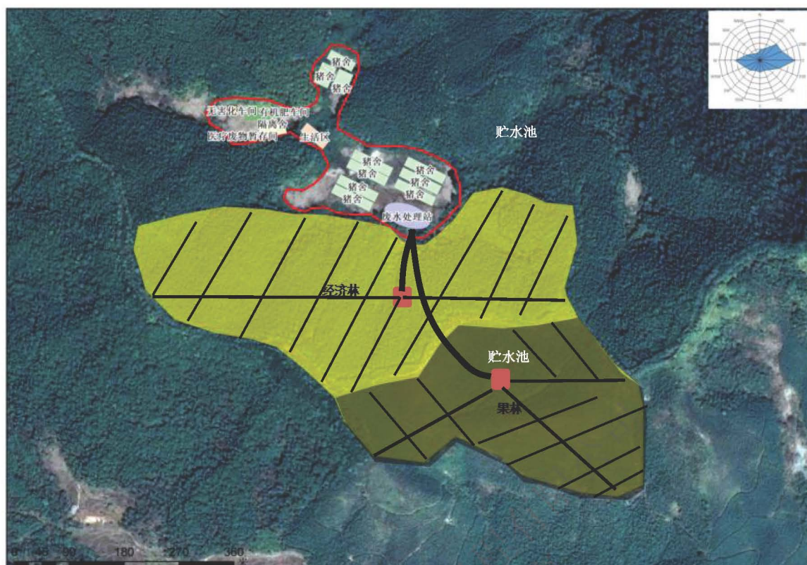
图 6-2 灌溉管网布置示意图
