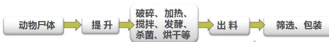
图 3-10 病死猪只无害化处理工艺
