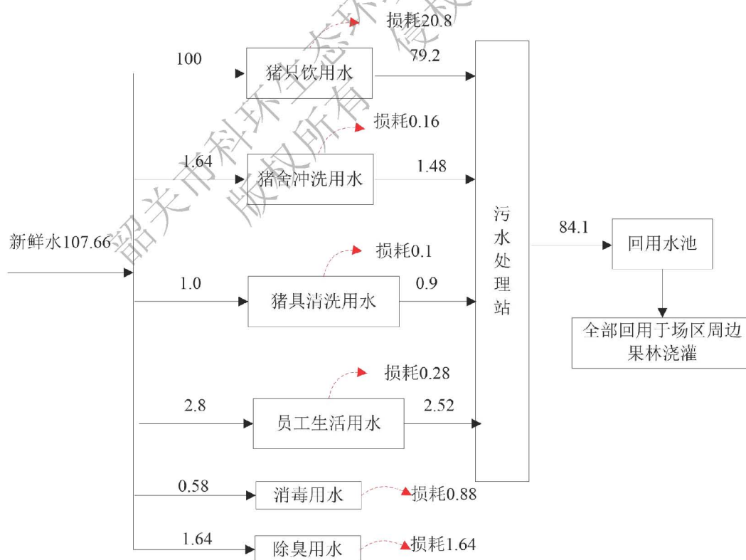
图 3-4 其它季节项目水平衡图 (单位: \text{m}^3/\text{d} )
