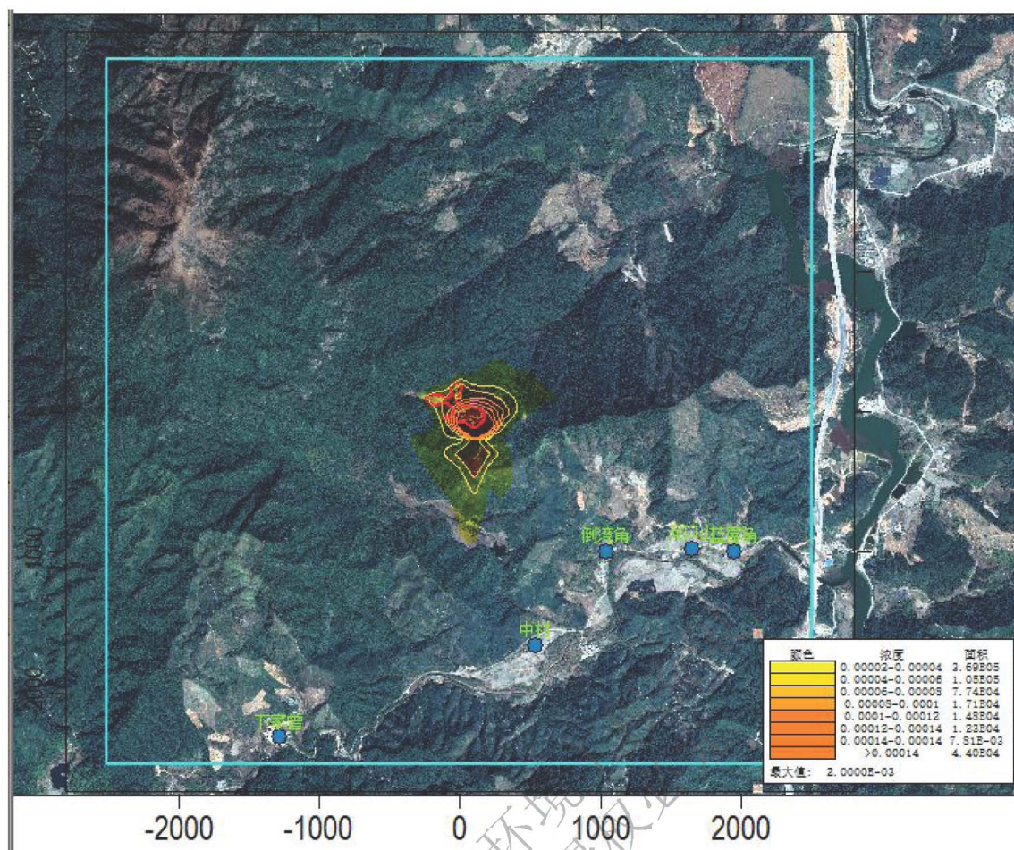
图 5-14 正常工况 PM_{10} 日均浓度贡献值分布图 ( mg/m^3 )
