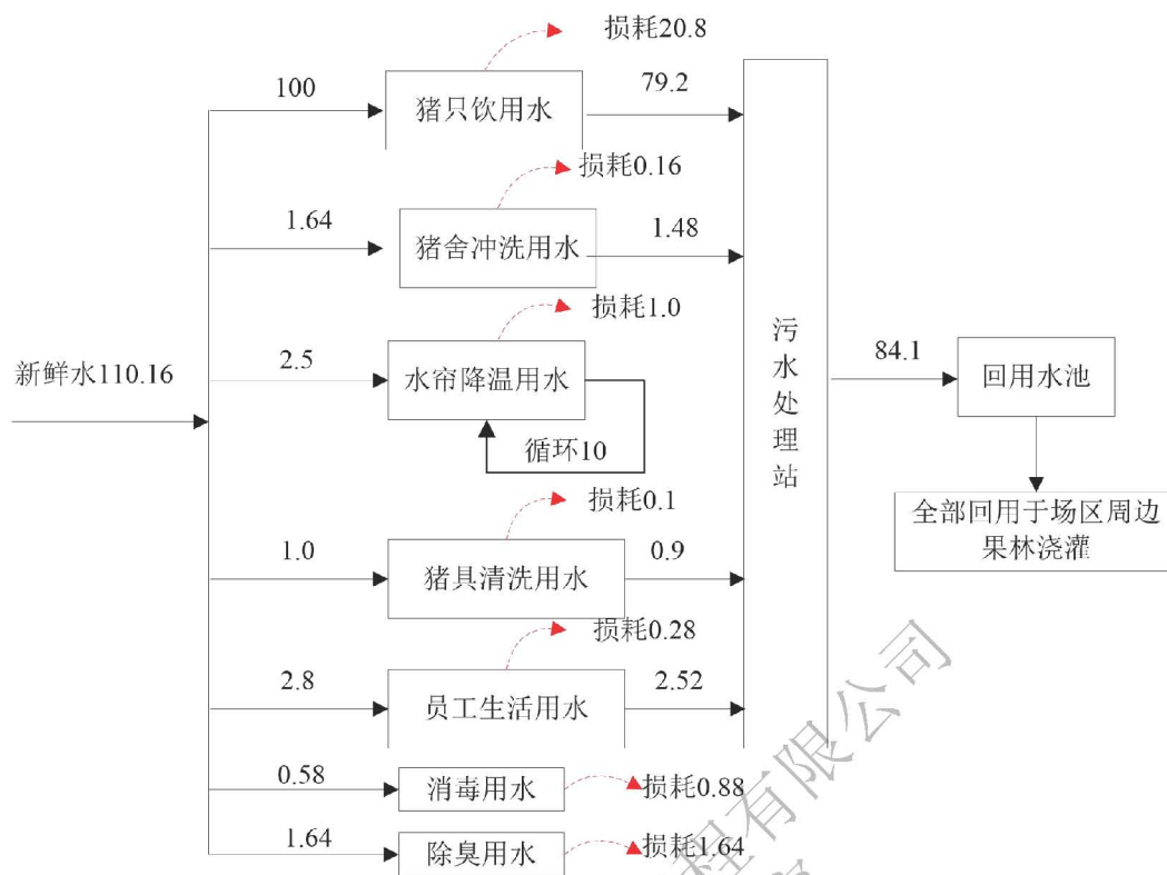
图 3-4 夏季项目水平衡图 (单位: \text{m}^3/\text{d} )
