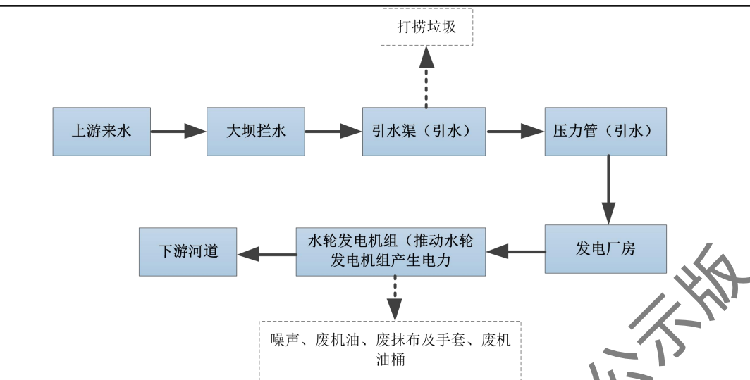
图 2-1 发电厂房工艺流程图
