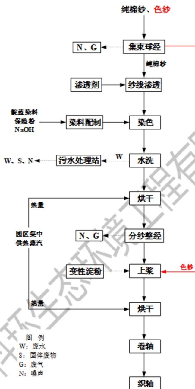
图2-3 升级改造后绳状浆染工艺流程及产污环节图
