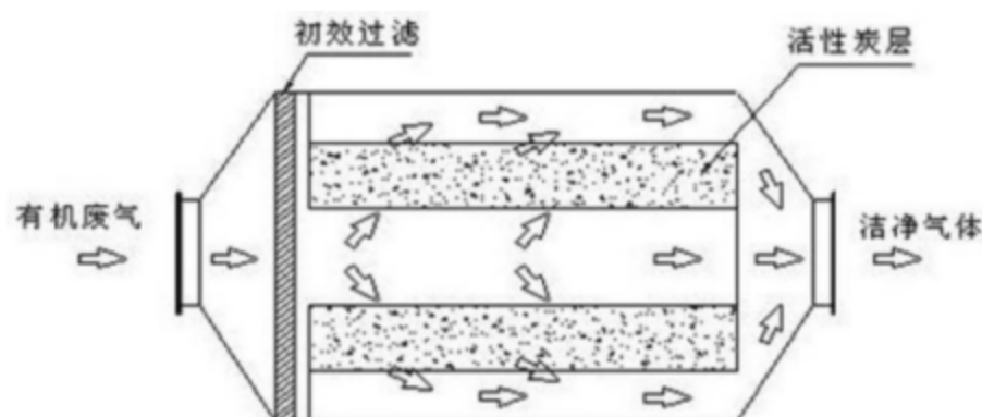
图 4-1 活性炭吸附工作原理图
