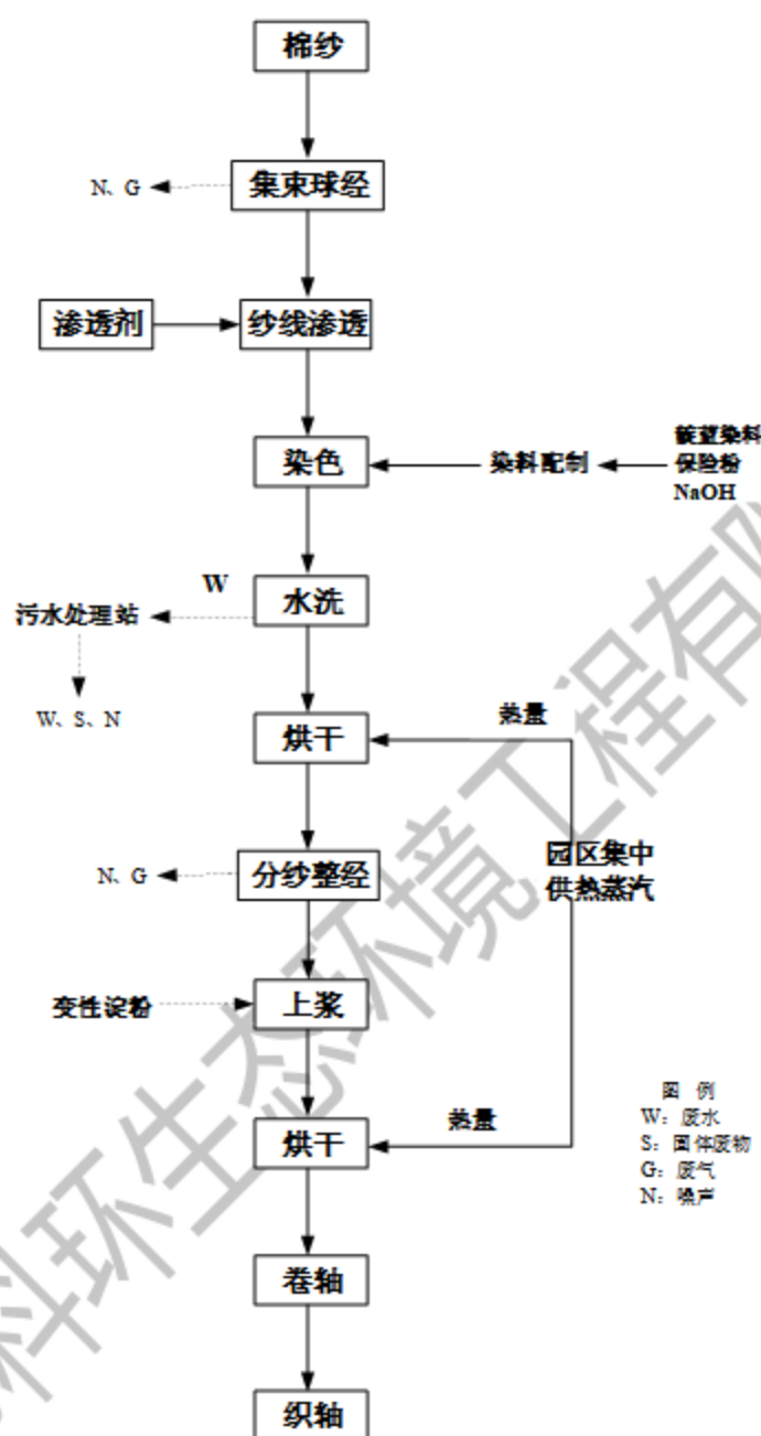
图 2-5 绳状浆染生产线生产工艺流程与产污节点图
