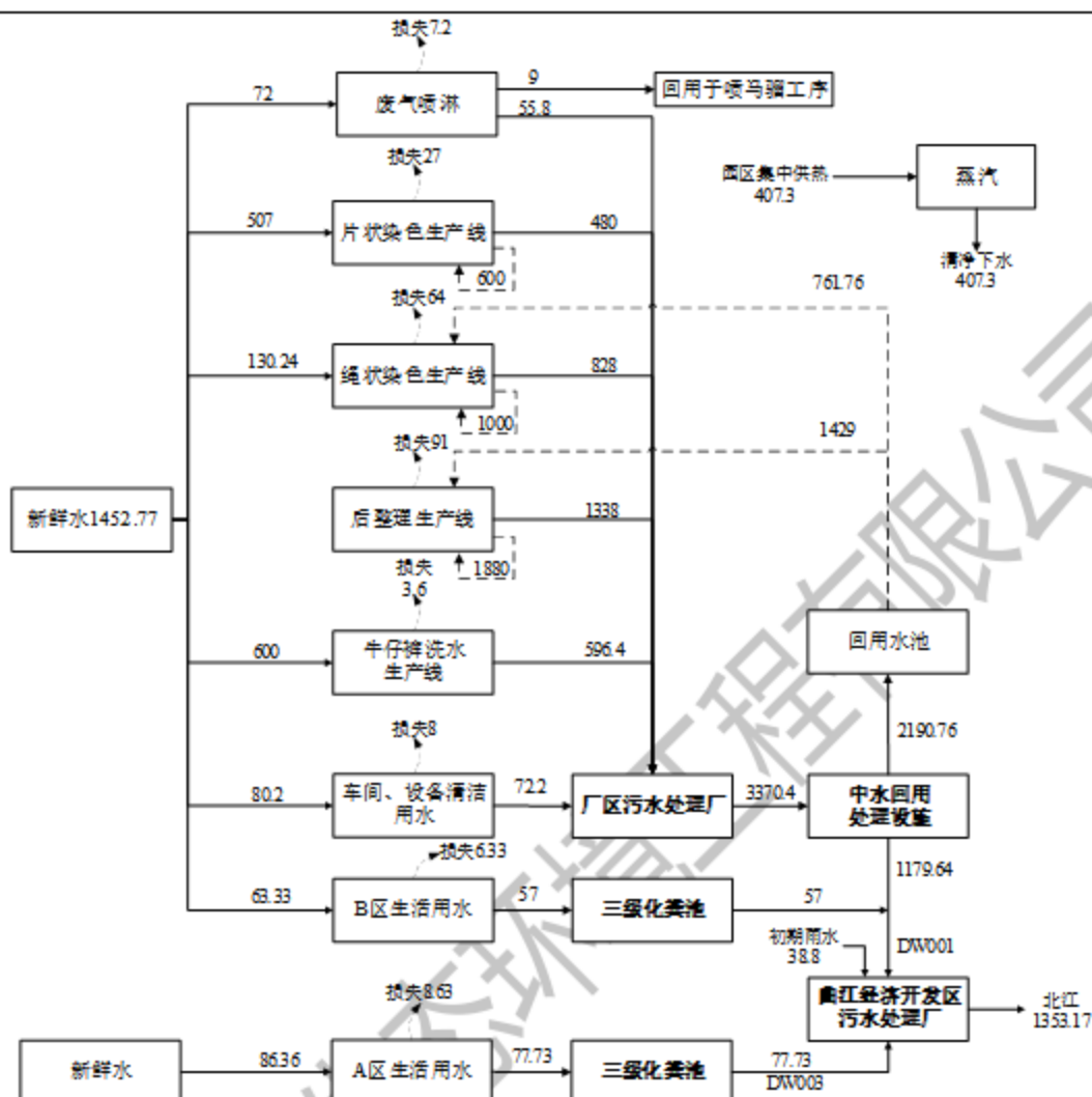
图2-8 现有项目水量平衡图 (m³/d)
