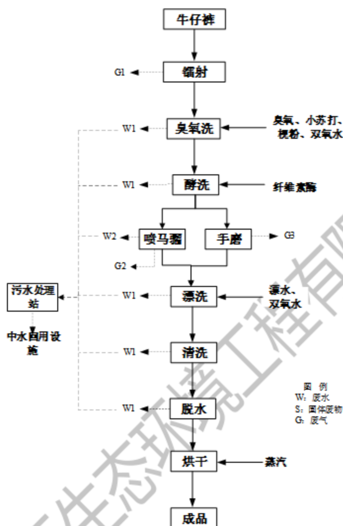
图 2-7 牛仔褲水洗生產線工藝流程與產污節點圖
